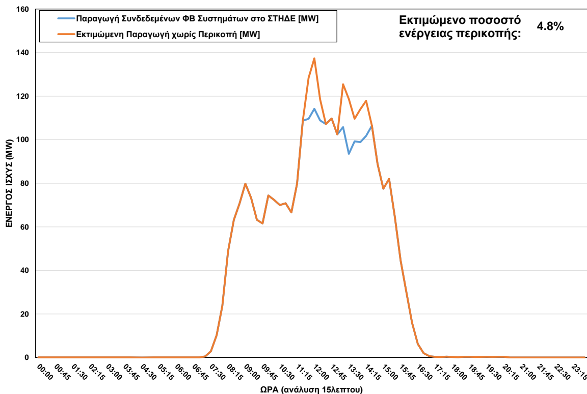
ΦΒ Παραγωγή στο ΣΤΗΔΕ στις 10/01/2024 (ώρα περικοπής: 11:45 - 14:15)
