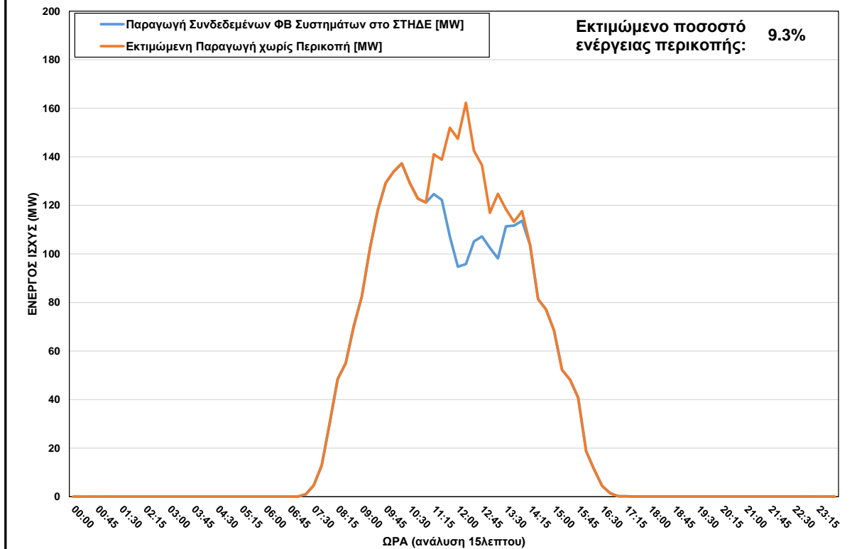
ΦΒ Παραγωγή στο ΣΤΗΔΕ στις 09/01/2024 (ώρα περικοπής: 11:15 - 14:00)
