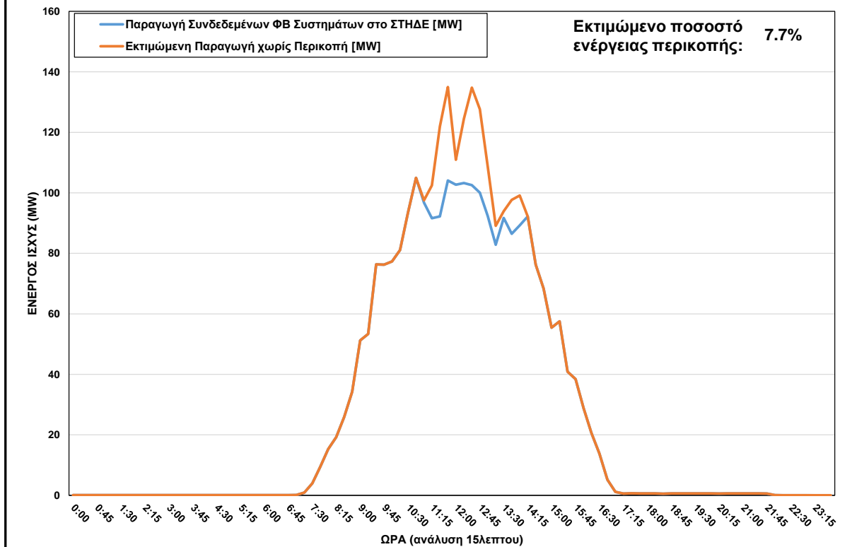
ΦΒ Παραγωγή στο ΣΤΗΔΕ στις 16/01/2024 (ώρα περικοπής: 11:00 - 14:00)
