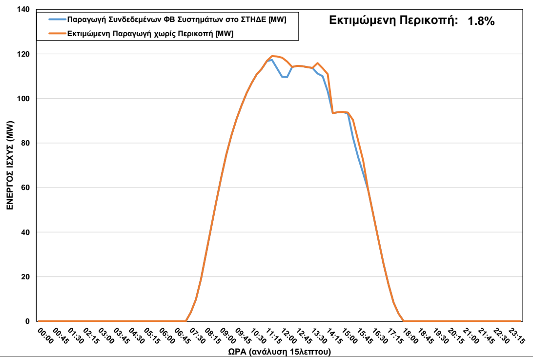
ΦΒ Παραγωγή στο ΣΤΗΔΕ κατά τη διάρκεια περικοπής στις 29/10/2022 ώρα 11:15 – 16:00
