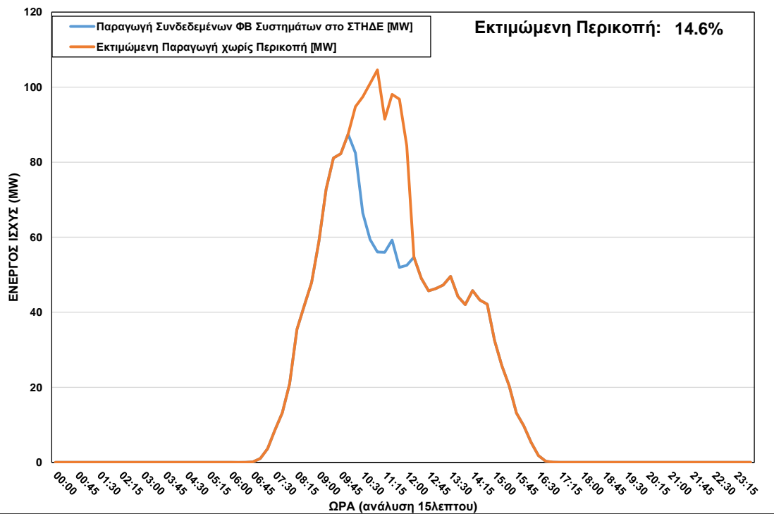
ΦΒ Παραγωγή στο ΣΤΗΔΕ κατά τη διάρκεια περικοπής στις 22/11/2022 ώρα 10:15 – 12:00
