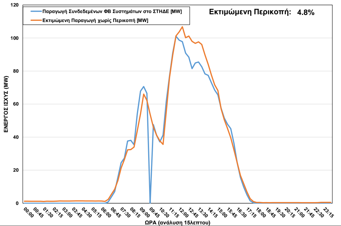
ΦΒ Παραγωγή στο ΣΤΗΔΕ κατά τη διάρκεια περικοπής στις 03/03/2022 ώρα 12:00 – 15:00
