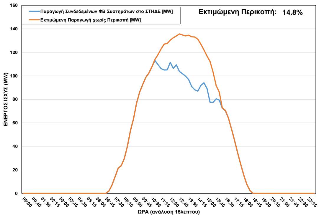
ΦΒ Παραγωγή στο ΣΤΗΔΕ κατά τη διάρκεια περικοπής στις 24/09/2022 ώρα 09:45 – 16:30
