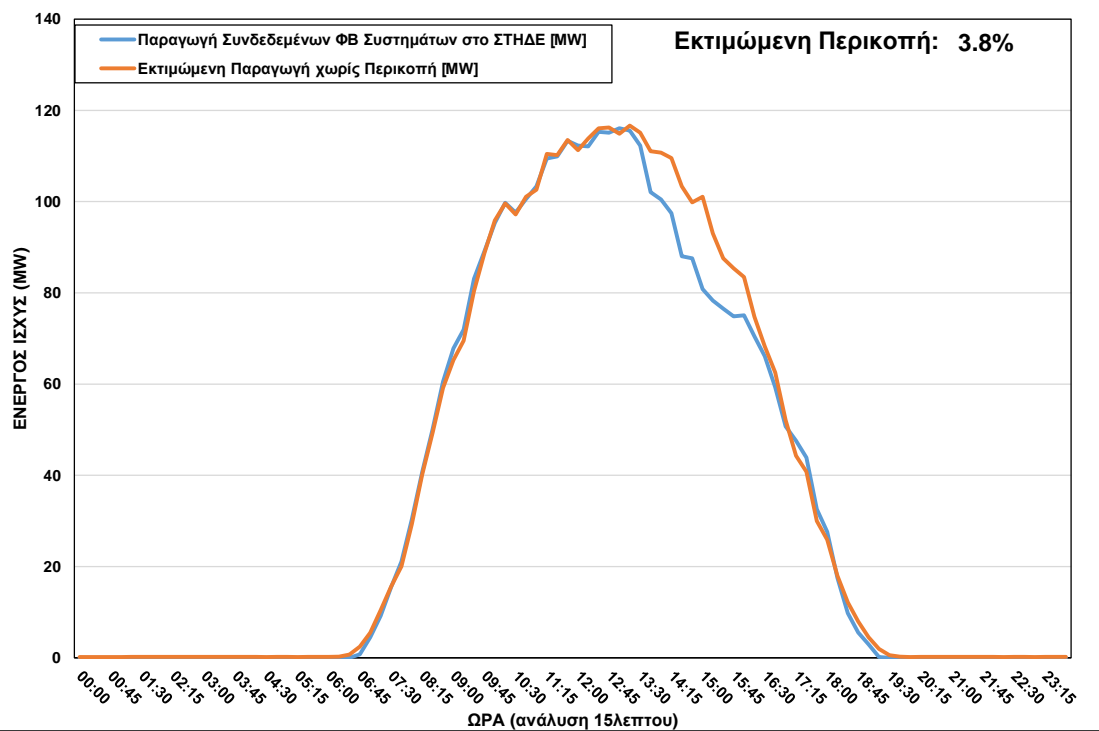
ΦΒ Παραγωγή στο ΣΤΗΔΕ κατά τη διάρκεια περικοπής στις 19/04/2022 ώρα 13:00 – 17:00
