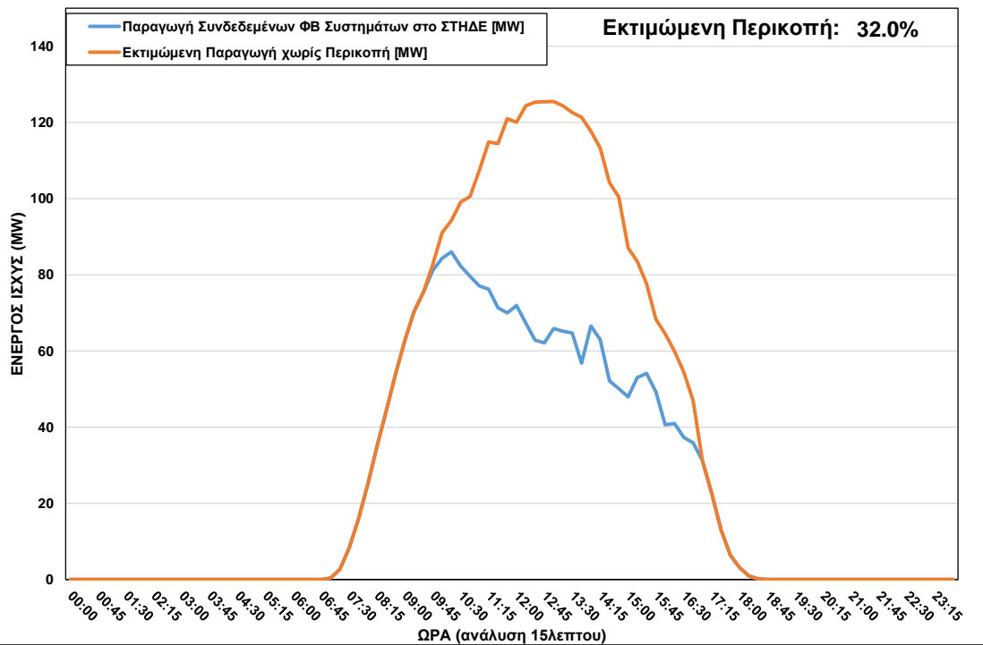
ΦΒ Παραγωγή στο ΣΤΗΔΕ κατά τη διάρκεια περικοπής στις 09/10/2022 ώρα 09:45 – 16:45
