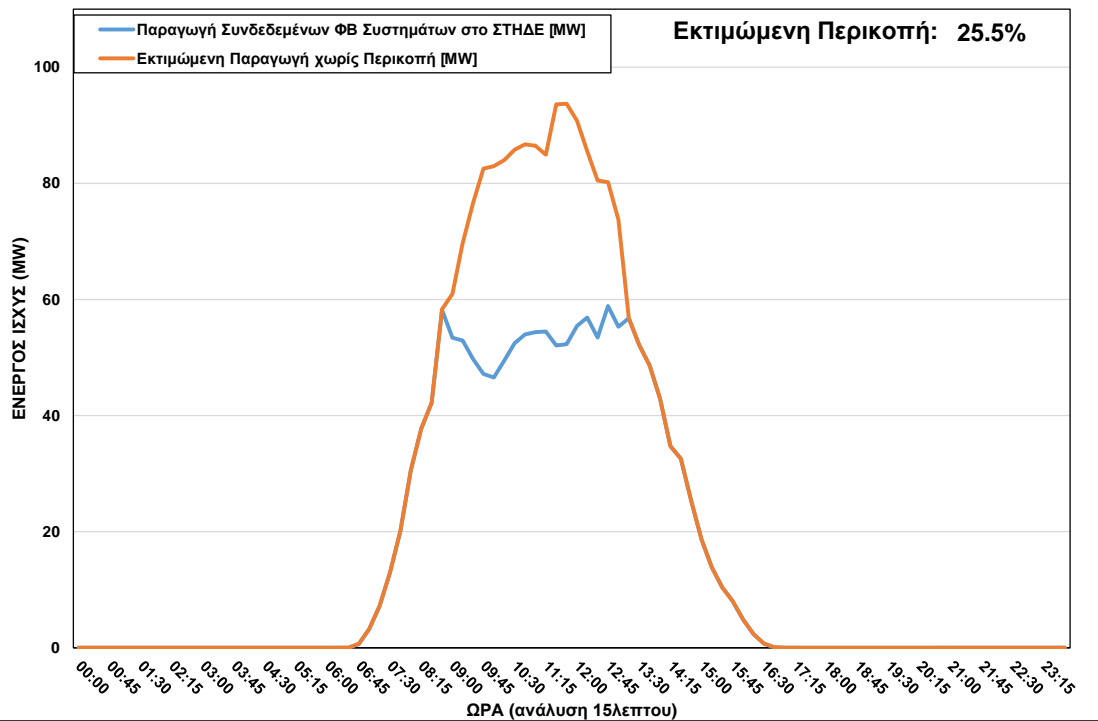
ΦΒ Παραγωγή στο ΣΤΗΔΕ κατά τη διάρκεια περικοπής στις 21/11/2022 ώρα 08:45 – 13:00
