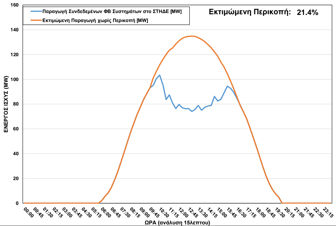
ΦΒ Παραγωγή στο ΣΤΗΔΕ κατά τη διάρκεια περικοπής στις 26/06/2022 ώρα 10:00 – 16:45
