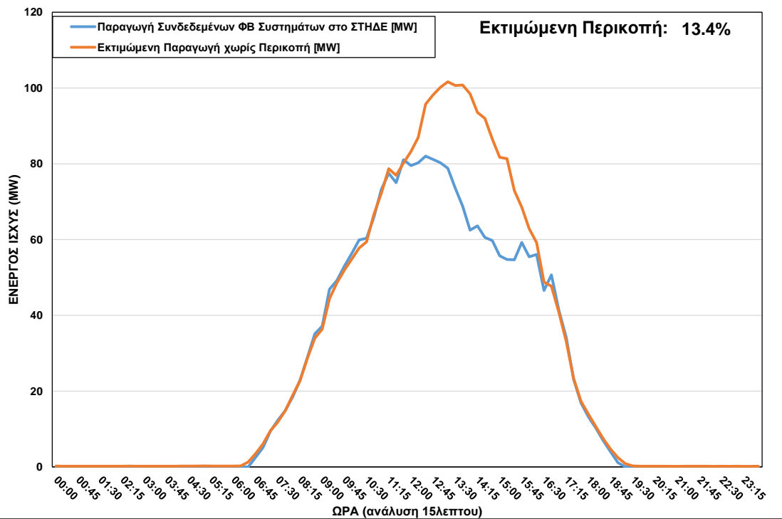
ΦΒ Παραγωγή στο ΣΤΗΔΕ κατά τη διάρκεια περικοπής στις 17/04/2022 ώρα 11:15 – 16:30
