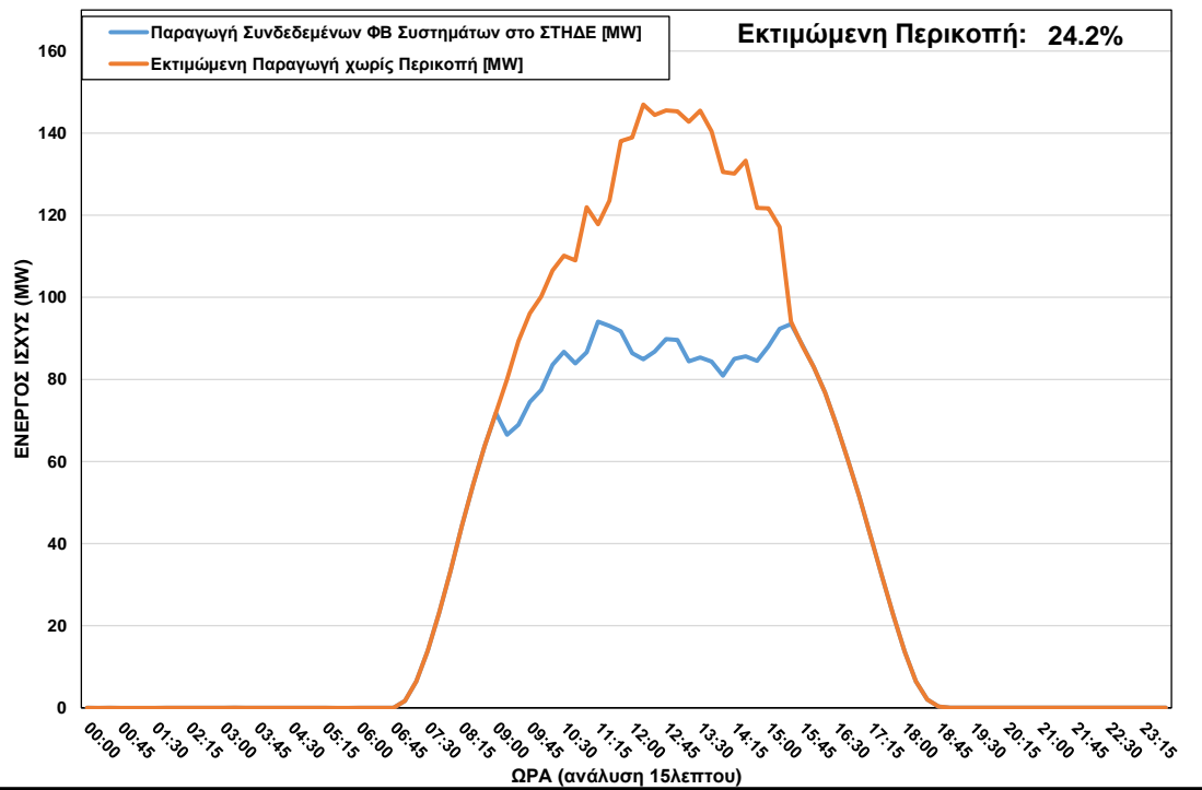
ΦΒ Παραγωγή στο ΣΤΗΔΕ κατά τη διάρκεια περικοπής στις 25/09/2022 ώρα 09:00 – 15:45
