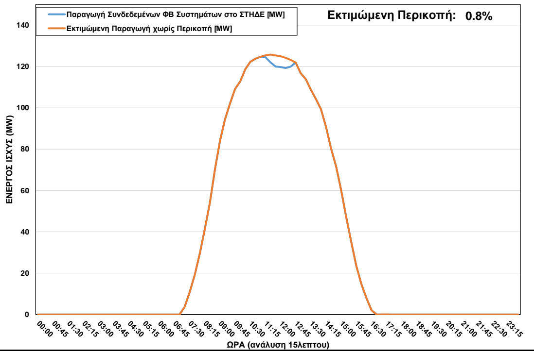
ΦΒ Παραγωγή στο ΣΤΗΔΕ κατά τη διάρκεια περικοπής στις 17/12/2022 ώρα 11:15 – 12:30
