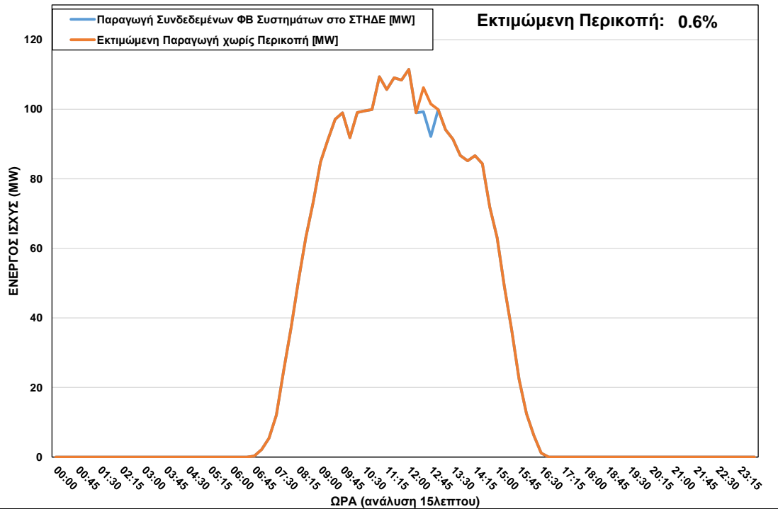
ΦΒ Παραγωγή στο ΣΤΗΔΕ κατά τη διάρκεια περικοπής στις 01/12/2022 ώρα 12:30 – 12:45
