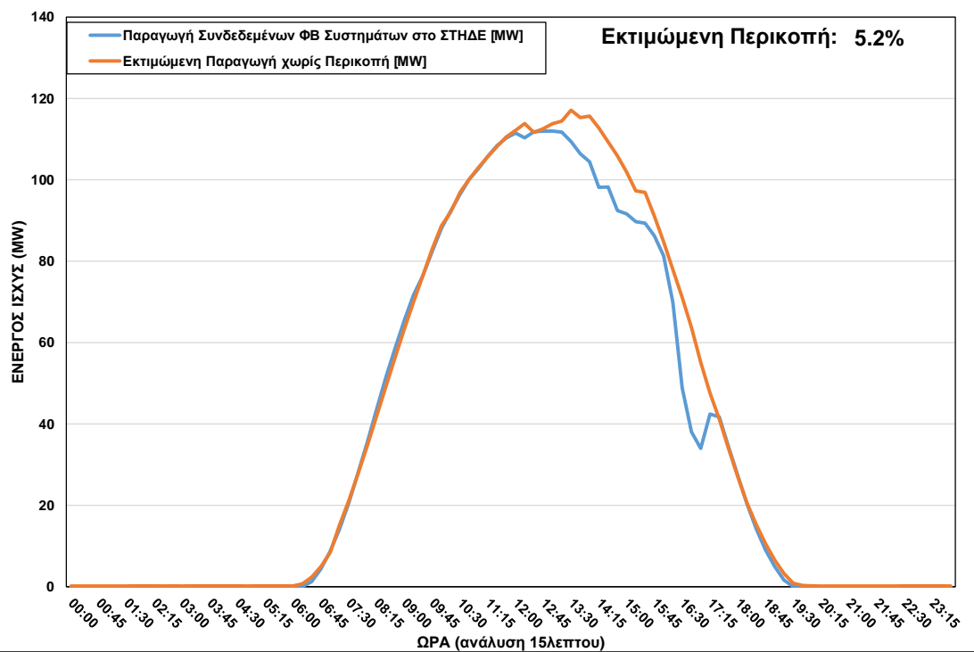
ΦΒ Παραγωγή στο ΣΤΗΔΕ κατά τη διάρκεια περικοπής στις 25/04/2022 ώρα 12:00 – 18:00
