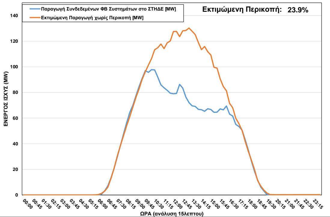
ΦΒ Παραγωγή στο ΣΤΗΔΕ κατά τη διάρκεια περικοπής στις 06/05/2022 ώρα 09:45 – 17:30
