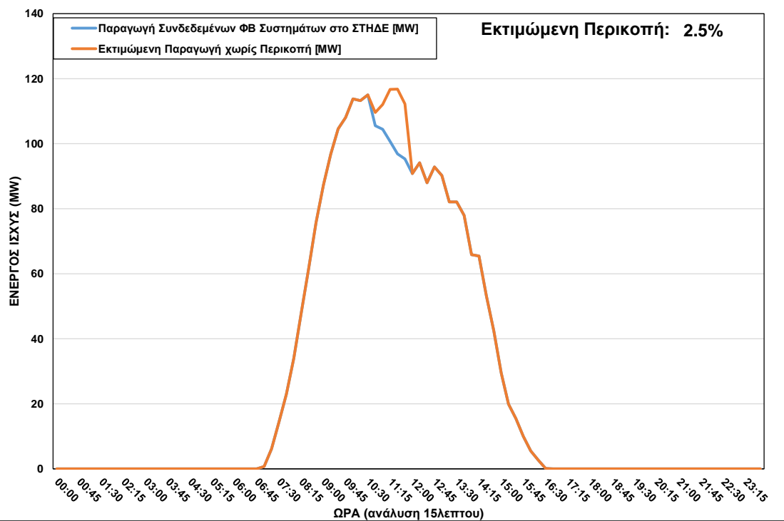
ΦΒ Παραγωγή στο ΣΤΗΔΕ κατά τη διάρκεια περικοπής στις 06/12/2022 ώρα 10:45 – 11:45
