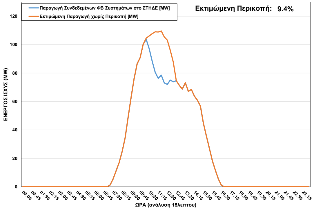
ΦΒ Παραγωγή στο ΣΤΗΔΕ κατά τη διάρκεια περικοπής στις 22/12/2022 ώρα 10:00 – 12:30
