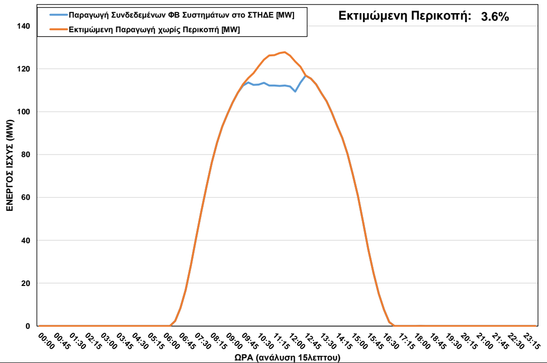
ΦΒ Παραγωγή στο ΣΤΗΔΕ κατά τη διάρκεια περικοπής στις 03/11/2022 ώρα 09:45 – 12:30
