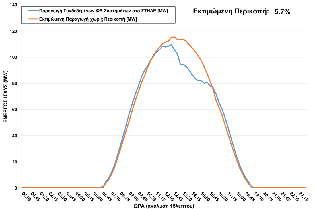
ΦΒ Παραγωγή στο ΣΤΗΔΕ κατά τη διάρκεια περικοπής στις 06/04/2022 ώρα 11:30 – 17:00
