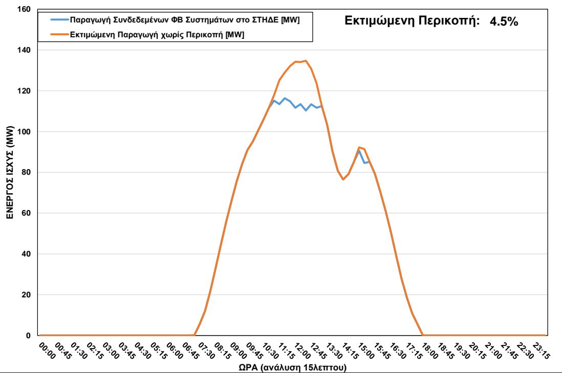
ΦΒ Παραγωγή στο ΣΤΗΔΕ κατά τη διάρκεια περικοπής στις 25/10/2022 ώρα 11:00 – 15:15
