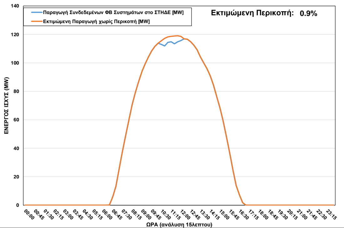
ΦΒ Παραγωγή στο ΣΤΗΔΕ κατά τη διάρκεια περικοπής στις 02/11/2022 ώρα 10:30 – 11:45
