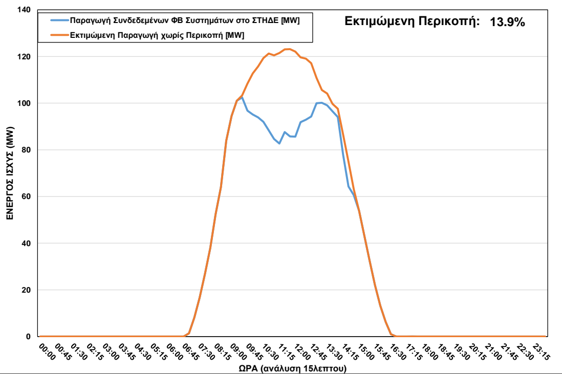
ΦΒ Παραγωγή στο ΣΤΗΔΕ κατά τη διάρκεια περικοπής στις 04/12/2022 ώρα 09:30 – 14:45
