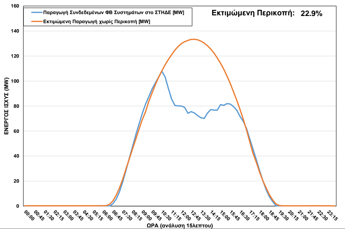
ΦΒ Παραγωγή στο ΣΤΗΔΕ κατά τη διάρκεια περικοπής στις 14/04/2022 ώρα 10:30 – 16:45
