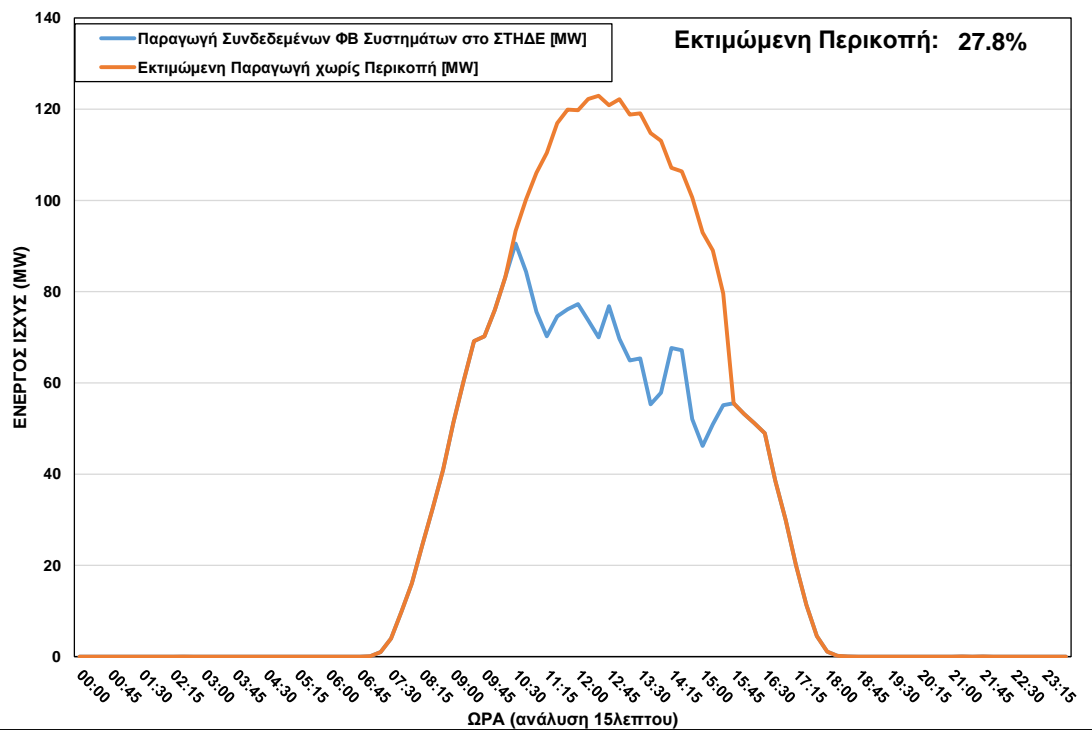
ΦΒ Παραγωγή στο ΣΤΗΔΕ κατά τη διάρκεια περικοπής στις 18/10/2022 ώρα 10:30 – 15:30
