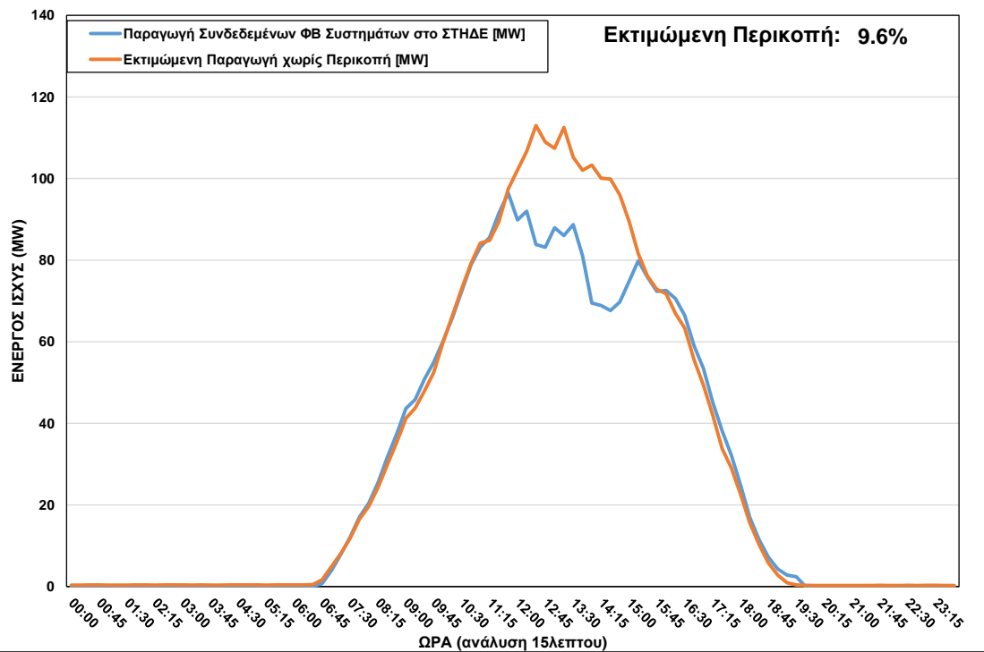
ΦΒ Παραγωγή στο ΣΤΗΔΕ κατά τη διάρκεια περικοπής στις 05/04/2022 ώρα 11:30 – 17:00
