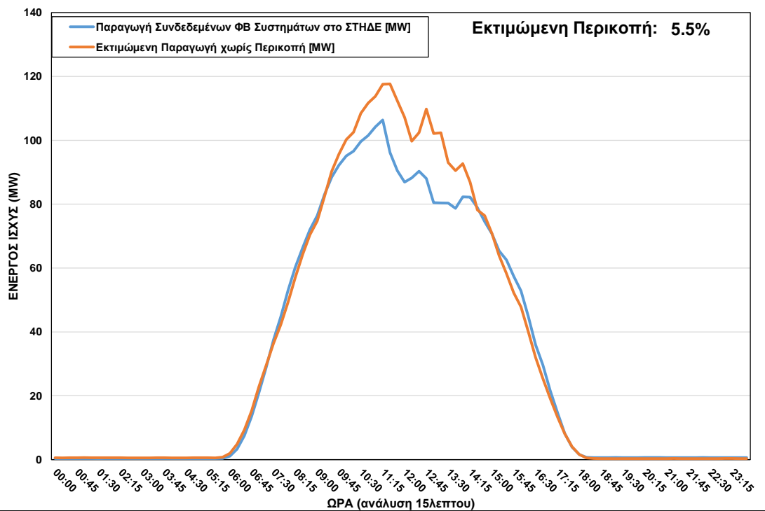
ΦΒ Παραγωγή στο ΣΤΗΔΕ κατά τη διάρκεια περικοπής στις 26/03/2022 ώρα 11:15 – 13:30
