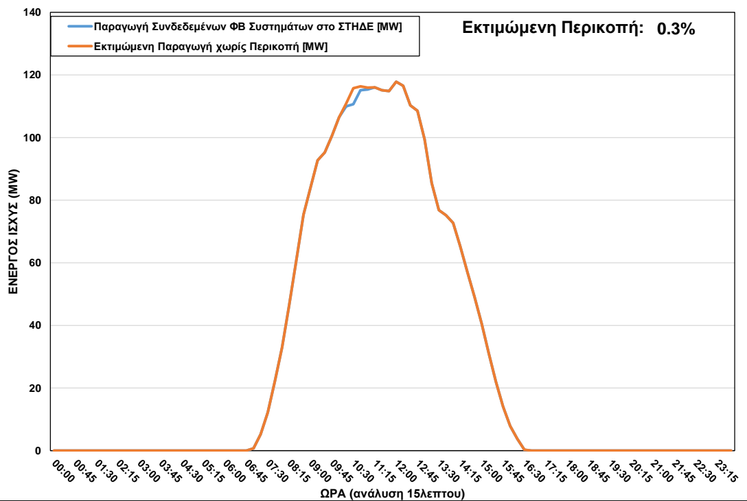
ΦΒ Παραγωγή στο ΣΤΗΔΕ κατά τη διάρκεια περικοπής στις 08/12/2022 ώρα 10:15 – 11:00
