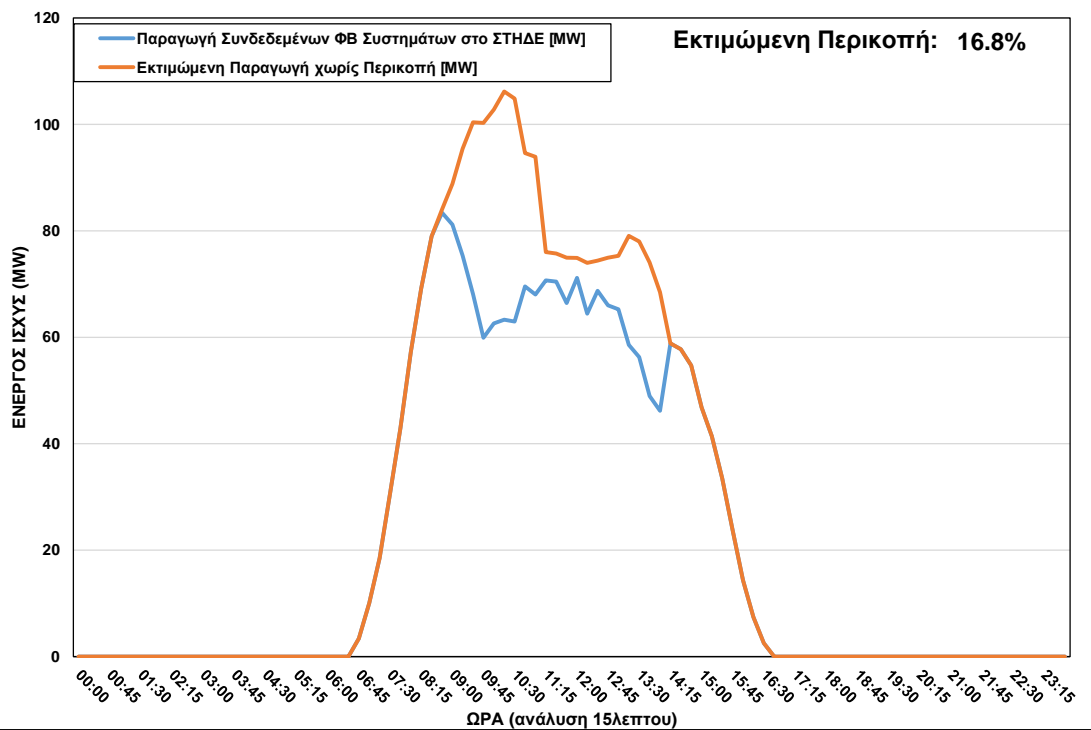
ΦΒ Παραγωγή στο ΣΤΗΔΕ κατά τη διάρκεια περικοπής στις 08/11/2022 ώρα 08:45 – 14:00
