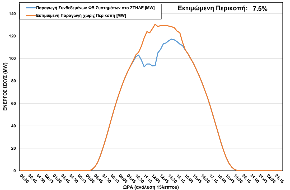
ΦΒ Παραγωγή στο ΣΤΗΔΕ κατά τη διάρκεια περικοπής στις 13/08/2022 ώρα 10:00 – 15:00
