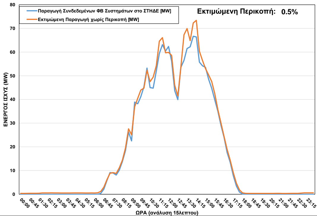
ΦΒ Παραγωγή στο ΣΤΗΔΕ κατά τη διάρκεια περικοπής στις 06/03/2022 ώρα 15:00 – 16:15
