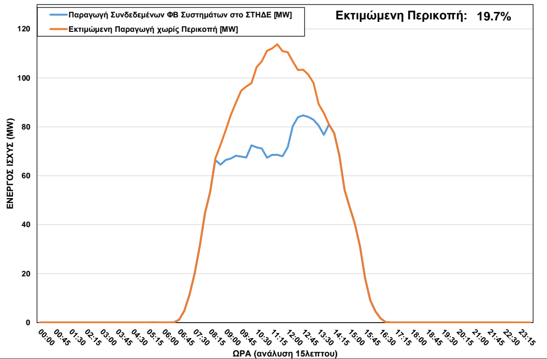
ΦΒ Παραγωγή στο ΣΤΗΔΕ κατά τη διάρκεια περικοπής στις 20/11/2022 ώρα 08:30 – 13:45
