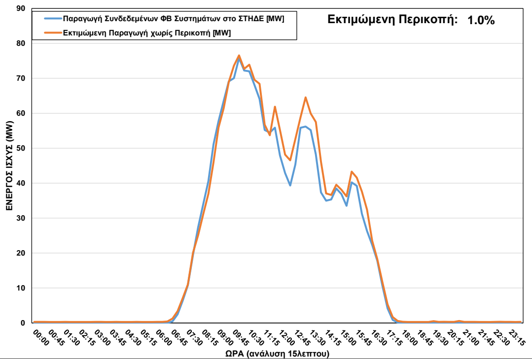
ΦΒ Παραγωγή στο ΣΤΗΔΕ κατά τη διάρκεια περικοπής στις 24/02/2022 ώρα 15:15 – 16:30
