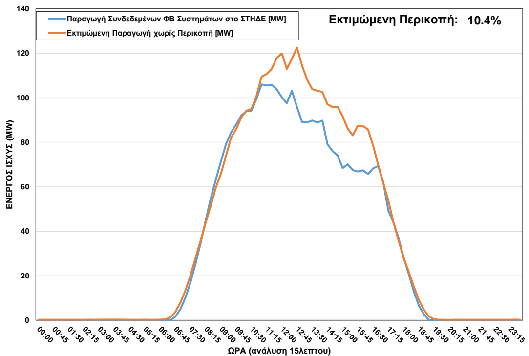
ΦΒ Παραγωγή στο ΣΤΗΔΕ κατά τη διάρκεια περικοπής στις 12/04/2022 ώρα 11:00 – 18:00
