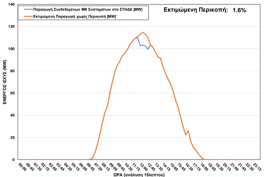
ΦΒ Παραγωγή στο ΣΤΗΔΕ κατά τη διάρκεια περικοπής στις 15/10/2022 ώρα 11:45 – 12:45
