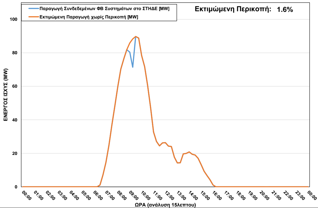
ΦΒ Παραγωγή στο ΣΤΗΔΕ κατά τη διάρκεια περικοπής στις 07/11/2022 ώρα 09:00 – 09:15
