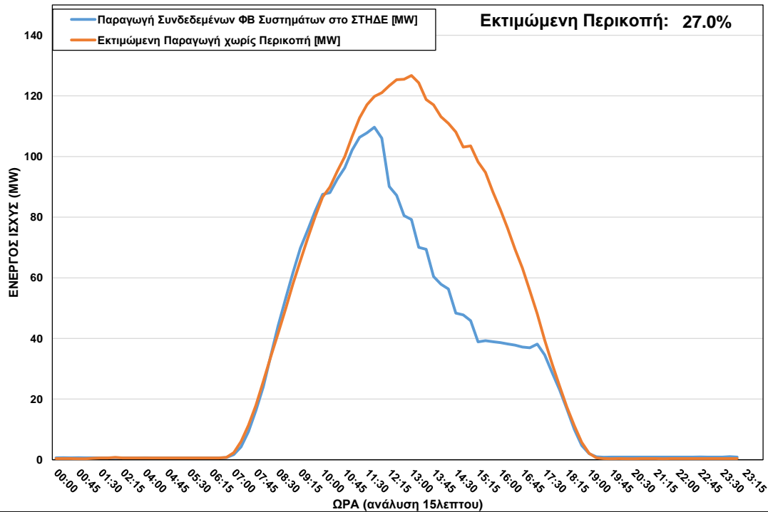
ΦΒ Παραγωγή στο ΣΤΗΔΕ κατά τη διάρκεια περικοπής στις 27/03/2022 ώρα 11:45 – 18:15
