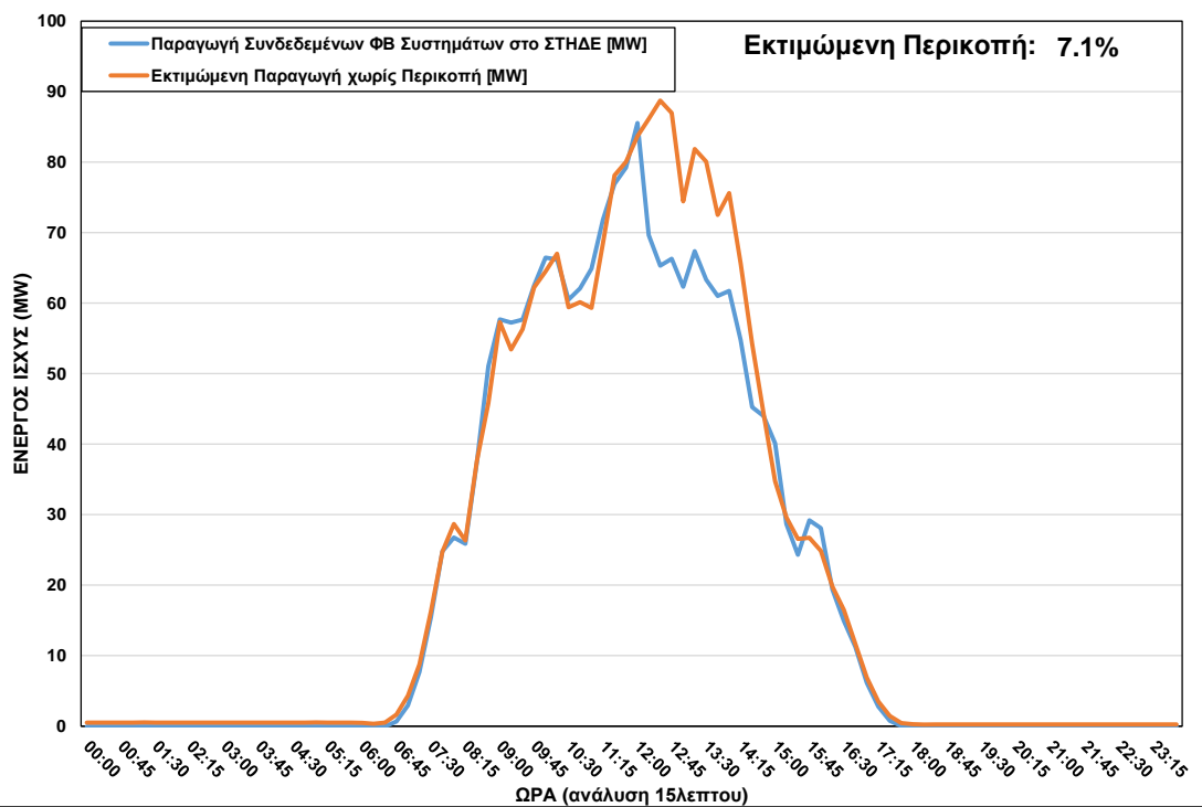
ΦΒ Παραγωγή στο ΣΤΗΔΕ κατά τη διάρκεια περικοπής στις 21/02/2022 ώρα 11:45 – 14:30
