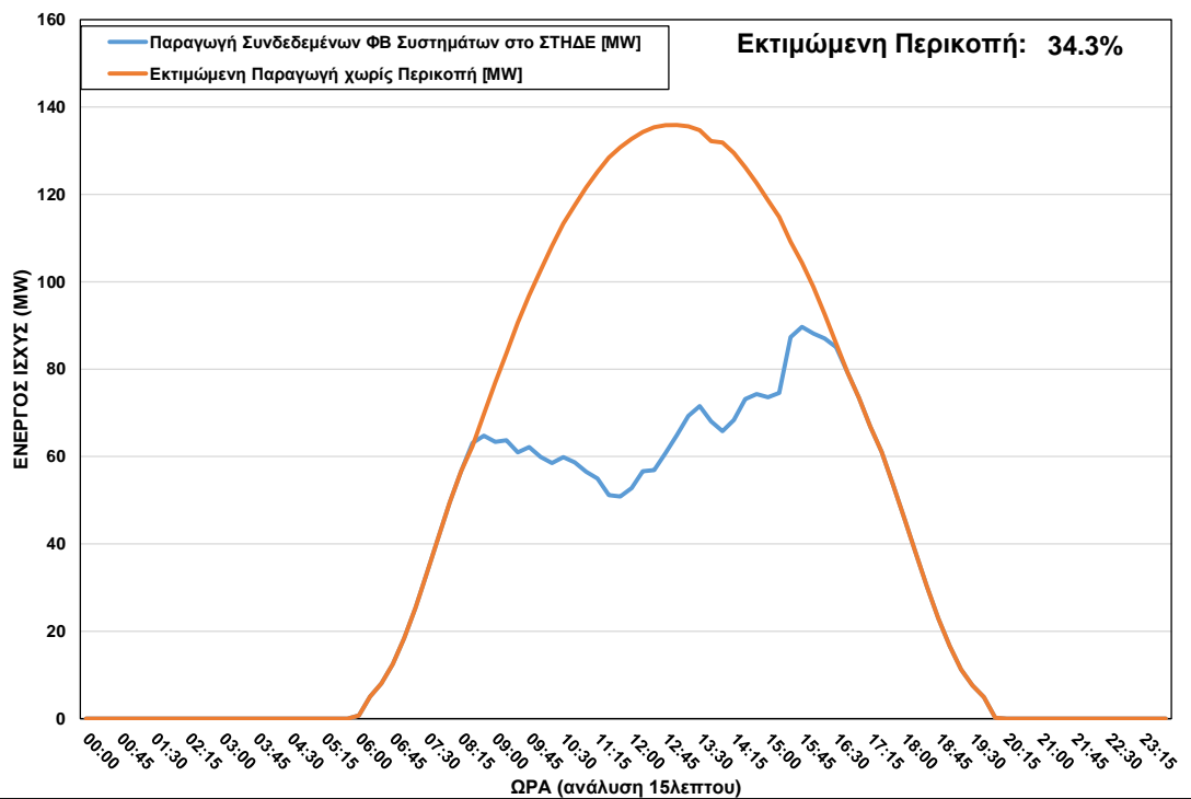
ΦΒ Παραγωγή στο ΣΤΗΔΕ κατά τη διάρκεια περικοπής στις 25/06/2022 ώρα 08:30 – 16:30
