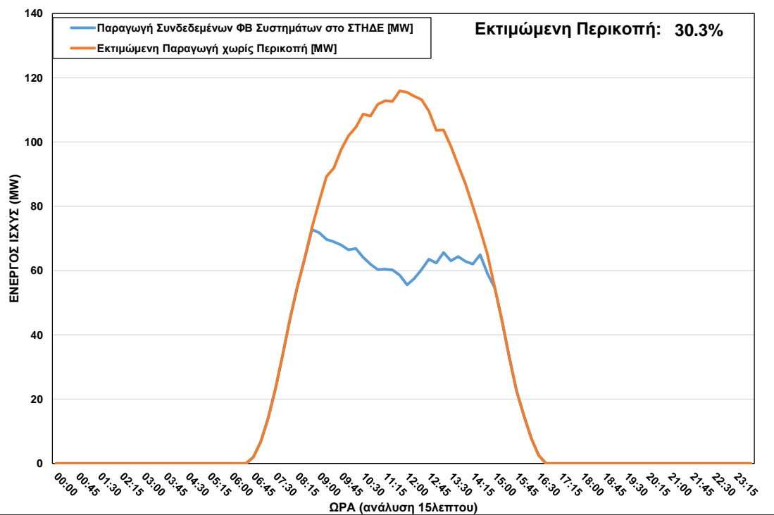
ΦΒ Παραγωγή στο ΣΤΗΔΕ κατά τη διάρκεια περικοπής στις 13/11/2022 ώρα 08:45 – 14:45
