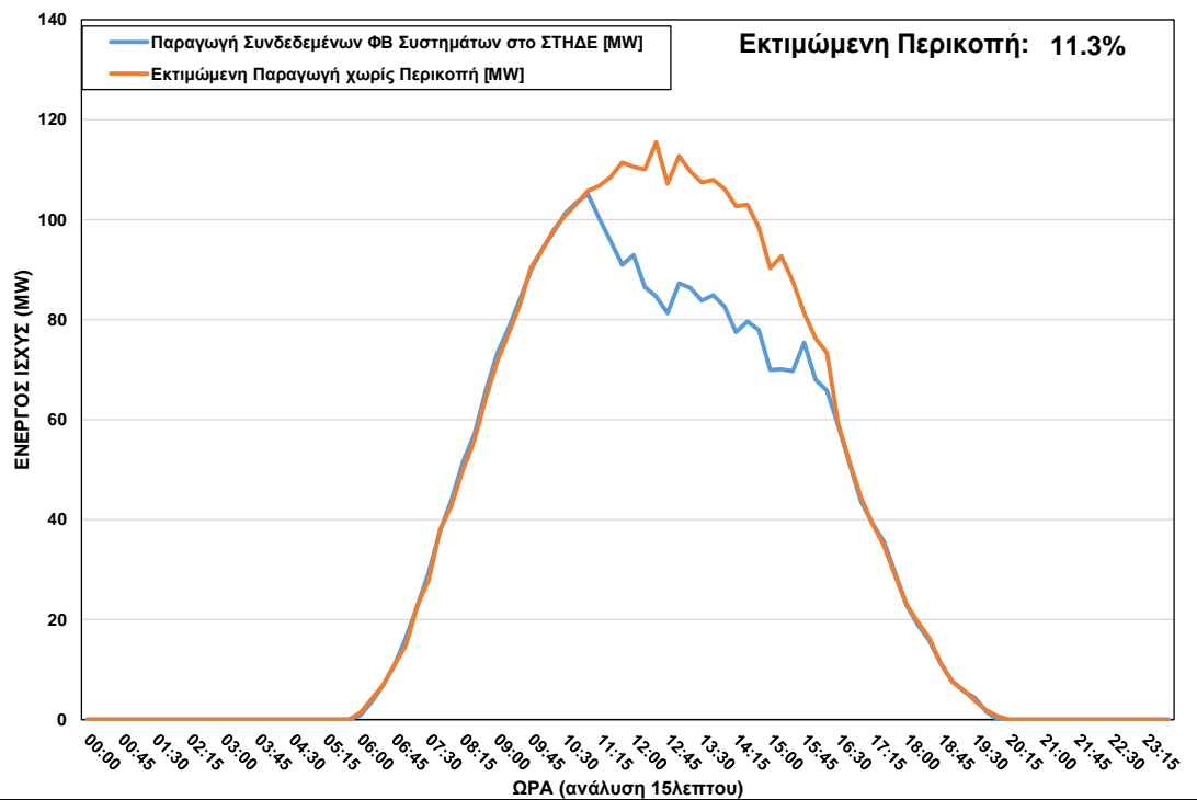
ΦΒ Παραγωγή στο ΣΤΗΔΕ κατά τη διάρκεια περικοπής στις 13/06/2022 ώρα 10:30 – 16:15
