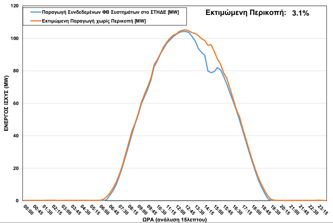
ΦΒ Παραγωγή στο ΣΤΗΔΕ κατά τη διάρκεια περικοπής στις 24/04/2022 ώρα 12:15 – 16:30
