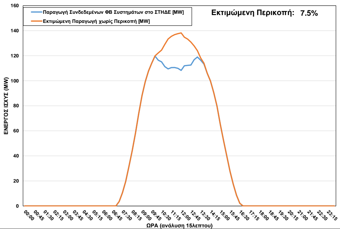
ΦΒ Παραγωγή στο ΣΤΗΔΕ κατά τη διάρκεια περικοπής στις 18/12/2022 ώρα 10:00 – 13:45
