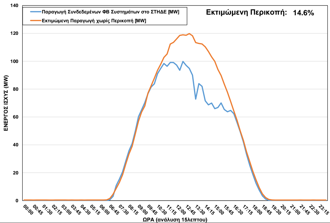
ΦΒ Παραγωγή στο ΣΤΗΔΕ κατά τη διάρκεια περικοπής στις 02/04/2022 ώρα 10:45 – 16:30
