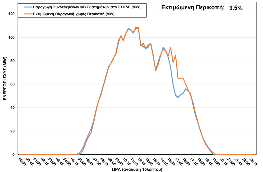
ΦΒ Παραγωγή στο ΣΤΗΔΕ κατά τη διάρκεια περικοπής στις 09/05/2022 ώρα 15:00 – 17:00
