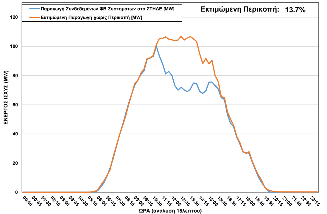
ΦΒ Παραγωγή στο ΣΤΗΔΕ κατά τη διάρκεια περικοπής στις 12/06/2022 ώρα 10:00 – 16:45
