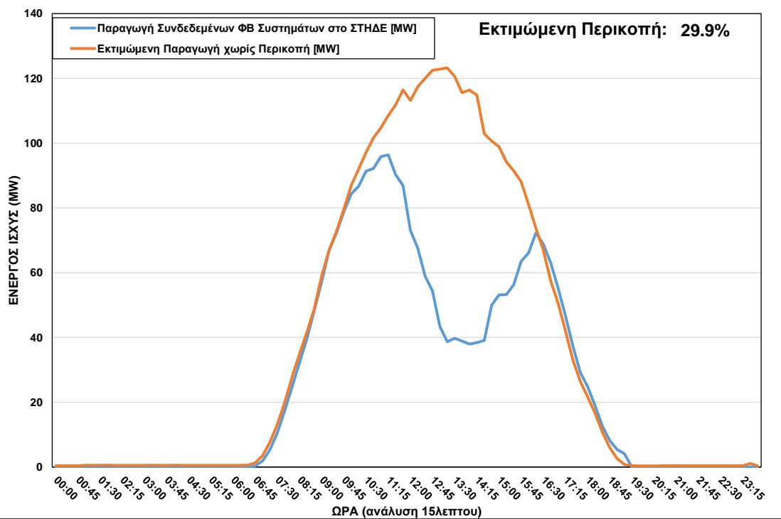
ΦΒ Παραγωγή στο ΣΤΗΔΕ κατά τη διάρκεια περικοπής στις 01/04/2022 ώρα 10:00 – 16:30
