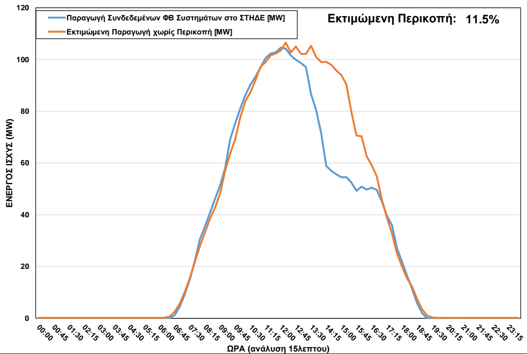
ΦΒ Παραγωγή στο ΣΤΗΔΕ κατά τη διάρκεια περικοπής στις 11/04/2022 ώρα 13:00 – 17:15
