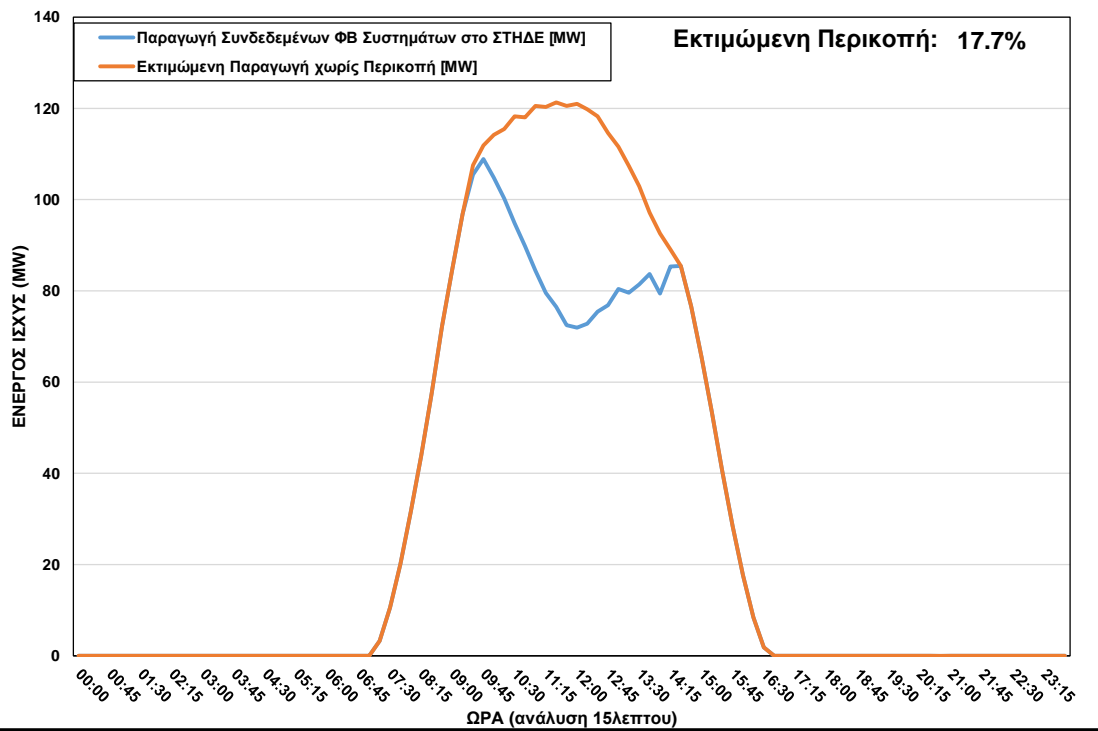
ΦΒ Παραγωγή στο ΣΤΗΔΕ κατά τη διάρκεια περικοπής στις 19/12/2022 ώρα 09:30 – 14:15
