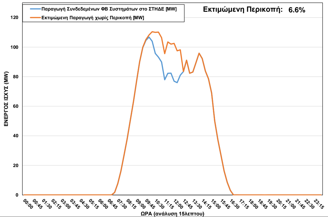
ΦΒ Παραγωγή στο ΣΤΗΔΕ κατά τη διάρκεια περικοπής στις 31/12/2022 ώρα 09:30 – 12:30
