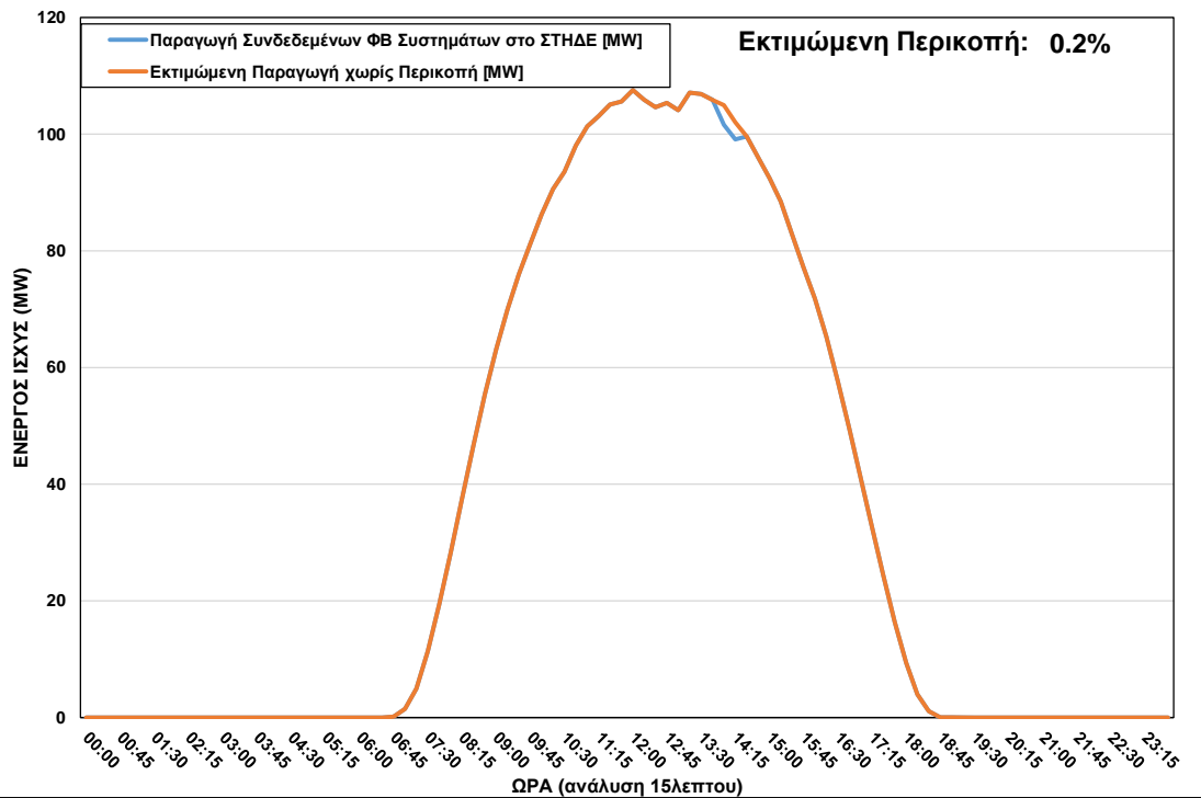
ΦΒ Παραγωγή στο ΣΤΗΔΕ κατά τη διάρκεια περικοπής στις 28/09/2022 ώρα 13:45 - 14:15
