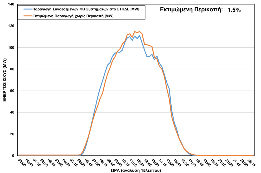
ΦΒ Παραγωγή στο ΣΤΗΔΕ κατά τη διάρκεια περικοπής στις 08/03/2022 ώρα 12:15 – 13:30
