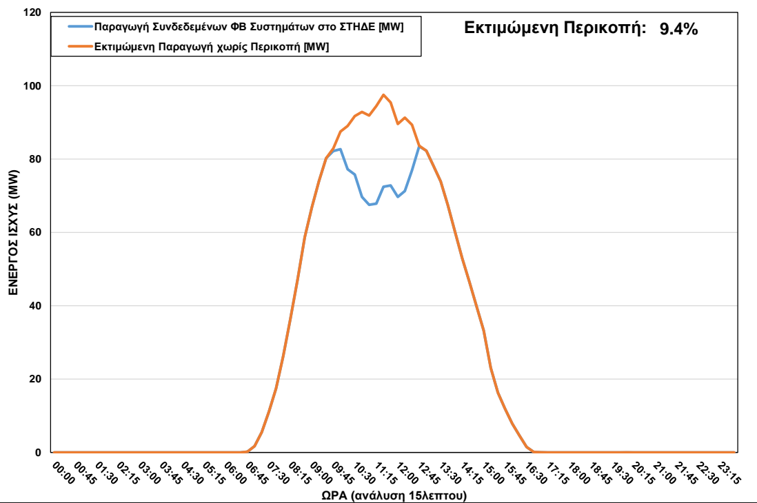
ΦΒ Παραγωγή στο ΣΤΗΔΕ κατά τη διάρκεια περικοπής στις 30/11/2022 ώρα 09:45 – 12:45
