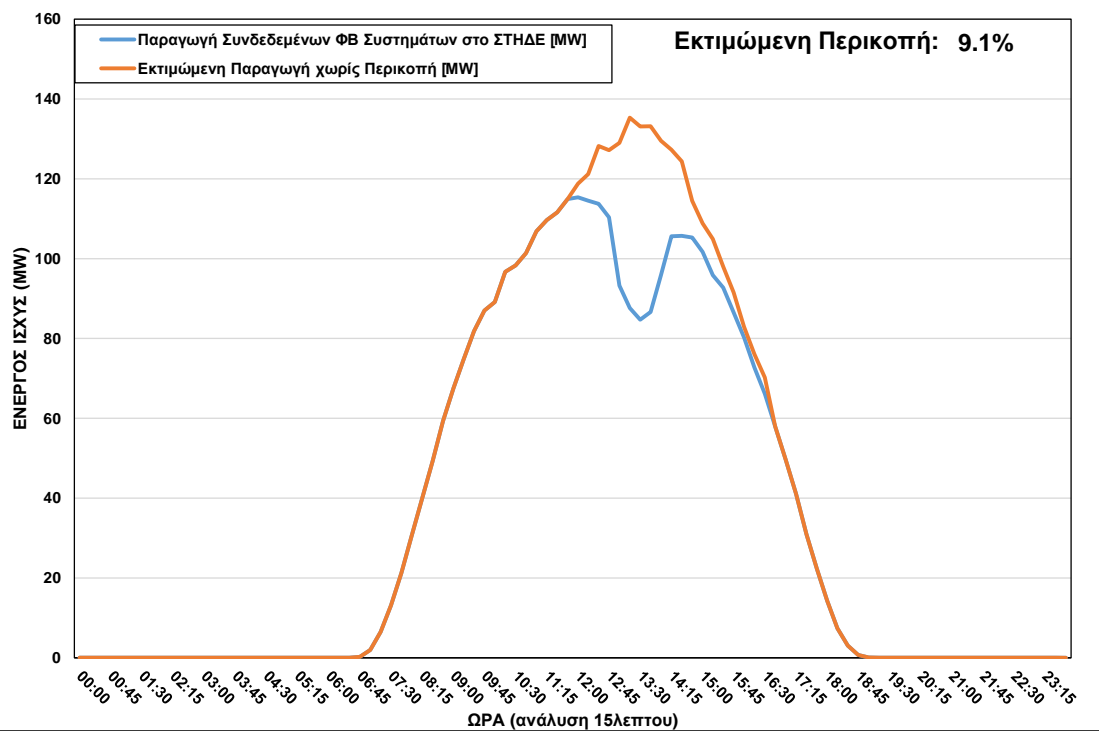
ΦΒ Παραγωγή στο ΣΤΗΔΕ κατά τη διάρκεια περικοπής στις 21/09/2022 ώρα 12:00 – 16:30
