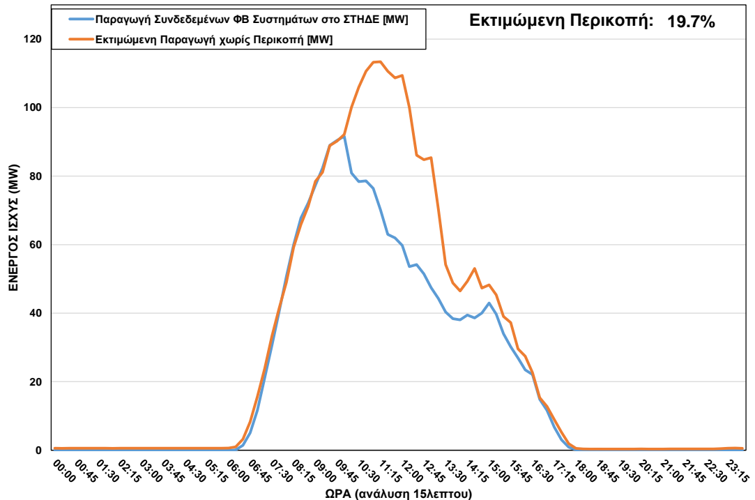
ΦΒ Παραγωγή στο ΣΤΗΔΕ κατά τη διάρκεια περικοπής στις 07/03/2022 ώρα 09:30 – 15:00
