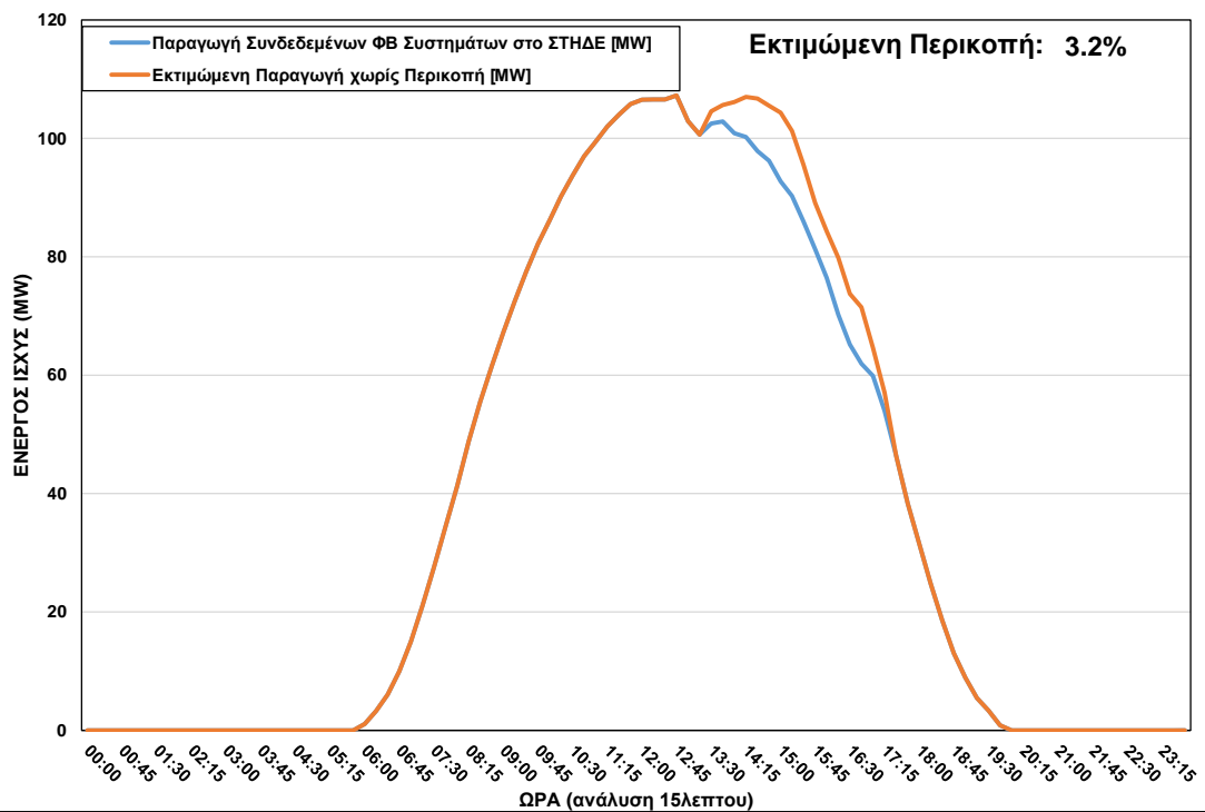
ΦΒ Παραγωγή στο ΣΤΗΔΕ κατά τη διάρκεια περικοπής στις 05/06/2022 ώρα 13:30 – 17:15
