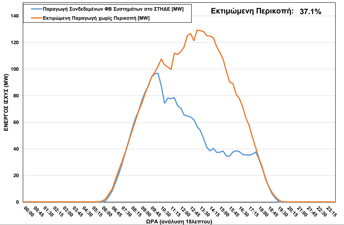
ΦΒ Παραγωγή στο ΣΤΗΔΕ κατά τη διάρκεια περικοπής στις 07/05/2022 ώρα 10:00 – 18:00
