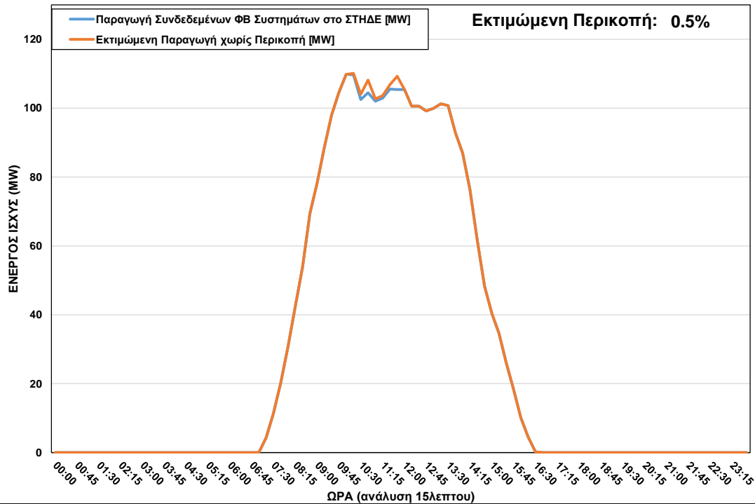
ΦΒ Παραγωγή στο ΣΤΗΔΕ κατά τη διάρκεια περικοπής στις 09/12/2022 ώρα 10:15 – 11:45
