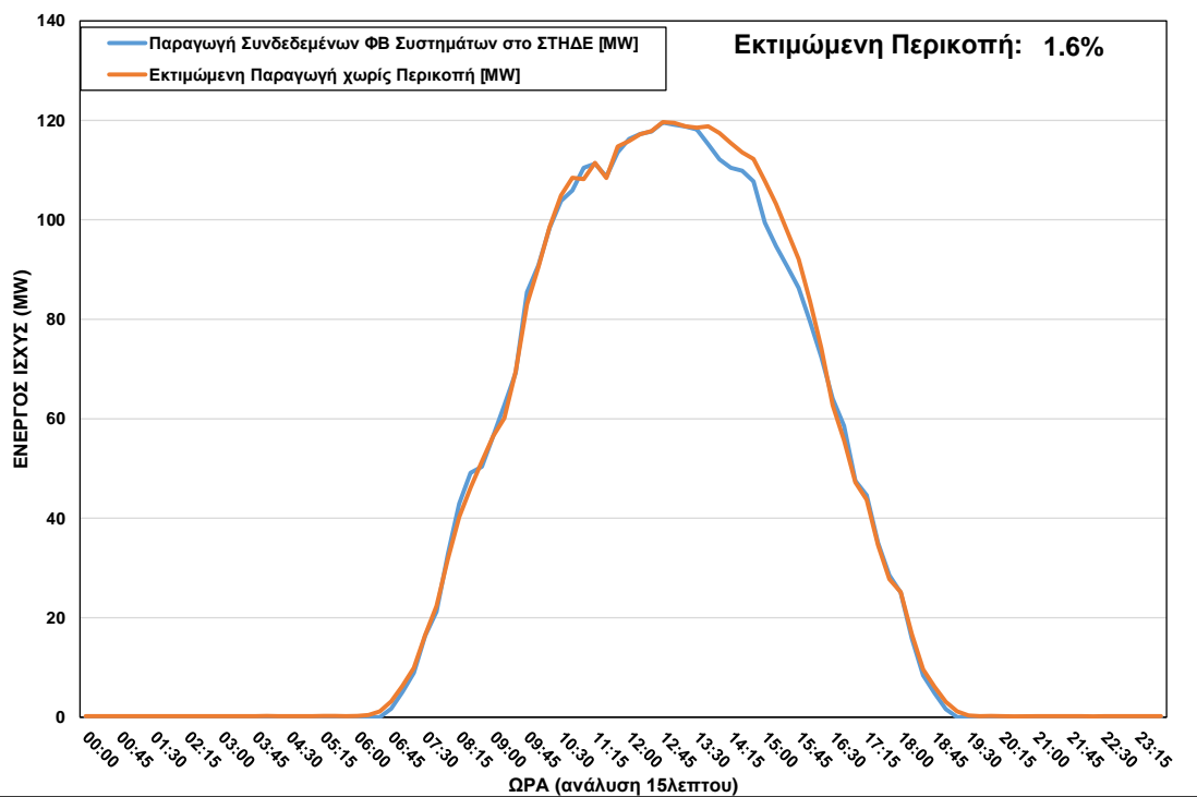
ΦΒ Παραγωγή στο ΣΤΗΔΕ κατά τη διάρκεια περικοπής στις 16/04/2022 ώρα 13:30 – 16:15
