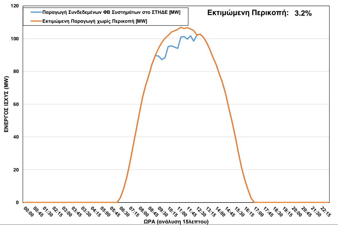
ΦΒ Παραγωγή στο ΣΤΗΔΕ κατά τη διάρκεια περικοπής στις 30/10/2022 ώρα 09:15 – 12:15
