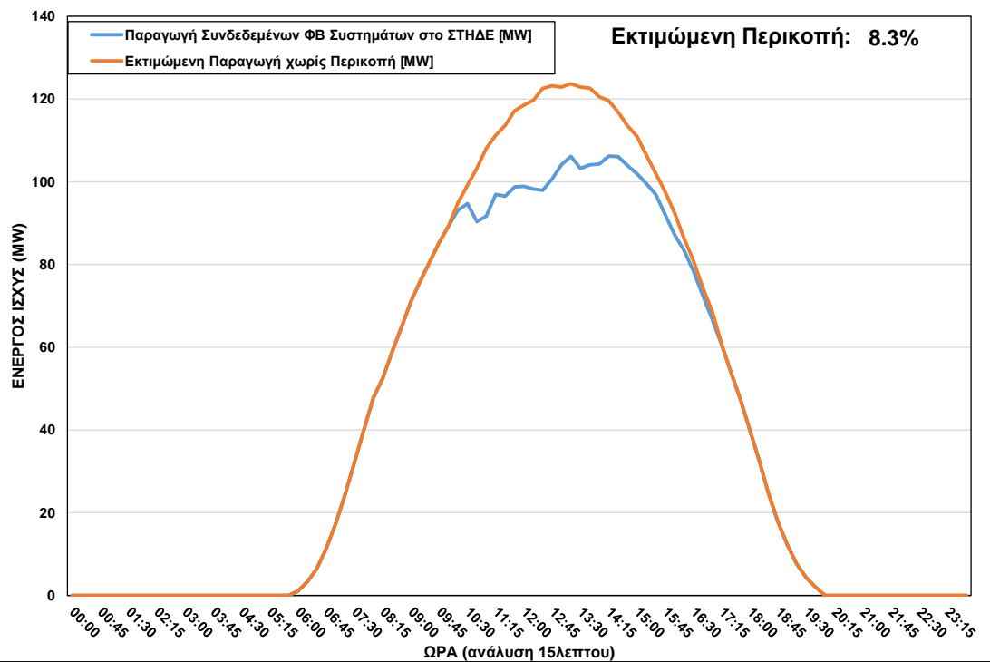
ΦΒ Παραγωγή στο ΣΤΗΔΕ κατά τη διάρκεια περικοπής στις 19/06/2022 ώρα 10:15 – 17:15
