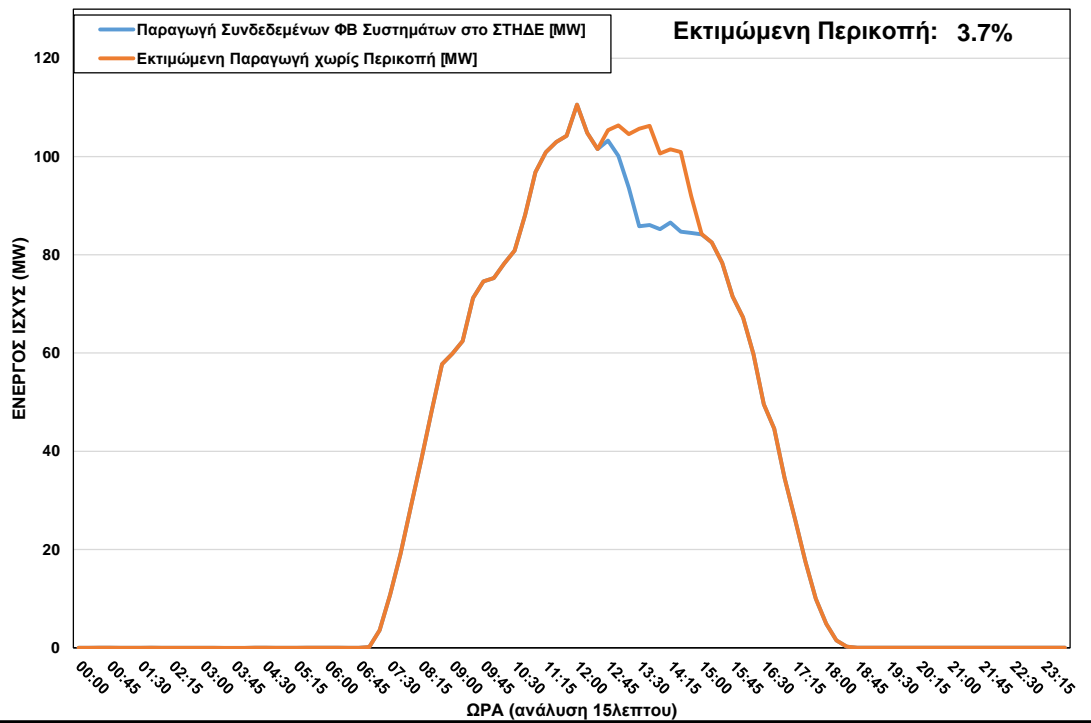
ΦΒ Παραγωγή στο ΣΤΗΔΕ κατά τη διάρκεια περικοπής στις 07/10/2022 ώρα 12:45 – 15:00
