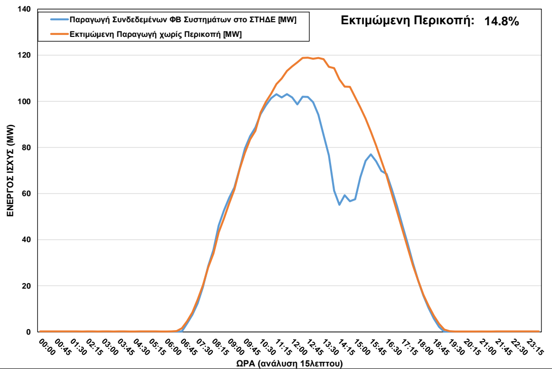
ΦΒ Παραγωγή στο ΣΤΗΔΕ κατά τη διάρκεια περικοπής στις 10/04/2022 ώρα 10:30 – 16:30
