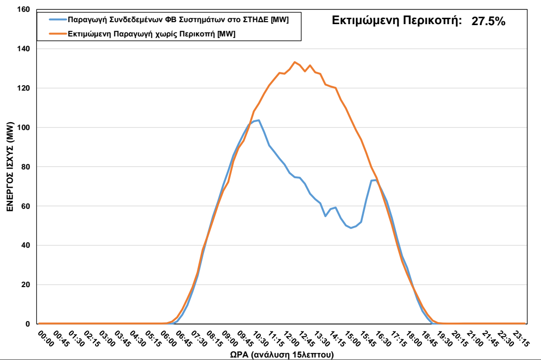
ΦΒ Παραγωγή στο ΣΤΗΔΕ κατά τη διάρκεια περικοπής στις 13/04/2022 ώρα 10:30 – 17:00
