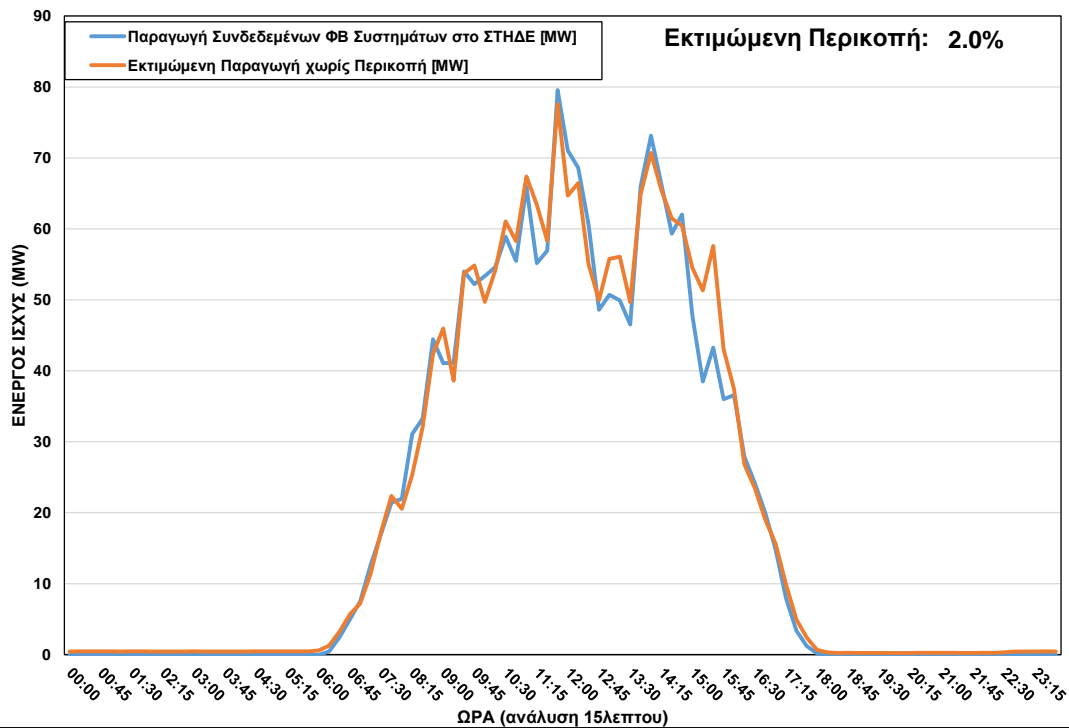
ΦΒ Παραγωγή στο ΣΤΗΔΕ κατά τη διάρκεια περικοπής στις 13/03/2022 ώρα 14:45 – 16:15
