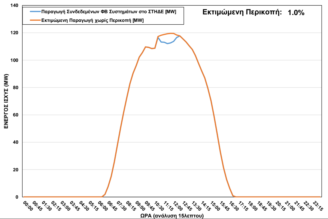
ΦΒ Παραγωγή στο ΣΤΗΔΕ κατά τη διάρκεια περικοπής στις 05/11/2022 ώρα 10:45 – 12:15
