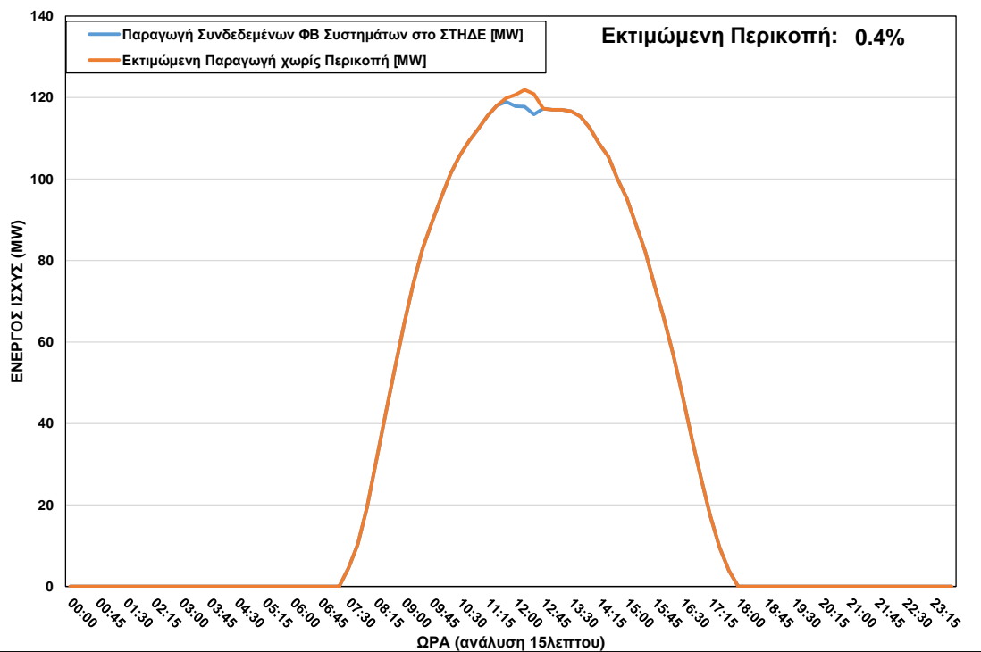
ΦΒ Παραγωγή στο ΣΤΗΔΕ κατά τη διάρκεια περικοπής στις 28/10/2022 ώρα 11:45 – 12:30
