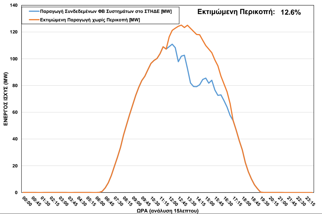
ΦΒ Παραγωγή στο ΣΤΗΔΕ κατά τη διάρκεια περικοπής στις 15/08/2022 ώρα 12:00 – 17:00
