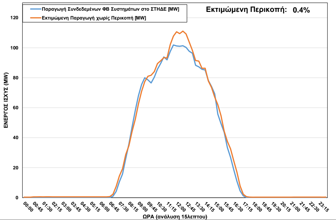
ΦΒ Παραγωγή στο ΣΤΗΔΕ κατά τη διάρκεια περικοπής στις 05/02/2022 ώρα 14:45 – 15:45
