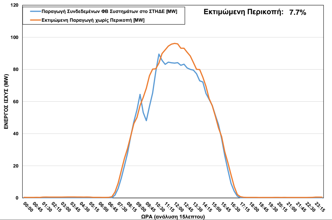
ΦΒ Παραγωγή στο ΣΤΗΔΕ κατά τη διάρκεια περικοπής στις 23/01/2022 ώρα 09:00 – 15:00
