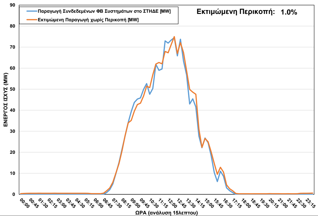
ΦΒ Παραγωγή στο ΣΤΗΔΕ κατά τη διάρκεια περικοπής στις 03/02/2022 ώρα 13:15 – 13:45
