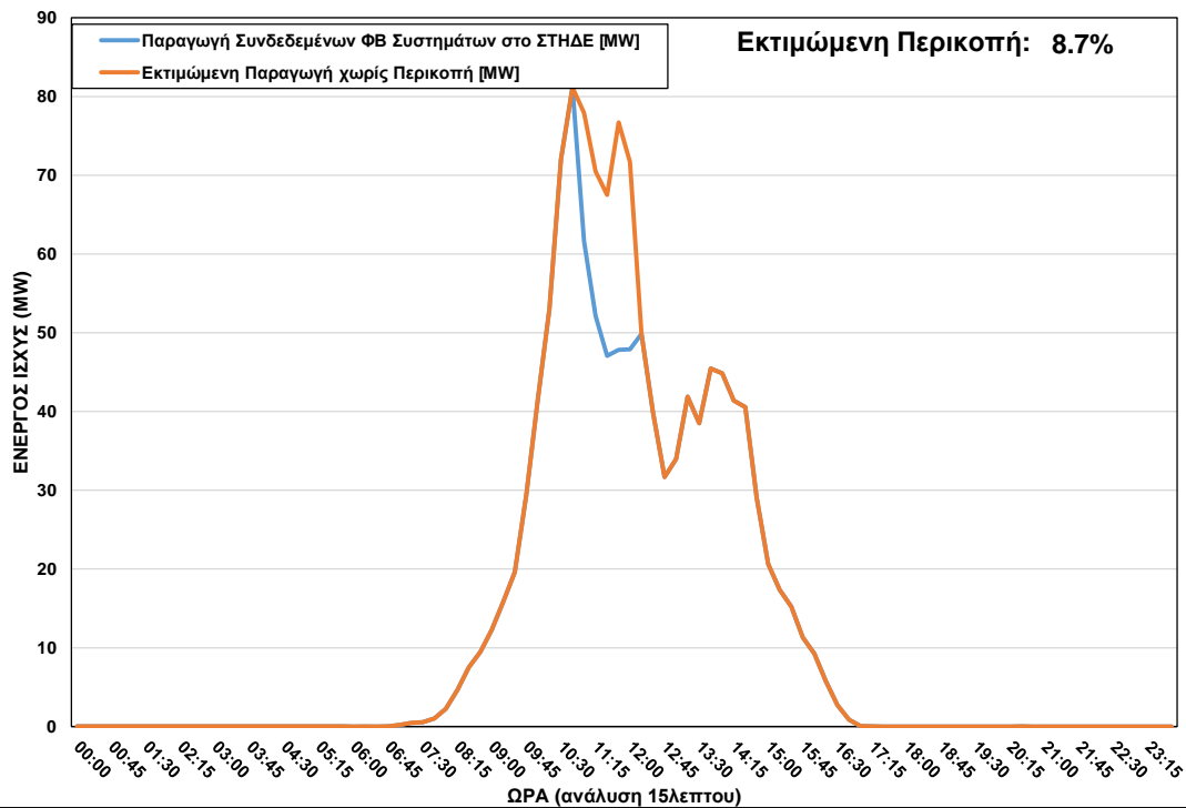
ΦΒ Παραγωγή στο ΣΤΗΔΕ κατά τη διάρκεια περικοπής στις 29/11/2022 ώρα 11:00 – 12:00
