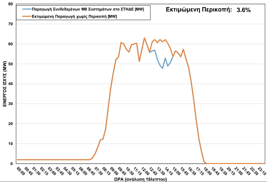
ΦΒ Παραγωγή στο ΣΤΗΔΕ κατά τη διάρκεια περικοπής στις 20/10/2022 ώρα 13:00 – 14:45
