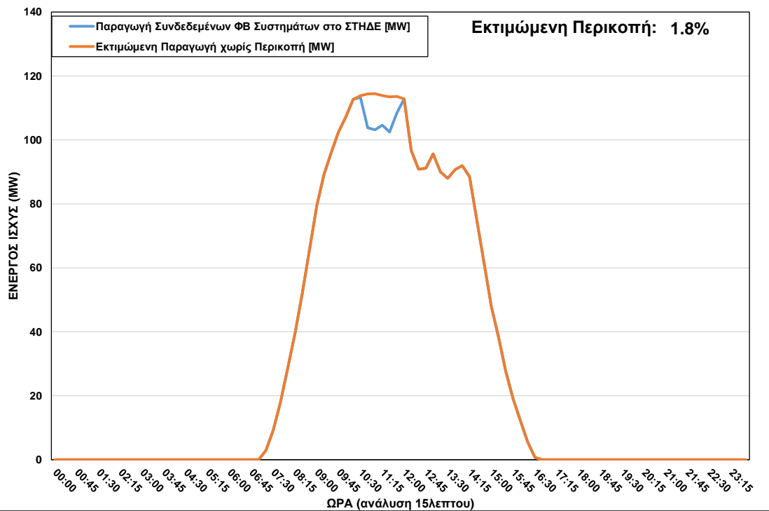
ΦΒ Παραγωγή στο ΣΤΗΔΕ κατά τη διάρκεια περικοπής στις 20/12/2022 ώρα 10:30 – 11:45
