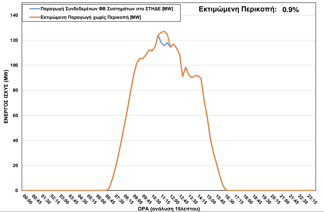
ΦΒ Παραγωγή στο ΣΤΗΔΕ κατά τη διάρκεια περικοπής στις 03/12/2022 ώρα 11:15 – 11:45
