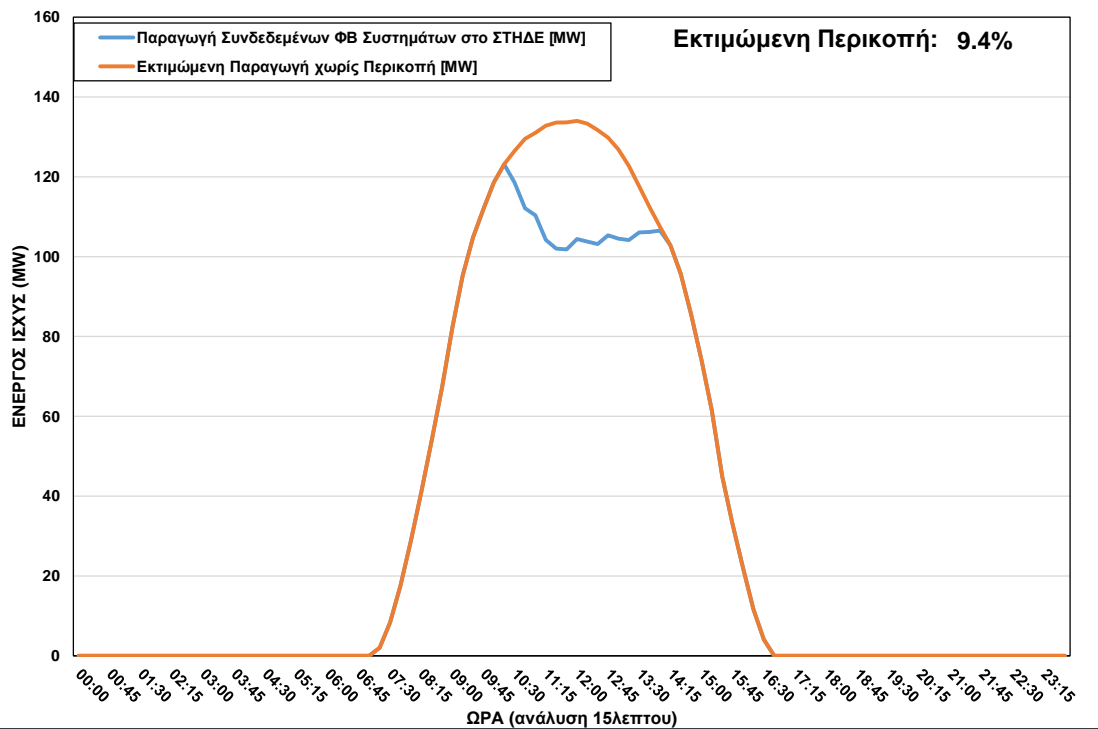
ΦΒ Παραγωγή στο ΣΤΗΔΕ κατά τη διάρκεια περικοπής στις 27/12/2022 ώρα 10:15 – 14:00
