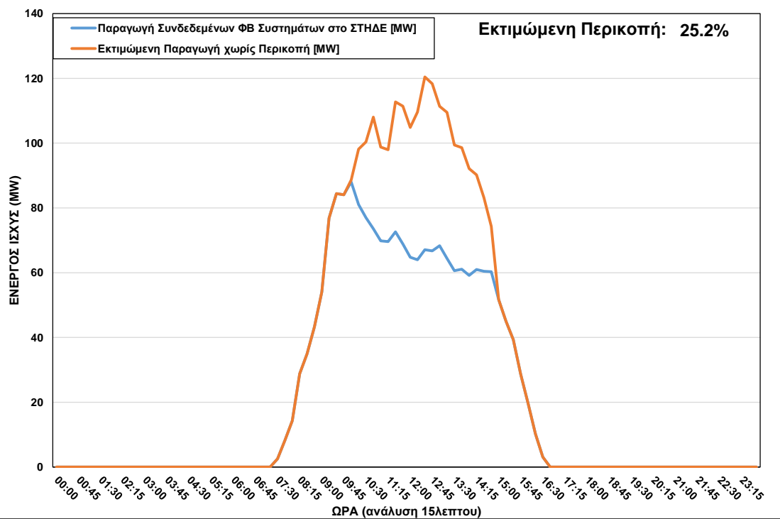
ΦΒ Παραγωγή στο ΣΤΗΔΕ κατά τη διάρκεια περικοπής στις 26/12/2022 ώρα 10:00 – 14:45
