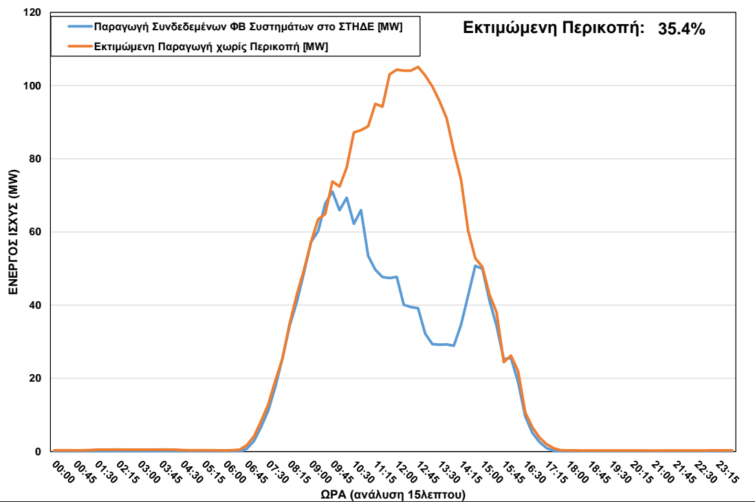
ΦΒ Παραγωγή στο ΣΤΗΔΕ κατά τη διάρκεια περικοπής στις 23/02/2022 ώρα 09:30 – 14:30
