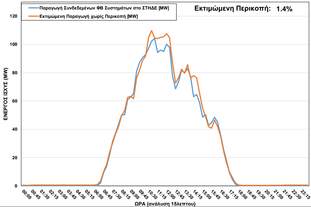
ΦΒ Παραγωγή στο ΣΤΗΔΕ κατά τη διάρκεια περικοπής στις 11/03/2022 ώρα 13:45 – 15:15
