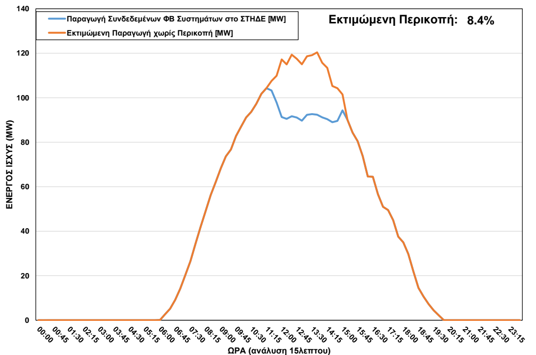
ΦΒ Παραγωγή στο ΣΤΗΔΕ κατά τη διάρκεια περικοπής στις 10/07/2022 ώρα 11:30 – 15:00
