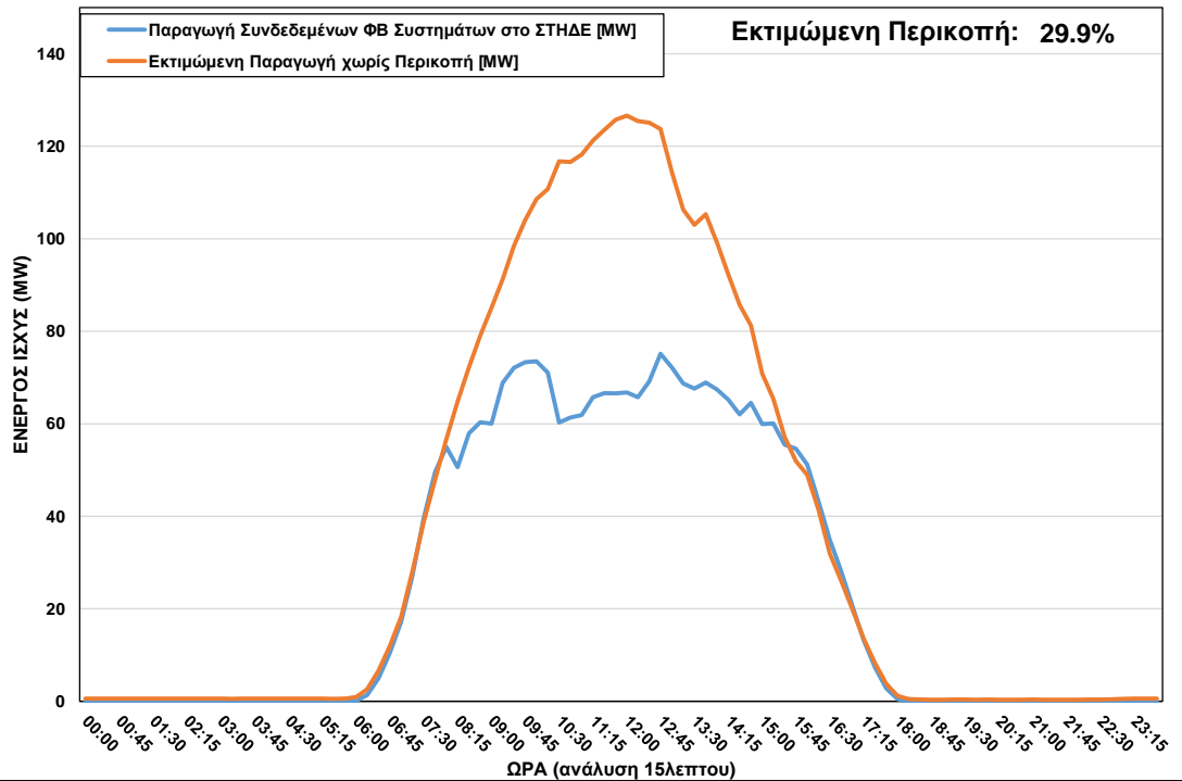
ΦΒ Παραγωγή στο ΣΤΗΔΕ κατά τη διάρκεια περικοπής στις 20/03/2022 ώρα 07:45 – 17:00
