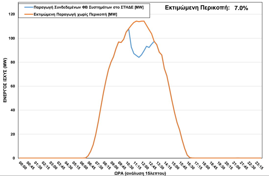
ΦΒ Παραγωγή στο ΣΤΗΔΕ κατά τη διάρκεια περικοπής στις 19/11/2022 ώρα 10:45 – 13:00
