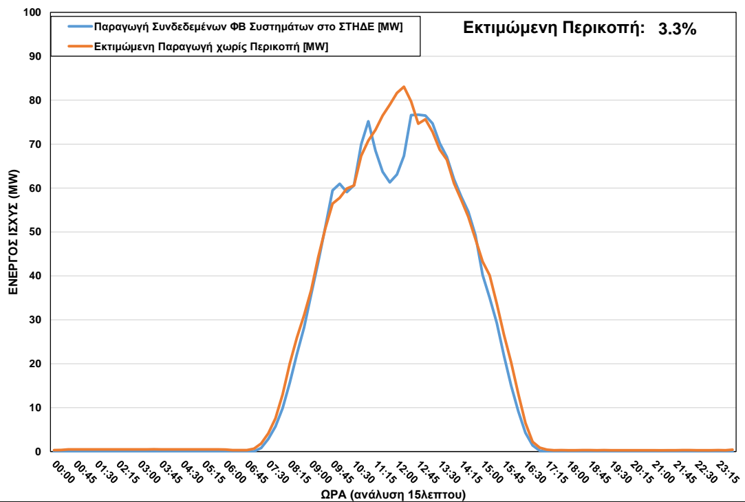
ΦΒ Παραγωγή στο ΣΤΗΔΕ κατά τη διάρκεια περικοπής στις 08/01/2022 ώρα 11:00 – 13:30
