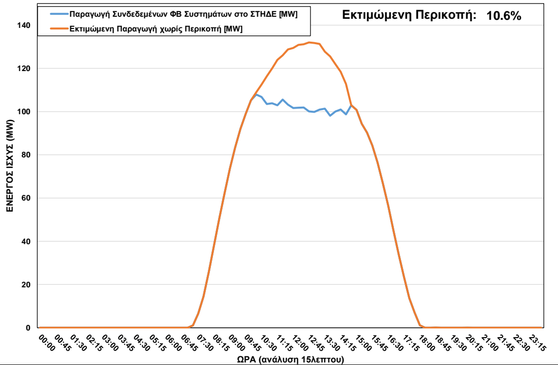
ΦΒ Παραγωγή στο ΣΤΗΔΕ κατά τη διάρκεια περικοπής στις 23/10/2022 ώρα 10:15 – 14:30
