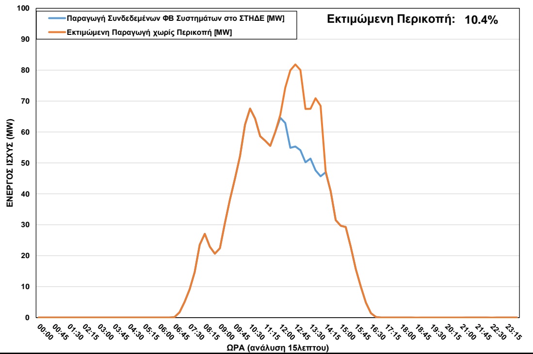
ΦΒ Παραγωγή στο ΣΤΗΔΕ κατά τη διάρκεια περικοπής στις 27/11/2022 ώρα 12:00 – 14:15
