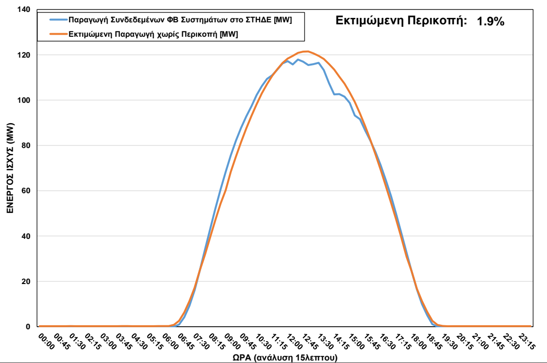
ΦΒ Παραγωγή στο ΣΤΗΔΕ κατά τη διάρκεια περικοπής στις 09/04/2022 ώρα 12:00 – 17:00
