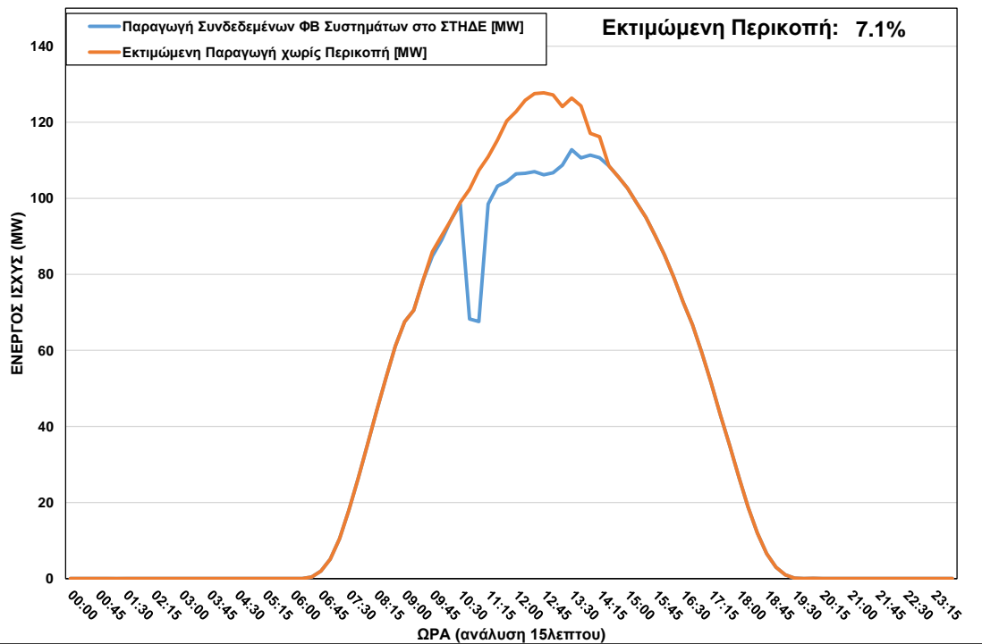
ΦΒ Παραγωγή στο ΣΤΗΔΕ κατά τη διάρκεια περικοπής στις 28/08/2022 ώρα 09:45 – 14:15
