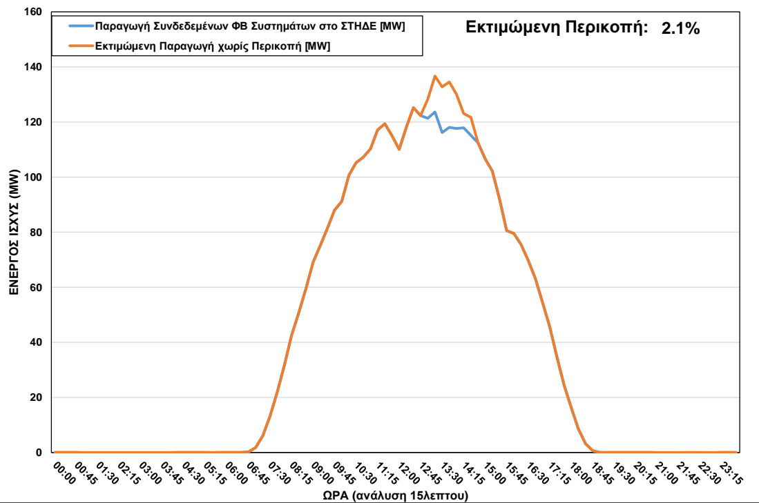
ΦΒ Παραγωγή στο ΣΤΗΔΕ κατά τη διάρκεια περικοπής στις 22/09/2022 ώρα 13:00 – 16:00
