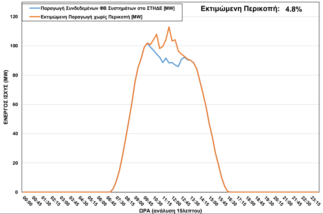
ΦΒ Παραγωγή στο ΣΤΗΔΕ κατά τη διάρκεια περικοπής στις 16/12/2022 ώρα 10:00 – 13:15
