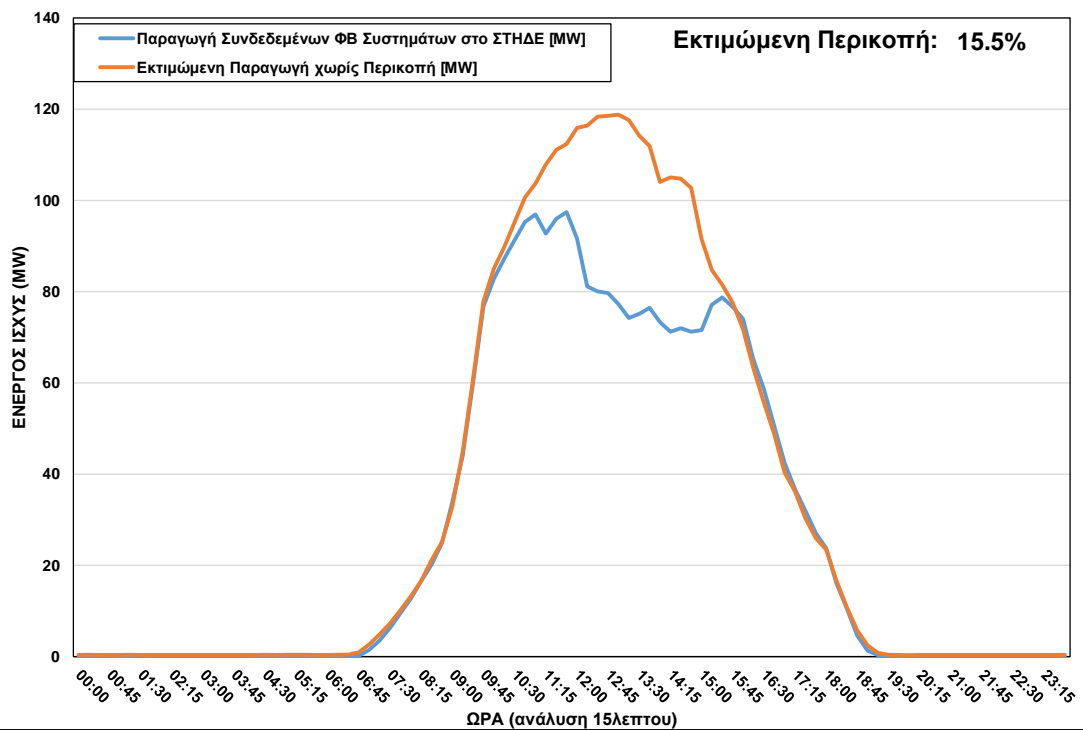
ΦΒ Παραγωγή στο ΣΤΗΔΕ κατά τη διάρκεια περικοπής στις 03/04/2022 ώρα 11:00 – 16:00
