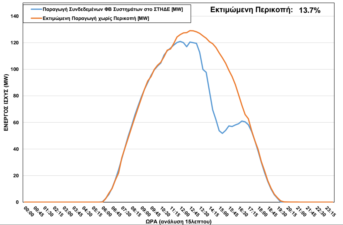
ΦΒ Παραγωγή στο ΣΤΗΔΕ κατά τη διάρκεια περικοπής στις 23/05/2022 ώρα 11:45 – 17:15
