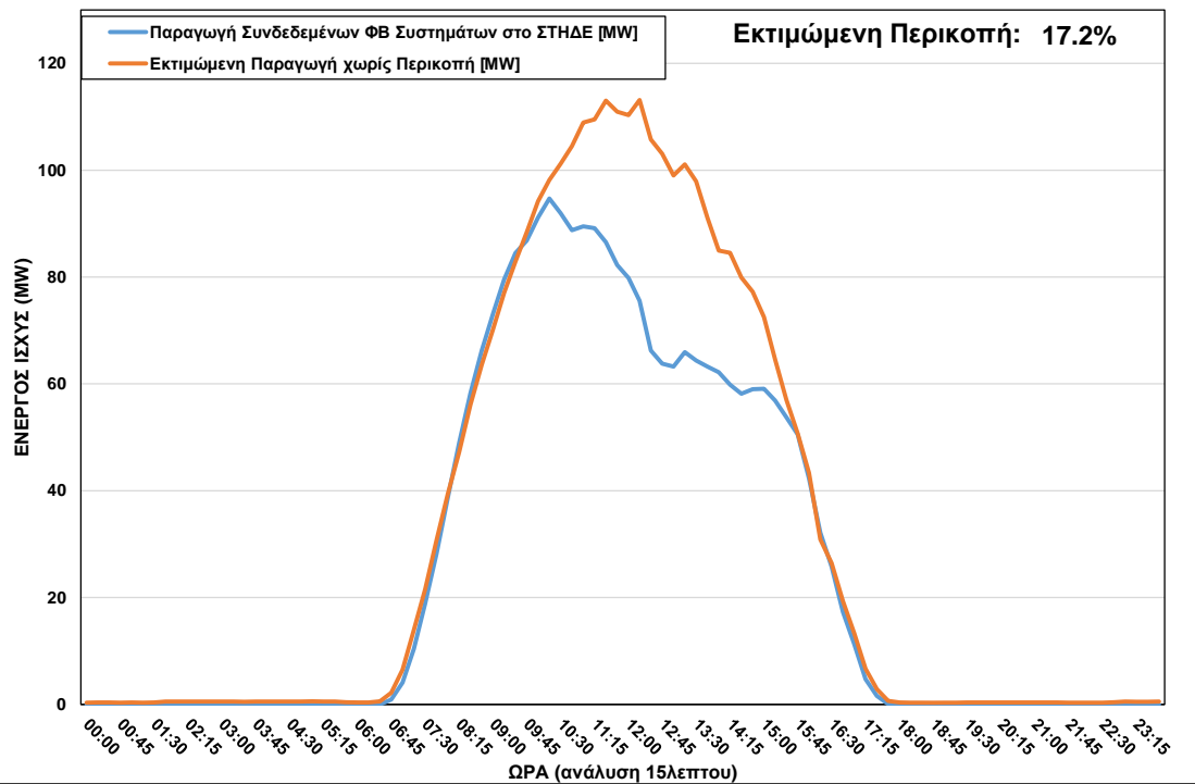
ΦΒ Παραγωγή στο ΣΤΗΔΕ κατά τη διάρκεια περικοπής στις 20/02/2022 ώρα 10:15 – 16:15
