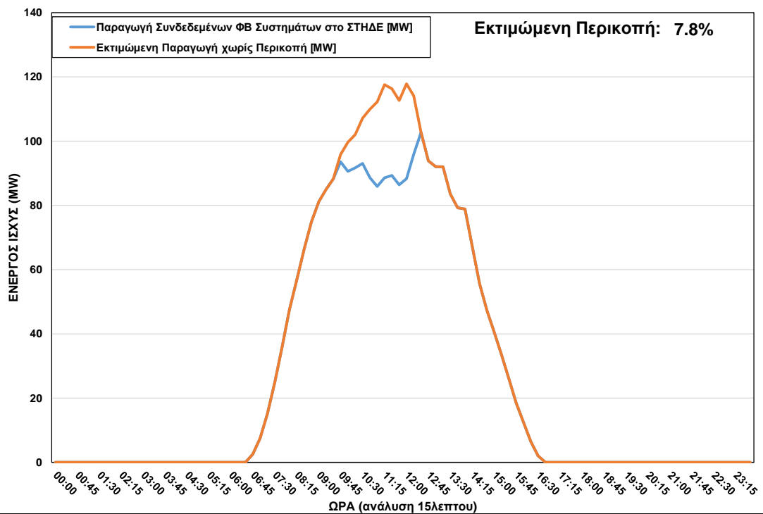
ΦΒ Παραγωγή στο ΣΤΗΔΕ κατά τη διάρκεια περικοπής στις 12/11/2022 ώρα 09:45 – 12:15
