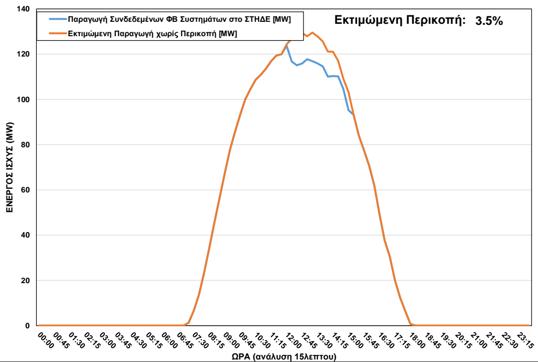
ΦΒ Παραγωγή στο ΣΤΗΔΕ κατά τη διάρκεια περικοπής στις 22/10/2022 ώρα 12:00 – 15:00
