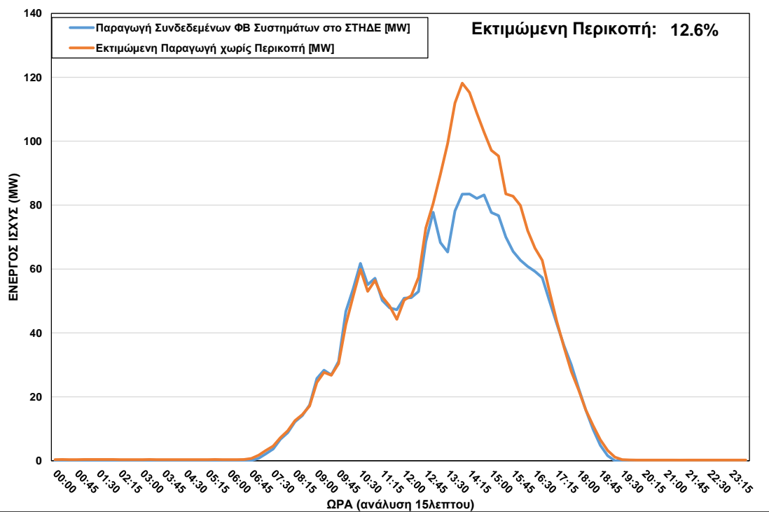
ΦΒ Παραγωγή στο ΣΤΗΔΕ κατά τη διάρκεια περικοπής στις 08/04/2022 ώρα 13:00 – 17:00
