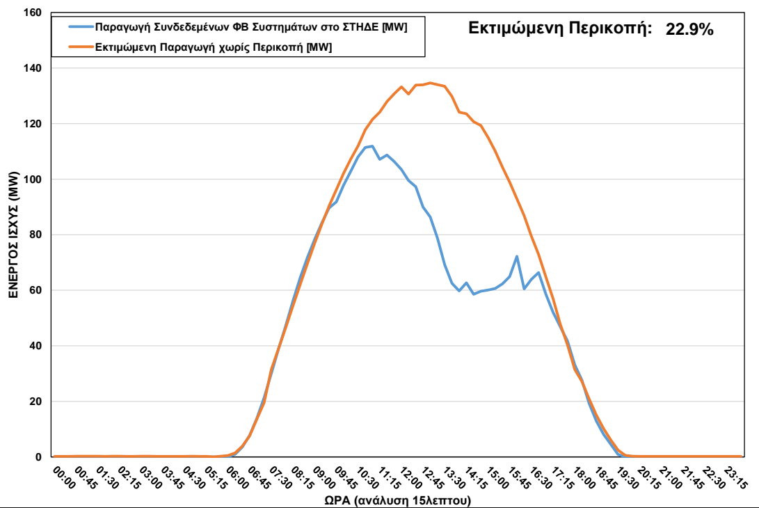
ΦΒ Παραγωγή στο ΣΤΗΔΕ κατά τη διάρκεια περικοπής στις 08/05/2022 ώρα 09:30 – 17:30
