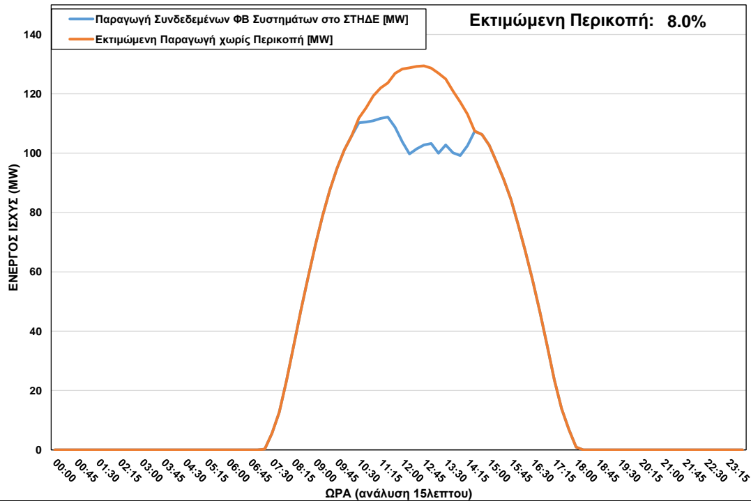
ΦΒ Παραγωγή στο ΣΤΗΔΕ κατά τη διάρκεια περικοπής στις 24/10/2022 ώρα 10:30 – 14:15
