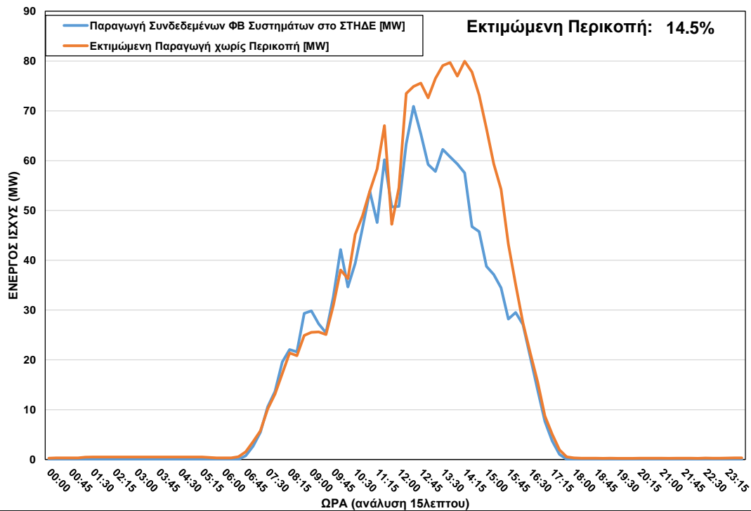
ΦΒ Παραγωγή στο ΣΤΗΔΕ κατά τη διάρκεια περικοπής στις 22/02/2022 ώρα 12:30 – 16:00
