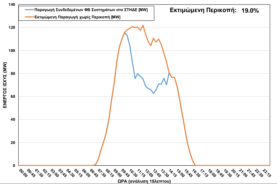
ΦΒ Παραγωγή στο ΣΤΗΔΕ κατά τη διάρκεια περικοπής στις 30/12/2022 ώρα 10:00 – 14:00
