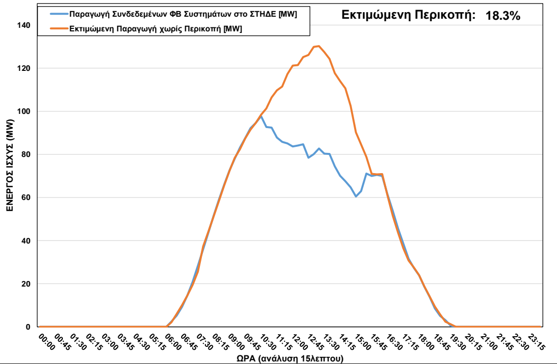
ΦΒ Παραγωγή στο ΣΤΗΔΕ κατά τη διάρκεια περικοπής στις 22/05/2022 ώρα 10:15 – 15:45
