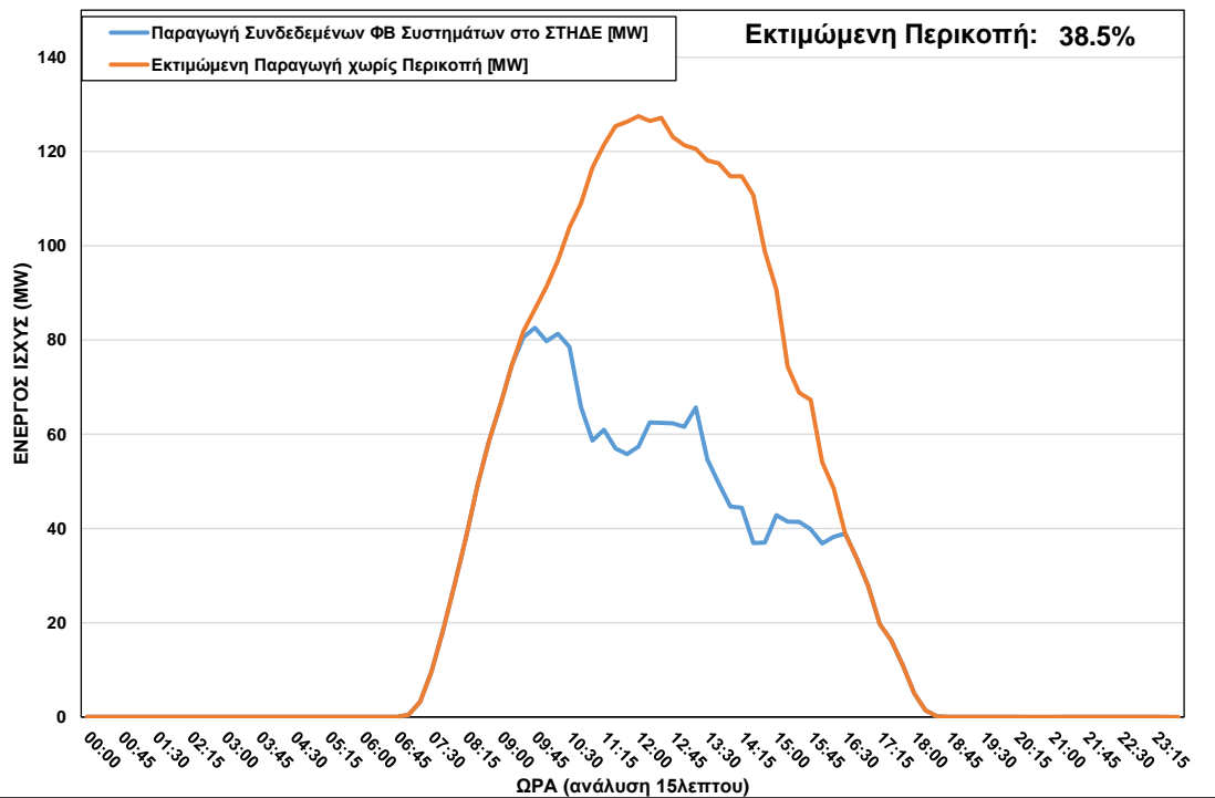
ΦΒ Παραγωγή στο ΣΤΗΔΕ κατά τη διάρκεια περικοπής στις 08/10/2022 ώρα 09:30 – 16:15
