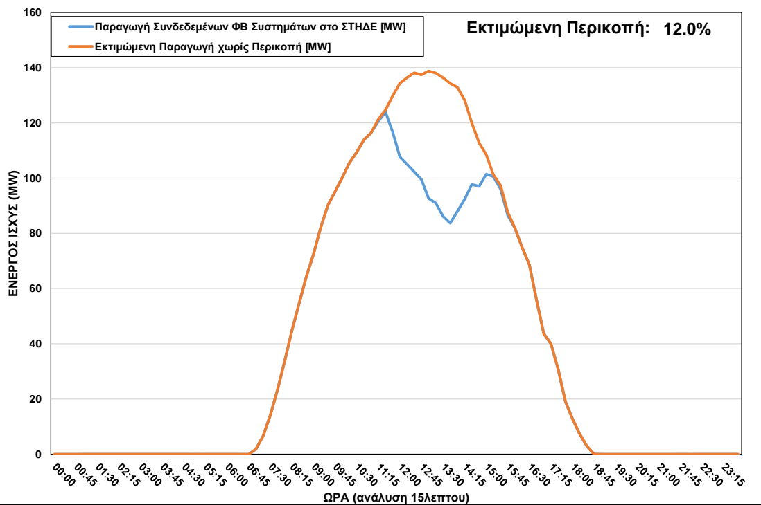
ΦΒ Παραγωγή στο ΣΤΗΔΕ κατά τη διάρκεια περικοπής στις 23/09/2022 ώρα 11:15 – 16:30
