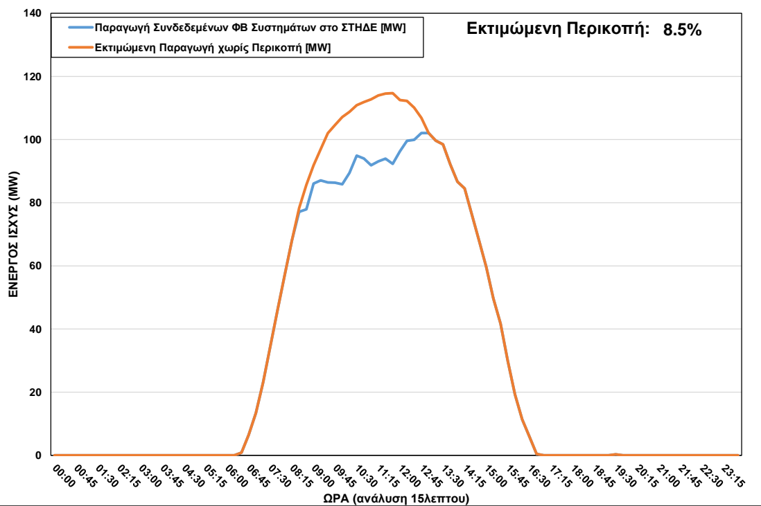
ΦΒ Παραγωγή στο ΣΤΗΔΕ κατά τη διάρκεια περικοπής στις 06/11/2022 ώρα 08:30 – 12:45
