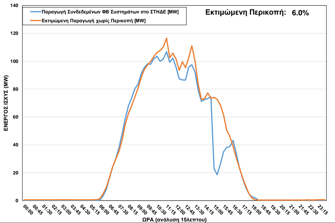
ΦΒ Παραγωγή στο ΣΤΗΔΕ κατά τη διάρκεια περικοπής στις 25/03/2022 ώρα 14:45 – 16:15
