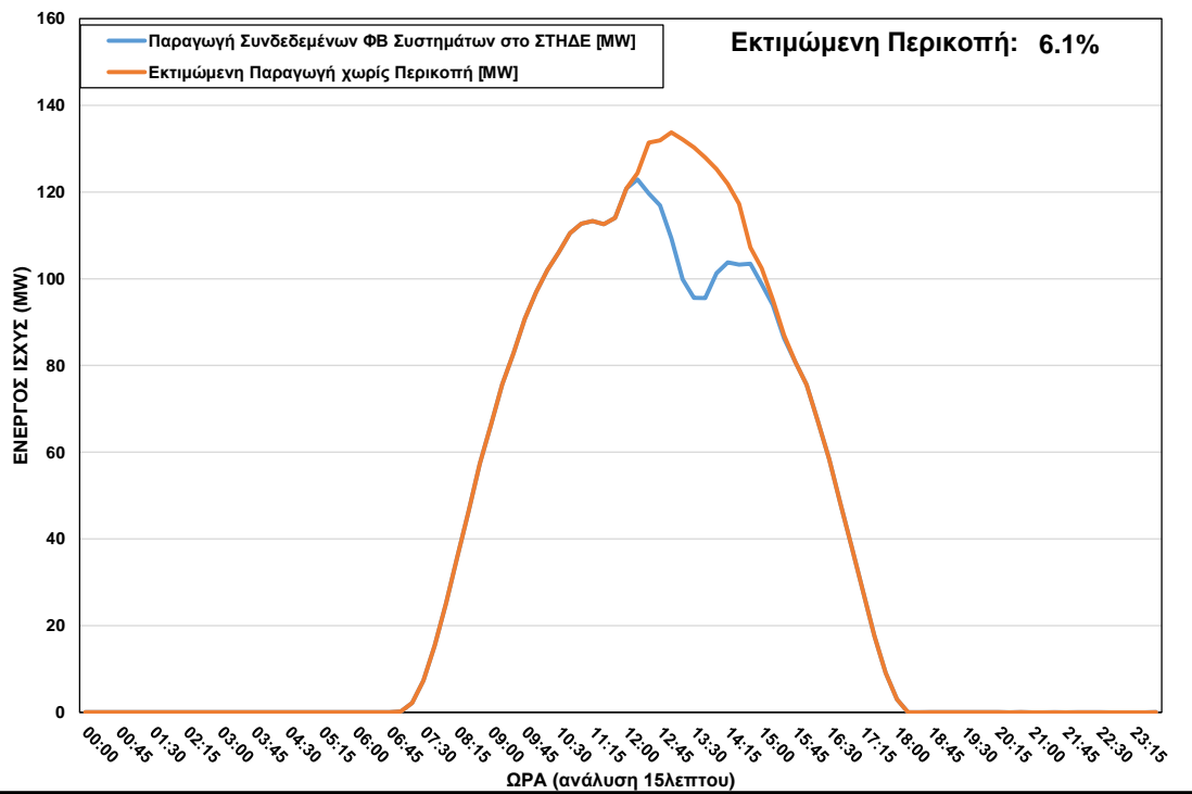
ΦΒ Παραγωγή στο ΣΤΗΔΕ κατά τη διάρκεια περικοπής στις 13/10/2022 ώρα 12:15 – 15:30
