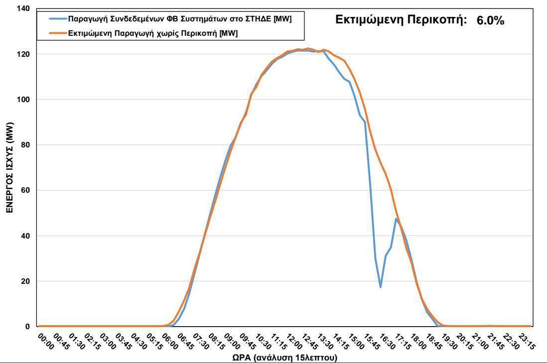
ΦΒ Παραγωγή στο ΣΤΗΔΕ κατά τη διάρκεια περικοπής στις 21/04/2022 ώρα 13:45 – 17:45
