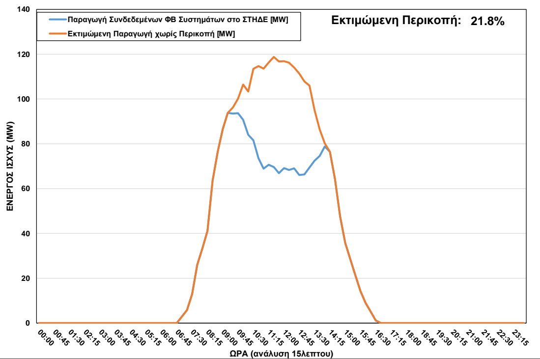
ΦΒ Παραγωγή στο ΣΤΗΔΕ κατά τη διάρκεια περικοπής στις 02/12/2022 ώρα 09:30 – 14:00
