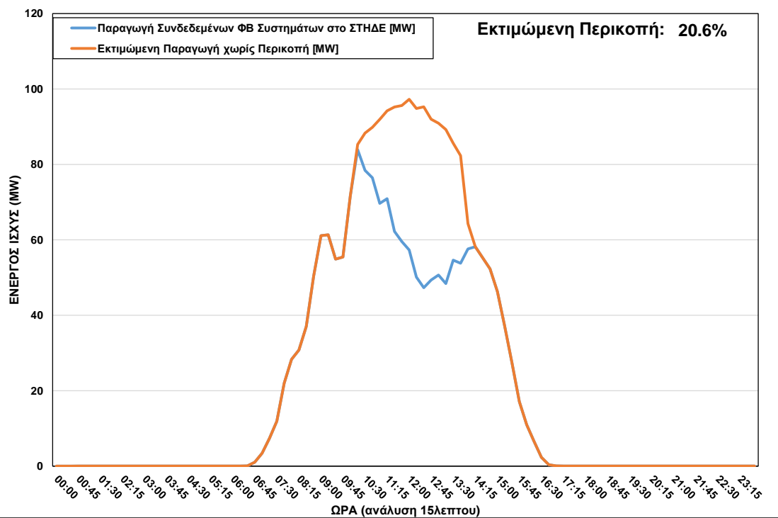
ΦΒ Παραγωγή στο ΣΤΗΔΕ κατά τη διάρκεια περικοπής στις 18/11/2022 ώρα 10:15 – 14:00
