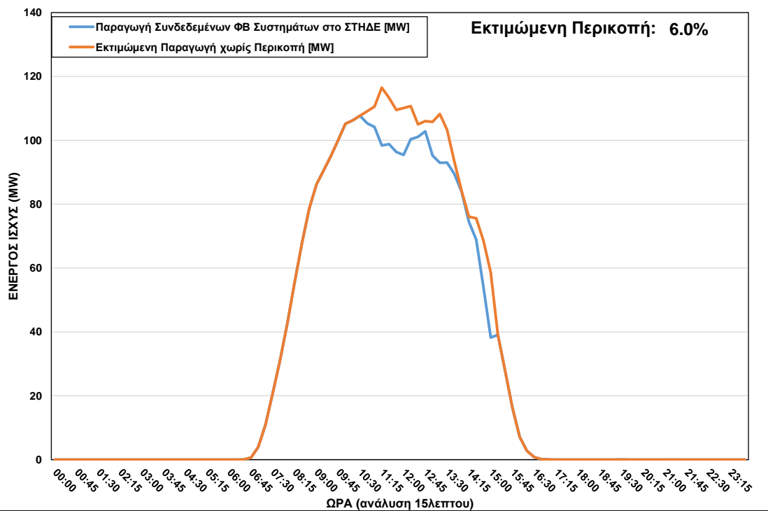
ΦΒ Παραγωγή στο ΣΤΗΔΕ κατά τη διάρκεια περικοπής στις 26/11/2022 ώρα 10:45 – 15:00
