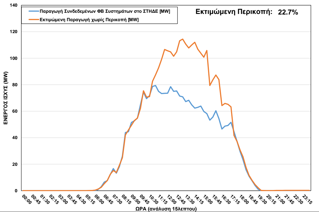
ΦΒ Παραγωγή στο ΣΤΗΔΕ κατά τη διάρκεια περικοπής στις 15/05/2022 ώρα 10:45 – 16:30
