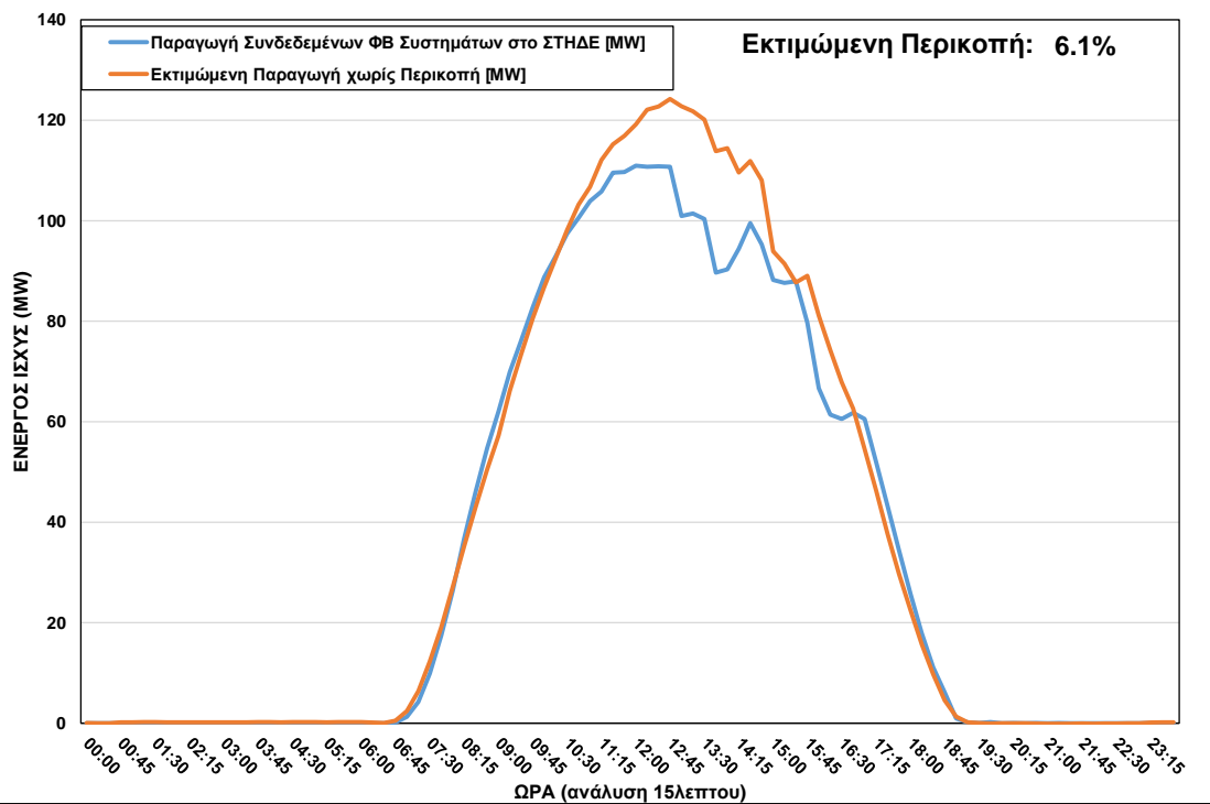
ΦΒ Παραγωγή στο ΣΤΗΔΕ κατά τη διάρκεια περικοπής στις 28/03/2022 ώρα 12:45 – 16:45
