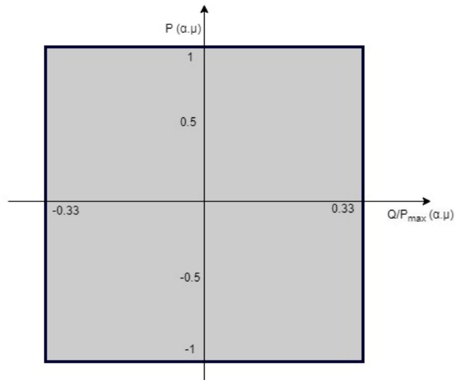
Σχεδιάγραμμα Δ5.3: Εύρος λειτουργίας Άεργου Ισχύος για P<P max
