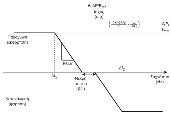
Σχεδιάγραμμα Δ5.10: Χαρακτηριστική ανταπόκρισης σε λειτουργία FSM
