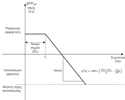
Σχεδιάγραμμα Δ5.8: Χαρακτηριστική ανταπόκρισης σε λειτουργία LFSM-O
