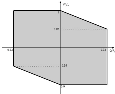
Σχεδιάγραμμα 5.2: Εύρος λειτουργίας Άεργου Ισχύος για P=P_{\max}
