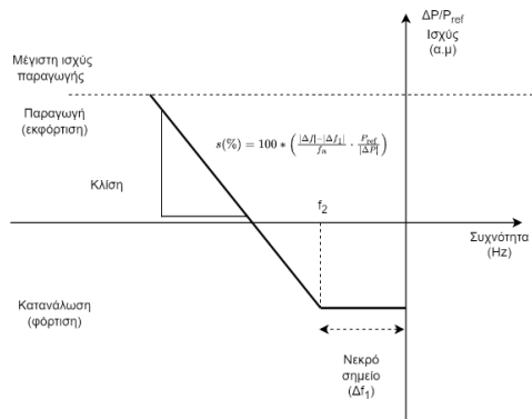
Σχεδιάγραμμα Δ5.9: Χαρακτηριστική ανταπόκρισης σε λειτουργία LFSM-U
