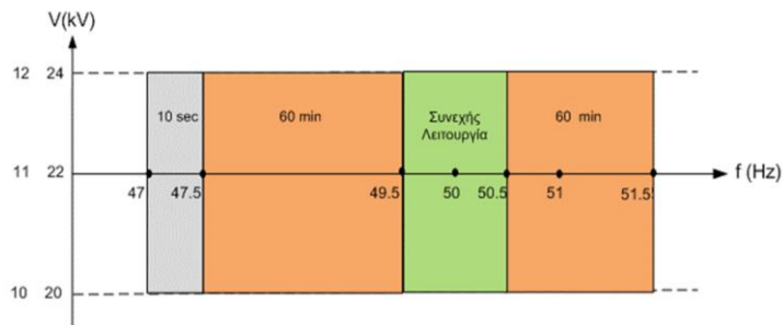
Σχεδιάγραμμα Δ5.1: Υποχρεωτική Δυνατότητα Λειτουργίας Συστημάτων ΑΠΕ (εντός του εύρους Τάσης κανονικής λειτουργίας του Ηλεκτρικού Συστήματος ) σε συνάρτηση με τη Συχνότητα .
