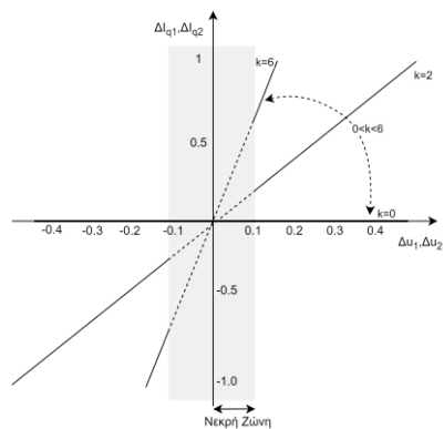
Σχεδιάγραμμα Δ5.7: Ρύθμιση Ταχύος Ρεύματος Σφάλματος
