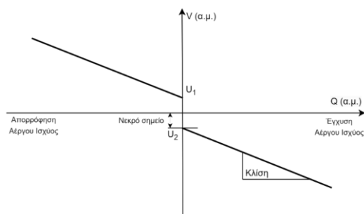
Σχεδιάγραμμα Δ5.12: Χαρακτηριστική άεργου ισχύος – τάσης
