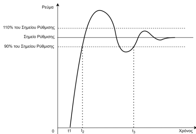
Σχεδιάγραμμα Δ5.6: Χρόνος Ανταπόκρισης ρύθμισης Ταχύος Ρεύματος Σφάλματος
