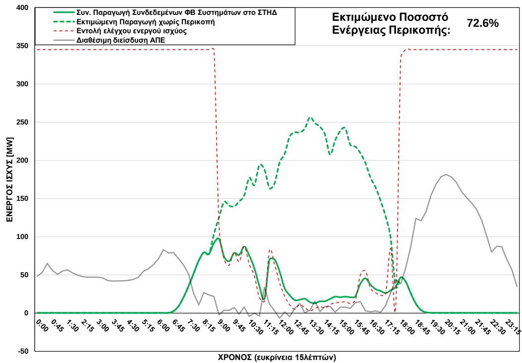
ΦΒ Παραγωγή στο ΣΤΗΔ στις 06/04/2025 (ώρα περικοπής: 08:45 - 17:30)
