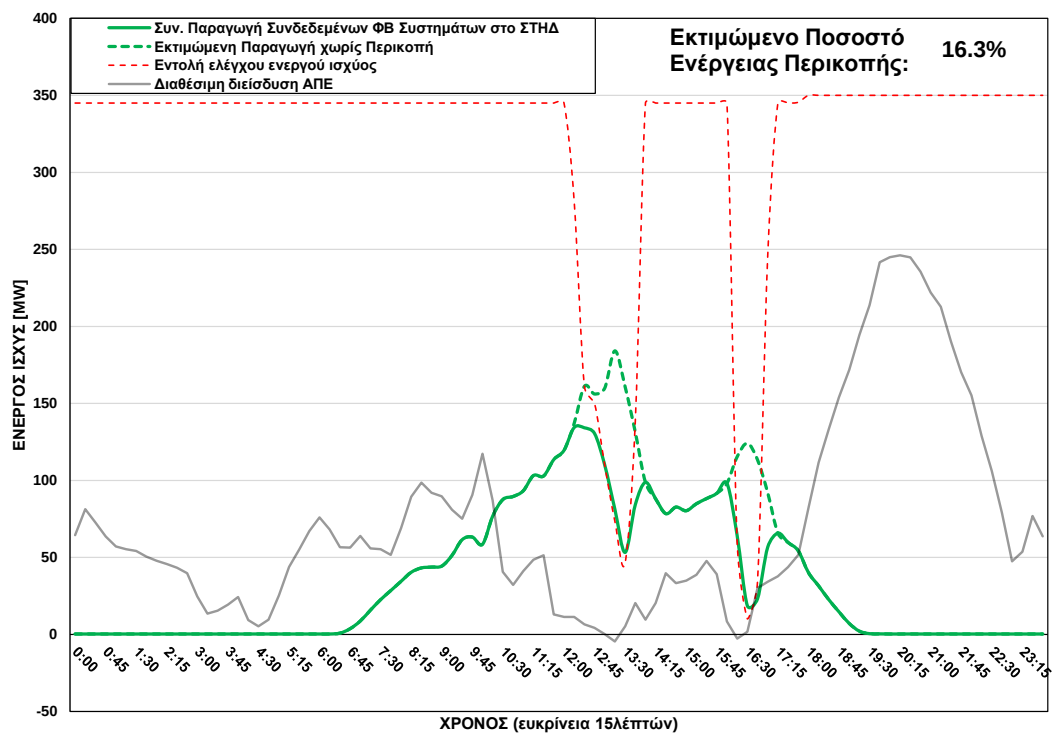
ΦΒ Παραγωγή στο ΣΤΗΔ στις 13/04/2025 (ώρα περικοπής: 12:15 - 17:00)
