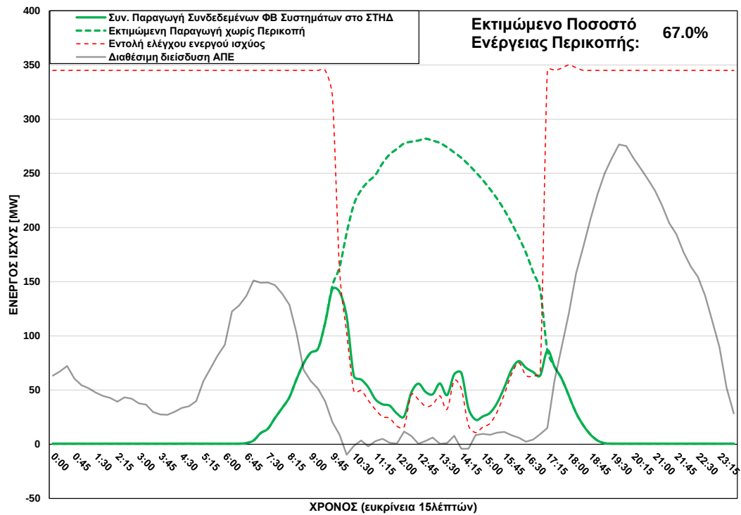
ΦΒ Παραγωγή στο ΣΤΗΔ στις 08/04/2025 (ώρα περικοπής: 09:45 - 17:00)
