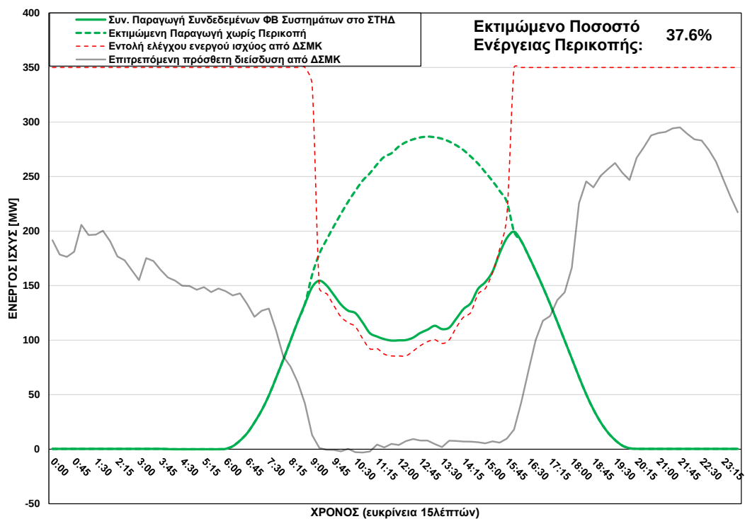
ΦΒ Παραγωγή στο ΣΤΗΔ στις 20/07/2025 (ώρα περικοπής: 09:00 - 15:45)
