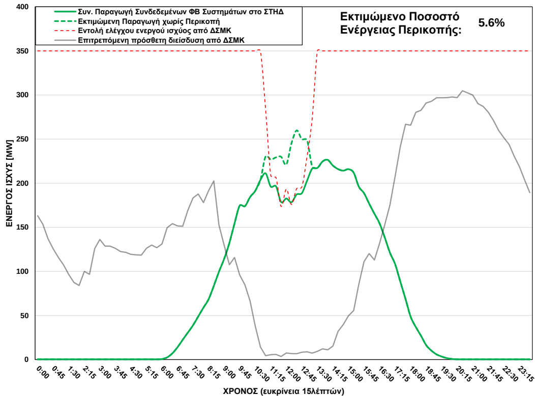
ΦΒ Παραγωγή στο ΣΤΗΔ στις 16/07/2025 (ώρα περικοπής: 11:00 - 13:15)
