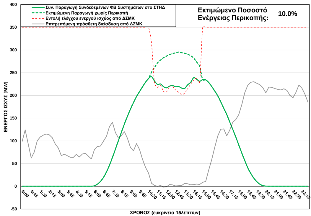
ΦΒ Παραγωγή στο ΣΤΗΔ στις 08/07/2025 (ώρα περικοπής: 10:45 - 14:45)
