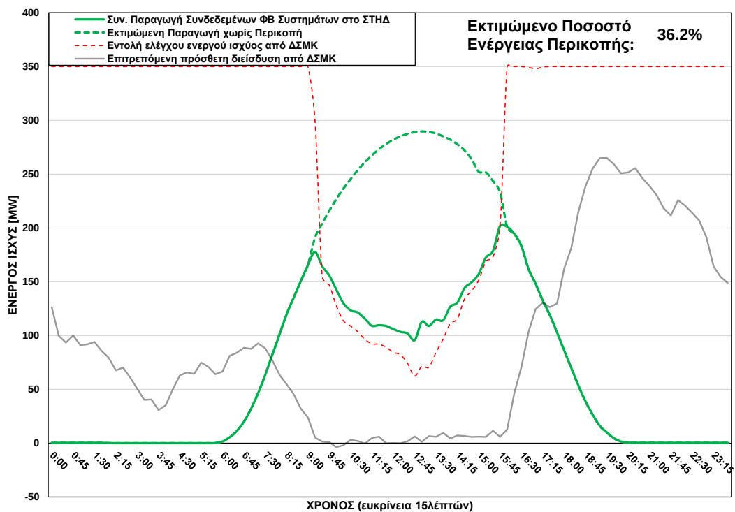
ΦΒ Παραγωγή στο ΣΤΗΔ στις 02/07/2025 (ώρα περικοπής: 09:15 - 15:45)
