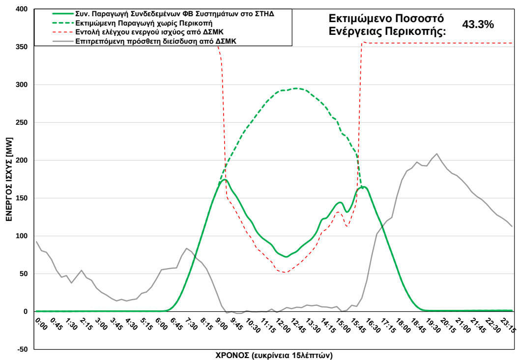
ΦΒ Παραγωγή στο ΣΤΗΔ στις 29/08/2025 (ώρα περικοπής: 09:15 - 16:00)
