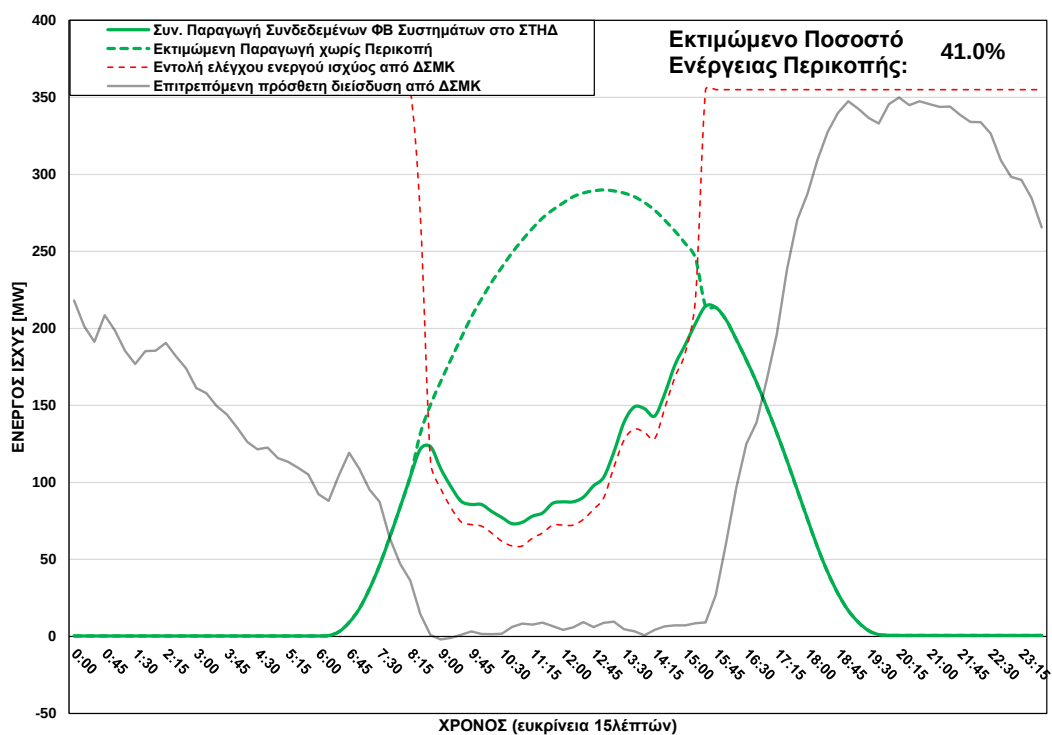
ΦΒ Παραγωγή στο ΣΤΗΔ στις 10/08/2025 (ώρα περικοπής: 08:30 - 15:15)
