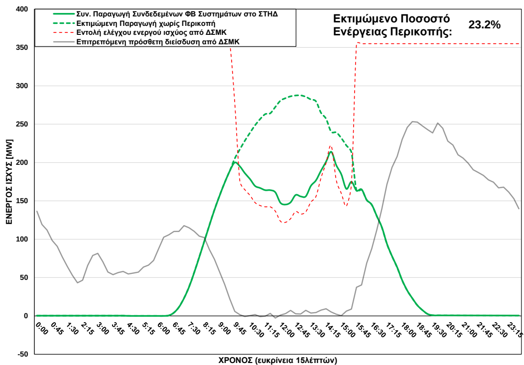
ΦΒ Παραγωγή στο ΣΤΗΔ στις 27/08/2025 (ώρα περικοπής: 09:45 - 15:30)
