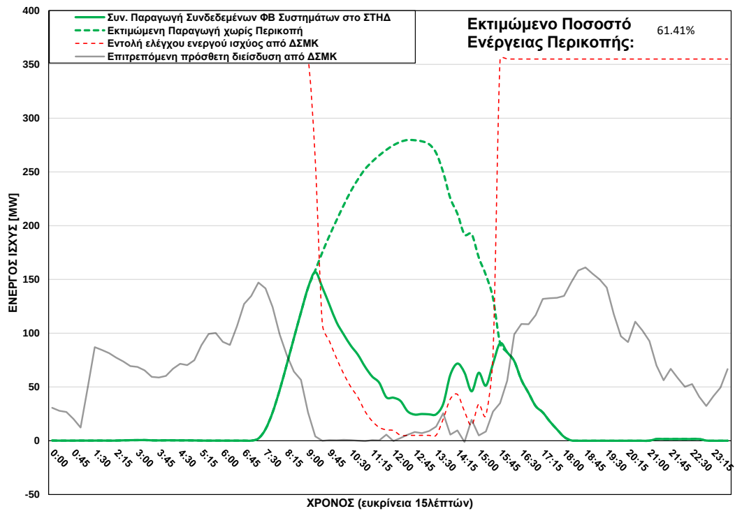
ΦΒ Παραγωγή στο ΣΤΗΔ στις 22/10/2025 (ώρα περικοπής: 09:15 - 15:30)
