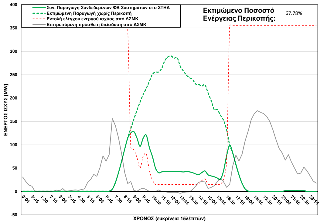
ΦΒ Παραγωγή στο ΣΤΗΔ στις 15/10/2025 (ώρα περικοπής: 08:30 - 16:30)
