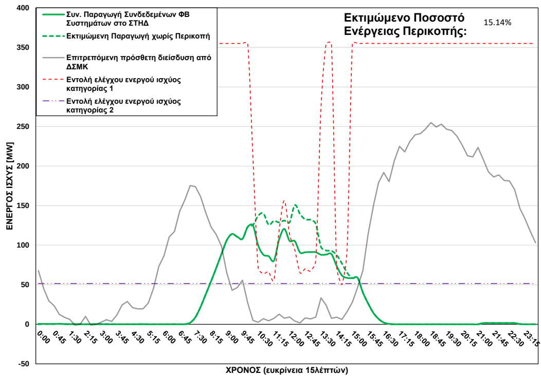
ΦΒ Παραγωγή στο ΣΤΗΔ στις 23/12/2025 (ώρα περικοπής: 10:15 - 14:45)
