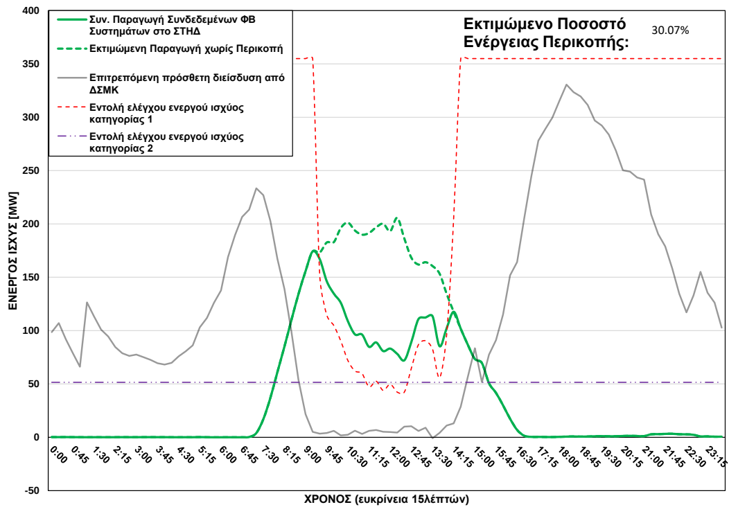
ΦΒ Παραγωγή στο ΣΤΗΔ στις 30/12/2025 (ώρα περικοπής: 09:15 - 14:15)
