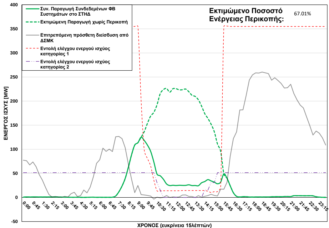
ΦΒ Παραγωγή στο ΣΤΗΔ στις 29/12/2025 (ώρα περικοπής: 09:15 - 15:30)
