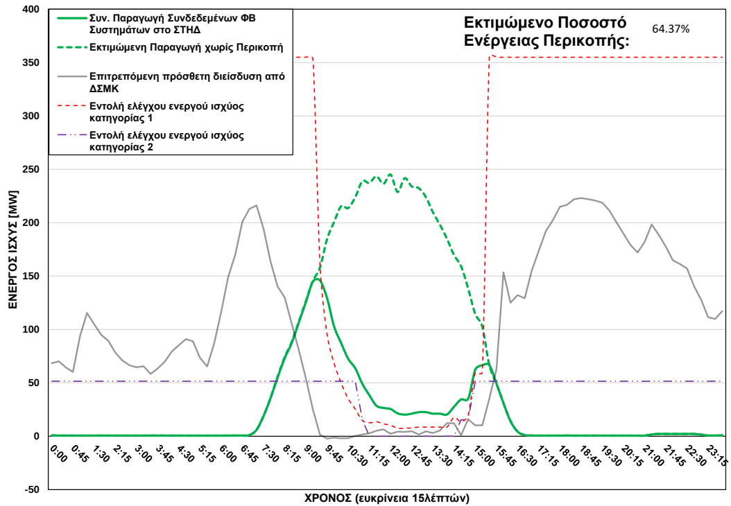
ΦΒ Παραγωγή στο ΣΤΗΔ στις 19/12/2025 (ώρα περικοπής: 09:15 - 15:15)
