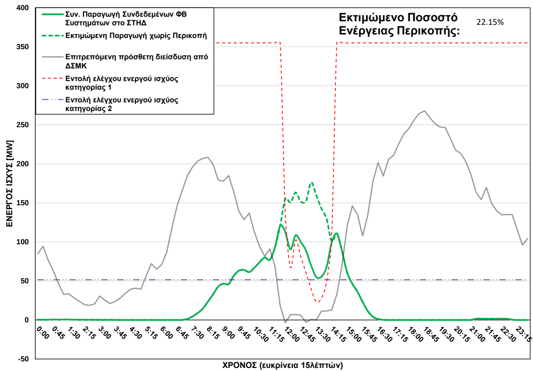
ΦΒ Παραγωγή στο ΣΤΗΔ στις 11/12/2025 (ώρα περικοπής: 12:00 - 14:15)
