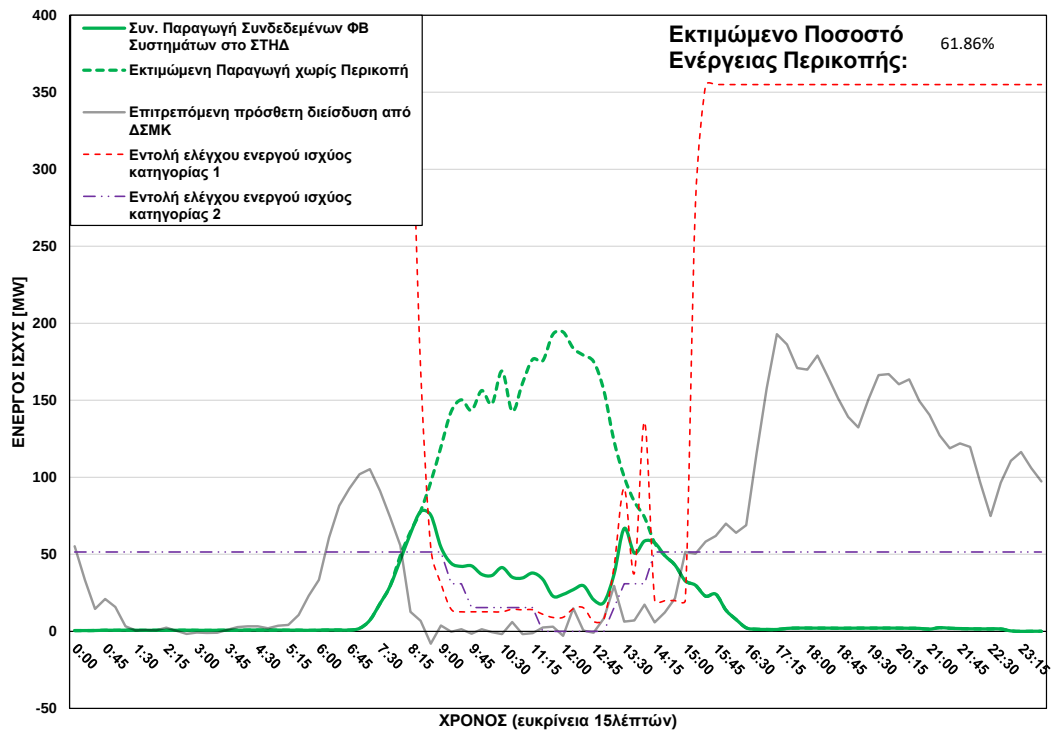
ΦΒ Παραγωγή στο ΣΤΗΔ στις 05/12/2025 (ώρα περικοπής: 08:00 - 14:00)
