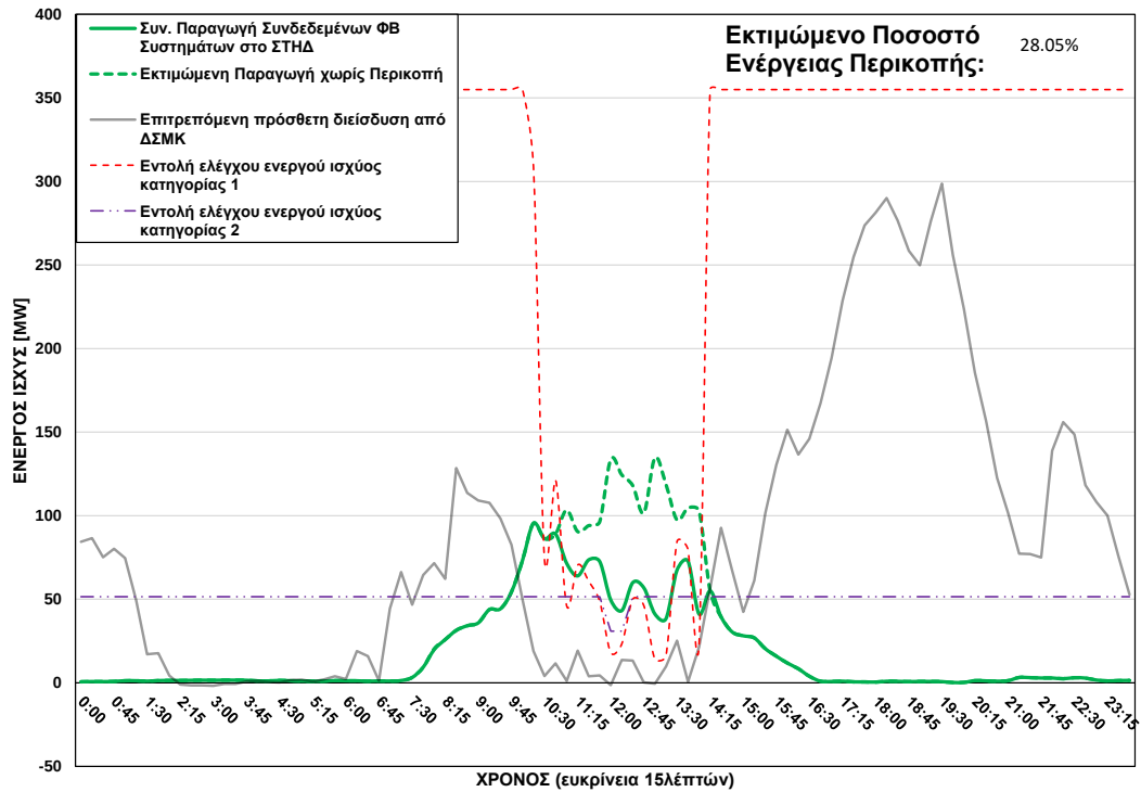
ΦΒ Παραγωγή στο ΣΤΗΔ στις 31/12/2025 (ώρα περικοπής: 10:15 - 14:00)
