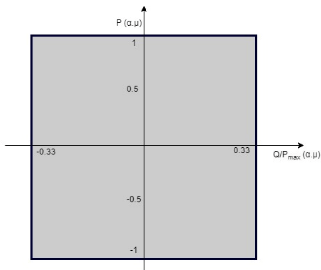
Σχεδιάγραμμα Δ5.3: Εύρος λειτουργίας Άεργου Ισχύος για P < P_{max}
