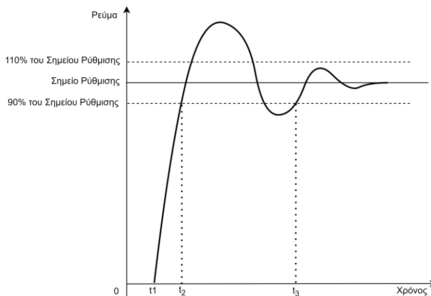
Σχεδιάγραμμα Δ5.6: Χρόνος Ανταπόκρισης ρύθμισης Ταχέος Ρεύματος Σφάλματος
