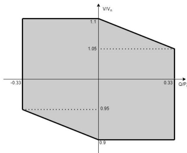
Σχεδιάγραμμα 5.2: Εύρος λειτουργίας Άεργου Ισχύος για P=P_{max}
