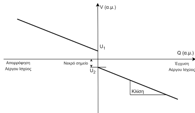
Σχεδιάγραμμα Δ5.12: Χαρακτηριστική άεργου ισχύος – τάσης
