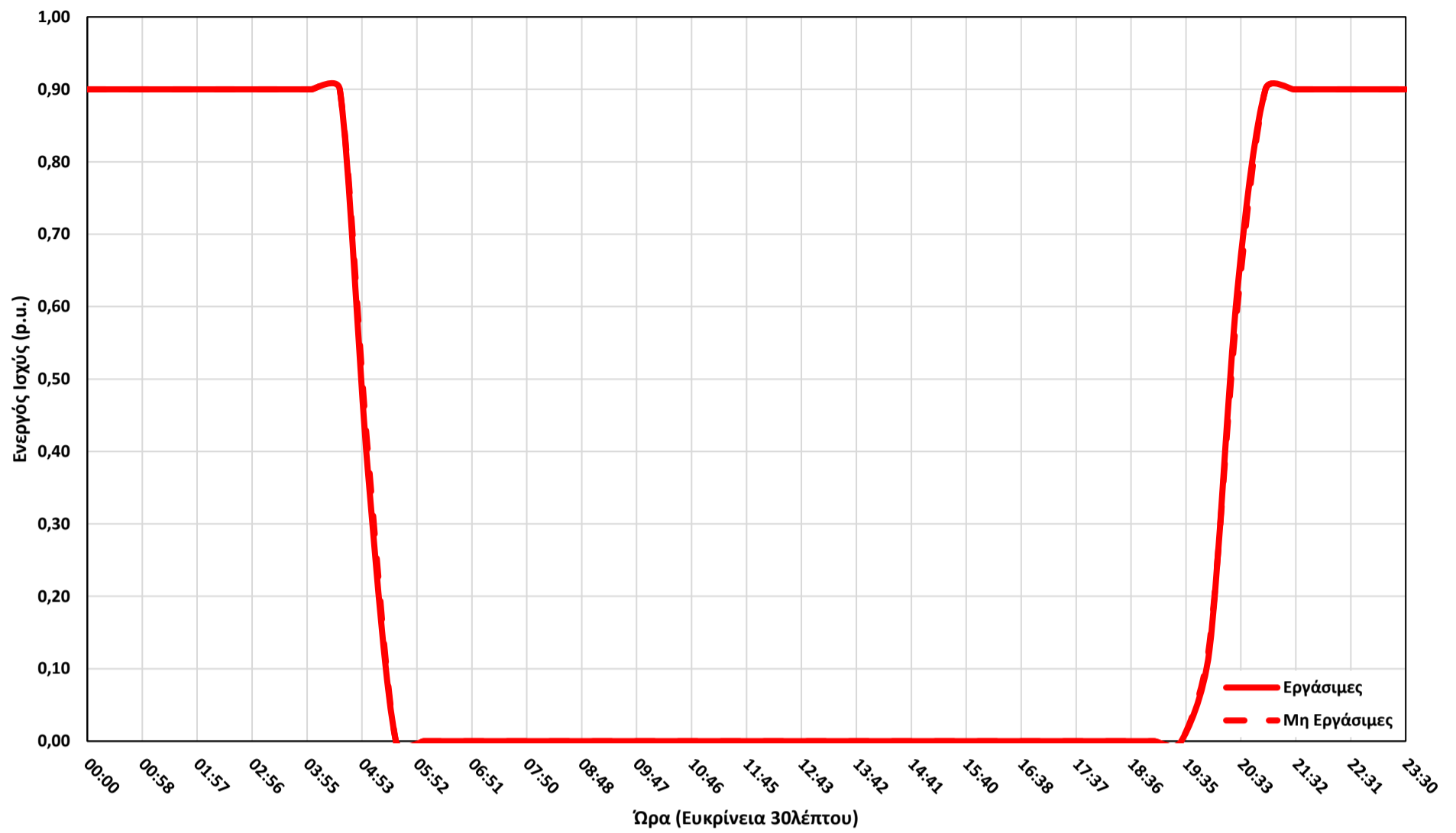
Τυπικό Προφίλ Ενεργού Ισχύος Οδικού Φωτισμού για το Καλοκαίρι
