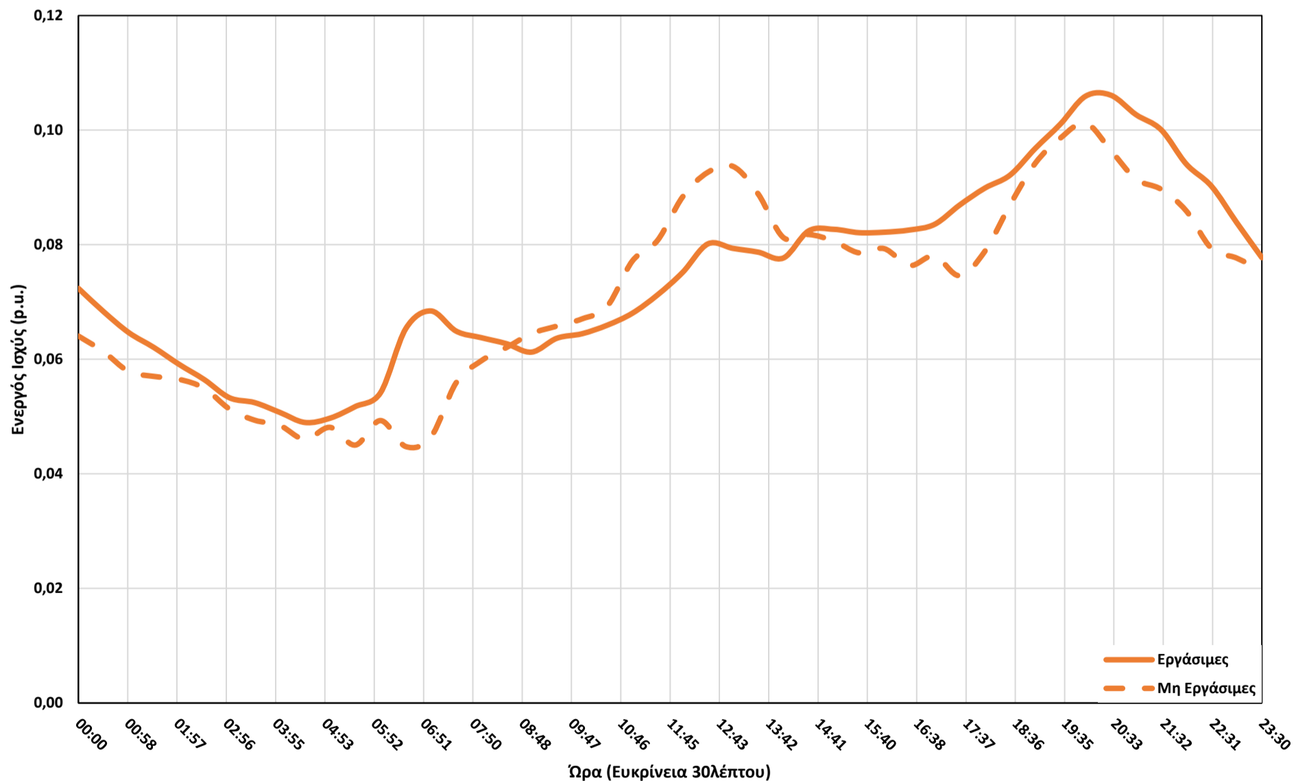
Τυπικό Προφίλ Ενεργού Ισχύος Οικιακών Καταναλωτών για το Φθινόπωρο
