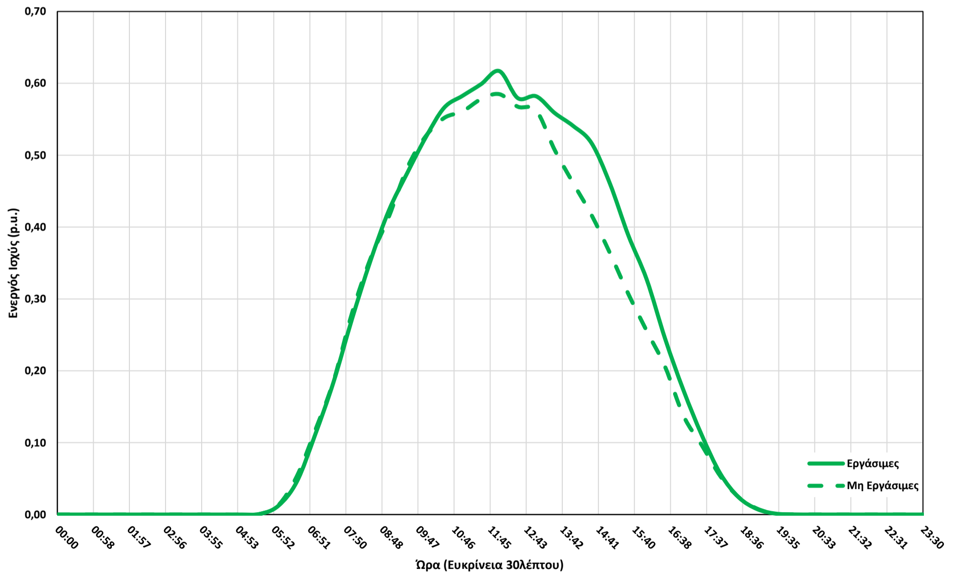
Τυπικό Προφίλ Ενεργού Ισχύος ΦΒ Συστημάτων σε στέγη (P >= 500kWp) για την Άνοιξη
