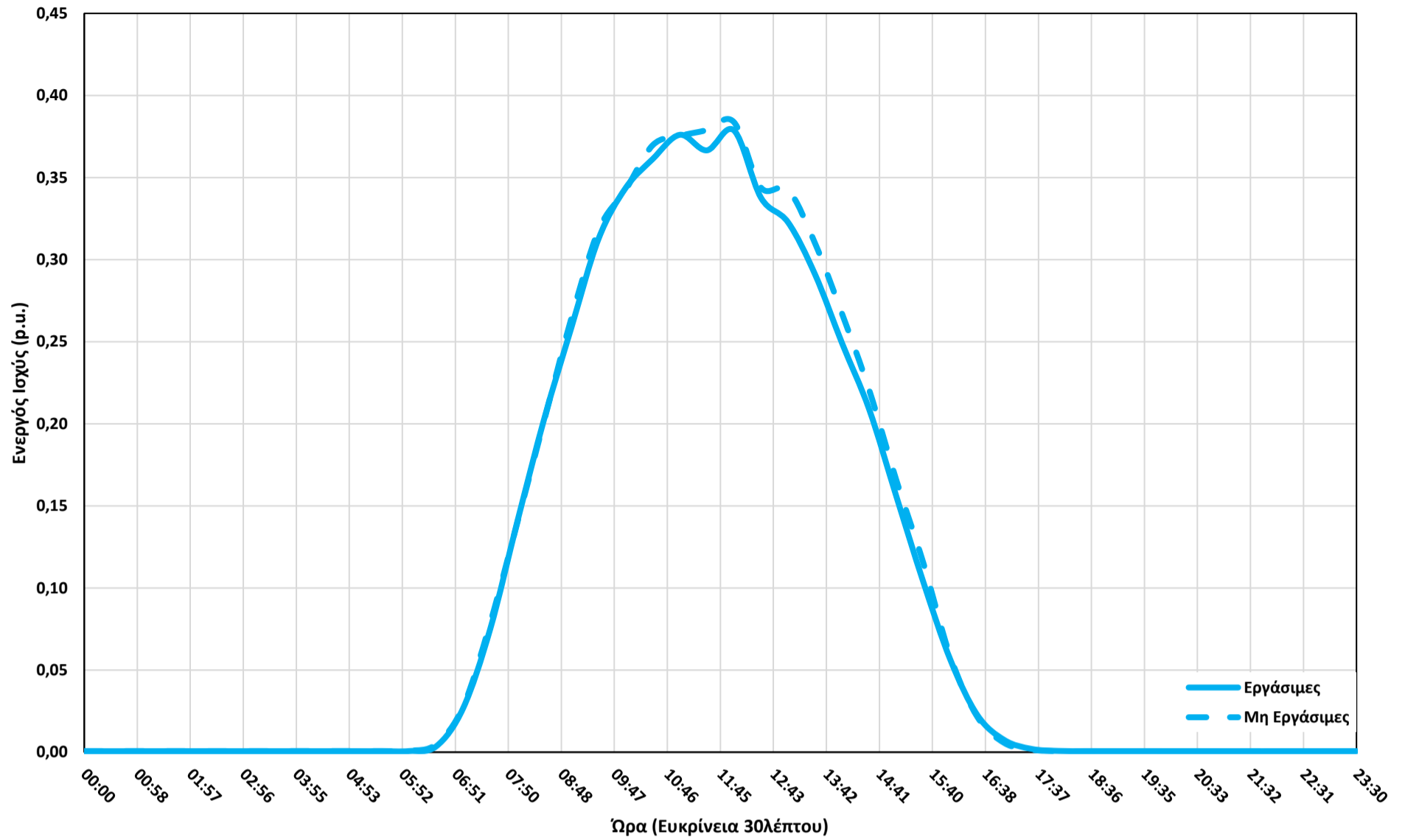
Τυπικό Προφίλ Ενεργού Ισχύος ΦΒ Συστημάτων σε στέγη (P >= 500kWp) για το Χειμώνα
