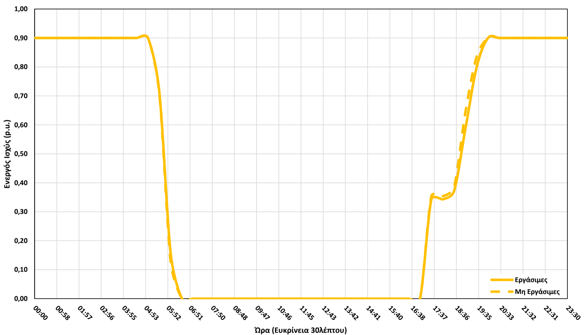
Τυπικό Προφίλ Ενεργού Ισχύος Οδικού Φωτισμού για το Φθινόπωρο
