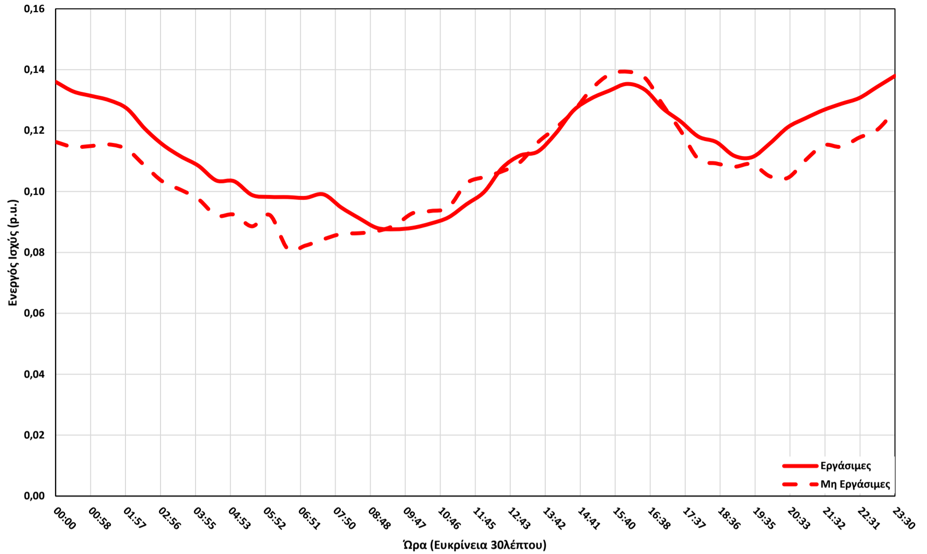
Τυπικό Προφίλ Ενεργού Ισχύος Οικιακών Καταναλωτών για το Καλοκαίρι
