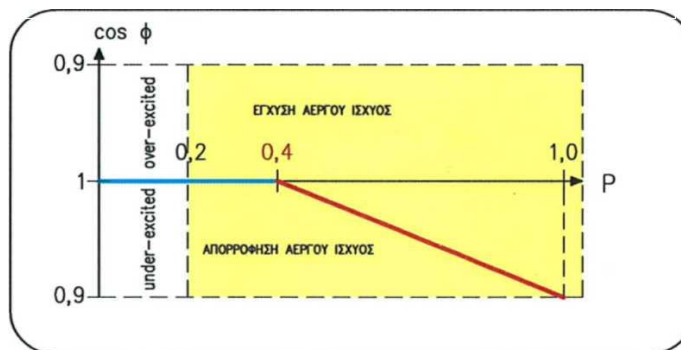
ΧΑΡΑΚΤΗΡΙΣΤΙΚΗ ΚΑΜΠΥΛΗ ΔΙΑΚΥΜΑΝΣΗΣ ΤΟΥ ΣΥΝΤΕΛΕΣΤΗ ΙΣΧΥΟΣ ΣΕ ΣΥΝΑΡΤΗΣΗ ΜΕ ΤΗΝ ΜΕΤΑΒΟΛΗ ΤΗΣ ΠΑΡΑΓΩΓΗΣ ΕΝΕΡΓΟΥ ΙΣΧΥΟΣ
