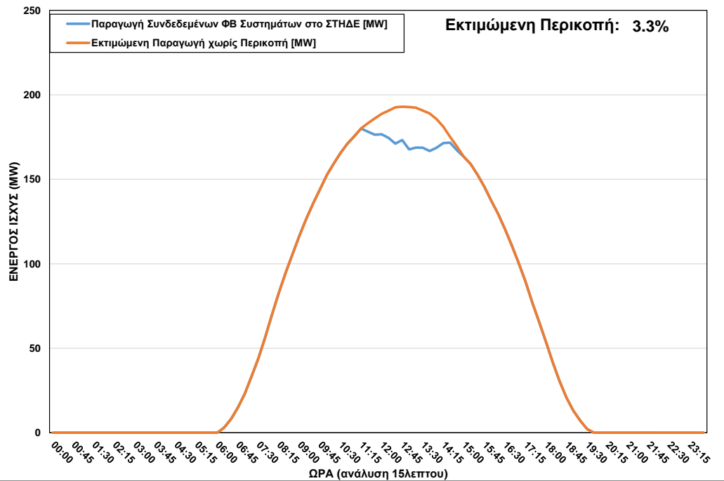
ΦΒ Παραγωγή στο ΣΤΗΔΕ κατά τη διάρκεια περικοπής στις 15/05/2023 ώρα 11:15 – 14:45
