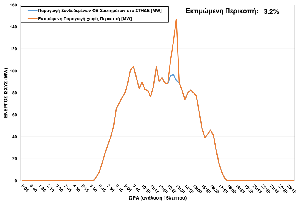
ΦΒ Παραγωγή στο ΣΤΗΔΕ κατά τη διάρκεια περικοπής στις 14-03-23 ώρα 13:00 – 13:30
