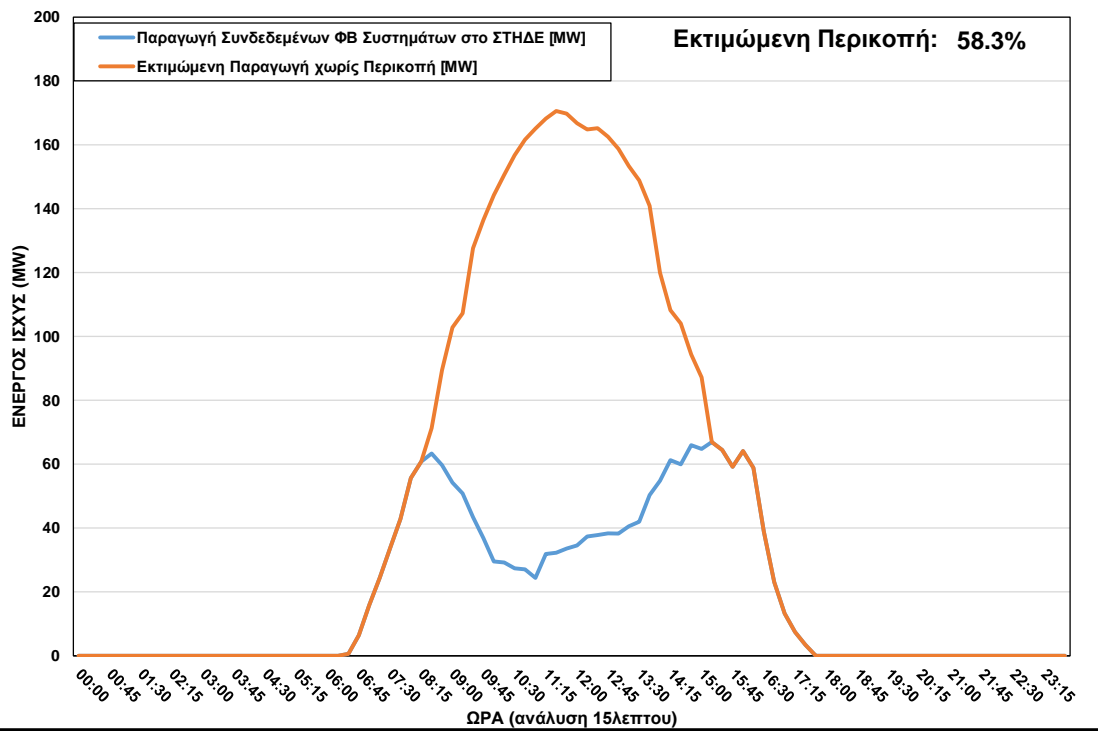
ΦΒ Παραγωγή στο ΣΤΗΔΕ κατά τη διάρκεια περικοπής στις 05/03/2023 ώρα 08:15 – 15:00
