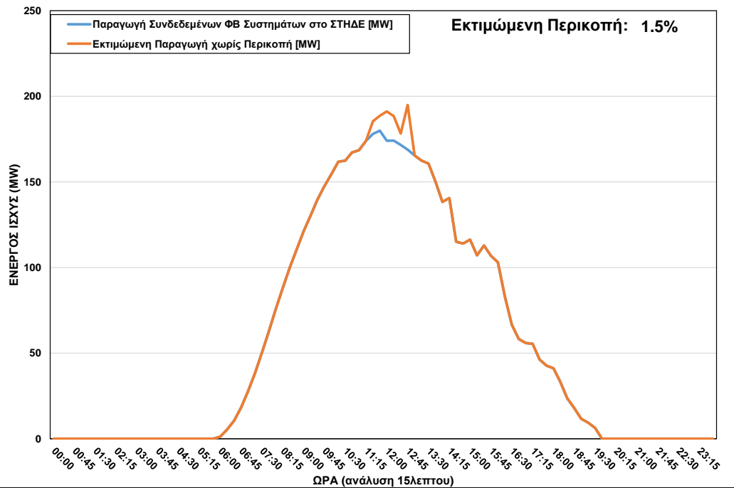
ΦΒ Παραγωγή στο ΣΤΗΔΕ κατά τη διάρκεια περικοπής στις 26/05/2023 ώρα 11:30 – 12:45
