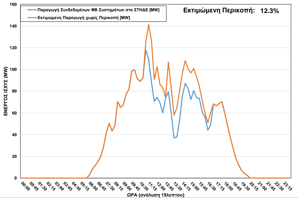
ΦΒ Παραγωγή στο ΣΤΗΔΕ κατά τη διάρκεια περικοπής στις 27/05/2023 ώρα 11:00 – 16:45
