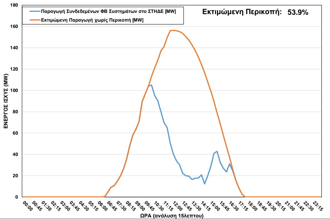
ΦΒ Παραγωγή στο ΣΤΗΔΕ κατά τη διάρκεια περικοπής στις 27/02/2023 ώρα 09:45 – 16:45
