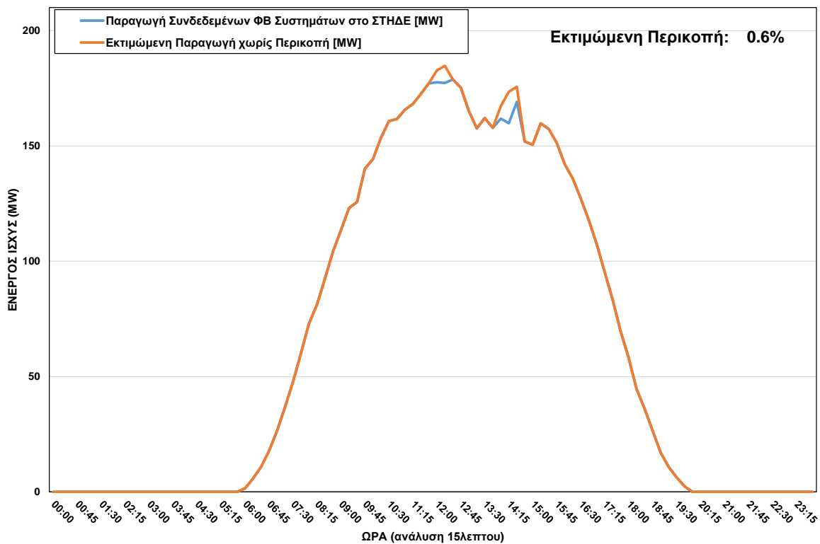
ΦΒ Παραγωγή στο ΣΤΗΔΕ κατά τη διάρκεια περικοπής στις 14/06/2023 ώρα 12:00 - 14:30
