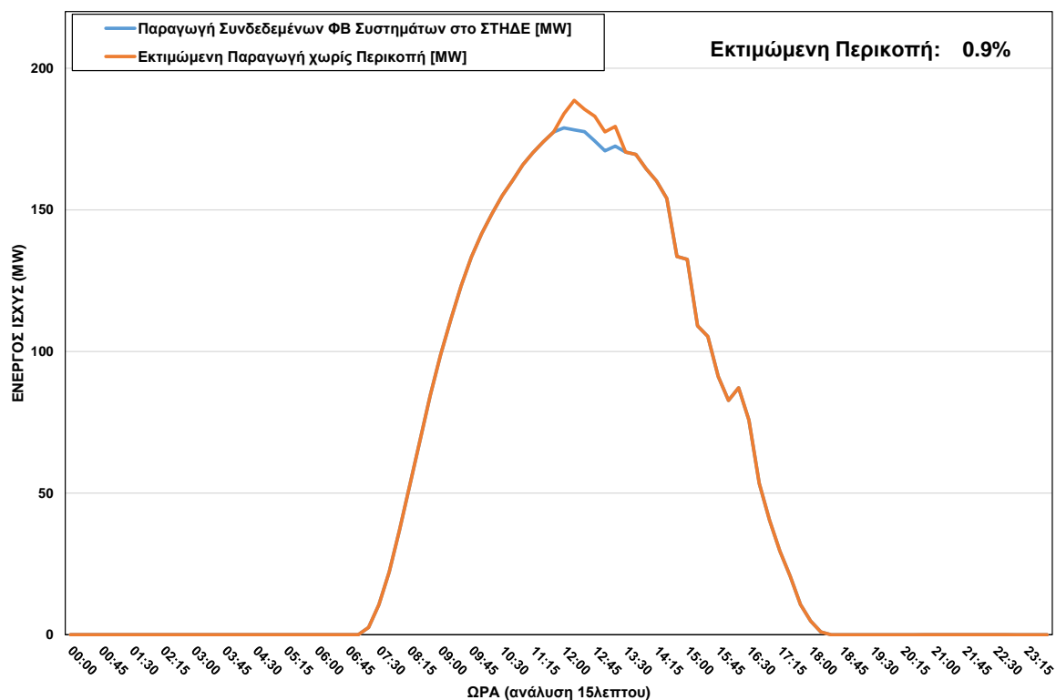
ΦΒ Παραγωγή στο ΣΤΗΔΕ κατά τη διάρκεια περικοπής στις 13/10/2023 ώρα 12:00 - 13:15
