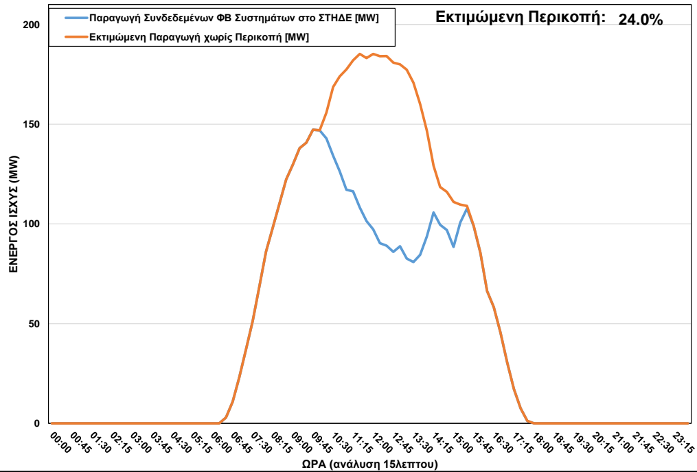
ΦΒ Παραγωγή στο ΣΤΗΔΕ κατά τη διάρκεια περικοπής στις 09/03/2023 ώρα 10:00 – 16:00
