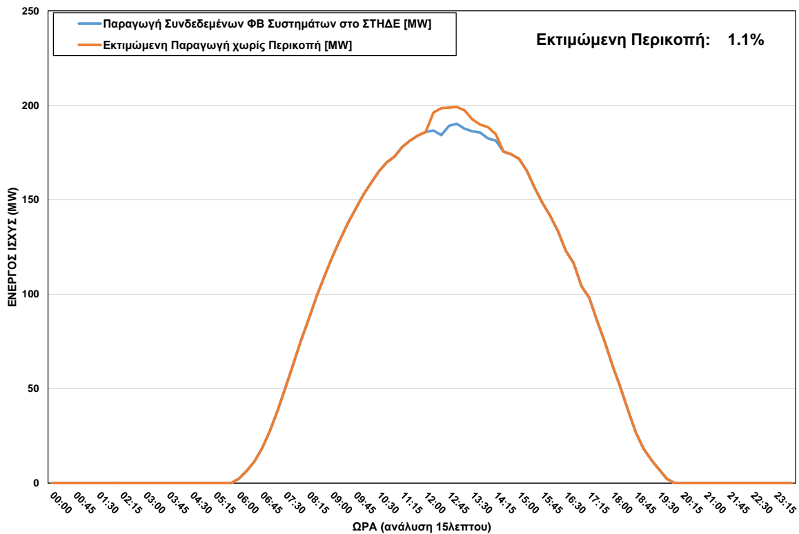
ΦΒ Παραγωγή στο ΣΤΗΔΕ κατά τη διάρκεια περικοπής στις 07/06/2023 ώρα 12:15 - 14:15
