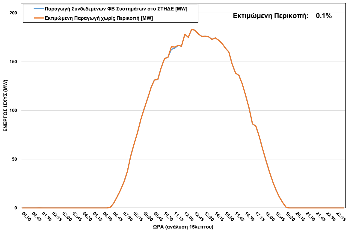
ΦΒ Παραγωγή στο ΣΤΗΔΕ κατά τη διάρκεια περικοπής στις 13/08/2023 ώρα 11:00 - 11:15
