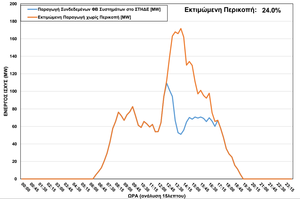
ΦΒ Παραγωγή στο ΣΤΗΔΕ κατά τη διάρκεια περικοπής στις 27/04/2023 ώρα 12:45 – 17:00
