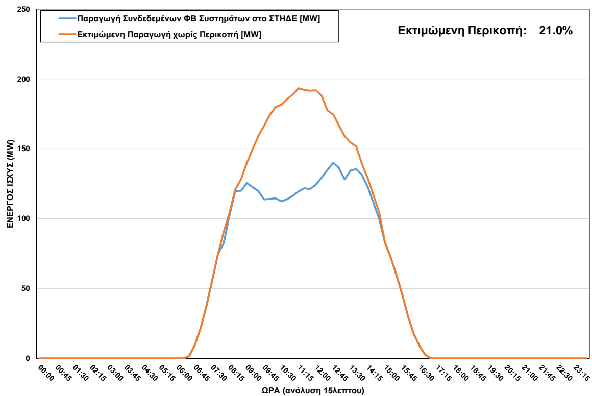
ΦΒ Παραγωγή στο ΣΤΗΔΕ κατά τη διάρκεια περικοπής στις 05/11/2023 ώρα 07:45 - 14:45
