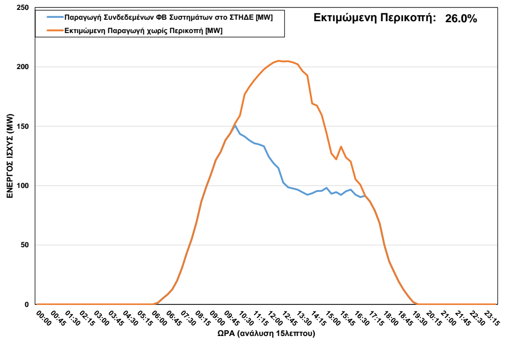
ΦΒ Παραγωγή στο ΣΤΗΔΕ κατά τη διάρκεια περικοπής στις 12/05/2023 ώρα 10:15 – 16:45
