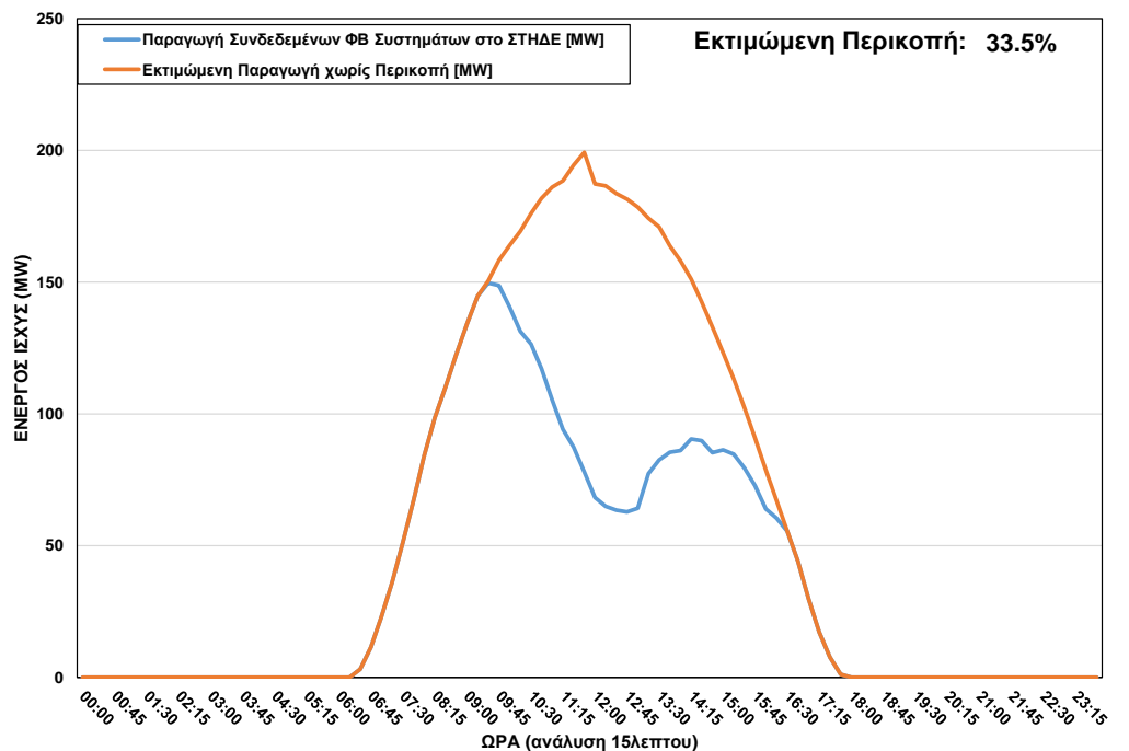
ΦΒ Παραγωγή στο ΣΤΗΔΕ κατά τη διάρκεια περικοπής στις 10/03/2023 ώρα 09:30 – 16:30
