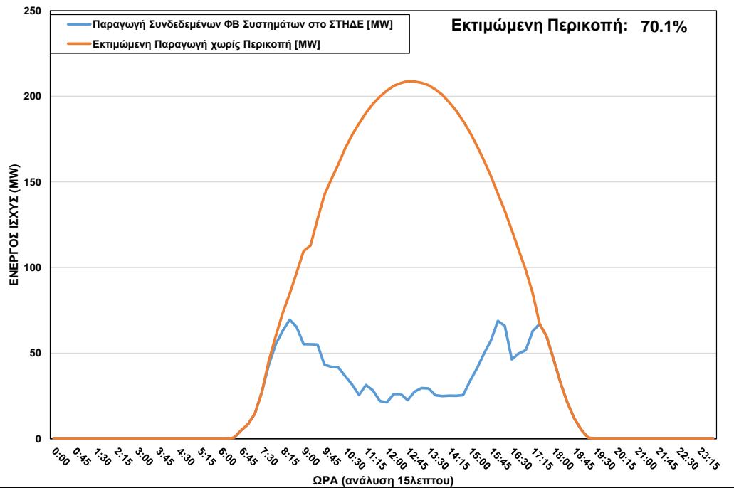
ΦΒ Παραγωγή στο ΣΤΗΔΕ κατά τη διάρκεια περικοπής στις 17-04-23 ώρα 7:45 - 17:15
