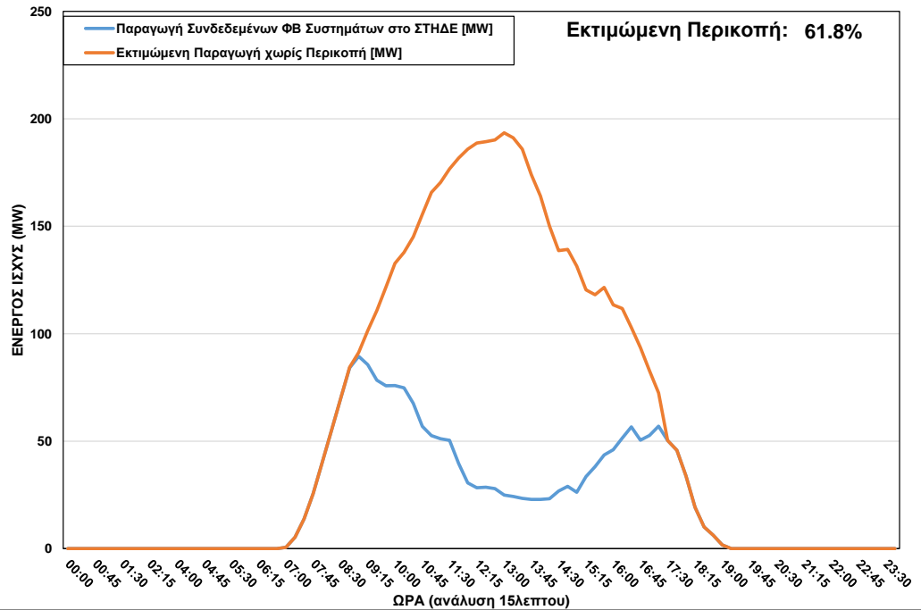
ΦΒ Παραγωγή στο ΣΤΗΔΕ κατά τη διάρκεια περικοπής στις 26/03/2023 ώρα 08:45 – 17:15
