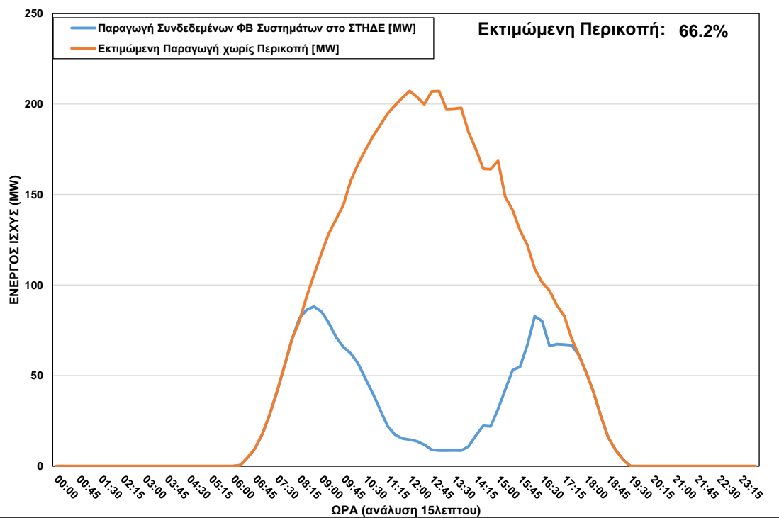
ΦΒ Παραγωγή στο ΣΤΗΔΕ κατά τη διάρκεια περικοπής στις 01/05/2023 ώρα 08:15 – 17:30
