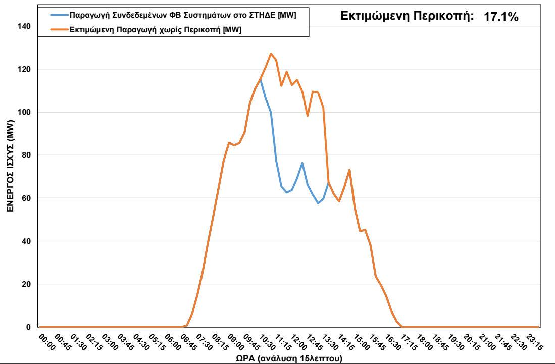
ΦΒ Παραγωγή στο ΣΤΗΔΕ κατά τη διάρκεια περικοπής στις 04/02/2023 ώρα 10:30 – 13:30
