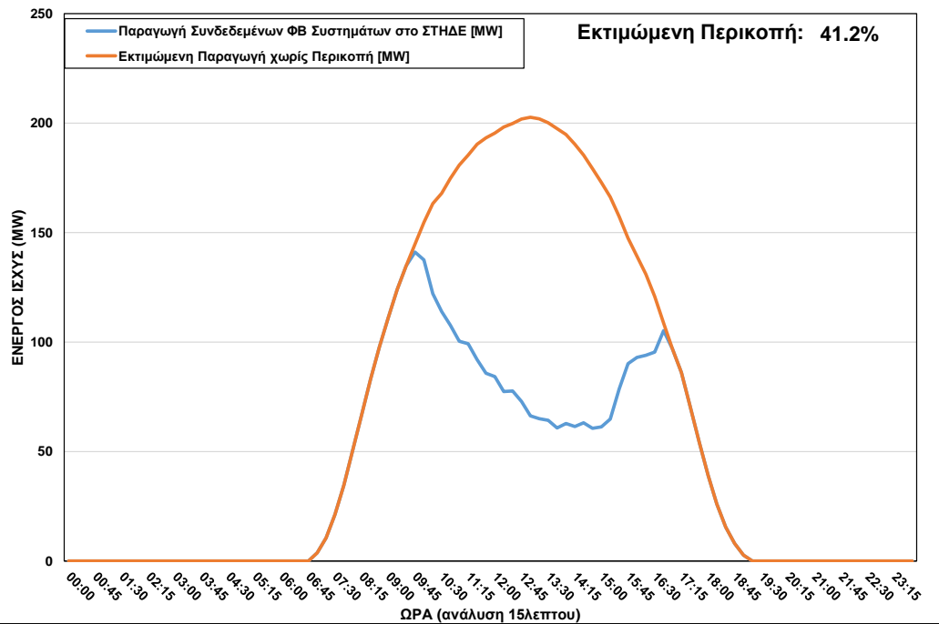
ΦΒ Παραγωγή στο ΣΤΗΔΕ κατά τη διάρκεια περικοπής στις 04/04/2023 ώρα 09:45 – 16:45
