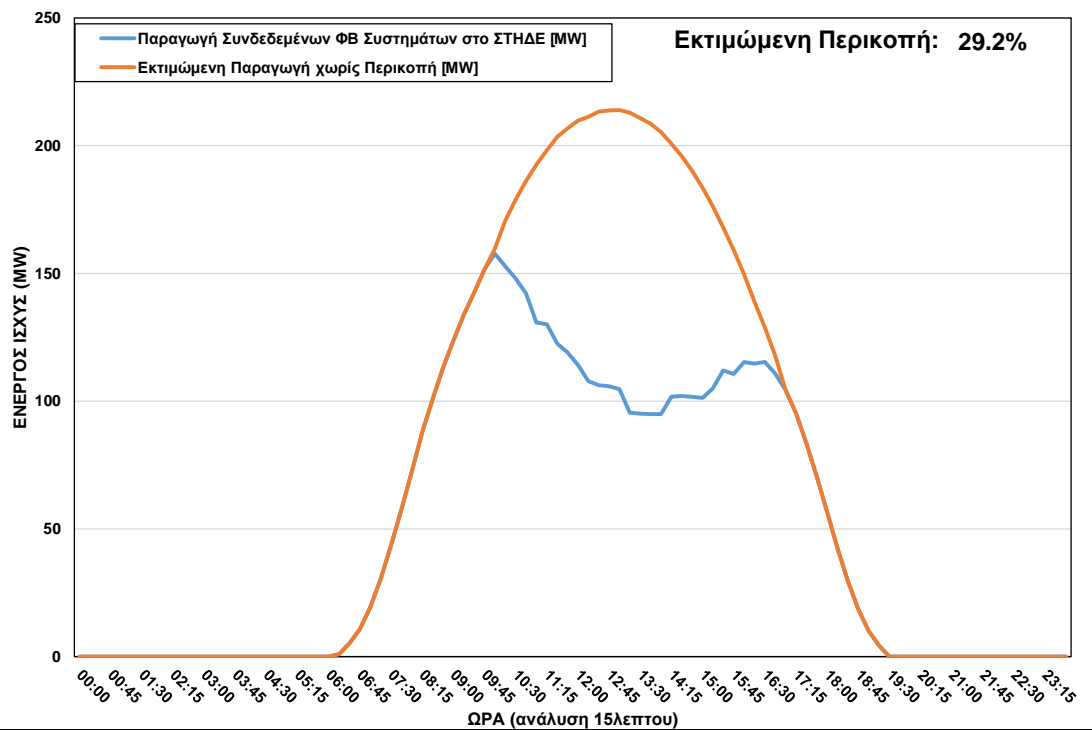
ΦΒ Παραγωγή στο ΣΤΗΔΕ κατά τη διάρκεια περικοπής στις 03/05/2023 ώρα 10:00 – 16:45
