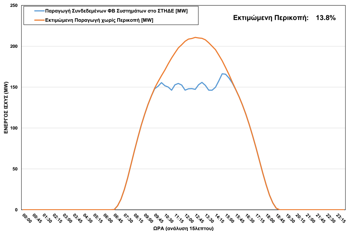
ΦΒ Παραγωγή στο ΣΤΗΔΕ κατά τη διάρκεια περικοπής στις 17/09/2023 ώρα 09:45 - 15:45
