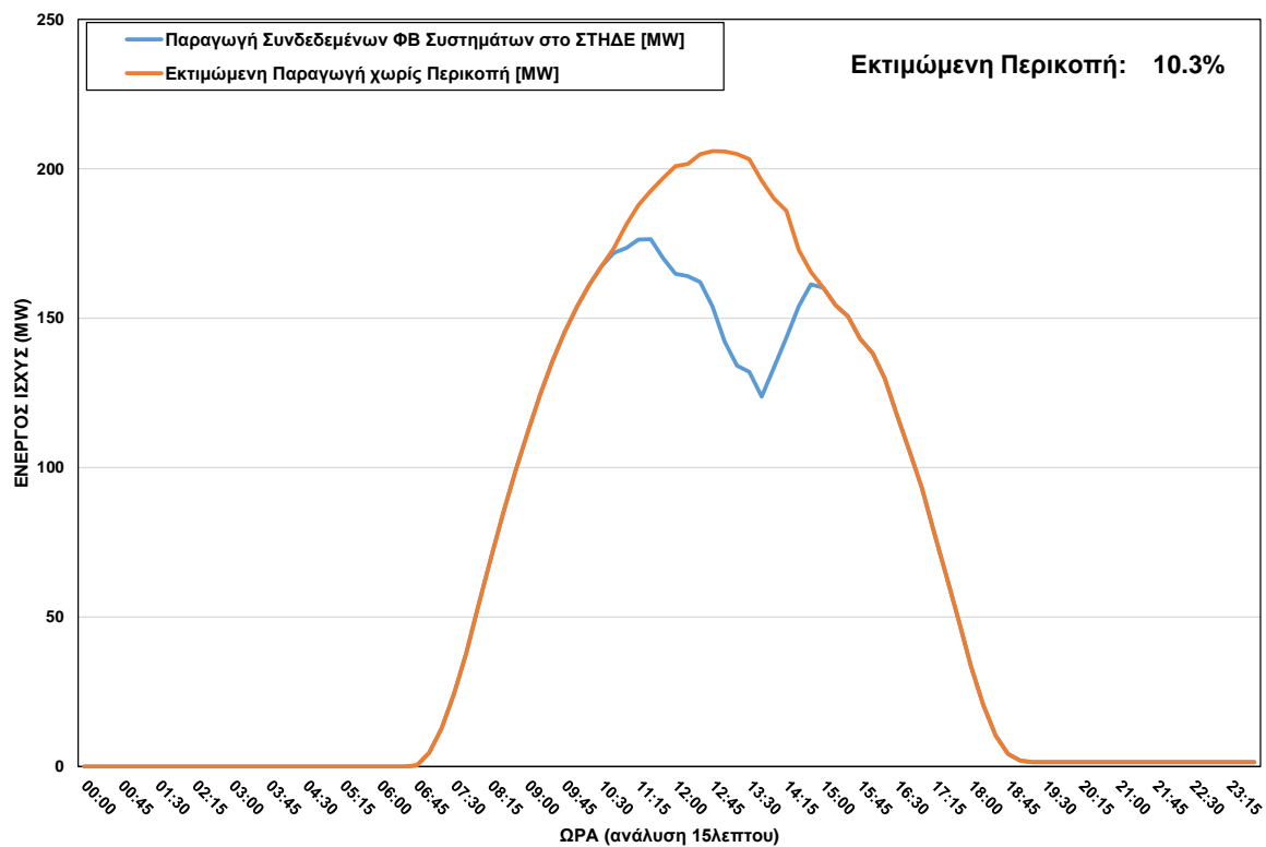
ΦΒ Παραγωγή στο ΣΤΗΔΕ κατά τη διάρκεια περικοπής στις 14/09/2023 ώρα 10:45 - 14:45
