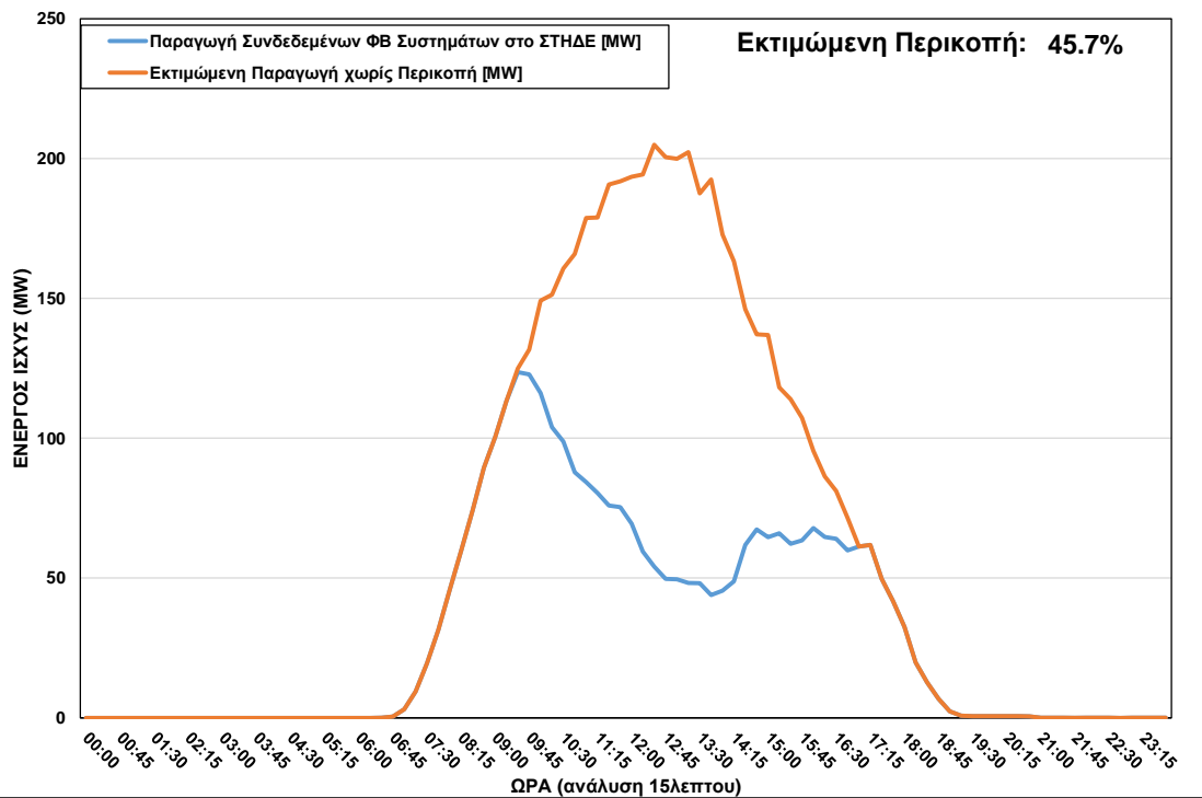
ΦΒ Παραγωγή στο ΣΤΗΔΕ κατά τη διάρκεια περικοπής στις 01/04/2023 ώρα 09:30 – 16:45
