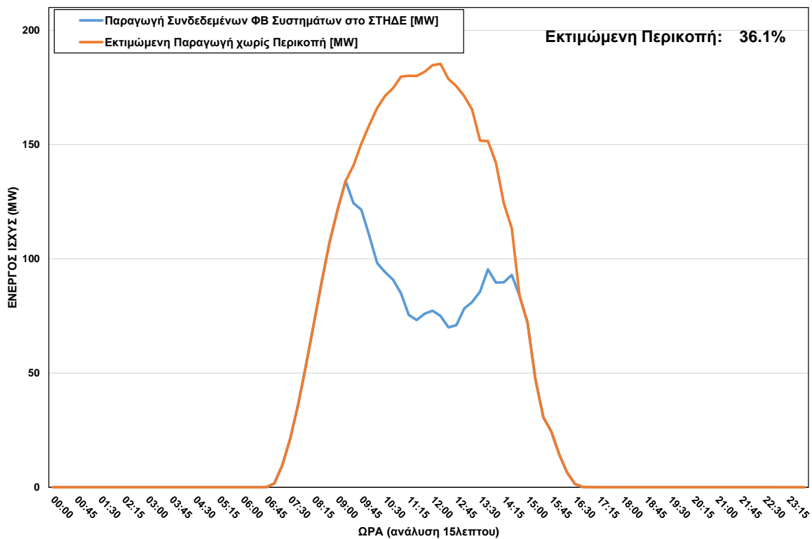
ΦΒ Παραγωγή στο ΣΤΗΔΕ κατά τη διάρκεια περικοπής στις 04/12/2023 ώρα 09:30 - 14:30
