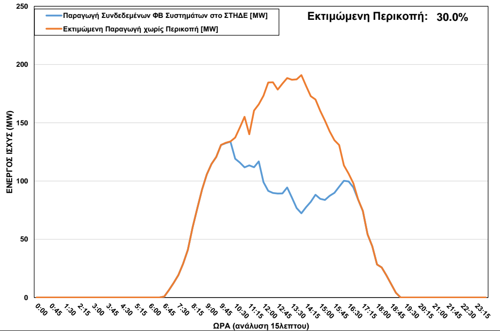
ΦΒ Παραγωγή στο ΣΤΗΔΕ κατά τη διάρκεια περικοπής στις 11-04-23 ώρα 9:45 - 17:15
