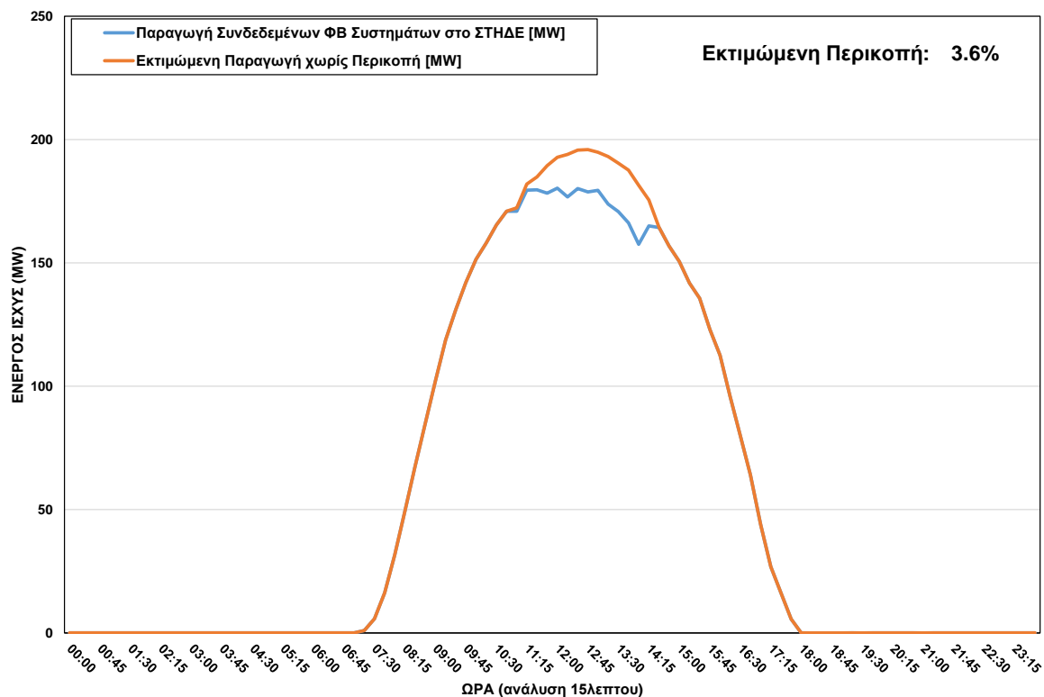
ΦΒ Παραγωγή στο ΣΤΗΔΕ κατά τη διάρκεια περικοπής στις 25/10/2023 ώρα 11:00 - 14:15
