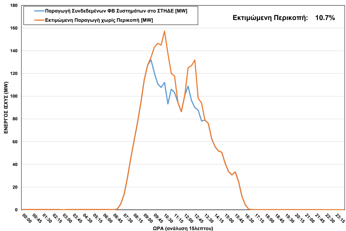
ΦΒ Παραγωγή στο ΣΤΗΔΕ κατά τη διάρκεια περικοπής στις 22/12/2023 ώρα 09:15 - 13:15
