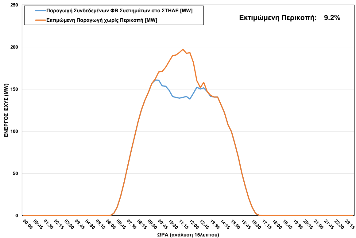
ΦΒ Παραγωγή στο ΣΤΗΔΕ κατά τη διάρκεια περικοπής στις 03/11/2023 ώρα 09:15 - 13:30
