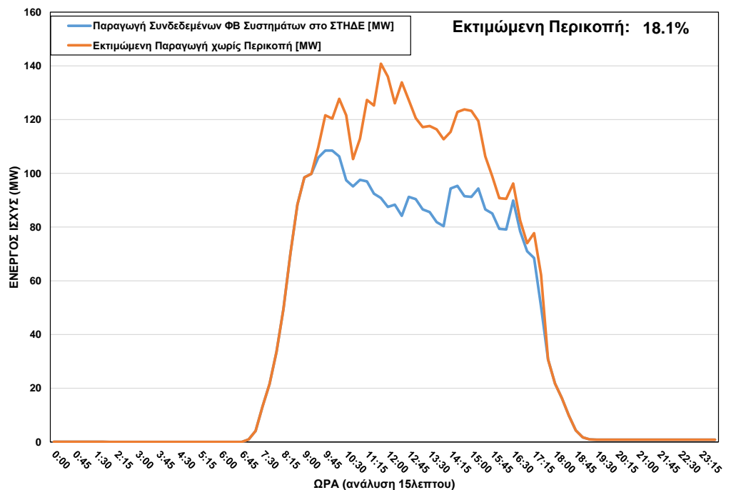
ΦΒ Παραγωγή στο ΣΤΗΔΕ κατά τη διάρκεια περικοπής στις 29-03-23 ώρα 9:30 - 17:30
