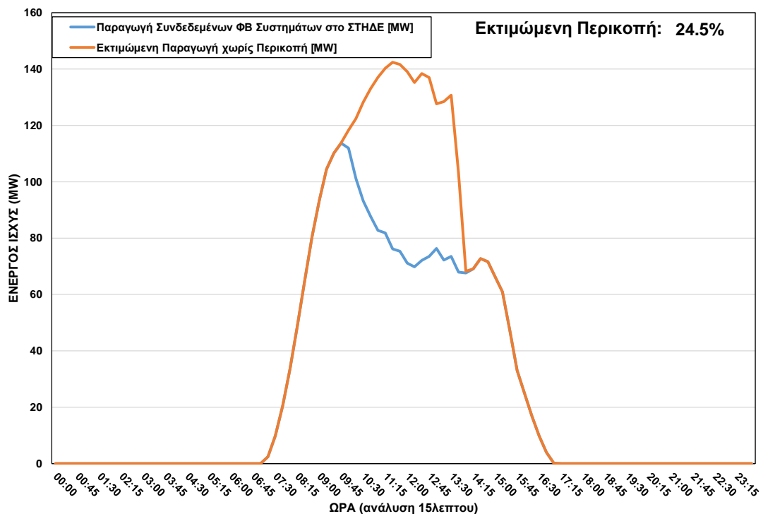
ΦΒ Παραγωγή στο ΣΤΗΔΕ κατά τη διάρκεια περικοπής στις 19/01/2023 ώρα 09:45 – 13:45
