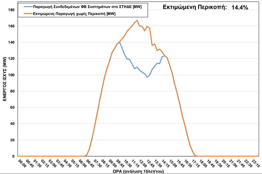
ΦΒ Παραγωγή στο ΣΤΗΔΕ κατά τη διάρκεια περικοπής στις 22/02/2023 ώρα 09:45 – 14:15
