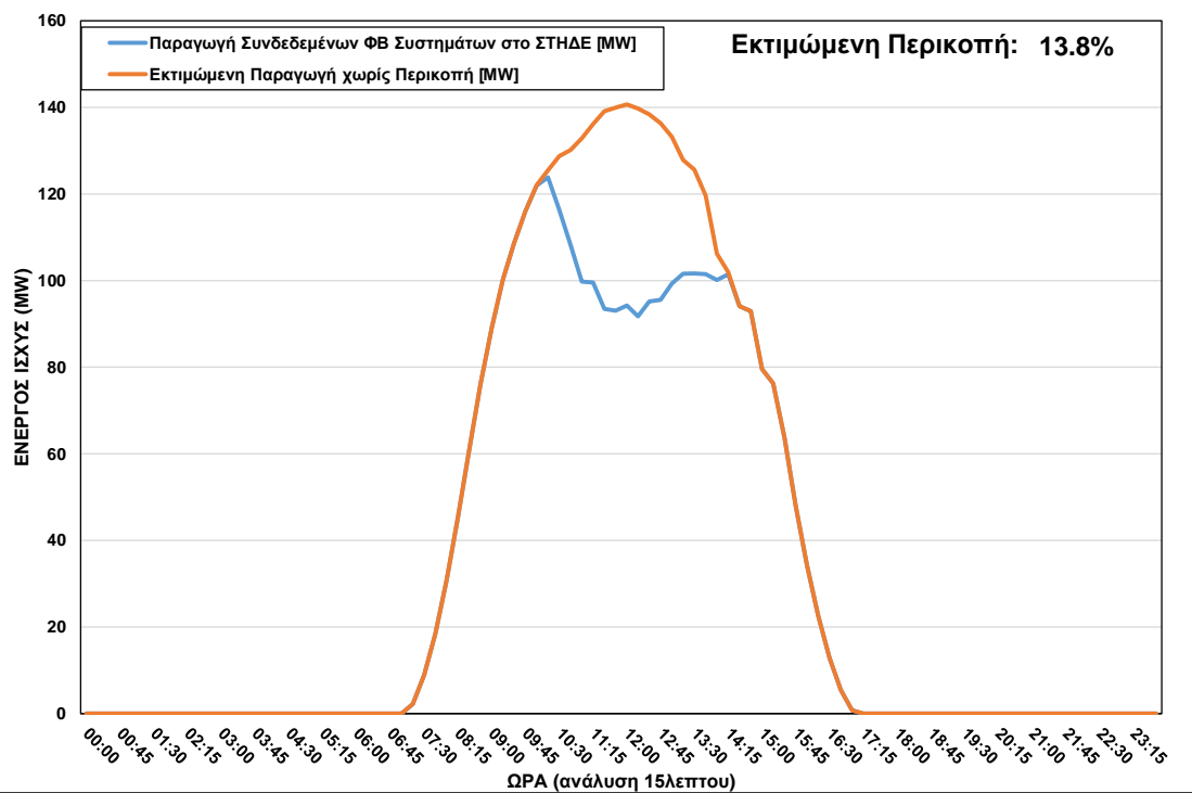
ΦΒ Παραγωγή στο ΣΤΗΔΕ κατά τη διάρκεια περικοπής στις 21/01/2023 ώρα 10:00 – 14:15
