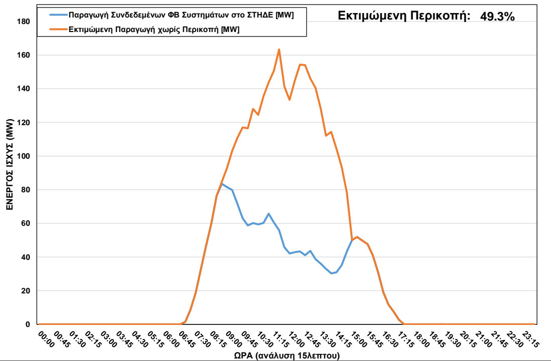
ΦΒ Παραγωγή στο ΣΤΗΔΕ κατά τη διάρκεια περικοπής στις 12/02/2023 ώρα 08:30 – 14:45
