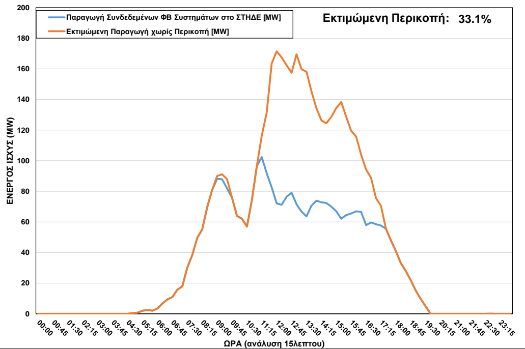
ΦΒ Παραγωγή στο ΣΤΗΔΕ κατά τη διάρκεια περικοπής στις 28/05/2023 ώρα 08:45 – 17:15
