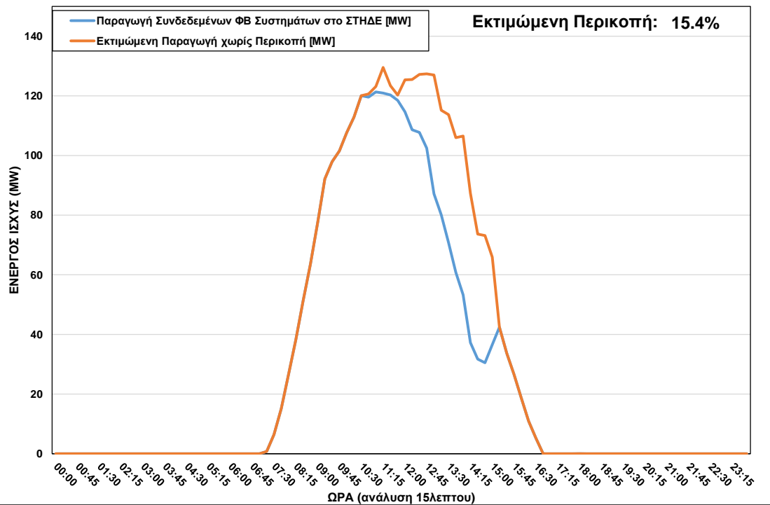
ΦΒ Παραγωγή στο ΣΤΗΔΕ κατά τη διάρκεια περικοπής στις 06/01/2023 ώρα 10:45 – 15:00
