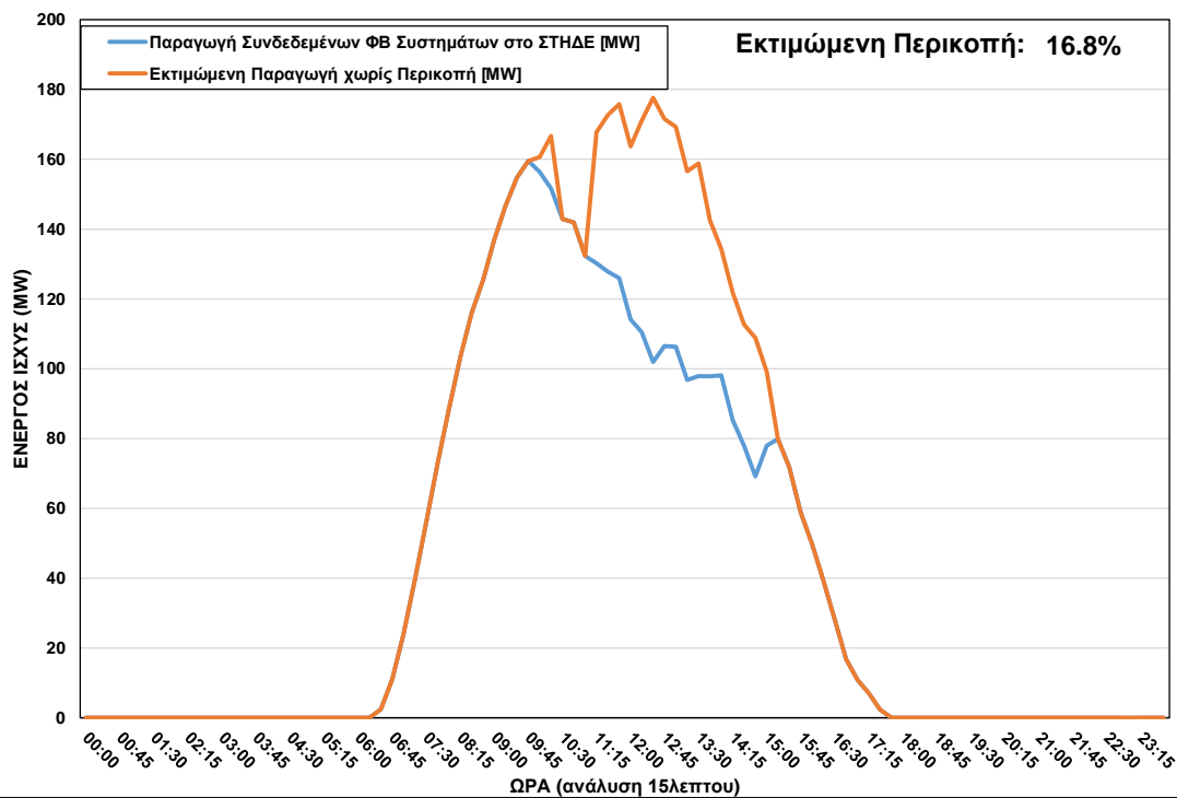
ΦΒ Παραγωγή στο ΣΤΗΔΕ κατά τη διάρκεια περικοπής στις 07/03/2023 ώρα 10:00 – 15:00
