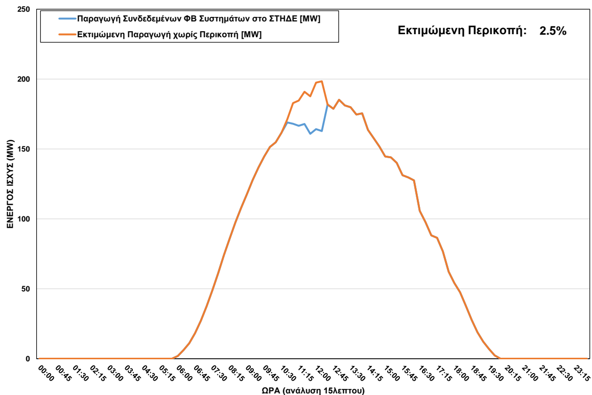
ΦΒ Παραγωγή στο ΣΤΗΔΕ κατά τη διάρκεια περικοπής στις 06/06/2023 ώρα 10:45 - 12:15
