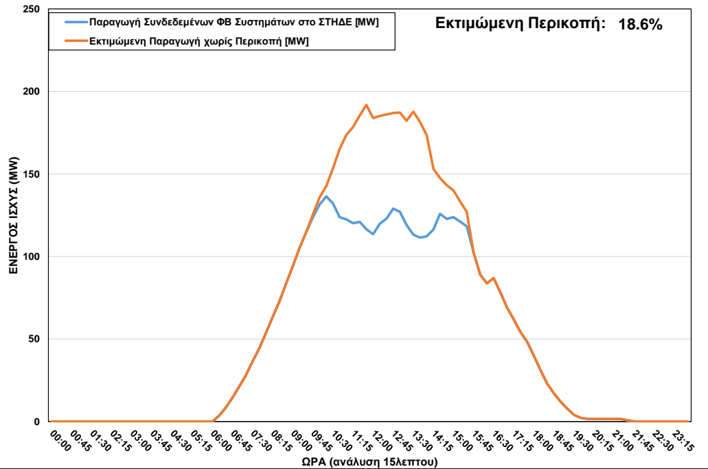
ΦΒ Παραγωγή στο ΣΤΗΔΕ κατά τη διάρκεια περικοπής στις 22/05/2023 ώρα 09:45 – 15:30
