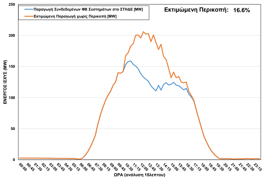
ΦΒ Παραγωγή στο ΣΤΗΔΕ κατά τη διάρκεια περικοπής στις 18/05/2023 ώρα 10:30 – 17:15
