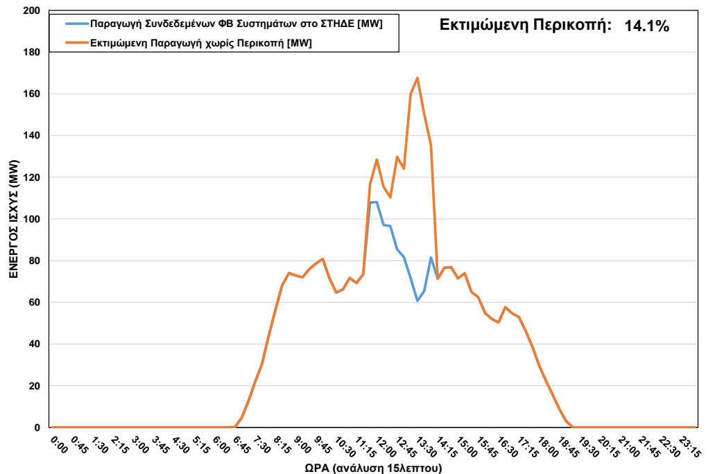
ΦΒ Παραγωγή στο ΣΤΗΔΕ κατά τη διάρκεια περικοπής στις 10-04-23 ώρα 11:45 – 14:00
