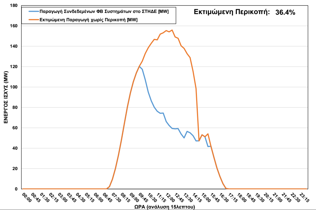
ΦΒ Παραγωγή στο ΣΤΗΔΕ κατά τη διάρκεια περικοπής στις 18/01/2023 ώρα 10:00 – 15:30
