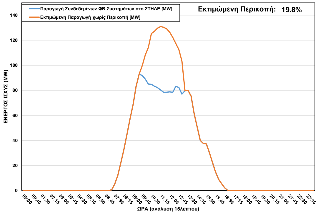
ΦΒ Παραγωγή στο ΣΤΗΔΕ κατά τη διάρκεια περικοπής στις 08/01/2023 ώρα 09:30 – 13:00
