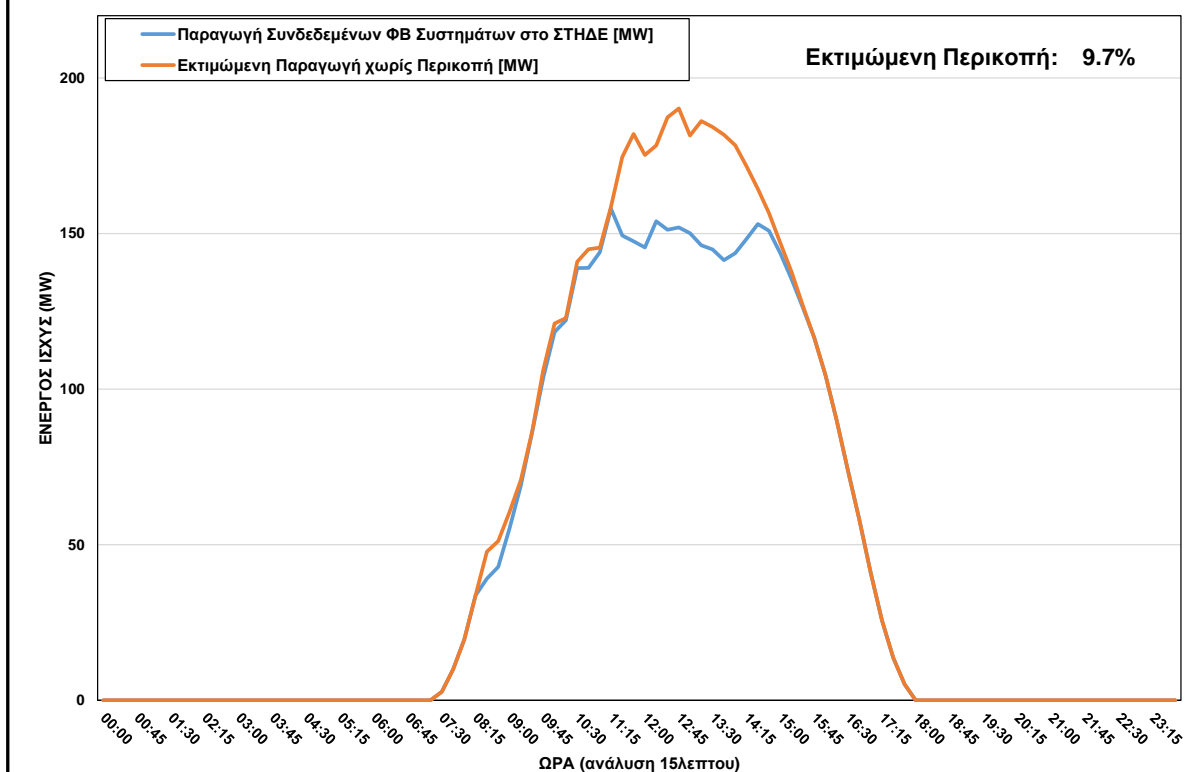
ΦΒ Παραγωγή στο ΣΤΗΔΕ κατά τη διάρκεια περικοπής στις 27/10/2023 ώρα 08:30 - 15:30
