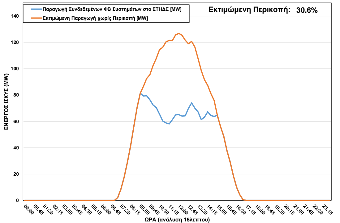
ΦΒ Παραγωγή στο ΣΤΗΔΕ κατά τη διάρκεια περικοπής στις 22/01/2023 ώρα 09:00 – 14:45
