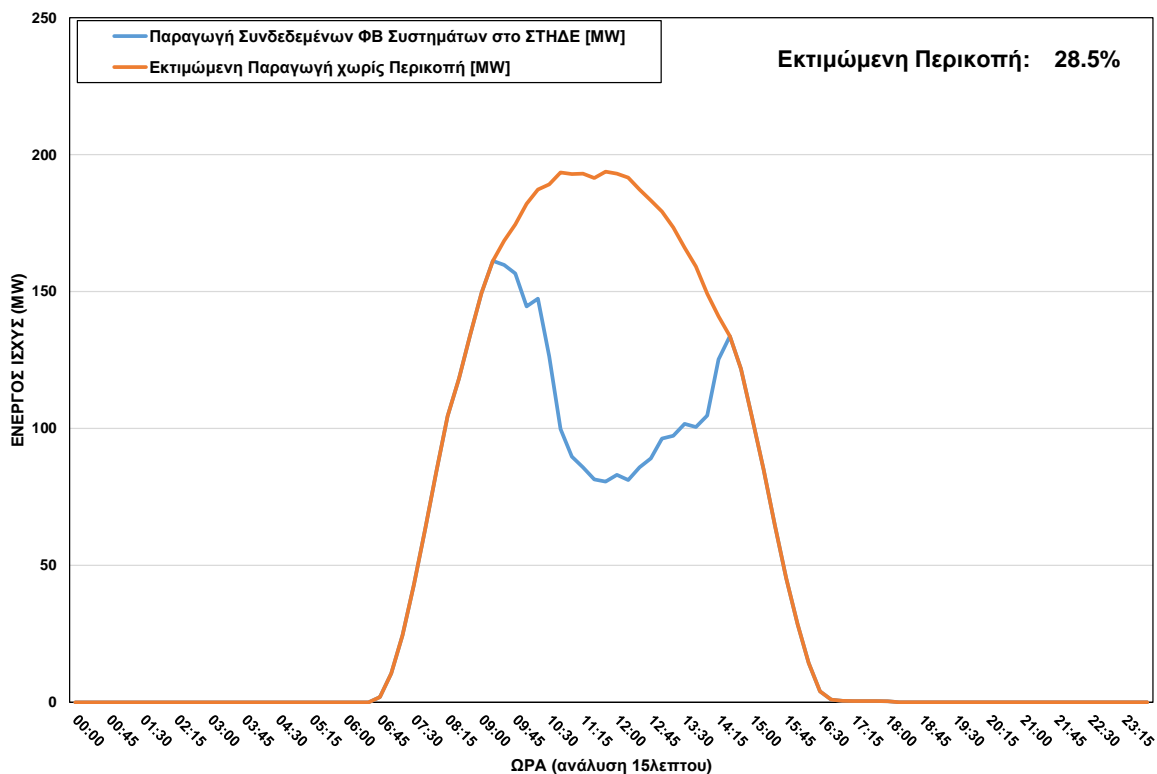
ΦΒ Παραγωγή στο ΣΤΗΔΕ κατά τη διάρκεια περικοπής στις 21/11/2023 ώρα 09:15 - 14:15
