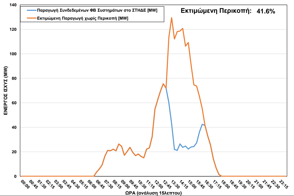
ΦΒ Παραγωγή στο ΣΤΗΔΕ κατά τη διάρκεια περικοπής στις 13/03/2023 ώρα 13:15 – 16:15
