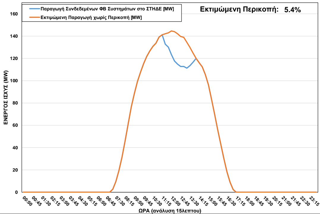
ΦΒ Παραγωγή στο ΣΤΗΔΕ κατά τη διάρκεια περικοπής στις 24/01/2023 ώρα 11:15 – 13:45
