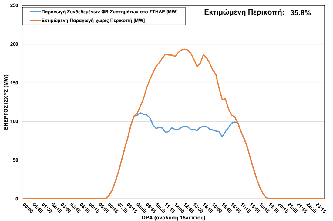
ΦΒ Παραγωγή στο ΣΤΗΔΕ κατά τη διάρκεια περικοπής στις 20/04/2023 ώρα 08:45 – 16:45
