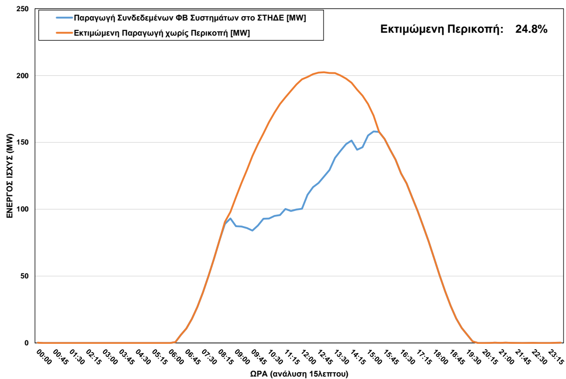
ΦΒ Παραγωγή στο ΣΤΗΔΕ κατά τη διάρκεια περικοπής στις 30/07/2023 ώρα 08:30 - 15:15
