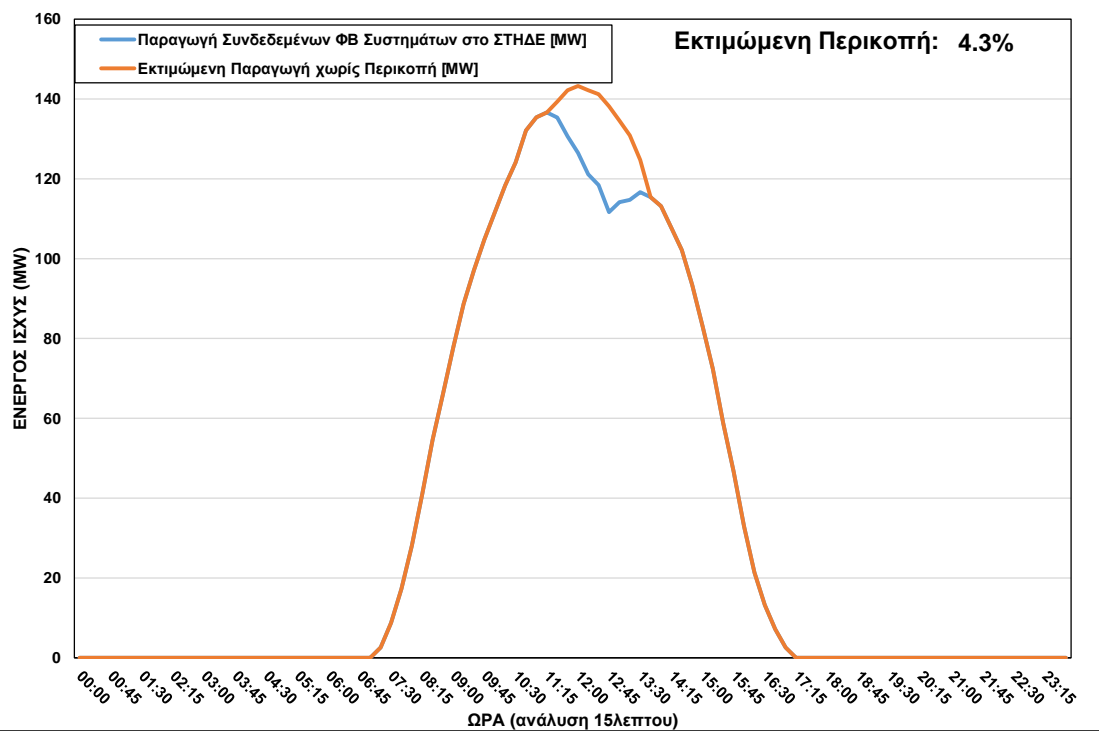
ΦΒ Παραγωγή στο ΣΤΗΔΕ κατά τη διάρκεια περικοπής στις 26/01/2023 ώρα 11:30 – 13:30
