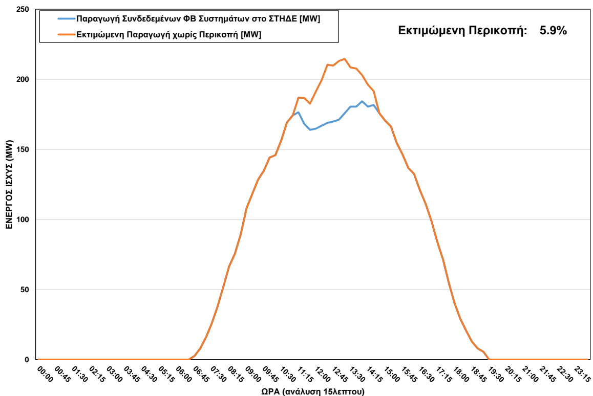
ΦΒ Παραγωγή στο ΣΤΗΔΕ κατά τη διάρκεια περικοπής στις 01/09/2023 ώρα 11:15 - 14:30
