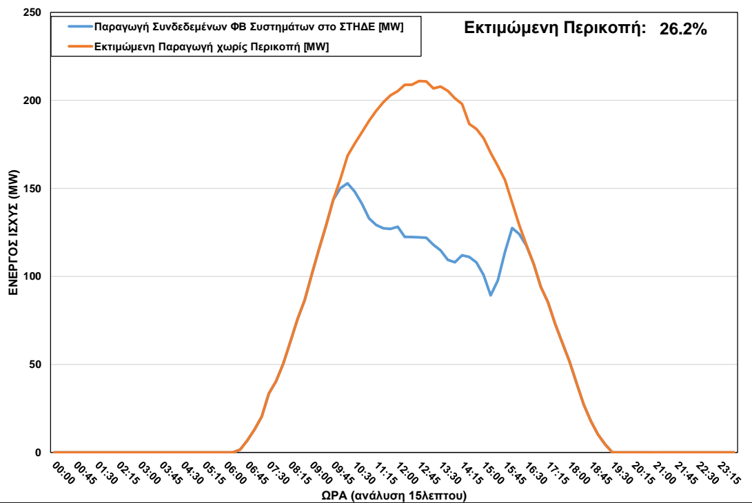
ΦΒ Παραγωγή στο ΣΤΗΔΕ κατά τη διάρκεια περικοπής στις 02/05/2023 ώρα 10:00 – 16:30
