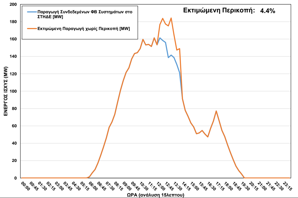
ΦΒ Παραγωγή στο ΣΤΗΔΕ κατά τη διάρκεια περικοπής στις 30/05/2023 ώρα 12:15 – 14:00
