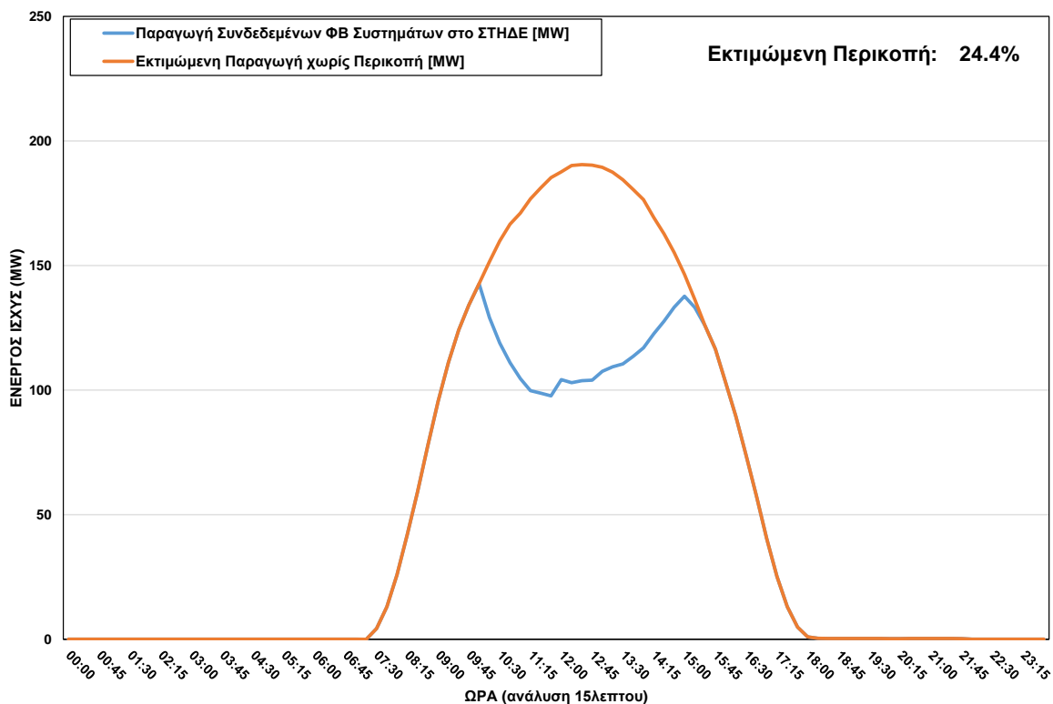
ΦΒ Παραγωγή στο ΣΤΗΔΕ κατά τη διάρκεια περικοπής στις 28/10/2023 ώρα 10:00 - 15:15
