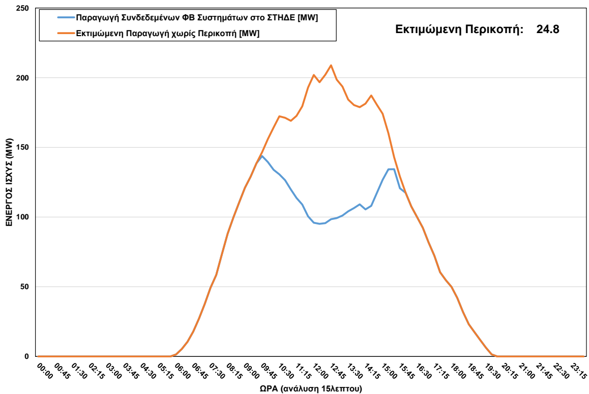
ΦΒ Παραγωγή στο ΣΤΗΔΕ κατά τη διάρκεια περικοπής στις 05/06/2023 ώρα 09:45 - 15:45
