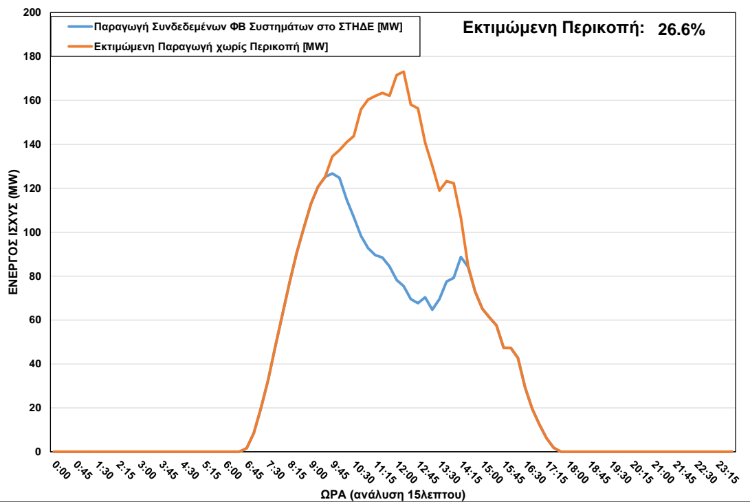
ΦΒ Παραγωγή στο ΣΤΗΔΕ κατά τη διάρκεια περικοπής στις 23-02-23 ώρα 9:30 - 14:30
