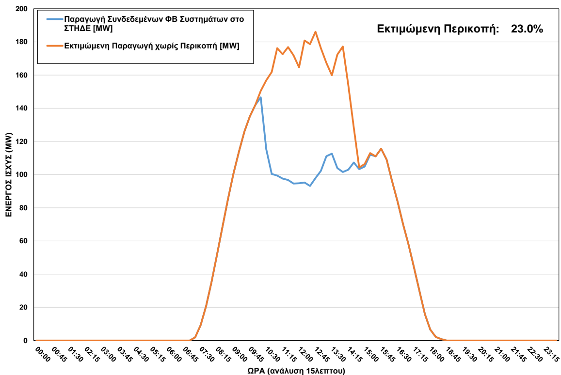
ΦΒ Παραγωγή στο ΣΤΗΔΕ κατά τη διάρκεια περικοπής στις 16/10/2023 ώρα 10:15 - 15:15
