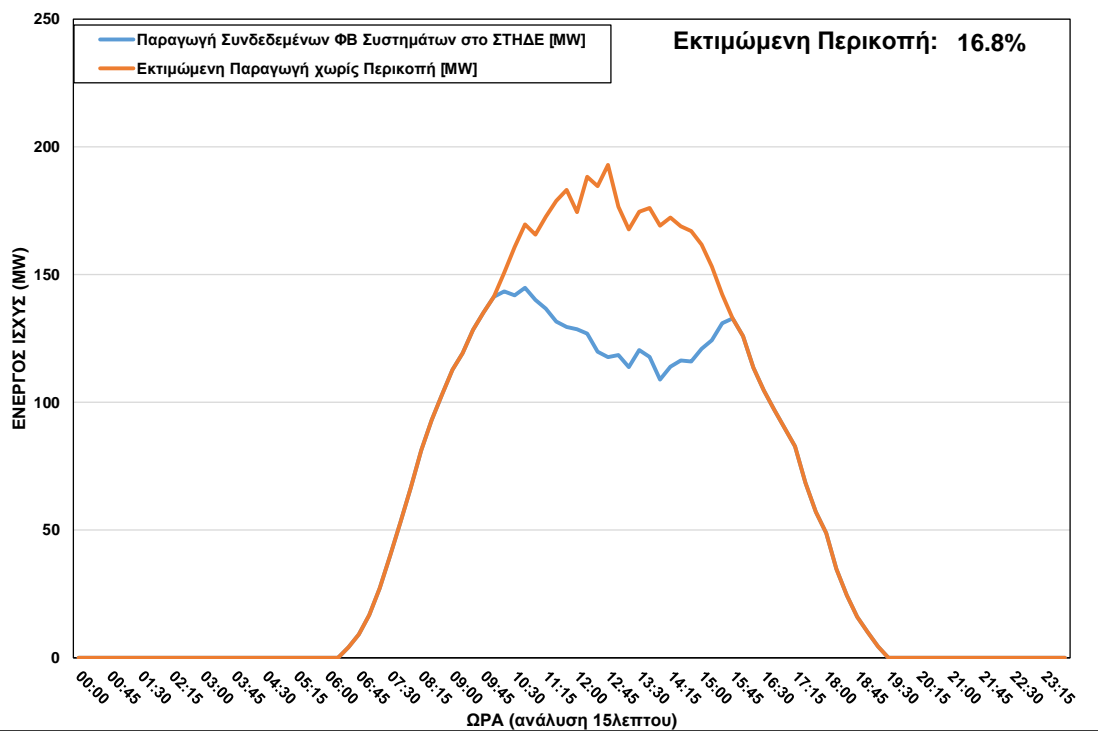
ΦΒ Παραγωγή στο ΣΤΗΔΕ κατά τη διάρκεια περικοπής στις 25/04/2023 ώρα 10:15 – 15:30
