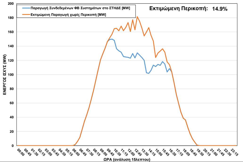
ΦΒ Παραγωγή στο ΣΤΗΔΕ κατά τη διάρκεια περικοπής στις 08/05/2023 ώρα 10:00 – 16:30
