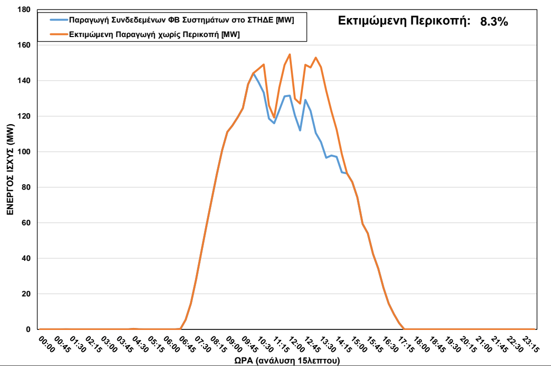
ΦΒ Παραγωγή στο ΣΤΗΔΕ κατά τη διάρκεια περικοπής στις 16/02/2023 ώρα 10:30 – 14:45
