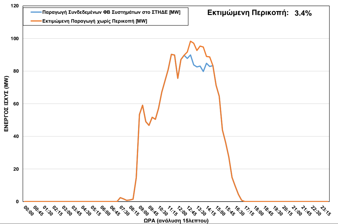
ΦΒ Παραγωγή στο ΣΤΗΔΕ κατά τη διάρκεια περικοπής στις 27/01/2023 ώρα 12:45 – 14:30
