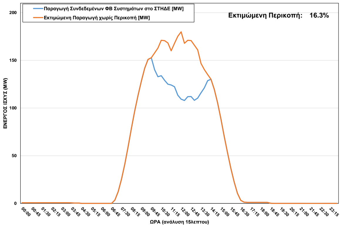
ΦΒ Παραγωγή στο ΣΤΗΔΕ κατά τη διάρκεια περικοπής στις 01/12/2023 ώρα 10:00 - 14:00
