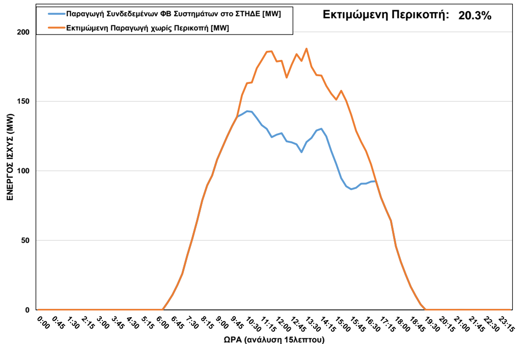
ΦΒ Παραγωγή στο ΣΤΗΔΕ κατά τη διάρκεια περικοπής στις 26-04-23 ώρα 10:15 – 16:45
