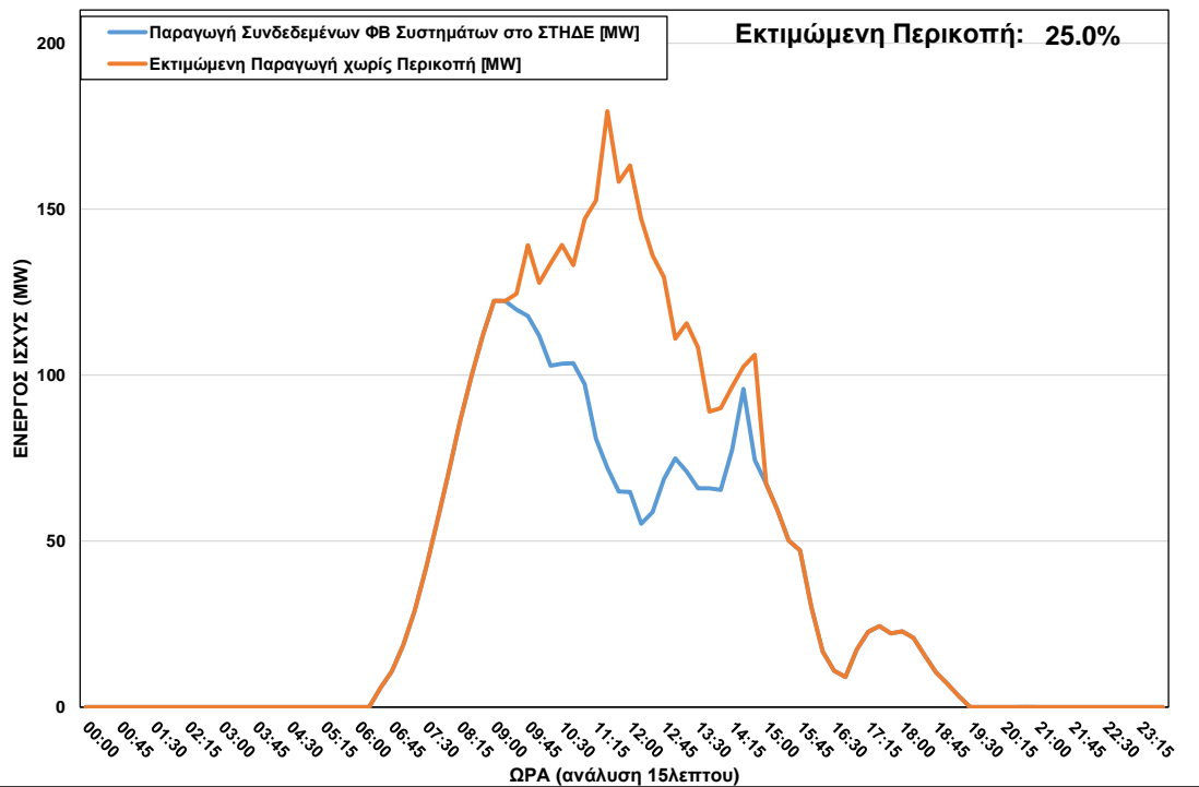
ΦΒ Παραγωγή στο ΣΤΗΔΕ κατά τη διάρκεια περικοπής στις 28/04/2023 ώρα 09:30 – 14:45
