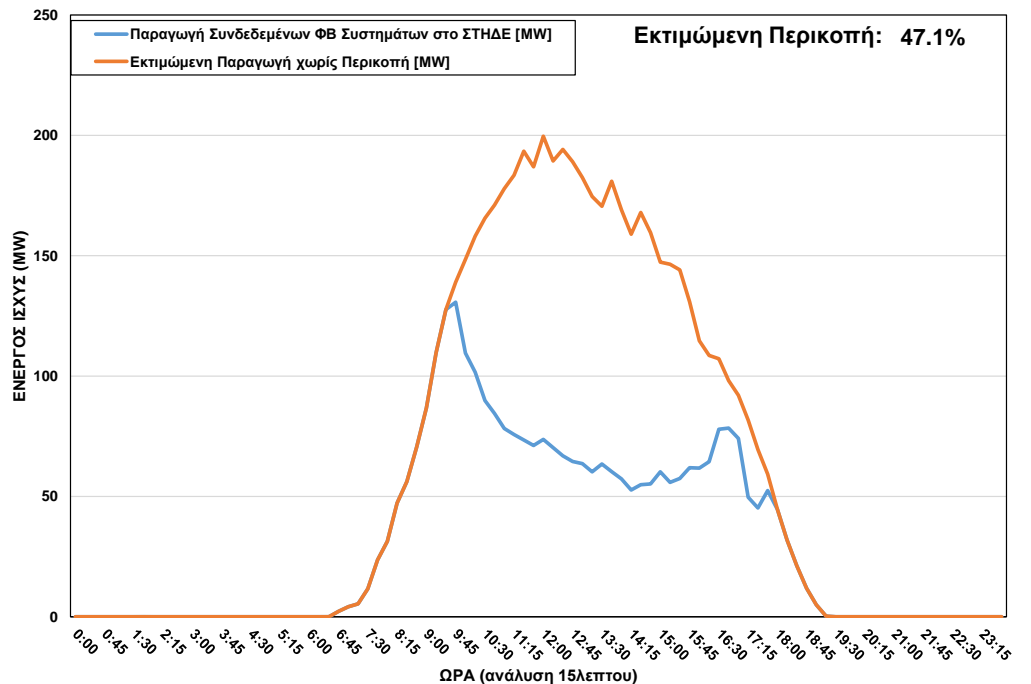
ΦΒ Παραγωγή στο ΣΤΗΔΕ κατά τη διάρκεια περικοπής στις 13-04-23 ώρα 9:45 - 17:45
