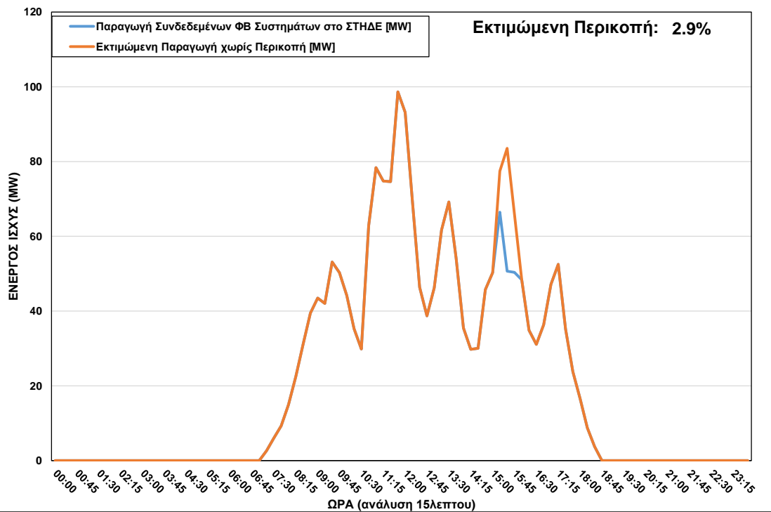
ΦΒ Παραγωγή στο ΣΤΗΔΕ κατά τη διάρκεια περικοπής στις 09/04/2023 ώρα 15:15 – 15:45
