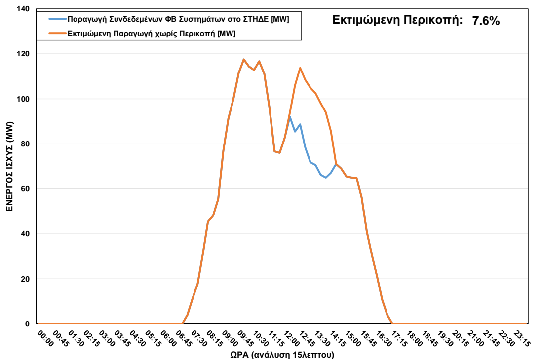
ΦΒ Παραγωγή στο ΣΤΗΔΕ κατά τη διάρκεια περικοπής στις 31/01/2023 ώρα 12:15 – 14:15
