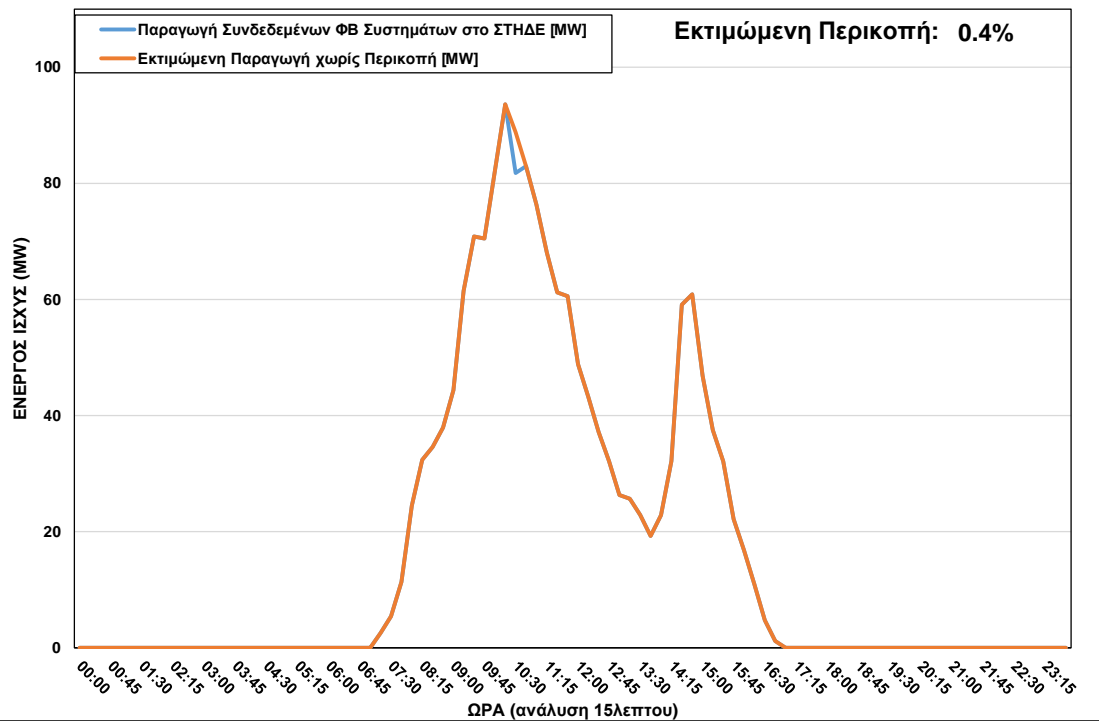
ΦΒ Παραγωγή στο ΣΤΗΔΕ κατά τη διάρκεια περικοπής στις 05/02/2023 ώρα 10:15 – 10:30
