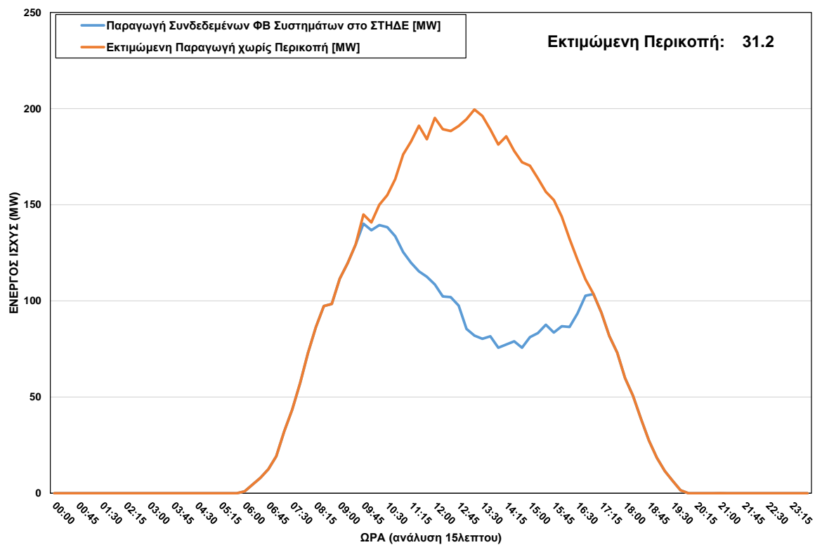
ΦΒ Παραγωγή στο ΣΤΗΔΕ κατά τη διάρκεια περικοπής στις 04/06/2023 ώρα 09:45 - 17:00
