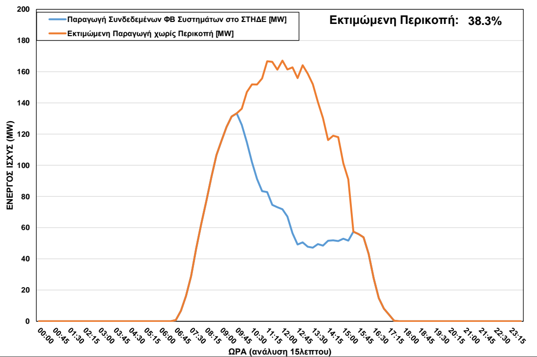
ΦΒ Παραγωγή στο ΣΤΗΔΕ κατά τη διάρκεια περικοπής στις 20/02/2023 ώρα 09:45 – 15:15
