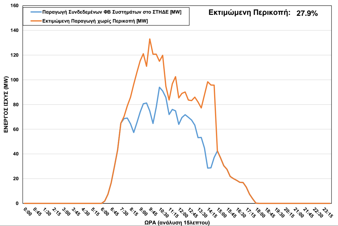
ΦΒ Παραγωγή στο ΣΤΗΔΕ κατά τη διάρκεια περικοπής στις 19-03-23 ώρα 7:45 - 15:00
