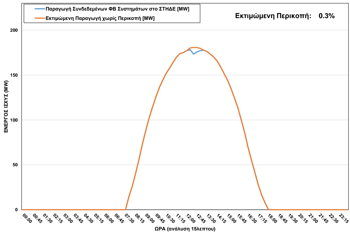
ΦΒ Παραγωγή στο ΣΤΗΔΕ κατά τη διάρκεια περικοπής στις 23/10/2023 ώρα 12:15 - 13:00
