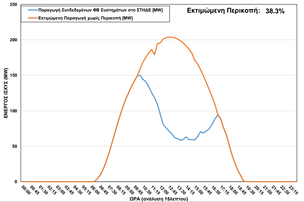
ΦΒ Παραγωγή στο ΣΤΗΔΕ κατά τη διάρκεια περικοπής στις 24/04/2023 ώρα 10:15 – 17:00
