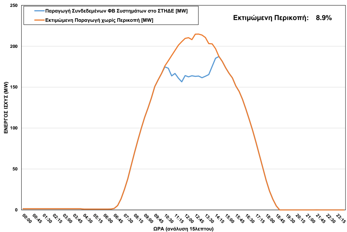
ΦΒ Παραγωγή στο ΣΤΗΔΕ κατά τη διάρκεια περικοπής στις 15/09/2023 ώρα 10:30 - 14:15
