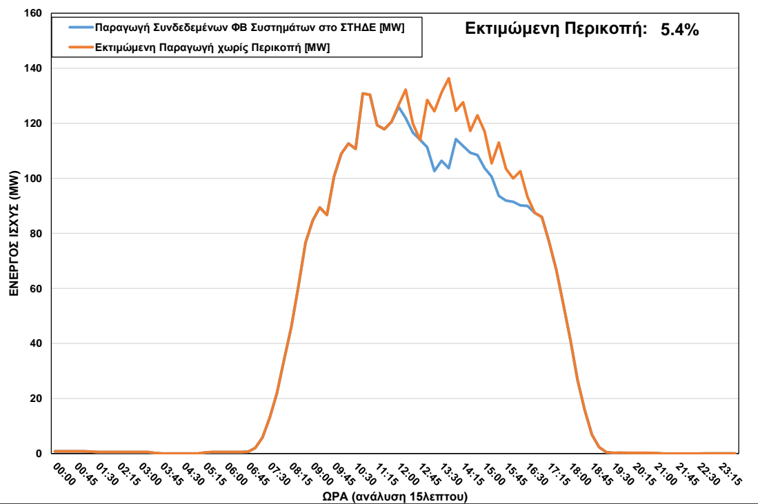
ΦΒ Παραγωγή στο ΣΤΗΔΕ κατά τη διάρκεια περικοπής στις 30/03/2023 ώρα 12:00 – 16:30
