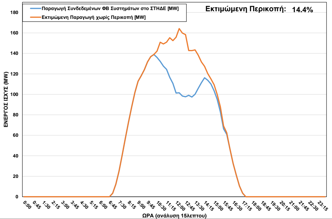
ΦΒ Παραγωγή στο ΣΤΗΔΕ κατά τη διάρκεια περικοπής στις 13-02-23 ώρα 10:15 – 16:00
