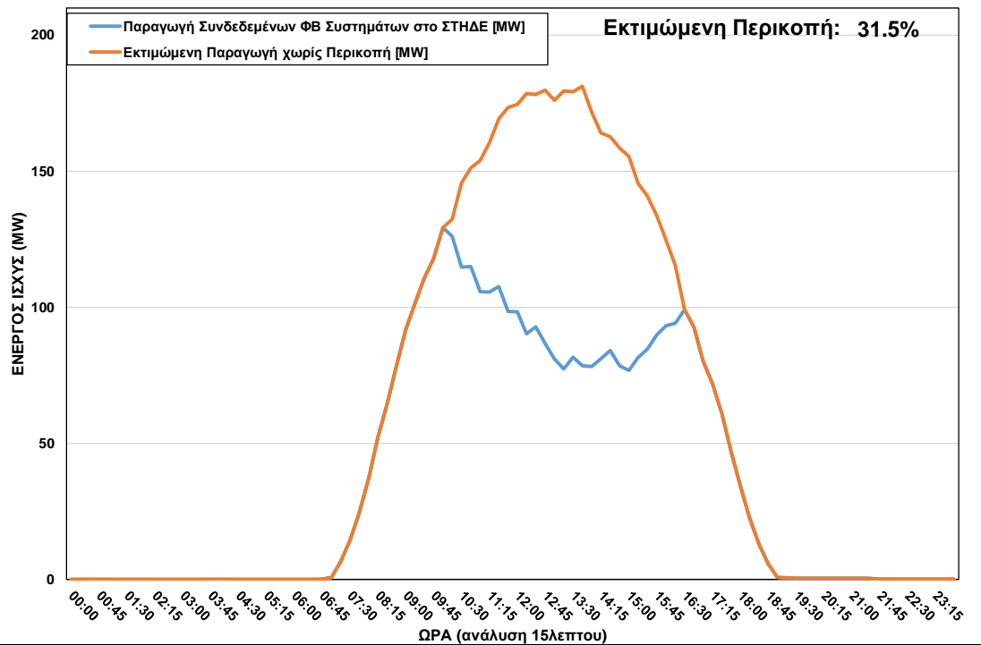
ΦΒ Παραγωγή στο ΣΤΗΔΕ κατά τη διάρκεια περικοπής στις 28/03/2023 ώρα 10:15 - 16:15
