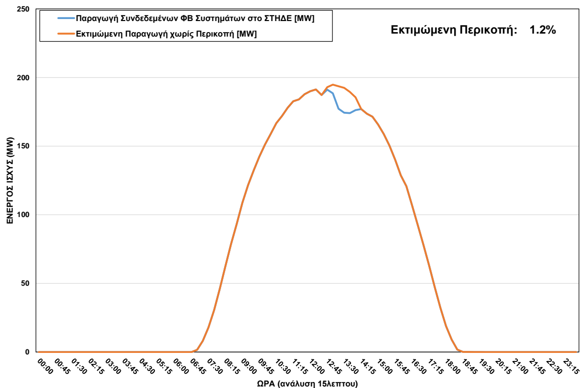
ΦΒ Παραγωγή στο ΣΤΗΔΕ κατά τη διάρκεια περικοπής στις 29/09/2023 ώρα 12:45 - 14:00
