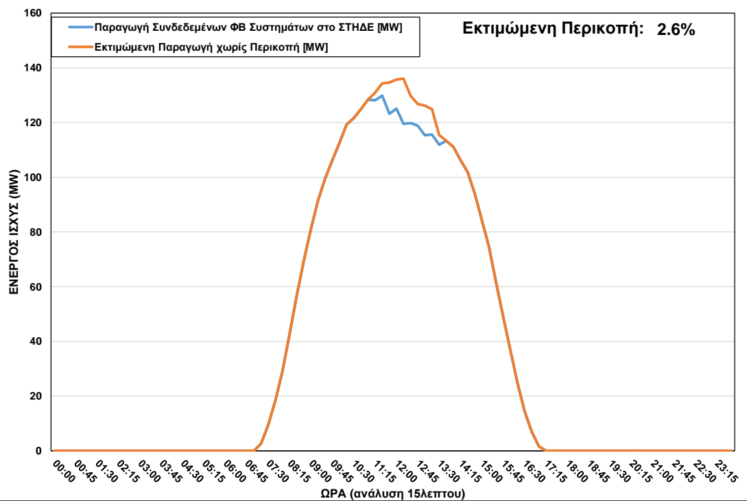
ΦΒ Παραγωγή στο ΣΤΗΔΕ κατά τη διάρκεια περικοπής στις 25/01/2023 ώρα 11:15 – 13:30
