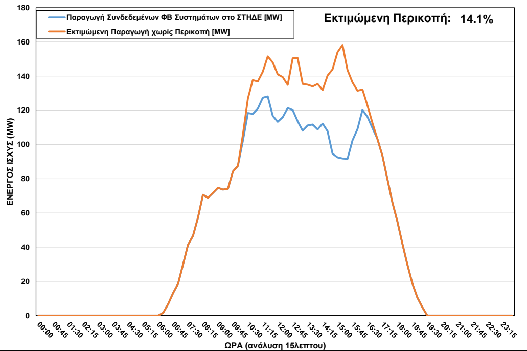
ΦΒ Παραγωγή στο ΣΤΗΔΕ κατά τη διάρκεια περικοπής στις 05/05/2023 ώρα 10:15 – 16:45
