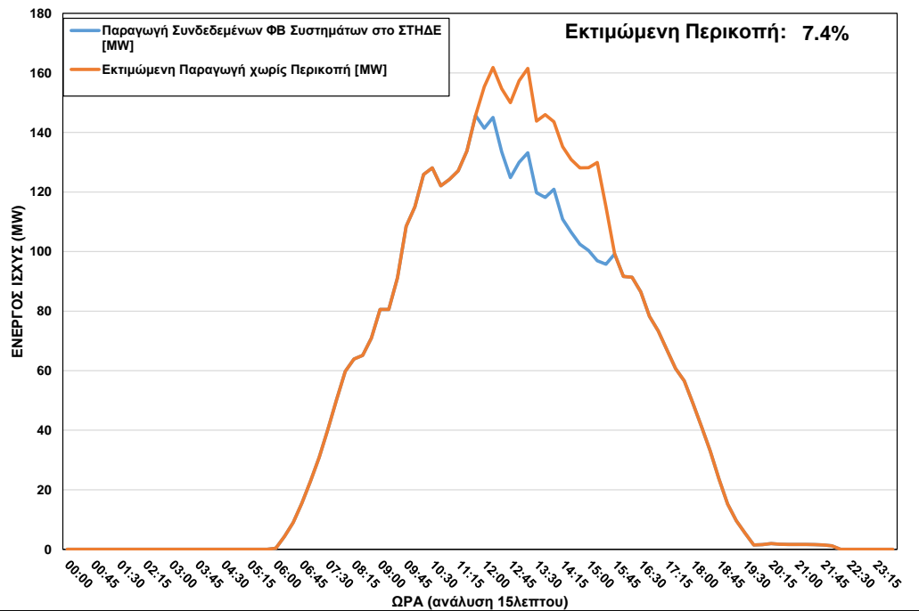
ΦΒ Παραγωγή στο ΣΤΗΔΕ κατά τη διάρκεια περικοπής στις 23/05/2023 ώρα 12:00 – 15:30
