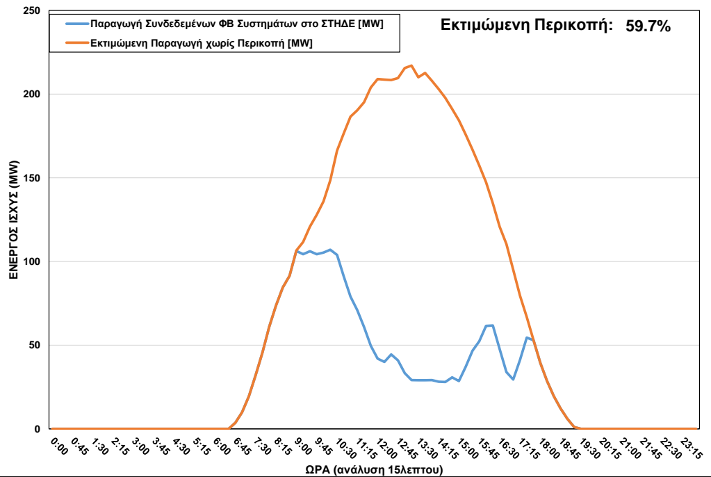
ΦΒ Παραγωγή στο ΣΤΗΔΕ κατά τη διάρκεια περικοπής στις 15-04-23 ώρα 9:00 – 17:30
