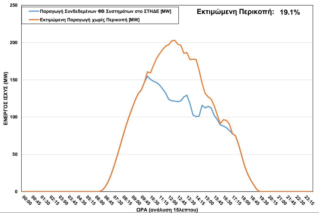
ΦΒ Παραγωγή στο ΣΤΗΔΕ κατά τη διάρκεια περικοπής στις 21/04/2023 ώρα 10:15 – 17:00
