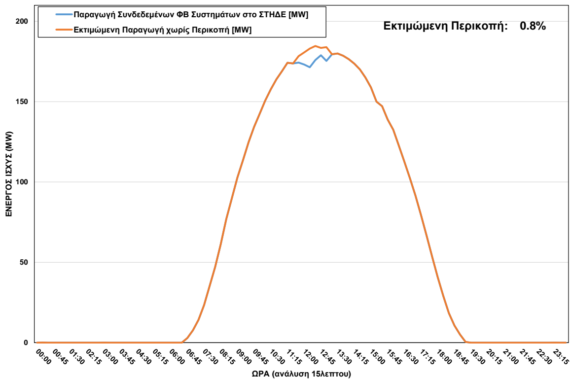
ΦΒ Παραγωγή στο ΣΤΗΔΕ κατά τη διάρκεια περικοπής στις 26/08/2023 ώρα 11:45 - 13:00
