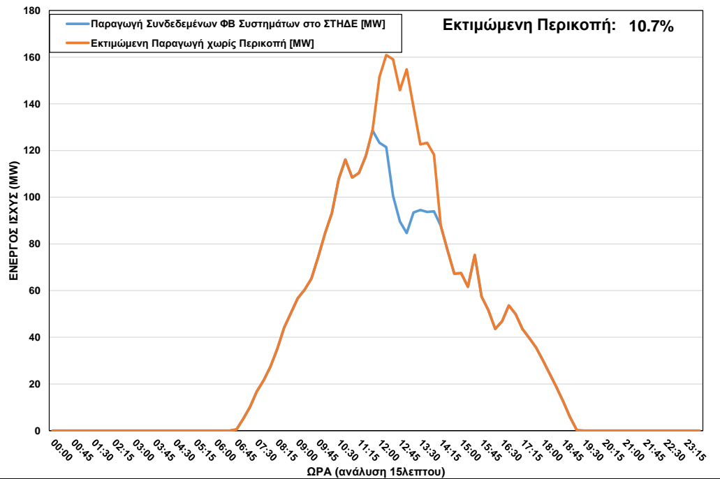
ΦΒ Παραγωγή στο ΣΤΗΔΕ κατά τη διάρκεια περικοπής στις 12/04/2023 ώρα 11:45 – 14:00
