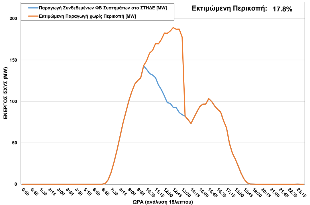
ΦΒ Παραγωγή στο ΣΤΗΔΕ κατά τη διάρκεια περικοπής στις 27-03-23 ώρα 10:15 – 13:30
