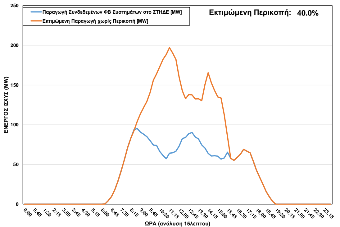
ΦΒ Παραγωγή στο ΣΤΗΔΕ κατά τη διάρκεια περικοπής στις 30-04-23 ώρα 8:30 – 15:45
