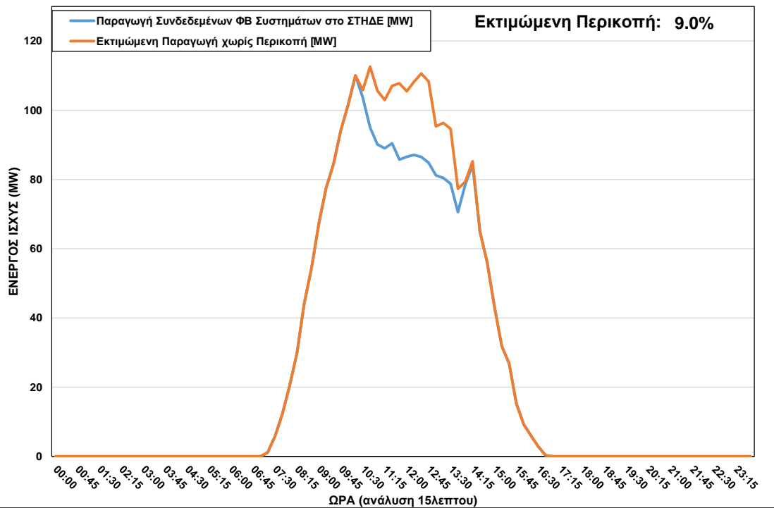
ΦΒ Παραγωγή στο ΣΤΗΔΕ κατά τη διάρκεια περικοπής στις 07/01/2023 ώρα 10:15 – 14:15
