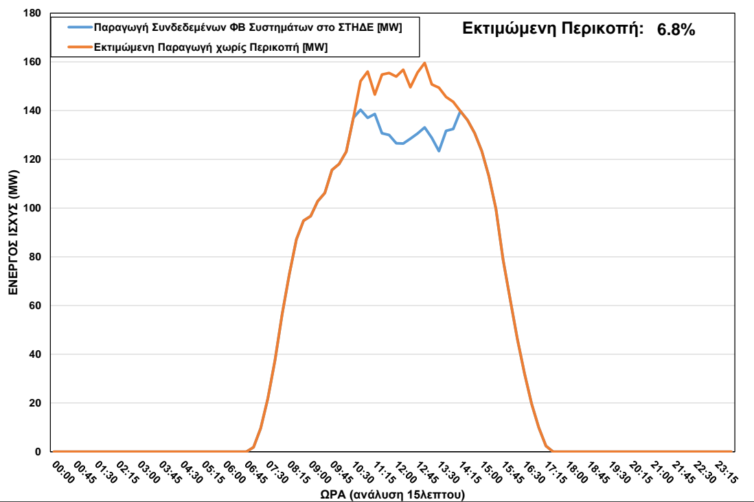
ΦΒ Παραγωγή στο ΣΤΗΔΕ κατά τη διάρκεια περικοπής στις 08/02/2023 ώρα 10:30 – 14:15
