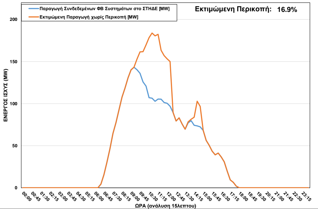
ΦΒ Παραγωγή στο ΣΤΗΔΕ κατά τη διάρκεια περικοπής στις 15/03/2023 ώρα 09:15 – 14:45
