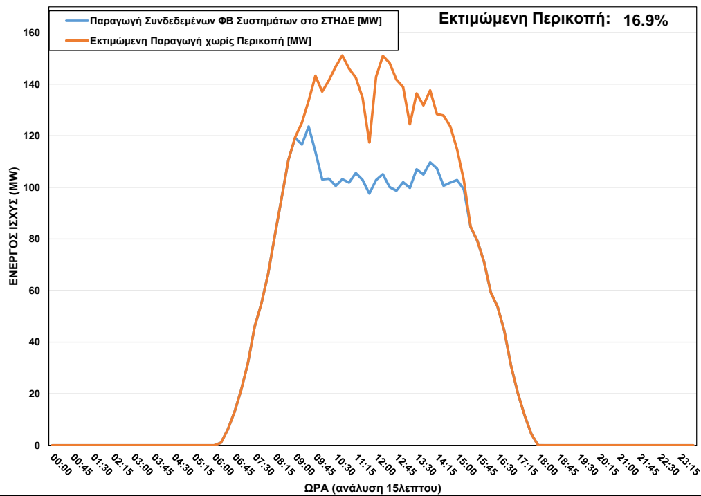
ΦΒ Παραγωγή στο ΣΤΗΔΕ κατά τη διάρκεια περικοπής στις 20/03/2023 ώρα 09:00 – 15:30
