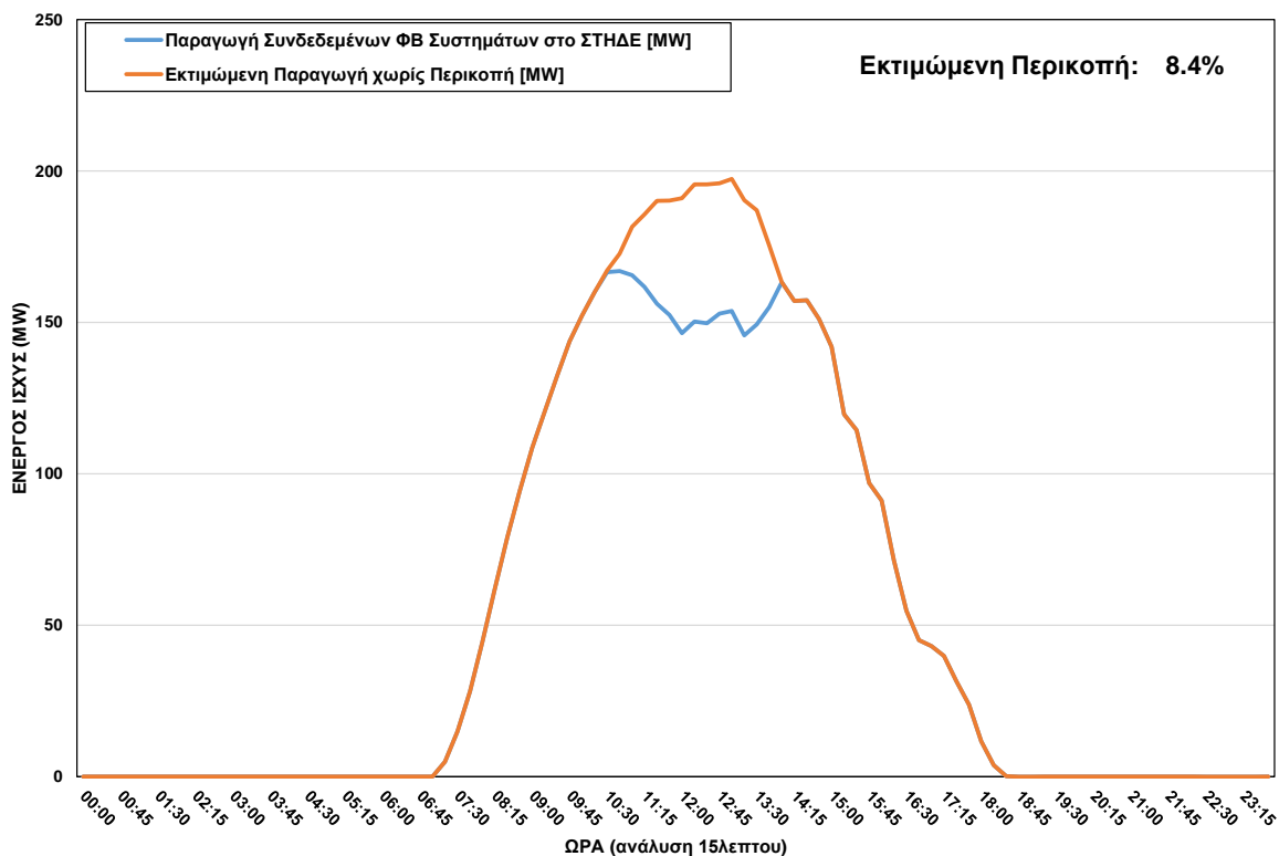
ΦΒ Παραγωγή στο ΣΤΗΔΕ κατά τη διάρκεια περικοπής στις 07/10/2023 ώρα 10:30 - 13:45
