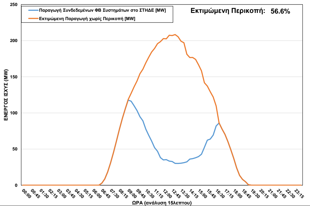
ΦΒ Παραγωγή στο ΣΤΗΔΕ κατά τη διάρκεια περικοπής στις 14/04/2023 ώρα 09:00 – 16:30
