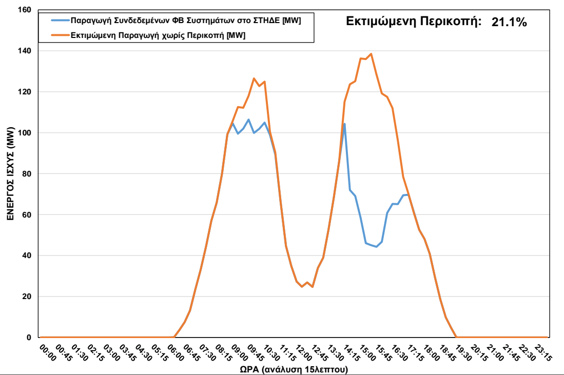
ΦΒ Παραγωγή στο ΣΤΗΔΕ κατά τη διάρκεια περικοπής στις 29/04/2023 ώρα 09:00 – 17:30
