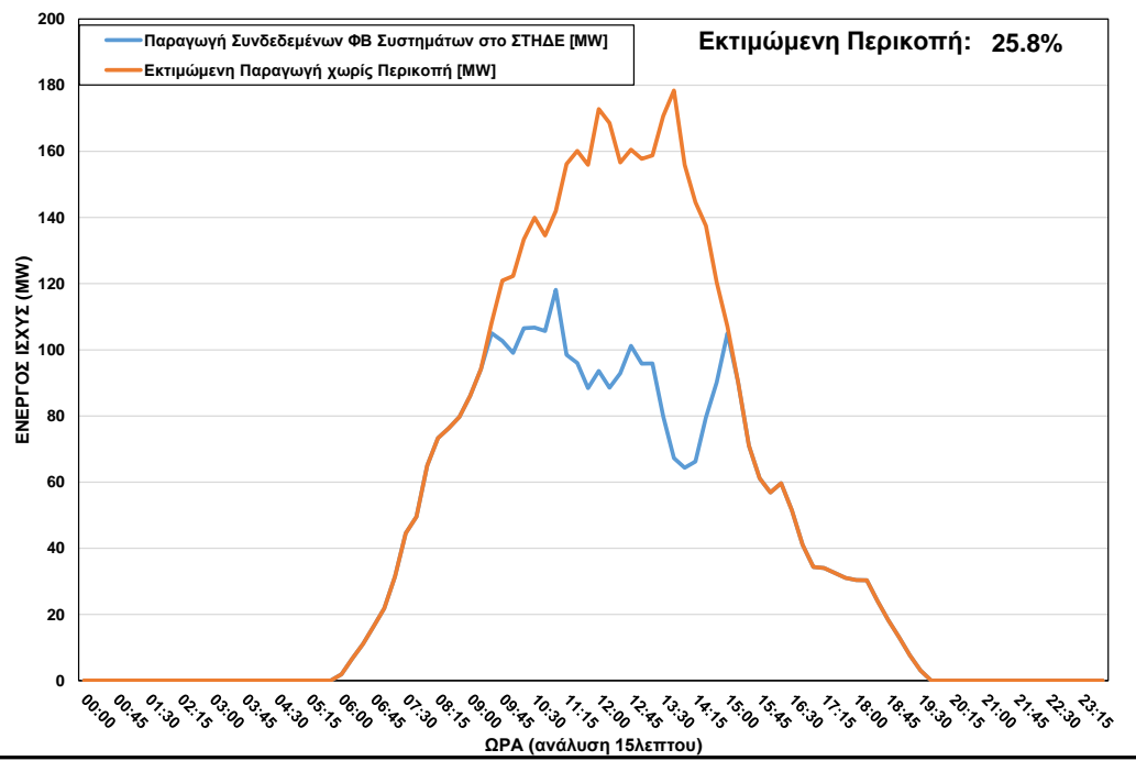
ΦΒ Παραγωγή στο ΣΤΗΔΕ κατά τη διάρκεια περικοπής στις 21/05/2023 ώρα 09:30 - 15:00
