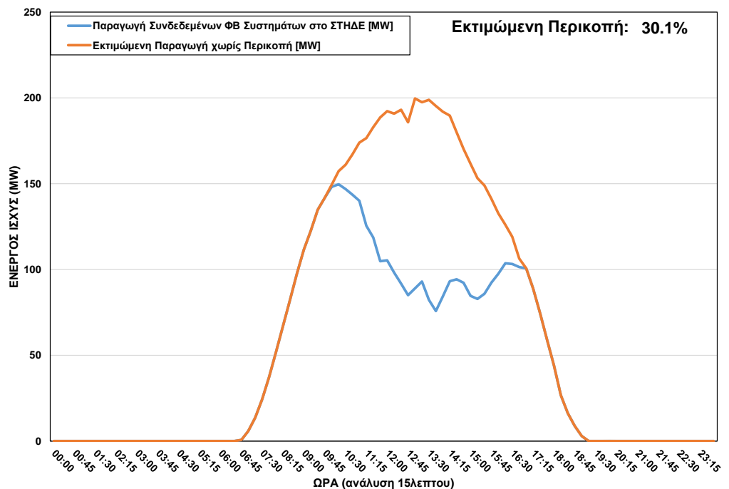
ΦΒ Παραγωγή στο ΣΤΗΔΕ κατά τη διάρκεια περικοπής στις 06/04/2023 ώρα 10:00 – 16:45
