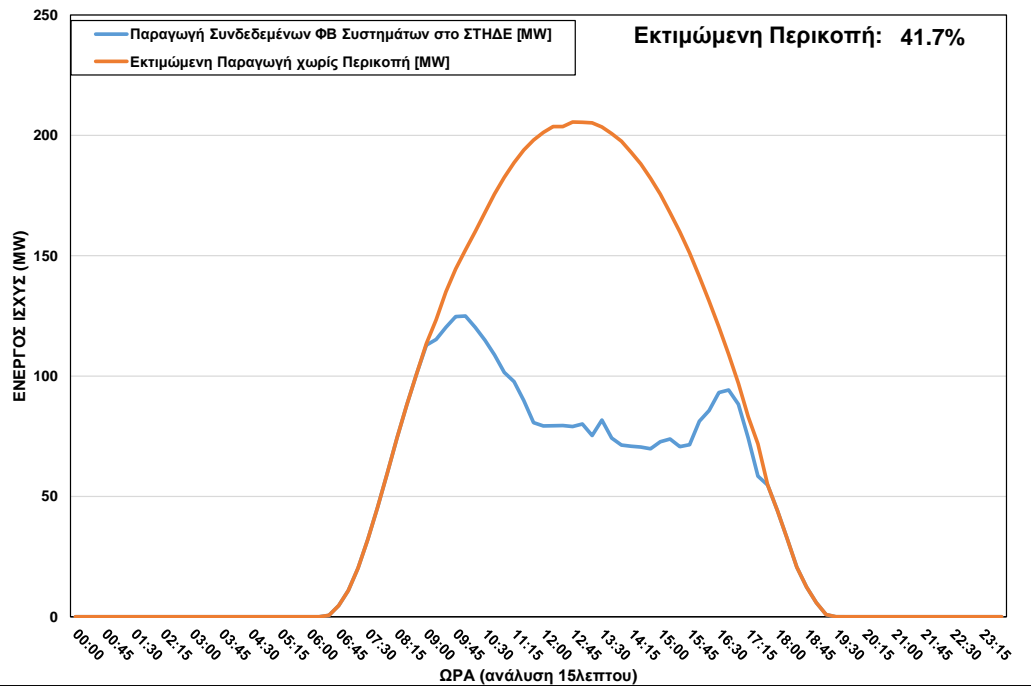
ΦΒ Παραγωγή στο ΣΤΗΔΕ κατά τη διάρκεια περικοπής στις 18/04/2023 ώρα 09:00 – 17:30
