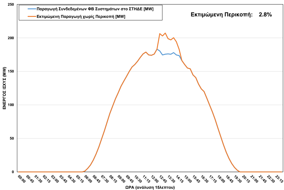
ΦΒ Παραγωγή στο ΣΤΗΔΕ κατά τη διάρκεια περικοπής στις 15/06/2023 ώρα 12:45 - 14:30
