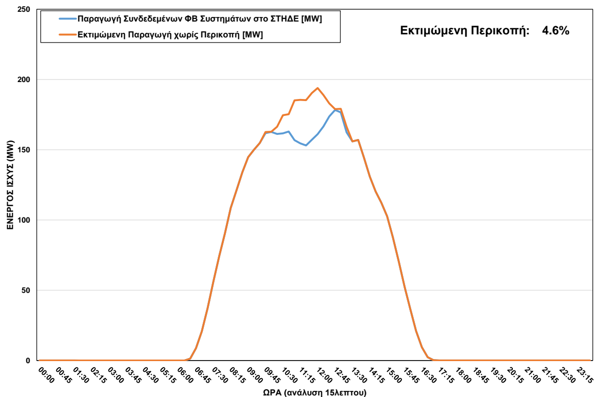
Φ/Β Παραγωγή στο ΣΤΗΔΕ κατά τη διάρκεια περικοπής στις 04/11/2023 ώρα 09:45 - 13:15
