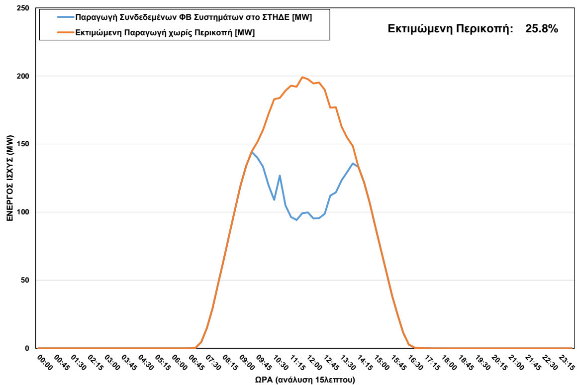
ΦΒ Παραγωγή στο ΣΤΗΔΕ κατά τη διάρκεια περικοπής στις 18/12/2023 ώρα 09:30 - 14:00
