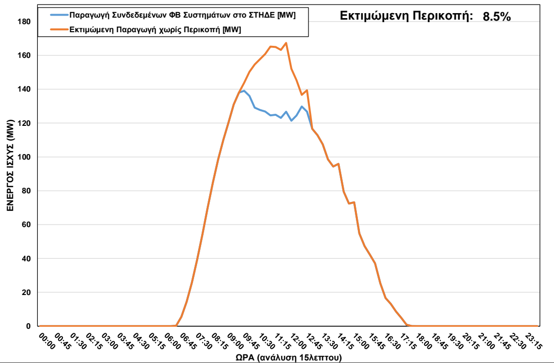
ΦΒ Παραγωγή στο ΣΤΗΔΕ κατά τη διάρκεια περικοπής στις 02/03/2023 ώρα 09:45 – 12:45
