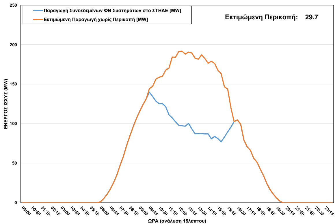
ΦΒ Παραγωγή στο ΣΤΗΔΕ κατά τη διάρκεια περικοπής στις 18/06/2023 ώρα 09:45 - 16:00
