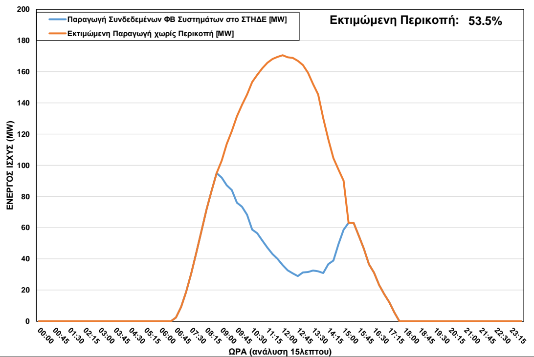
ΦΒ Παραγωγή στο ΣΤΗΔΕ κατά τη διάρκεια περικοπής στις 26/02/2023 ώρα 08:45 – 15:00
