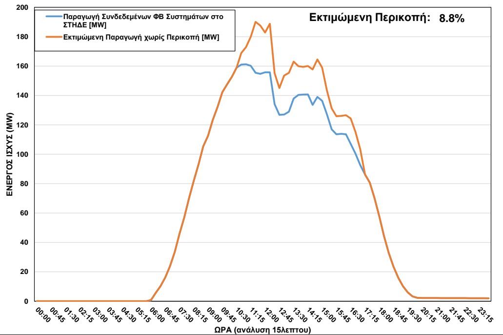
ΦΒ Παραγωγή στο ΣΤΗΔΕ κατά τη διάρκεια περικοπής στις 24/05/2023 ώρα 10:45 – 17:00
