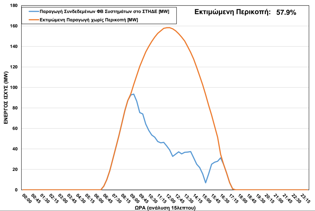
ΦΒ Παραγωγή στο ΣΤΗΔΕ κατά τη διάρκεια περικοπής στις 28/02/2023 ώρα 09:00 – 16:30
