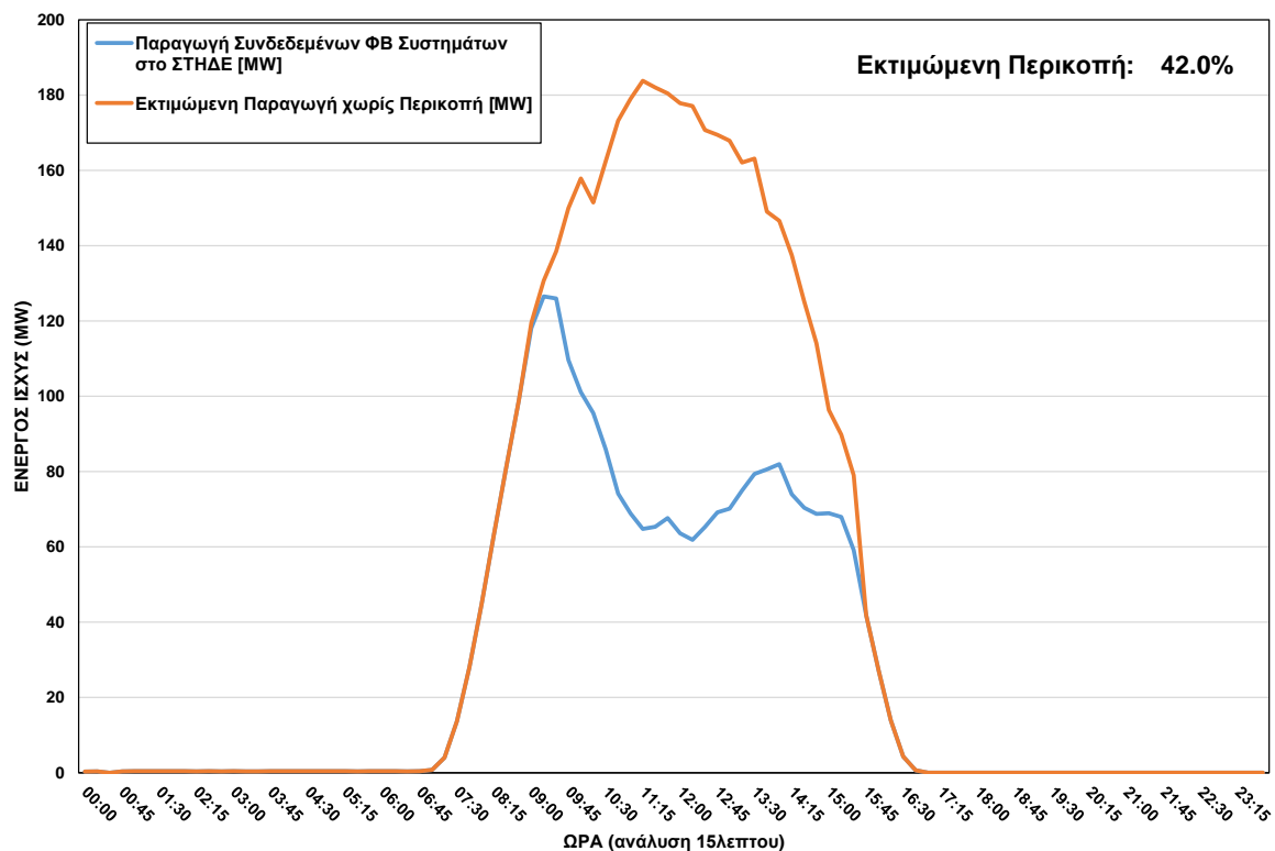
ΦΒ Παραγωγή στο ΣΤΗΔΕ κατά τη διάρκεια περικοπής στις 24/12/2023 ώρα 09:00 - 15:30
