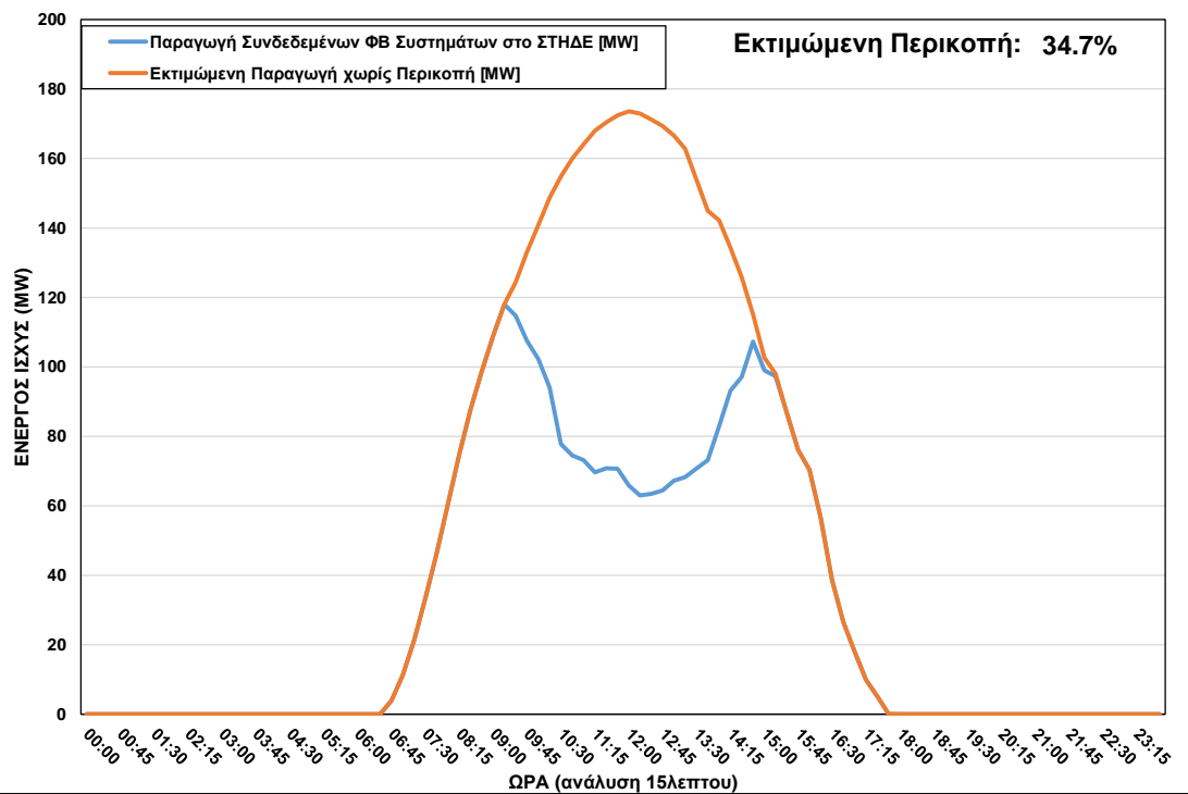
ΦΒ Παραγωγή στο ΣΤΗΔΕ κατά τη διάρκεια περικοπής στις 01/03/2023 ώρα 09:30 – 15:15
