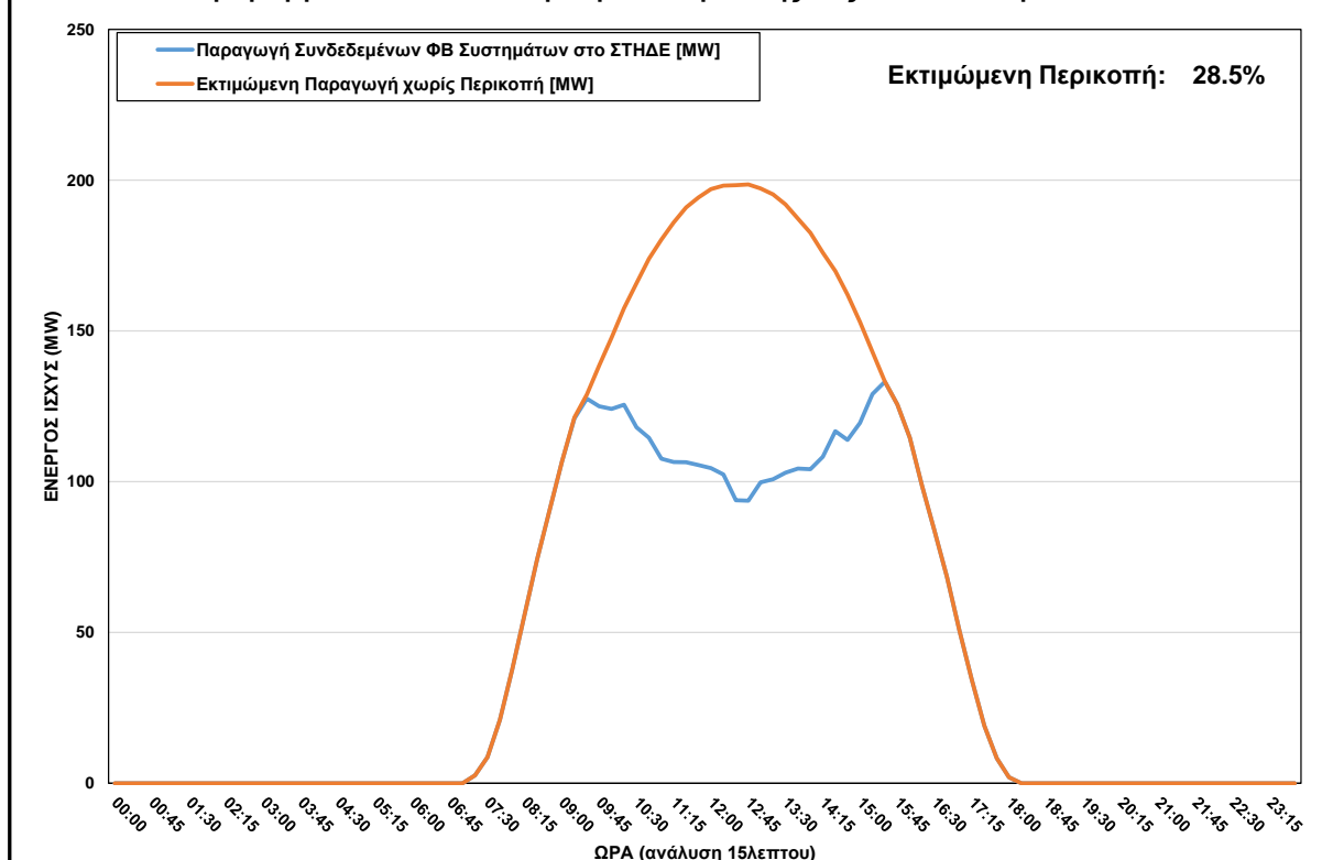
ΦΒ Παραγωγή στο ΣΤΗΔΕ κατά τη διάρκεια περικοπής στις 22/10/2023 ώρα 09:15 - 15:15
