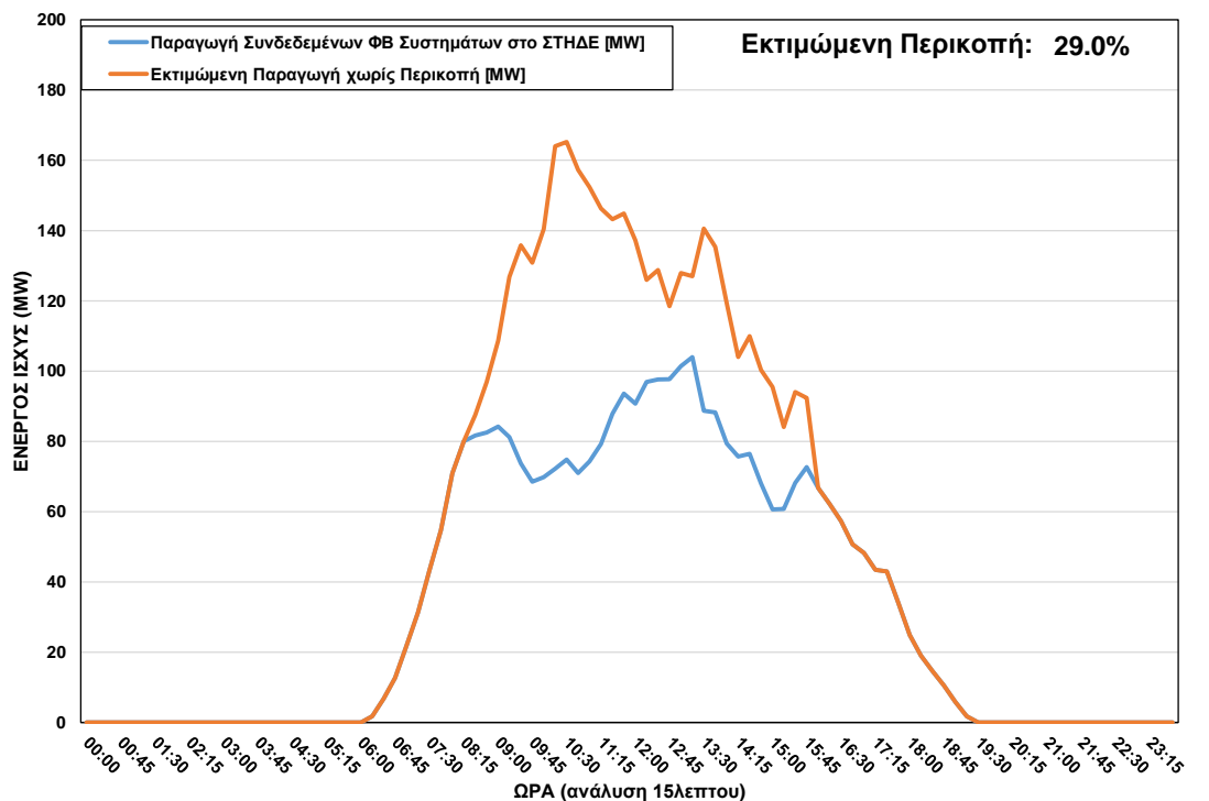
ΦΒ Παραγωγή στο ΣΤΗΔΕ κατά τη διάρκεια περικοπής στις 07/05/2023 ώρα 08:30 – 15:45
