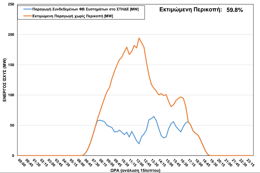
ΦΒ Παραγωγή στο ΣΤΗΔΕ κατά τη διάρκεια περικοπής στις 16/04/2023 ώρα 08:00 – 17:00
