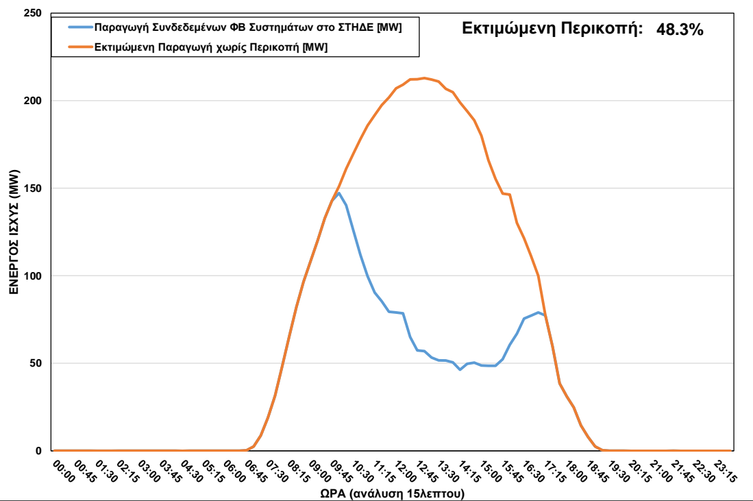
ΦΒ Παραγωγή στο ΣΤΗΔΕ κατά τη διάρκεια περικοπής στις 31/03/2023 ώρα 10:00 – 17:00
