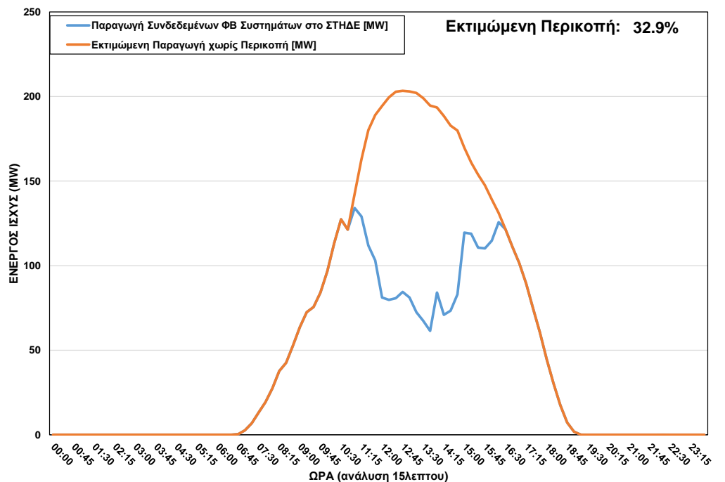
ΦΒ Παραγωγή στο ΣΤΗΔΕ κατά τη διάρκεια περικοπής στις 03/04/2023 ώρα 11:00 – 16:15
