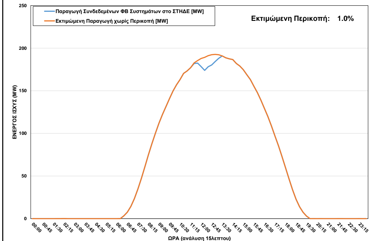
ΦΒ Παραγωγή στο ΣΤΗΔΕ κατά τη διάρκεια περικοπής στις 05/08/2023 ώρα 11:30 - 13:15
