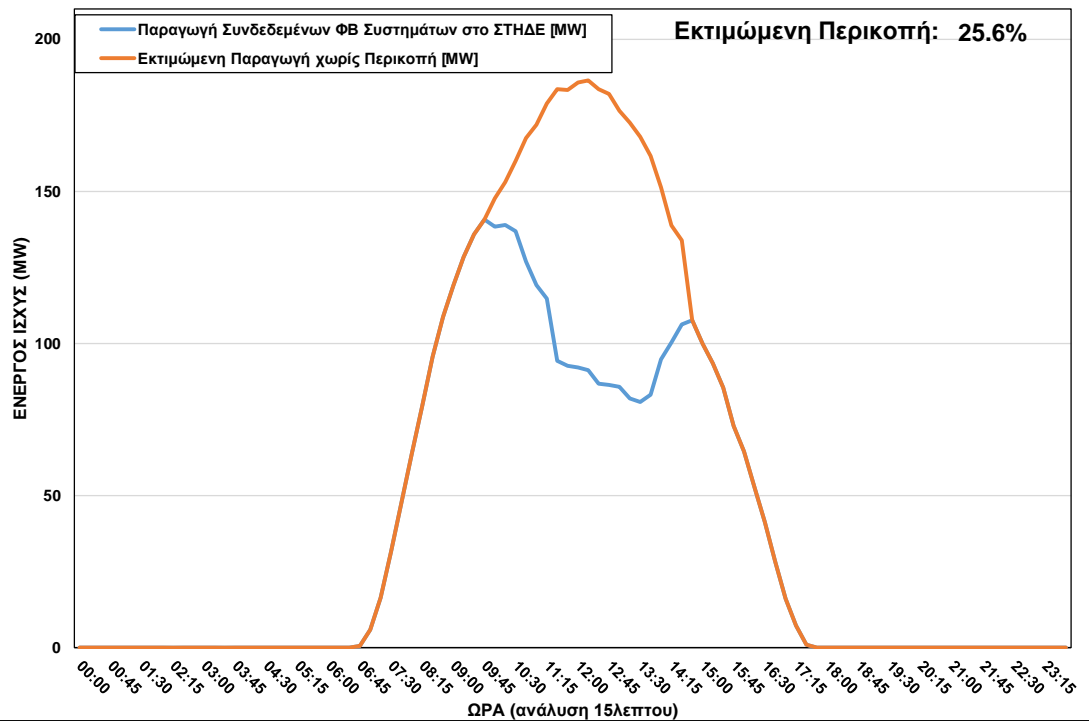
ΦΒ Παραγωγή στο ΣΤΗΔΕ κατά τη διάρκεια περικοπής στις 17/02/2023 ώρα 09:45 – 14:30
