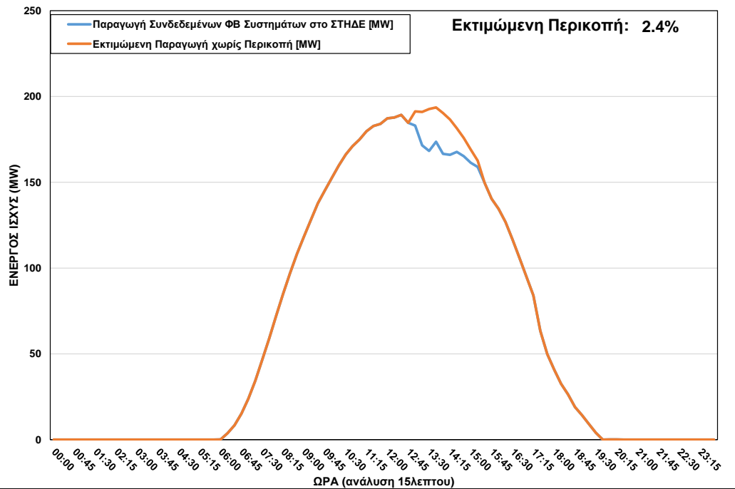
ΦΒ Παραγωγή στο ΣΤΗΔΕ κατά τη διάρκεια περικοπής στις 16/05/2023 ώρα 13:00 – 15:15
