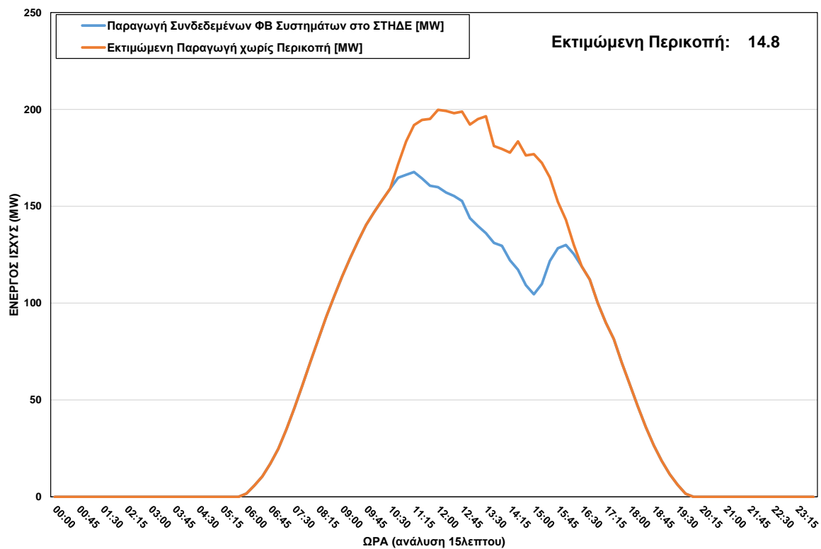
ΦΒ Παραγωγή στο ΣΤΗΔΕ κατά τη διάρκεια περικοπής στις 10/06/2023 ώρα 10:45 - 16:15
