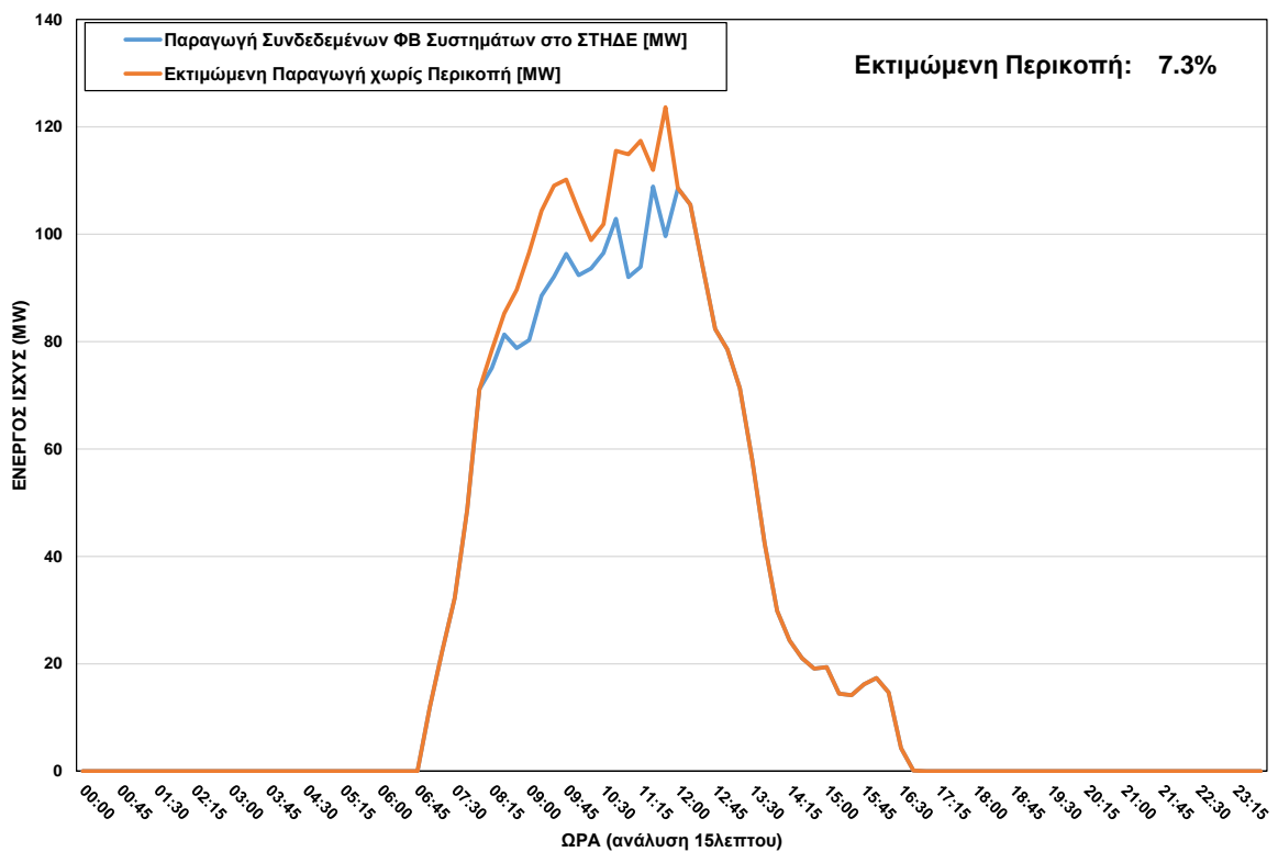
ΦΒ Παραγωγή στο ΣΤΗΔΕ κατά τη διάρκεια περικοπής στις 19/11/2023 ώρα 08:15 - 12:00
