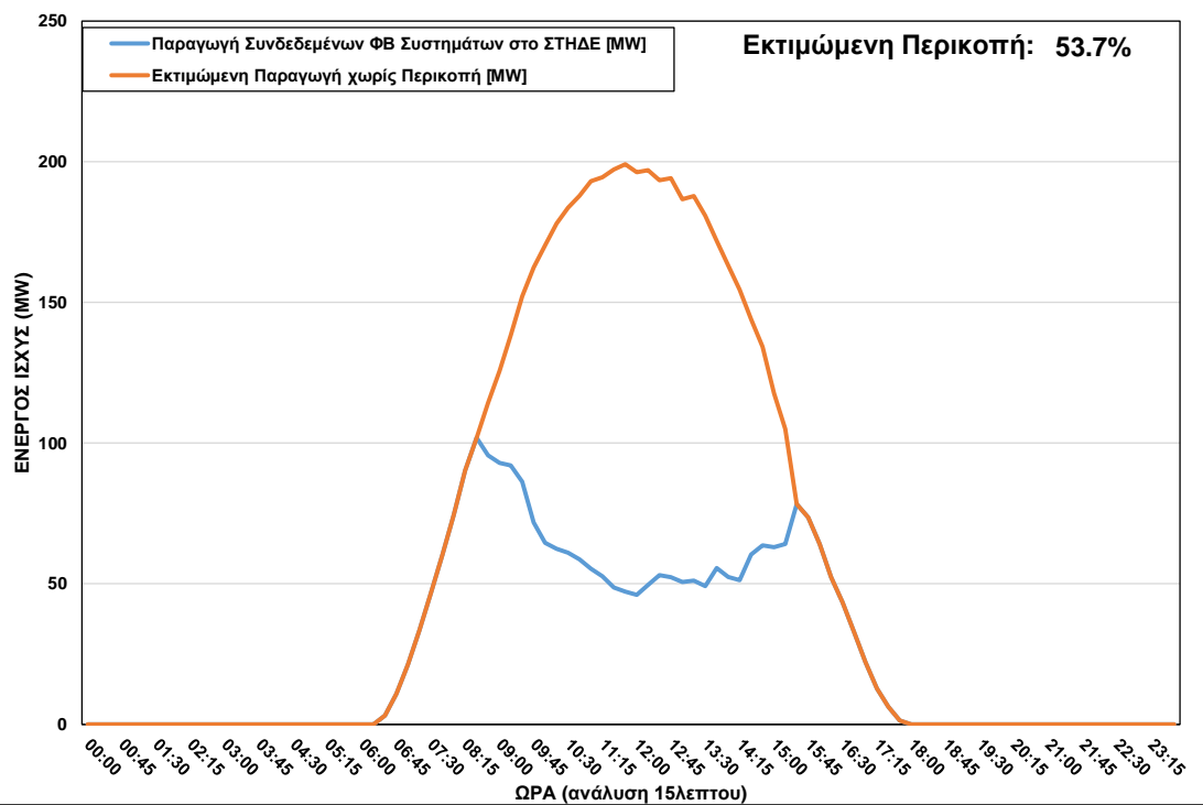
ΦΒ Παραγωγή στο ΣΤΗΔΕ κατά τη διάρκεια περικοπής στις 11/03/2023 ώρα 08:30 – 15:15
