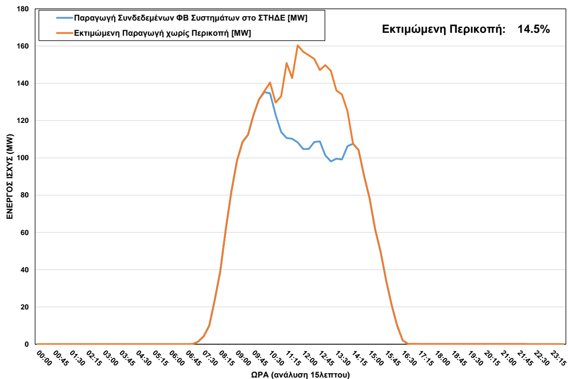
ΦΒ Παραγωγή στο ΣΤΗΔΕ κατά τη διάρκεια περικοπής στις 16/12/2023 ώρα 10:00 - 14:00
