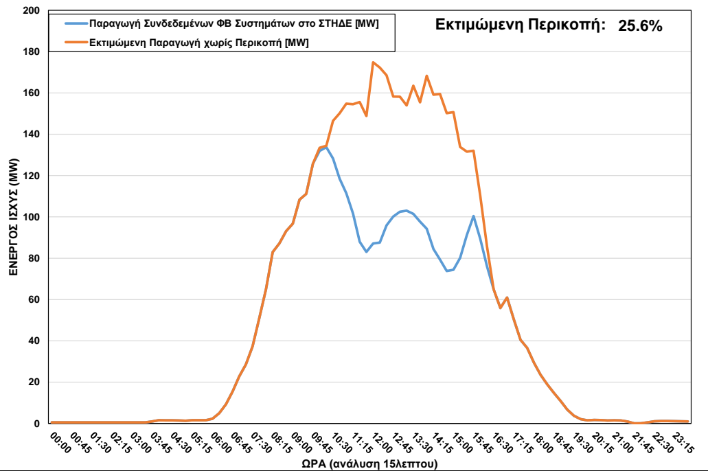
ΦΒ Παραγωγή στο ΣΤΗΔΕ κατά τη διάρκεια περικοπής στις 20/05/2023 ώρα 10:00 – 16:15
