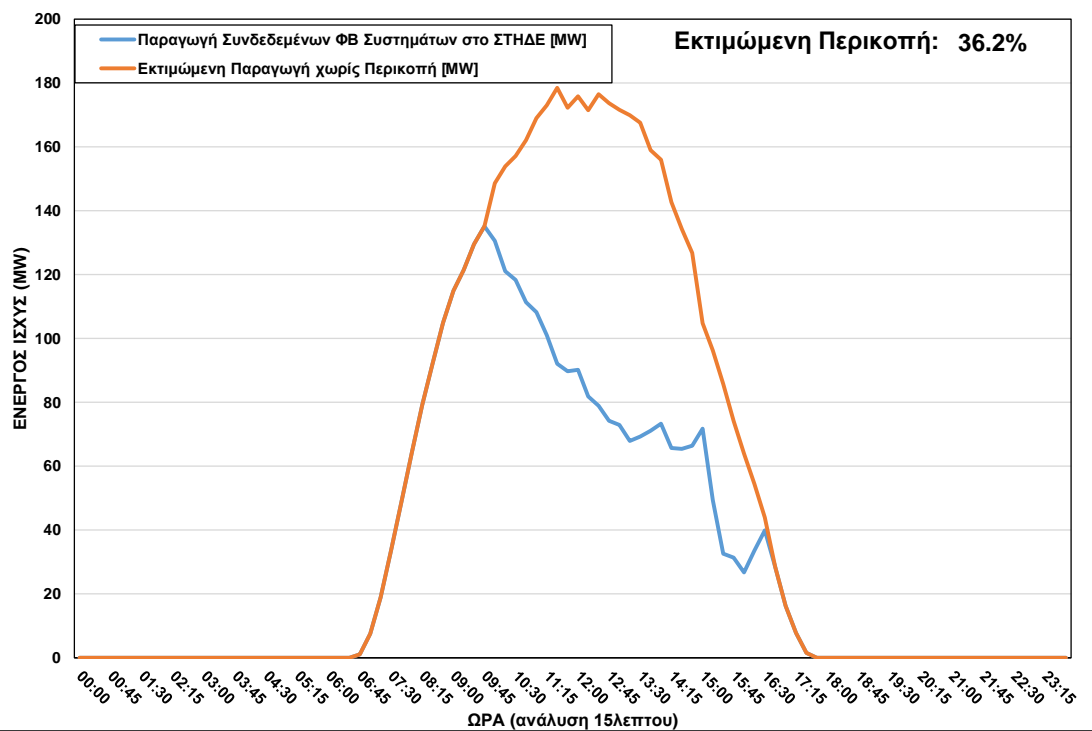
ΦΒ Παραγωγή στο ΣΤΗΔΕ κατά τη διάρκεια περικοπής στις 21/02/2023 ώρα 09:45 – 16:30
