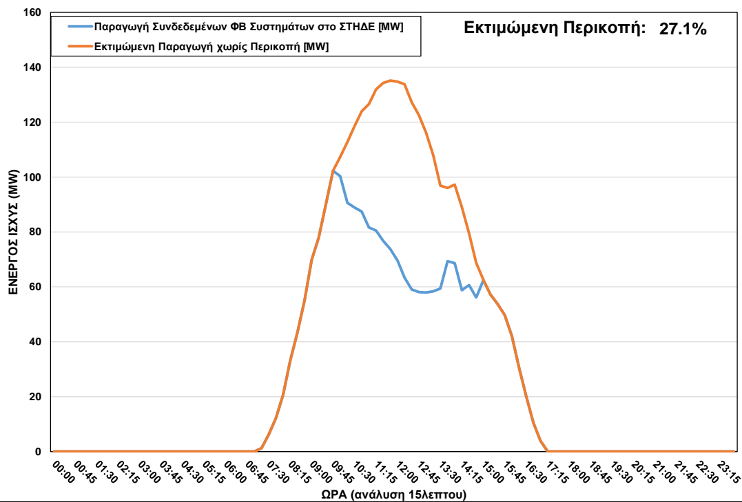
ΦΒ Παραγωγή στο ΣΤΗΔΕ κατά τη διάρκεια περικοπής στις 28/01/2023 ώρα 09:45 – 15:00
