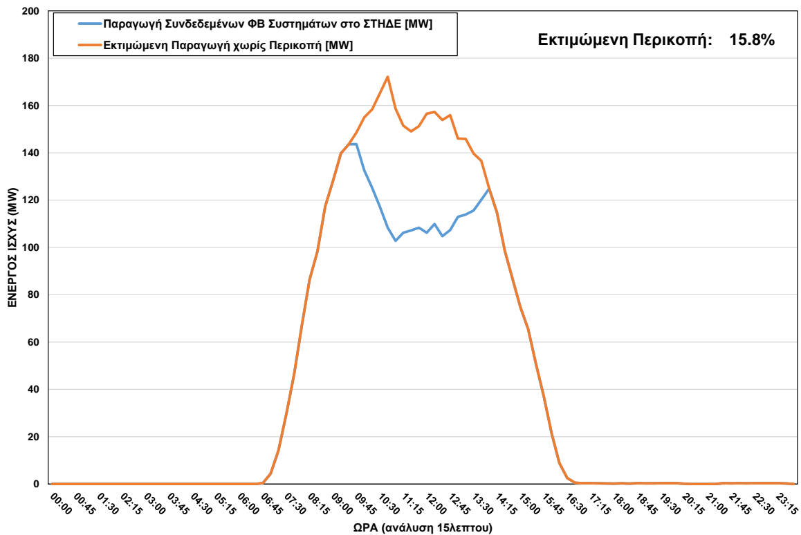
ΦΒ Παραγωγή στο ΣΤΗΔΕ κατά τη διάρκεια περικοπής στις 29/11/2023 ώρα 09:45 - 13:45
