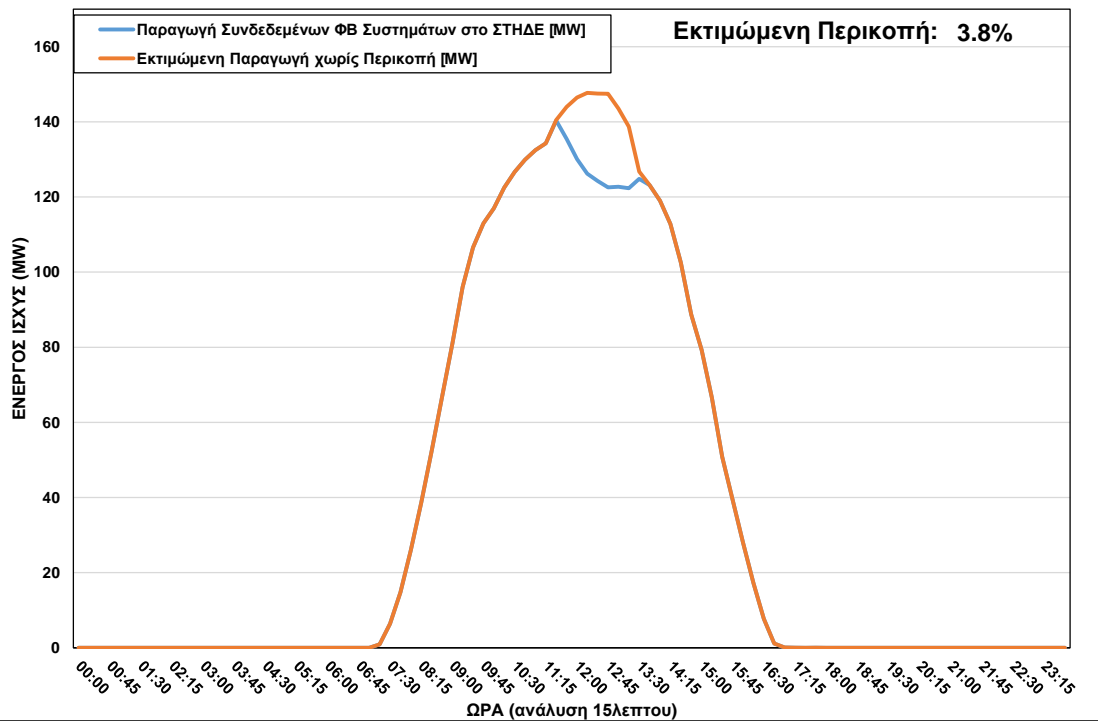
ΦΒ Παραγωγή στο ΣΤΗΔΕ κατά τη διάρκεια περικοπής στις 04/01/2023 ώρα 11:30 – 13:30
