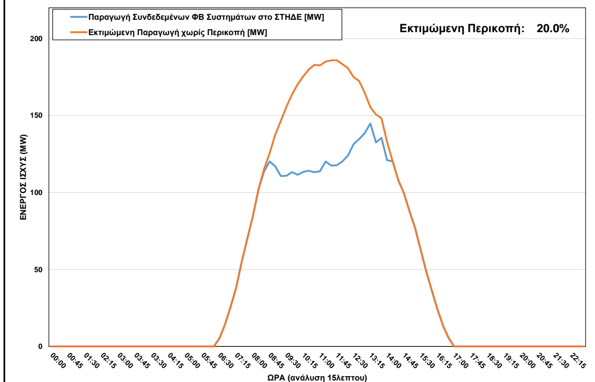
ΦΒ Παραγωγή στο ΣΤΗΔΕ κατά τη διάρκεια περικοπής στις 29/10/2023 ώρα 08:30 - 14:00
