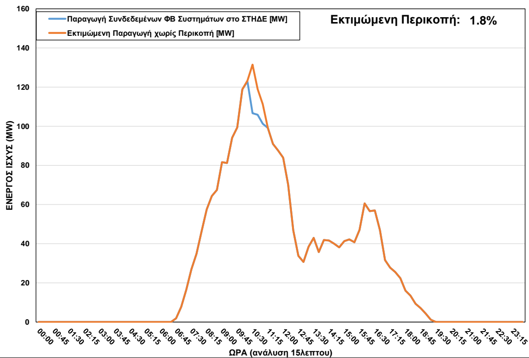
ΦΒ Παραγωγή στο ΣΤΗΔΕ κατά τη διάρκεια περικοπής στις 19/04/2023 ώρα 10:15 – 11:00
