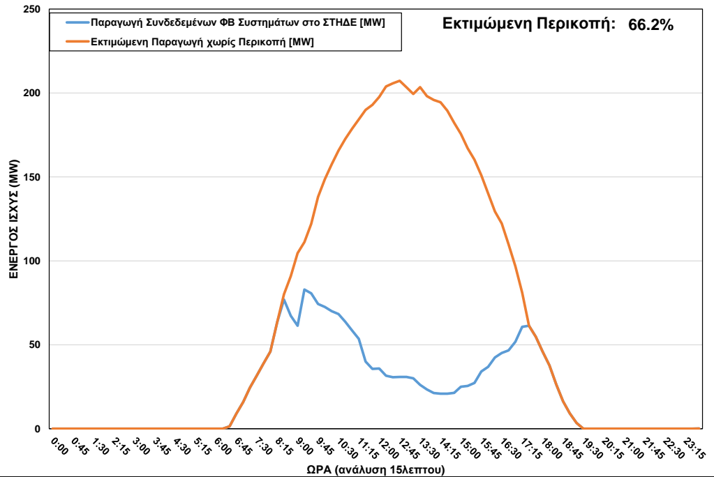
ΦΒ Παραγωγή στο ΣΤΗΔΕ κατά τη διάρκεια περικοπής στις 23-04-23 ώρα 8:30 - 17:15
