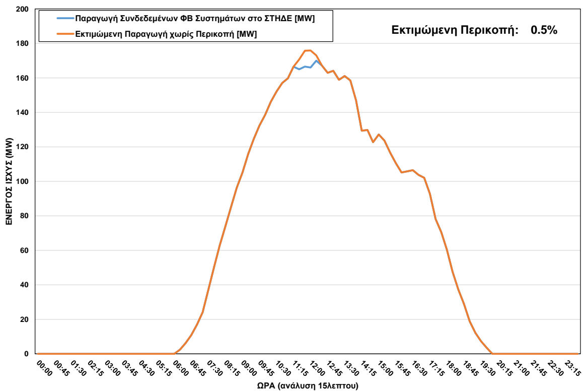
ΦΒ Παραγωγή στο ΣΤΗΔΕ κατά τη διάρκεια περικοπής στις 09/07/2023 ώρα 11:30 - 12:15
