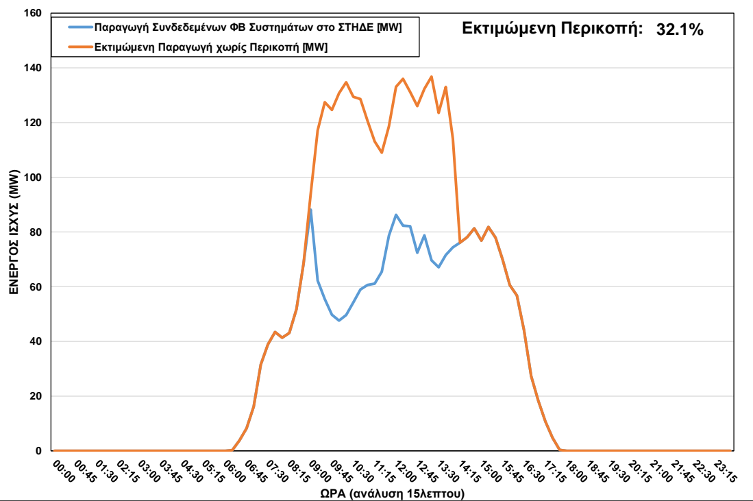
ΦΒ Παραγωγή στο ΣΤΗΔΕ κατά τη διάρκεια περικοπής στις 12/03/2023 ώρα 09:00 – 14:00
