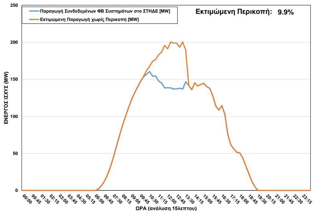
ΦΒ Παραγωγή στο ΣΤΗΔΕ κατά τη διάρκεια περικοπής στις 09/05/2023 ώρα 10:00 – 13:30
