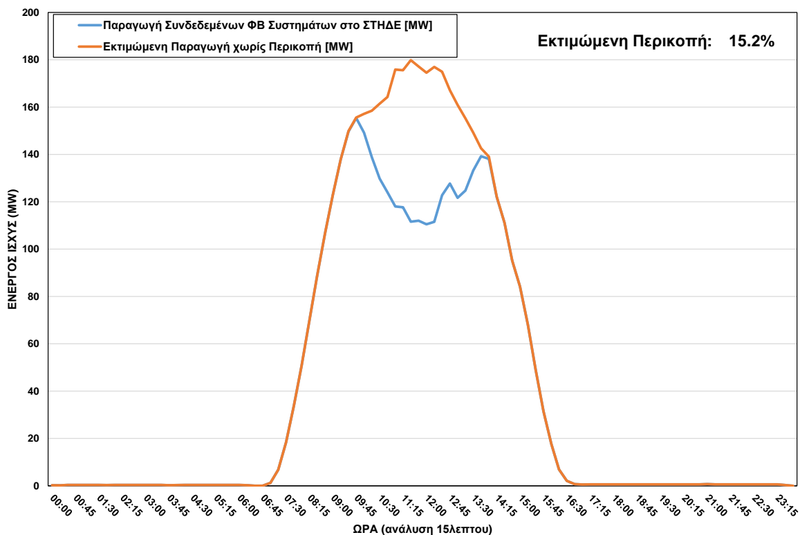
ΦΒ Παραγωγή στο ΣΤΗΔΕ κατά τη διάρκεια περικοπής στις 14/12/2023 ώρα 09:30 - 14:15
