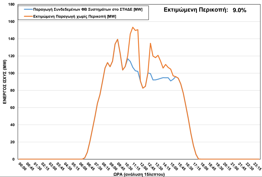
ΦΒ Παραγωγή στο ΣΤΗΔΕ κατά τη διάρκεια περικοπής στις 06/03/2023 ώρα 10:45 – 15:15
