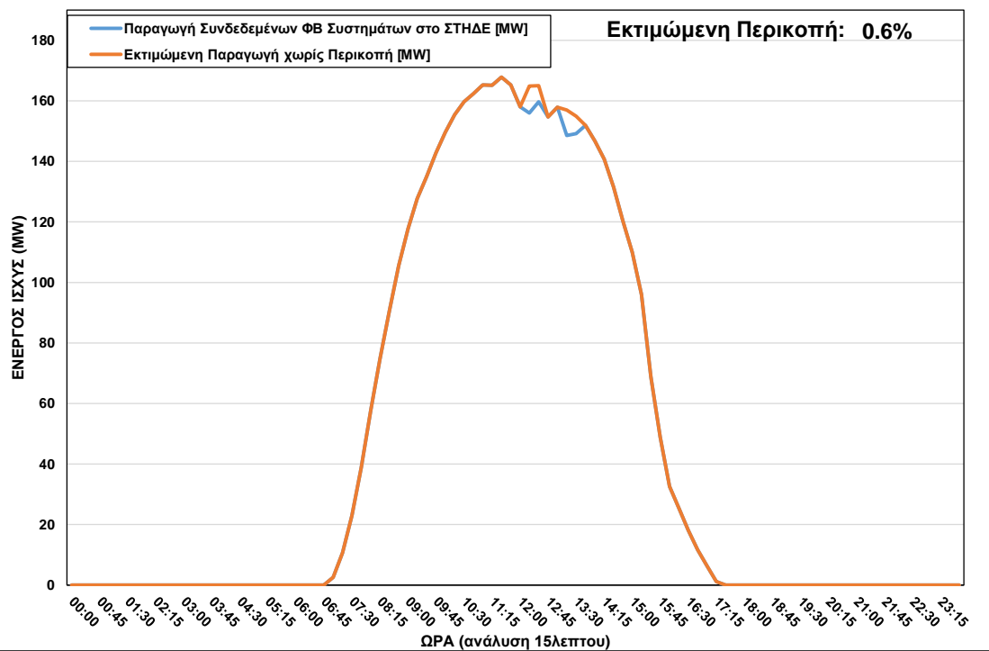
ΦΒ Παραγωγή στο ΣΤΗΔΕ κατά τη διάρκεια περικοπής στις 09/02/2023 ώρα 12:00 – 13:30
