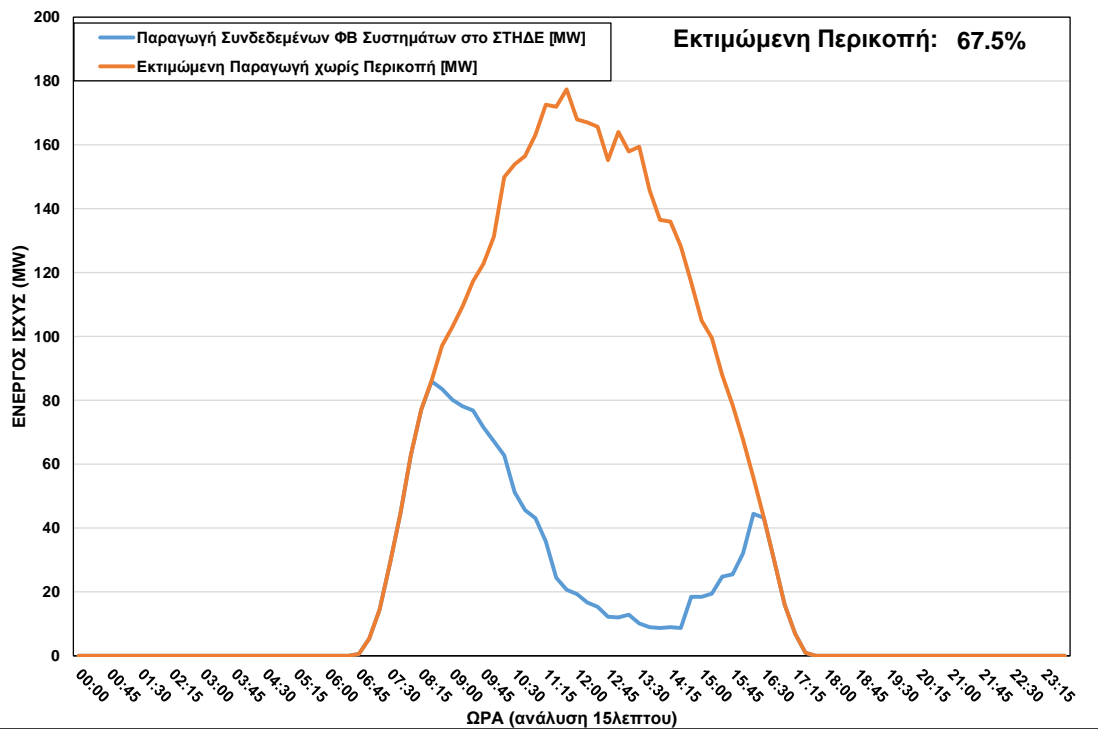
ΦΒ Παραγωγή στο ΣΤΗΔΕ κατά τη διάρκεια περικοπής στις 19/02/2023 ώρα 08:00 – 16:30
