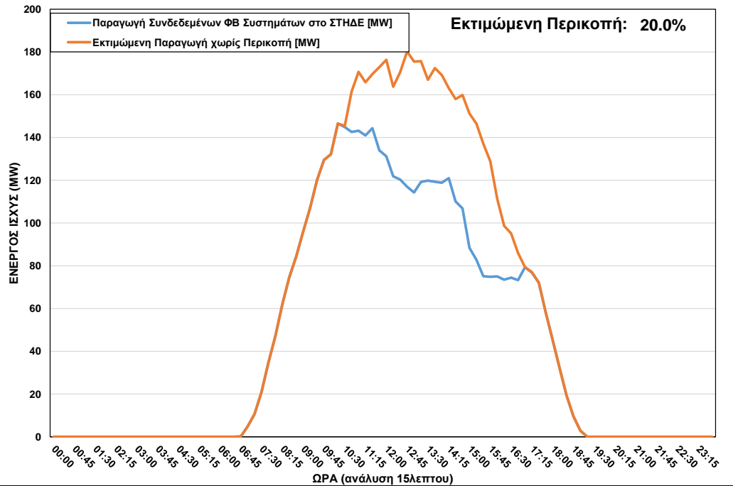
ΦΒ Παραγωγή στο ΣΤΗΔΕ κατά τη διάρκεια περικοπής στις 07/04/2023 ώρα 10:30 – 17:15
