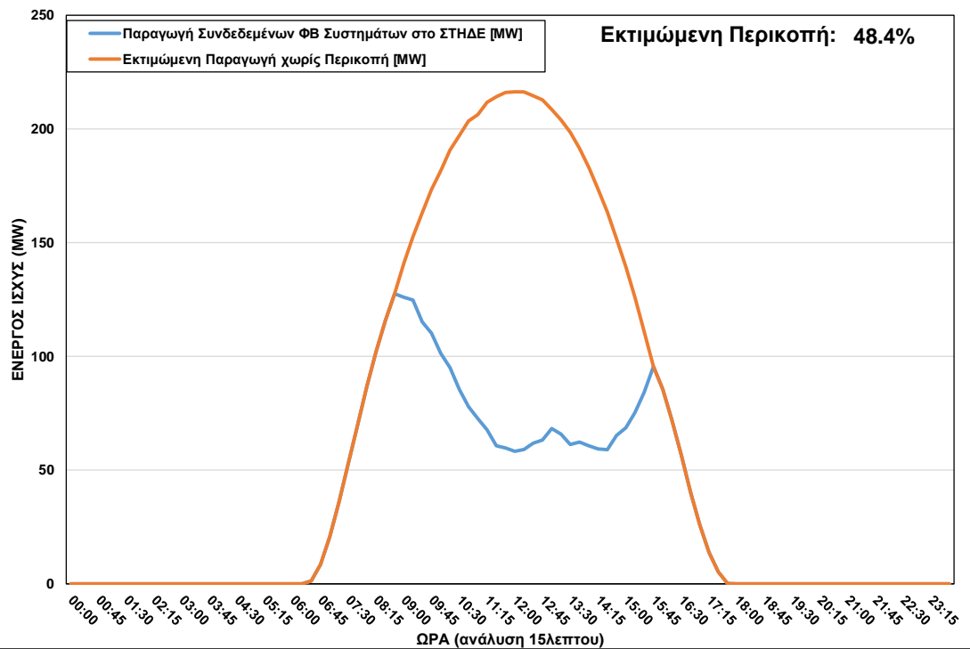
ΦΒ Παραγωγή στο ΣΤΗΔΕ κατά τη διάρκεια περικοπής στις 04/03/2023 ώρα 08:45 – 15:30
