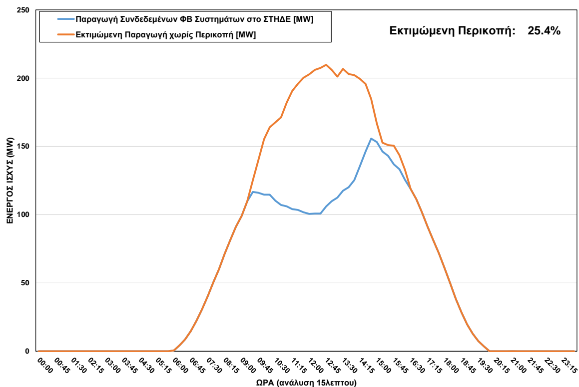
ΦΒ Παραγωγή στο ΣΤΗΔΕ κατά τη διάρκεια περικοπής στις 02/07/2023 ώρα 09:30 - 16:15
