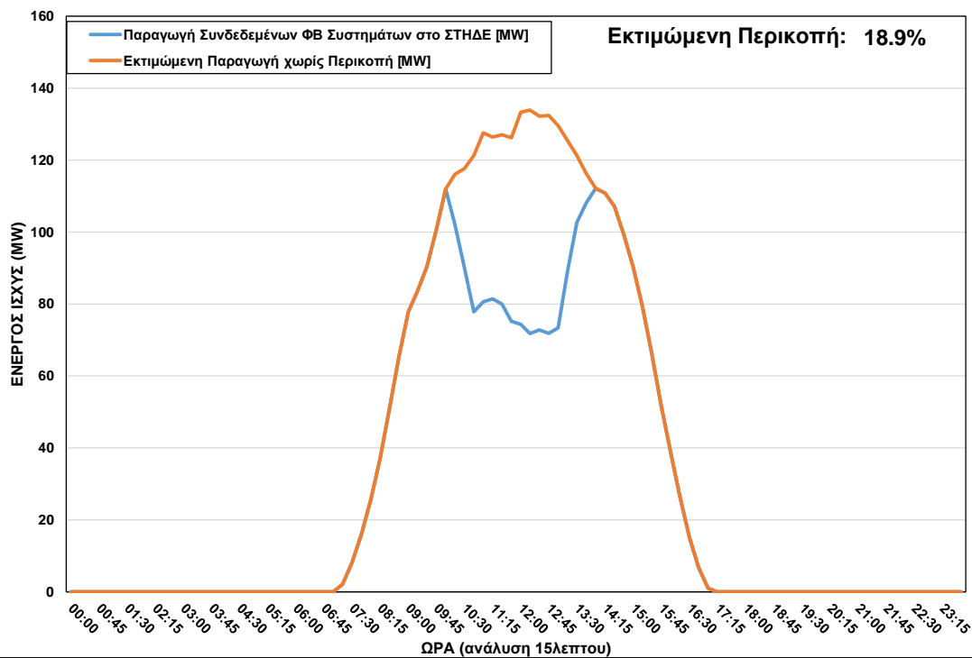
ΦΒ Παραγωγή στο ΣΤΗΔΕ κατά τη διάρκεια περικοπής στις 20/01/2023 ώρα 10:00 – 13:45
