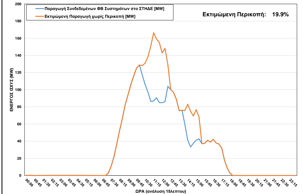
ΦΒ Παραγωγή στο ΣΤΗΔΕ κατά τη διάρκεια περικοπής στις 15/10/2023 ώρα 10:15 - 15:15
