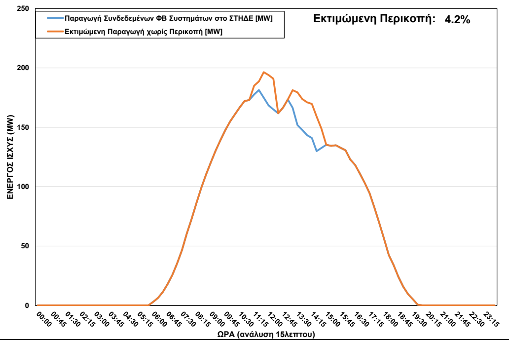
ΦΒ Παραγωγή στο ΣΤΗΔΕ κατά τη διάρκεια περικοπής στις 25/05/2023 ώρα 11:15 - 14:45
