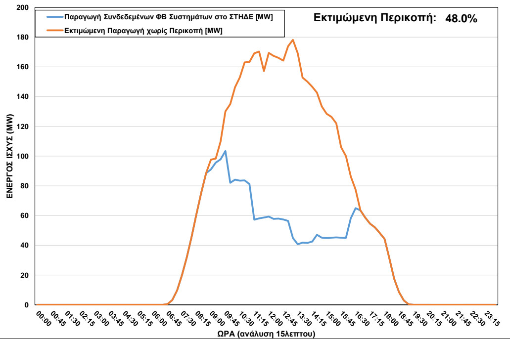
ΦΒ Παραγωγή στο ΣΤΗΔΕ κατά τη διάρκεια περικοπής στις 02/04/2023 ώρα 08:45 – 16:30
