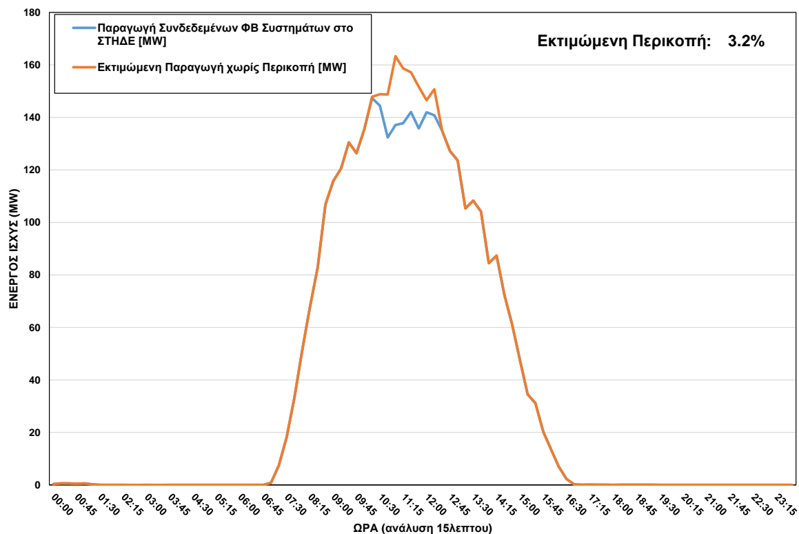
ΦΒ Παραγωγή στο ΣΤΗΔΕ κατά τη διάρκεια περικοπής στις 15/12/2023 ώρα 10:15 - 12:15
