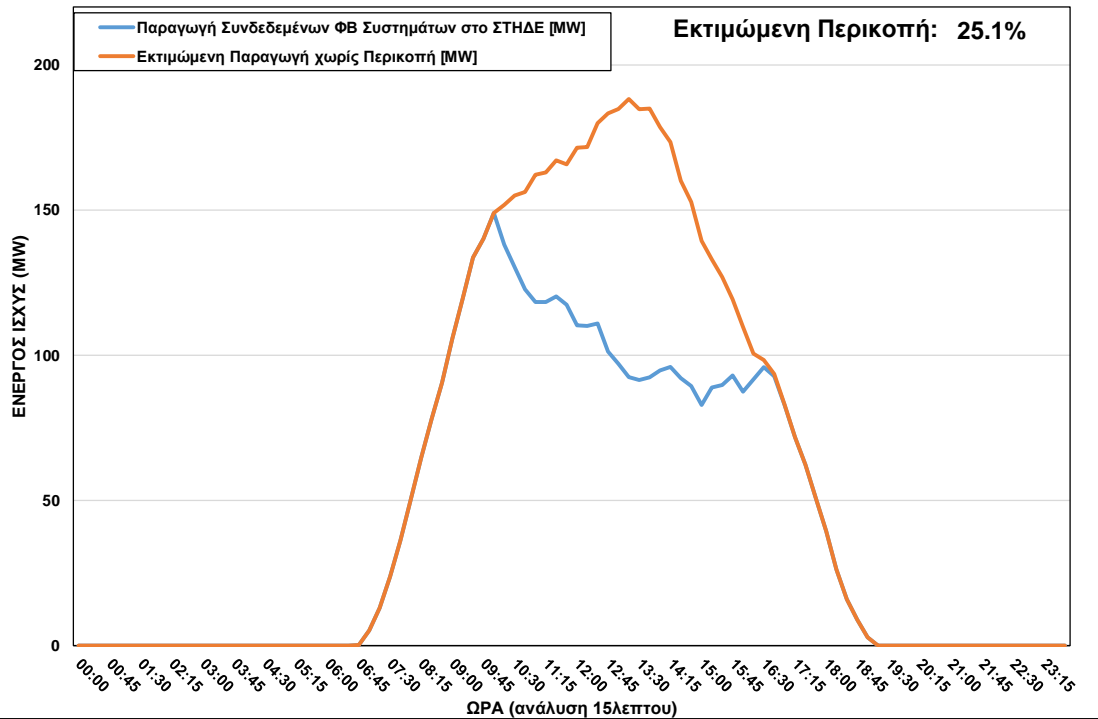
ΦΒ Παραγωγή στο ΣΤΗΔΕ κατά τη διάρκεια περικοπής στις 05/04/2023 ώρα 10:15 – 17:00
