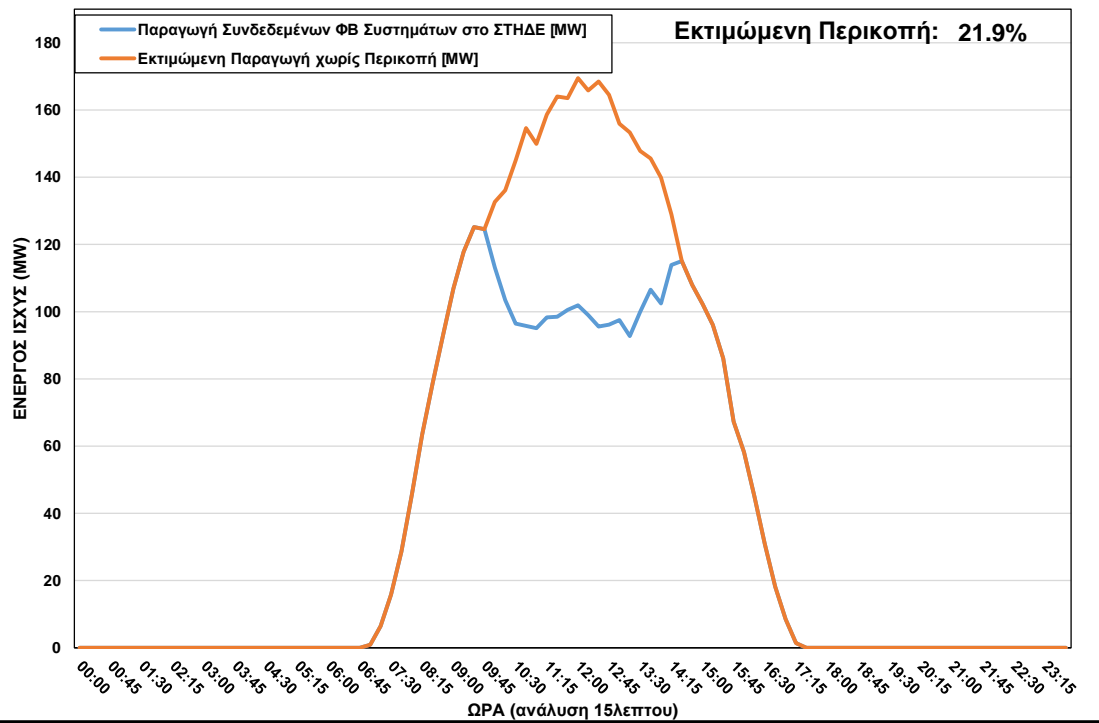
ΦΒ Παραγωγή στο ΣΤΗΔΕ κατά τη διάρκεια περικοπής στις 02/02/2023 ώρα 09:45 – 14:15
