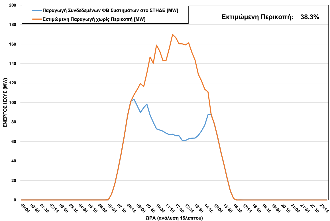
ΦΒ Παραγωγή στο ΣΤΗΔΕ κατά τη διάρκεια περικοπής στις 27/11/2023 ώρα 08:45 - 14:30
