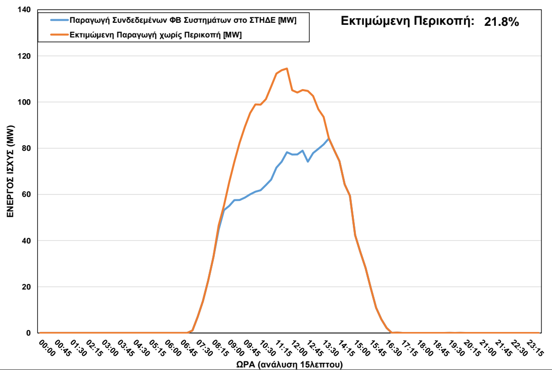
ΦΒ Παραγωγή στο ΣΤΗΔΕ κατά τη διάρκεια περικοπής στις 01/01/2023 ώρα 08:30 – 13:30
