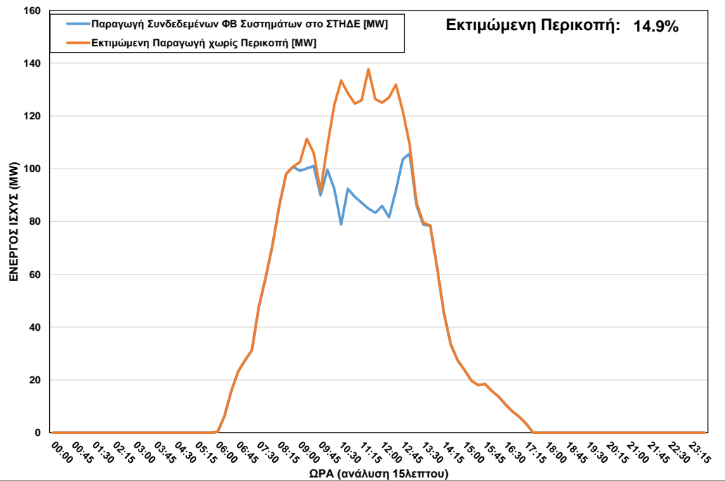
ΦΒ Παραγωγή στο ΣΤΗΔΕ κατά τη διάρκεια περικοπής στις 24/03/2023 ώρα 09:00 – 13:30
