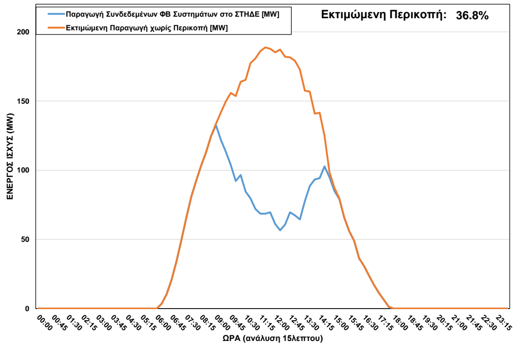
ΦΒ Παραγωγή στο ΣΤΗΔΕ κατά τη διάρκεια περικοπής στις 21/03/2023 ώρα 09:00 - 15:15
