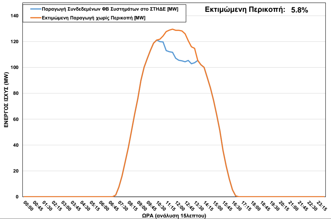
ΦΒ Παραγωγή στο ΣΤΗΔΕ κατά τη διάρκεια περικοπής στις 10/01/2023 ώρα 10:30 – 13:30
