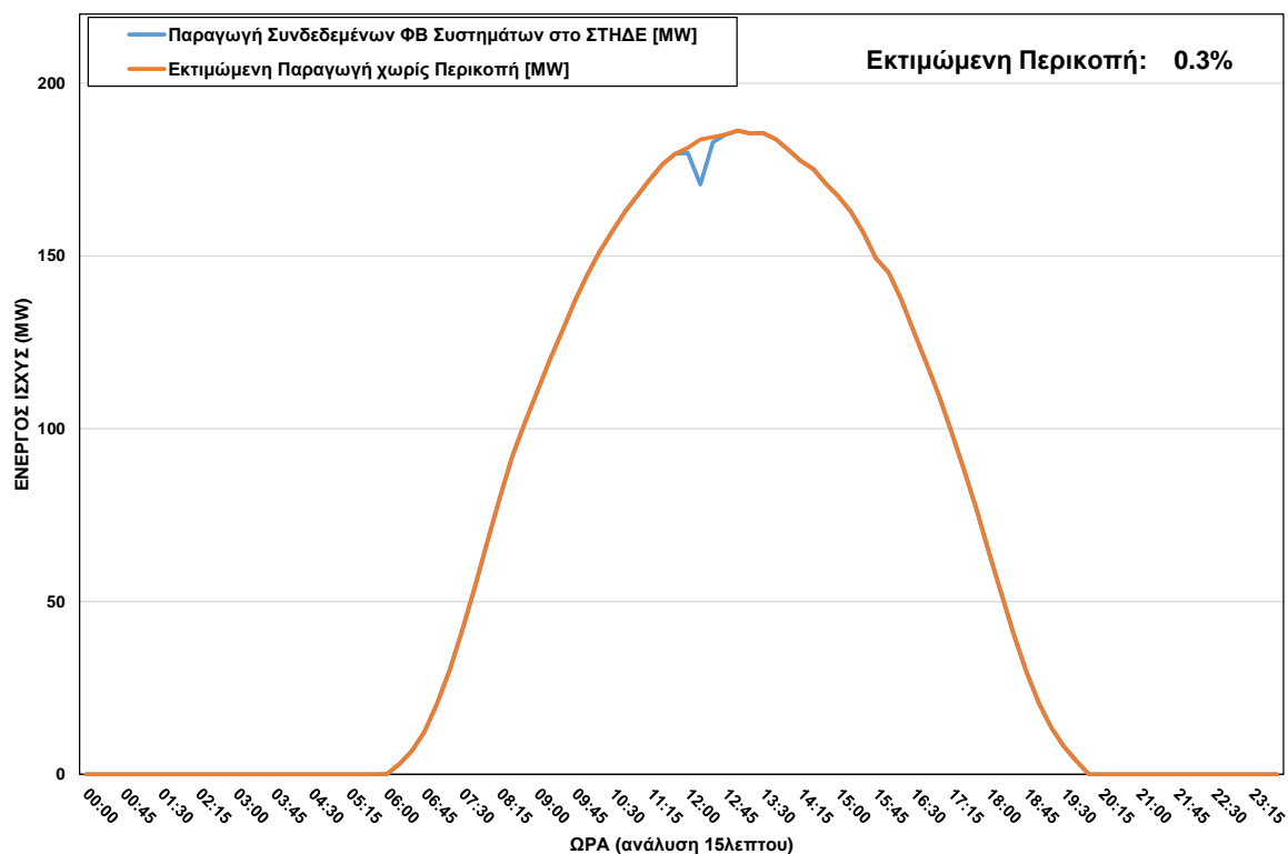
ΦΒ Παραγωγή στο ΣΤΗΔΕ κατά τη διάρκεια περικοπής στις 11/07/2023 ώρα 12:00 - 12:30
