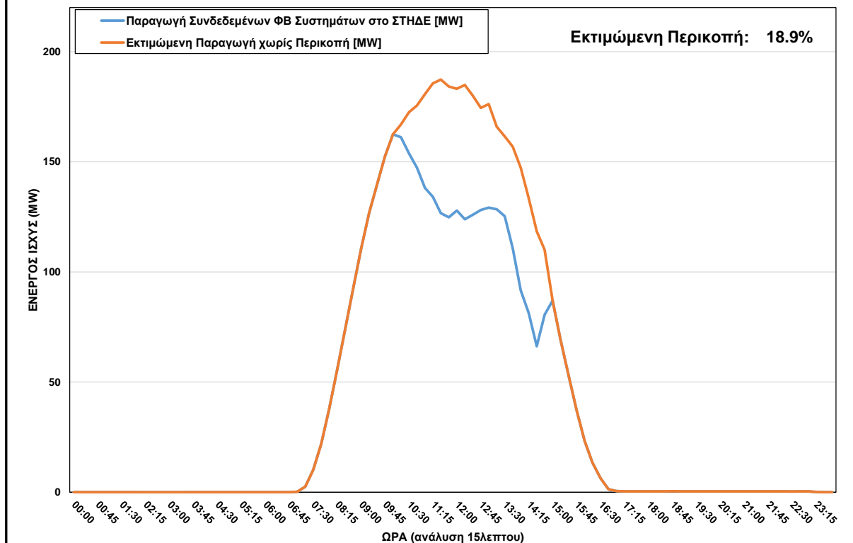
ΦΒ Παραγωγή στο ΣΤΗΔΕ κατά τη διάρκεια περικοπής στις 30/12/2023 ώρα 10:15 - 14:45
