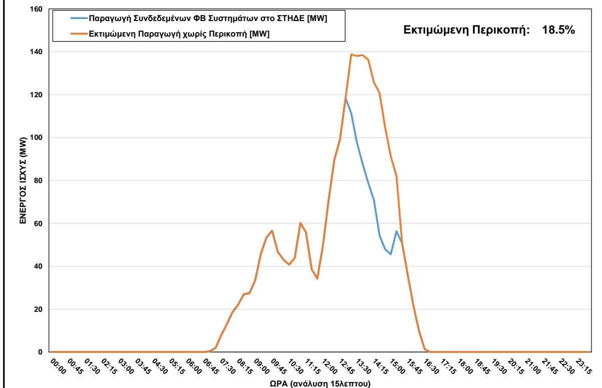
ΦΒ Παραγωγή στο ΣΤΗΔΕ κατά τη διάρκεια περικοπής στις 11/12/2023 ώρα 13:15 - 15:15
