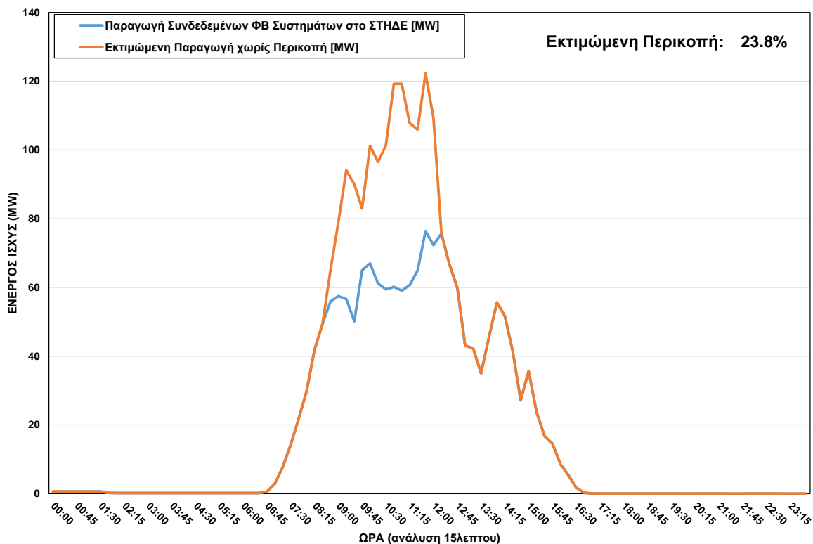
ΦΒ Παραγωγή στο ΣΤΗΔΕ κατά τη διάρκεια περικοπής στις 26/11/2023 ώρα 08:45 - 12:00
