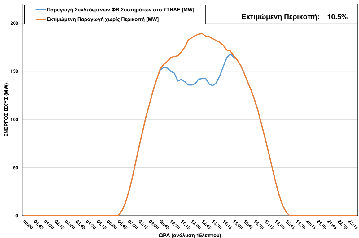
ΦΒ Παραγωγή στο ΣΤΗΔΕ κατά τη διάρκεια περικοπής στις 13/09/2023 ώρα 09:45 - 15:00
