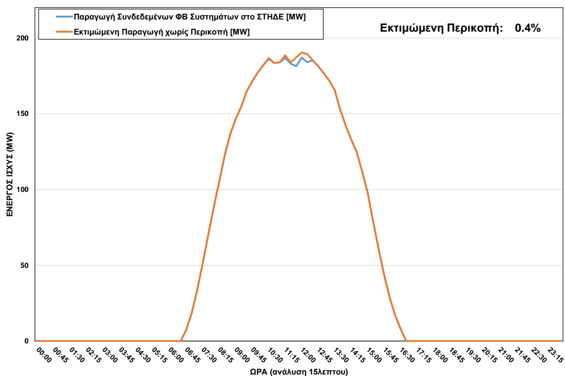
ΦΒ Παραγωγή στο ΣΤΗΔΕ κατά τη διάρκεια περικοπής στις 07/11/2023 ώρα 10:30 - 12:15
