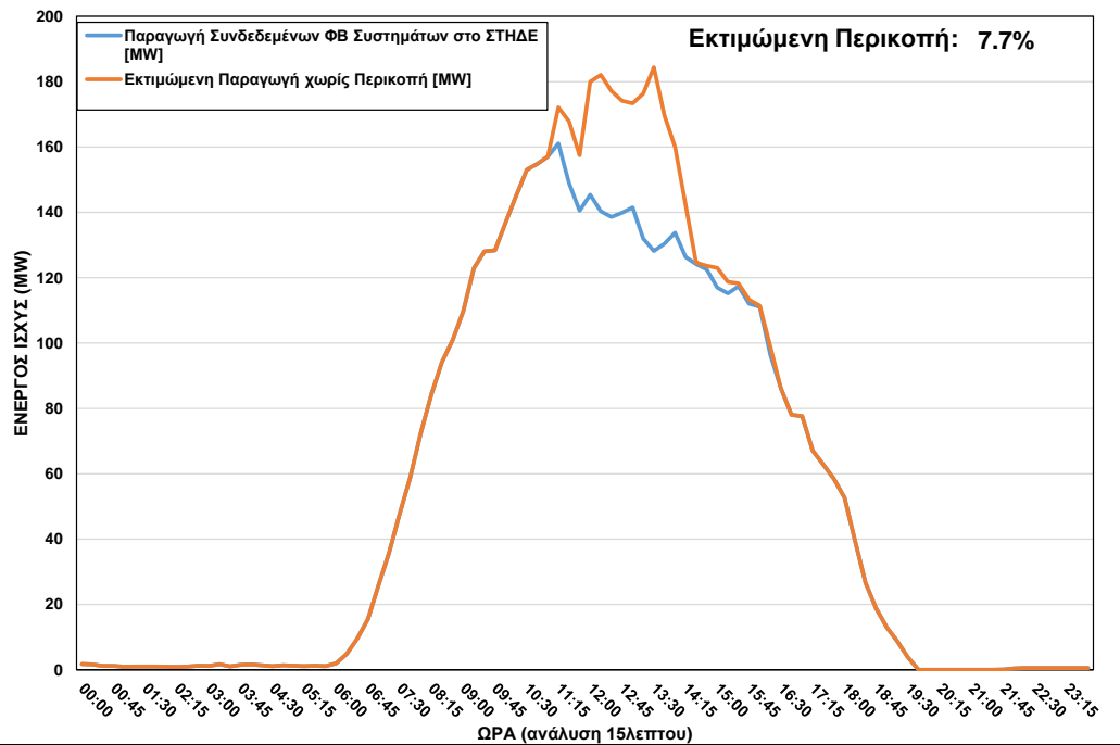
ΦΒ Παραγωγή στο ΣΤΗΔΕ κατά τη διάρκεια περικοπής στις 19/05/2023 ώρα 11:15 – 16:15
