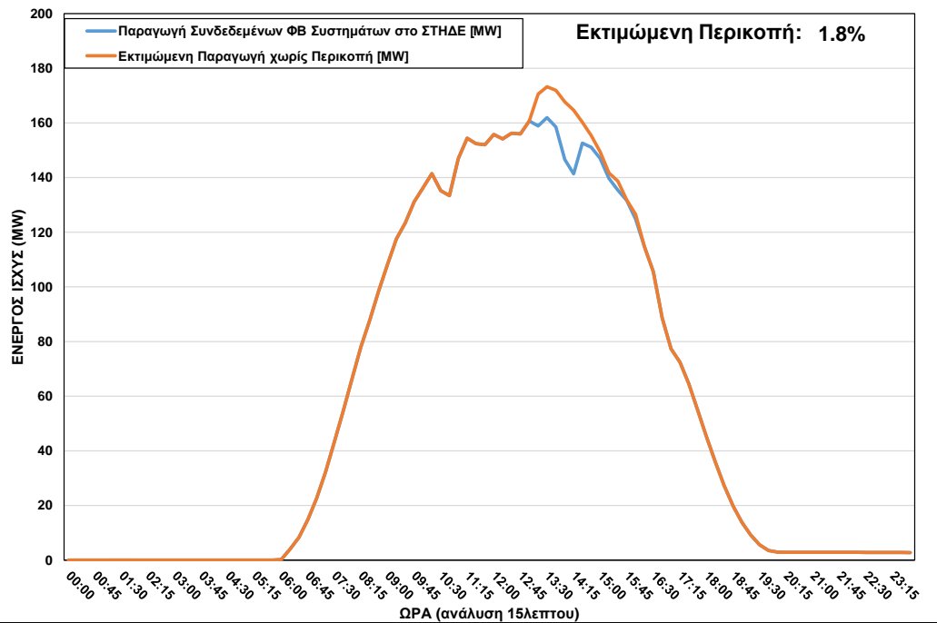
ΦΒ Παραγωγή στο ΣΤΗΔΕ κατά τη διάρκεια περικοπής στις 17/05/2023 ώρα 13:15 – 16:00
