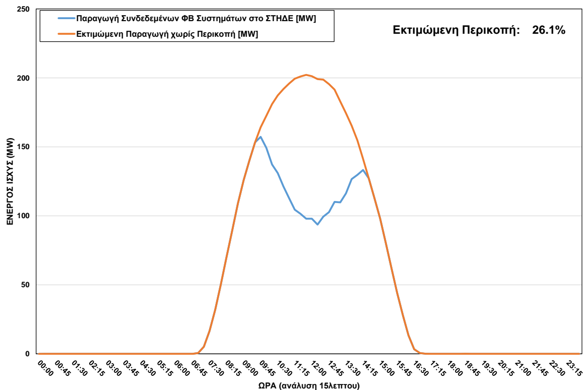
ΦΒ Παραγωγή στο ΣΤΗΔΕ κατά τη διάρκεια περικοπής στις 19/12/2023 ώρα 09:45 - 14:15
