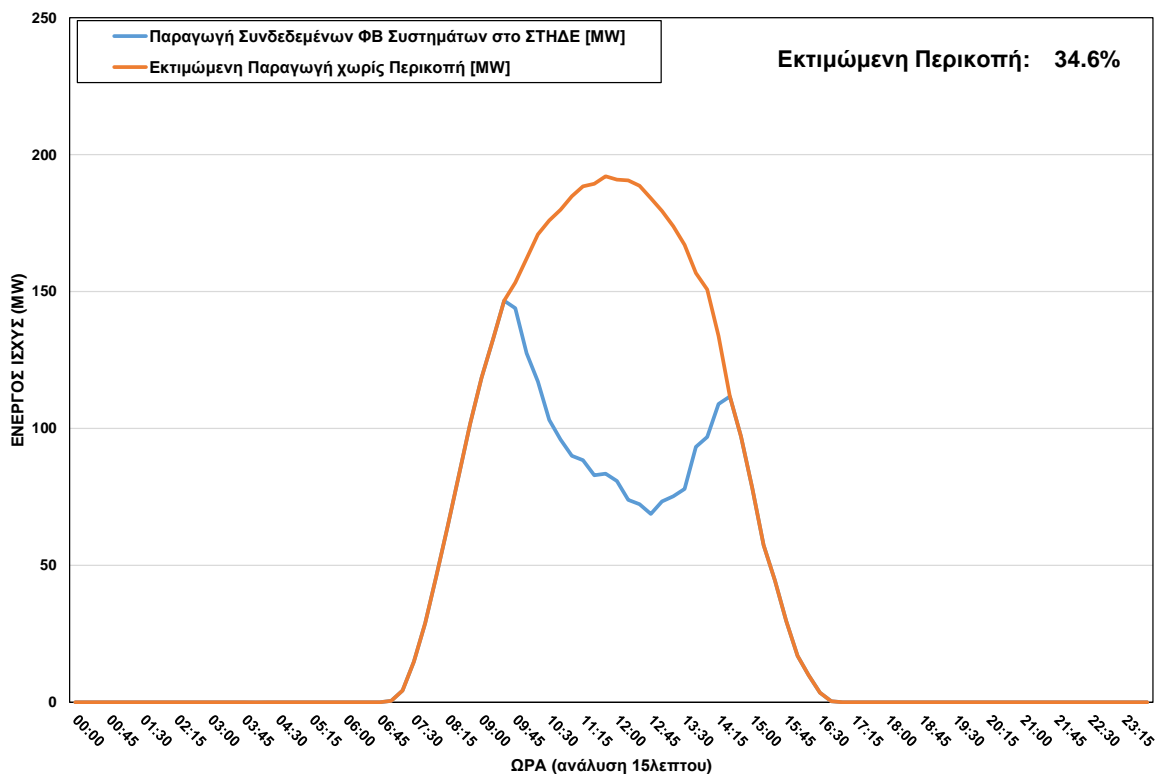
ΦΒ Παραγωγή στο ΣΤΗΔΕ κατά τη διάρκεια περικοπής στις 20/12/2023 ώρα 09:45 - 14:15
