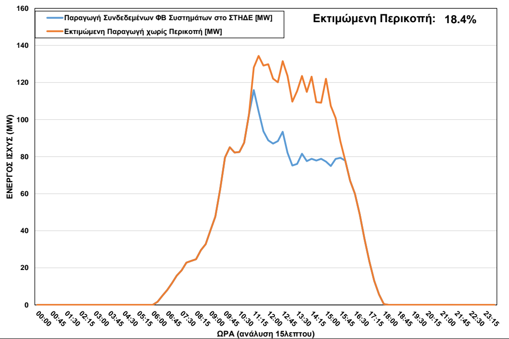
ΦΒ Παραγωγή στο ΣΤΗΔΕ κατά τη διάρκεια περικοπής στις 25/03/2023 ώρα 11:15 – 15:45
