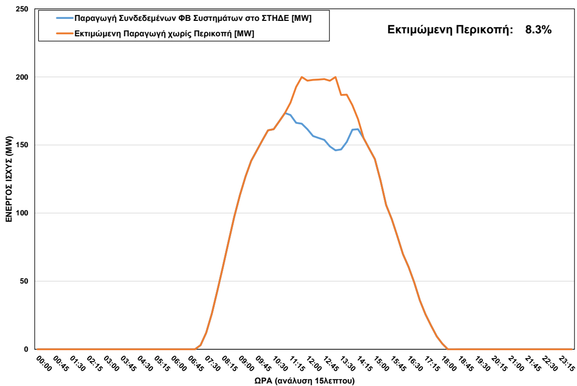
ΦΒ Παραγωγή στο ΣΤΗΔΕ κατά τη διάρκεια περικοπής στις 17/10/2023 ώρα 11:15 - 14:15
