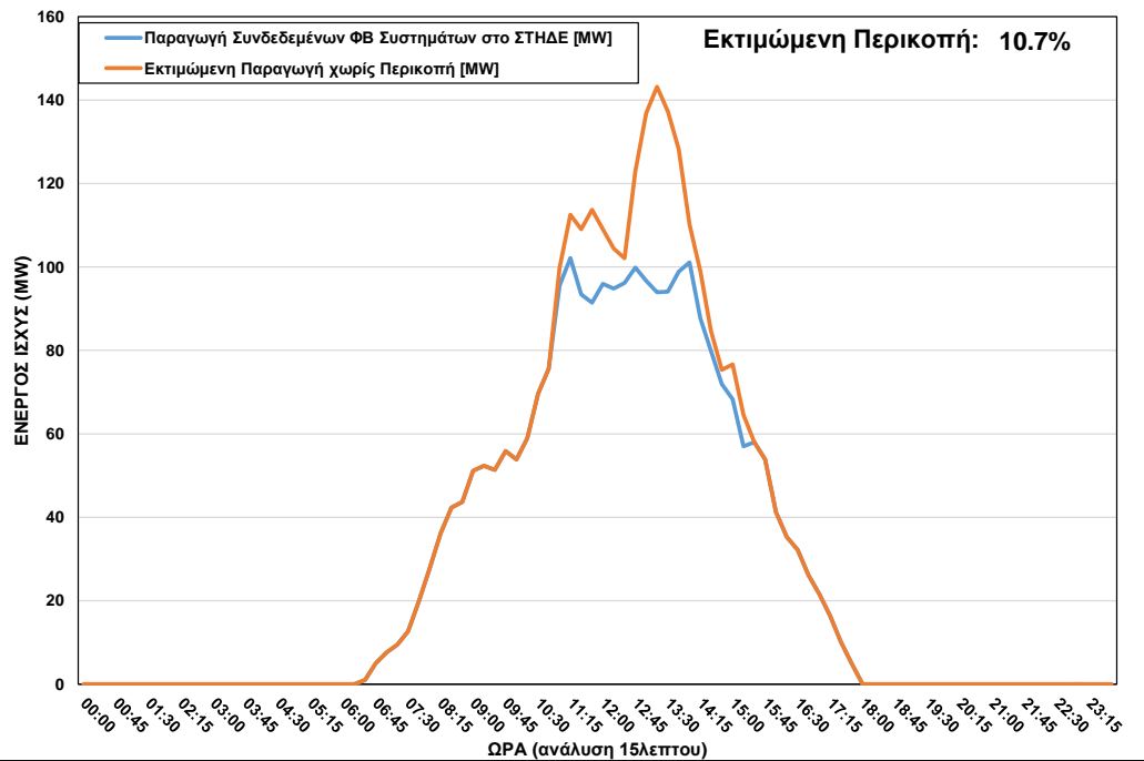
ΦΒ Παραγωγή στο ΣΤΗΔΕ κατά τη διάρκεια περικοπής στις 23/03/2023 ώρα 11:00 – 15:15
