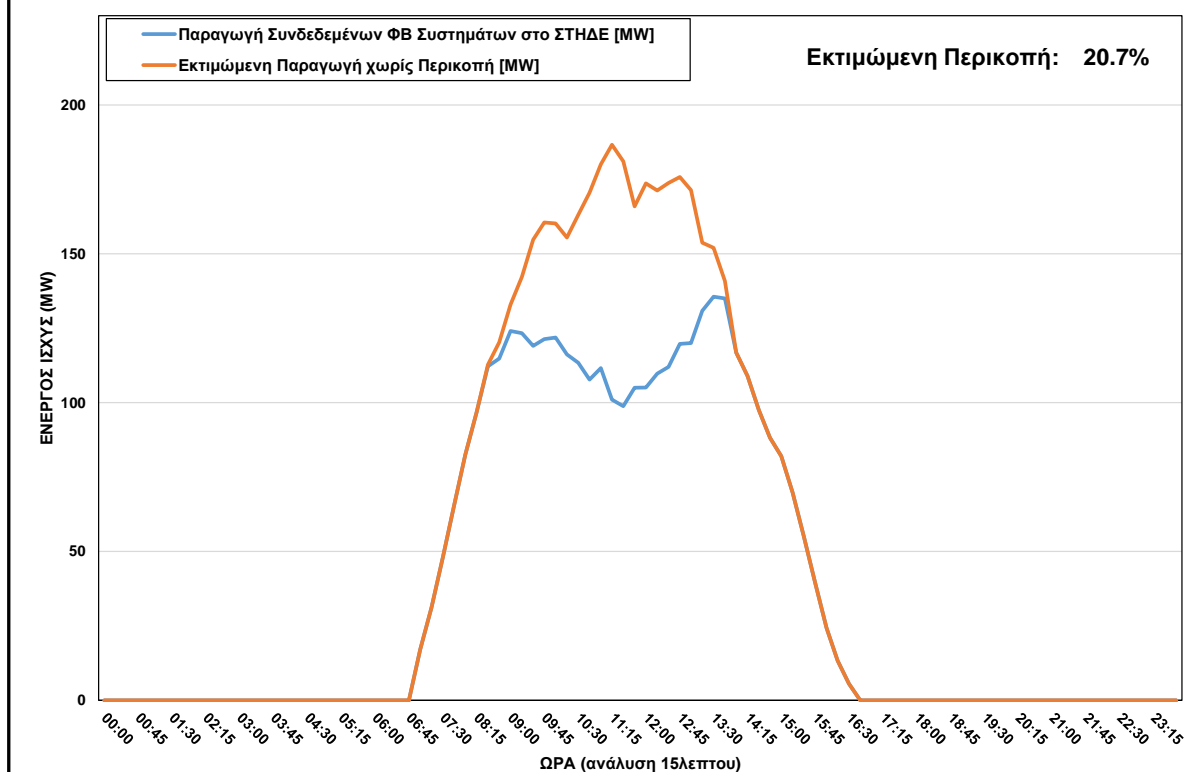
ΦΒ Παραγωγή στο ΣΤΗΔΕ κατά τη διάρκεια περικοπής στις 08/11/2023 ώρα 08:30 - 13:45
