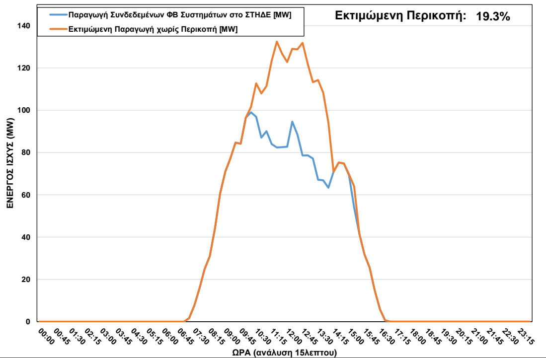
ΦΒ Παραγωγή στο ΣΤΗΔΕ κατά τη διάρκεια περικοπής στις 02/01/2023 ώρα 10:00 – 15:15
