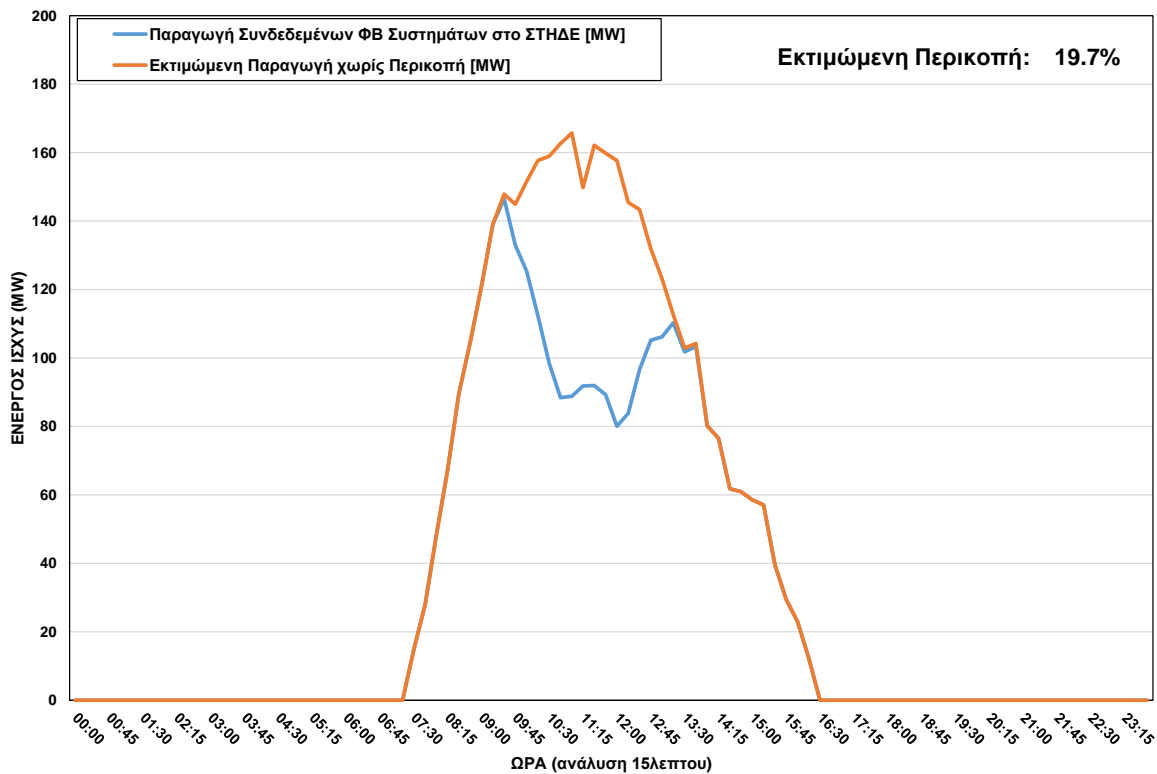
ΦΒ Παραγωγή στο ΣΤΗΔΕ κατά τη διάρκεια περικοπής στις 09/12/2023 ώρα 09:30 - 13:45
