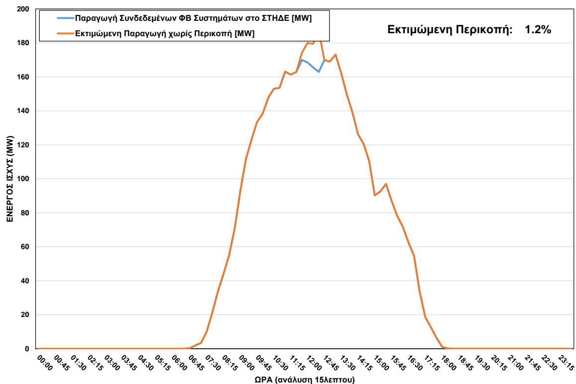
ΦΒ Παραγωγή στο ΣΤΗΔΕ κατά τη διάρκεια περικοπής στις 26/10/2023 ώρα 11:45 - 12:30
