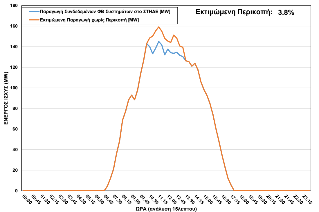
ΦΒ Παραγωγή στο ΣΤΗΔΕ κατά τη διάρκεια περικοπής στις 15/02/2023 ώρα 10:15 – 13:15
