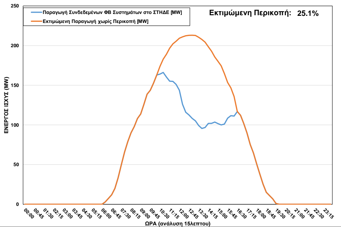
ΦΒ Παραγωγή στο ΣΤΗΔΕ κατά τη διάρκεια περικοπής στις 04/05/2023 ώρα 10:30 – 16:15
