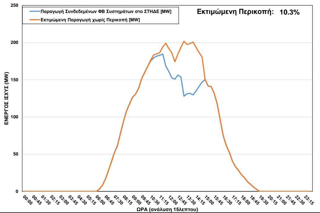
ΦΒ Παραγωγή στο ΣΤΗΔΕ κατά τη διάρκεια περικοπής στις 11/05/2023 ώρα 10:30 - 14:45
