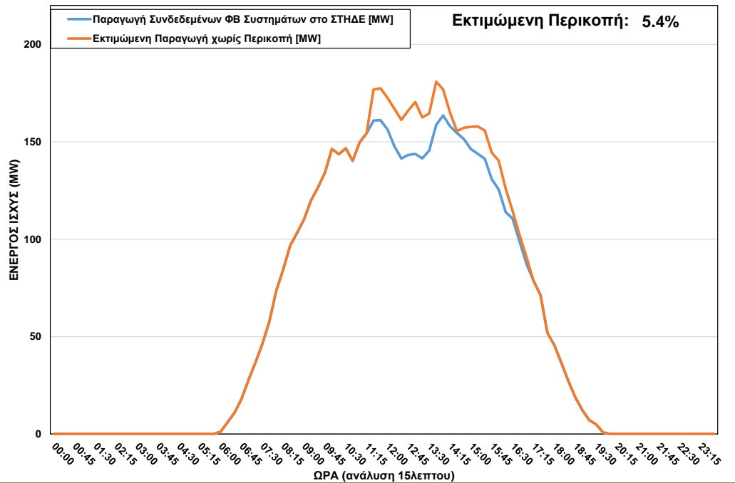
ΦΒ Παραγωγή στο ΣΤΗΔΕ κατά τη διάρκεια περικοπής στις 31/05/2023 ώρα 11:30 – 17:00
