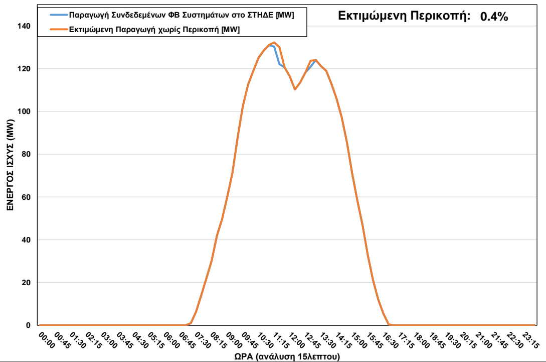
ΦΒ Παραγωγή στο ΣΤΗΔΕ κατά τη διάρκεια περικοπής στις 03/01/2023 ώρα 11:00 – 13:00
