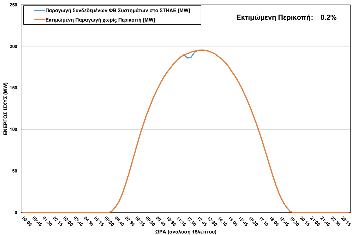
ΦΒ Παραγωγή στο ΣΤΗΔΕ κατά τη διάρκεια περικοπής στις 12/08/2023 ώρα 11:45 - 12:15
