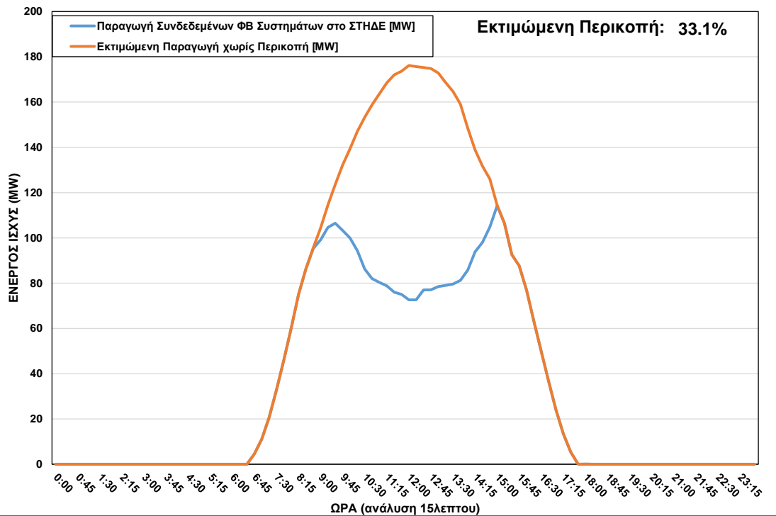
ΦΒ Παραγωγή στο ΣΤΗΔΕ κατά τη διάρκεια περικοπής στις 03-03-23 ώρα 8:45 - 14:45
