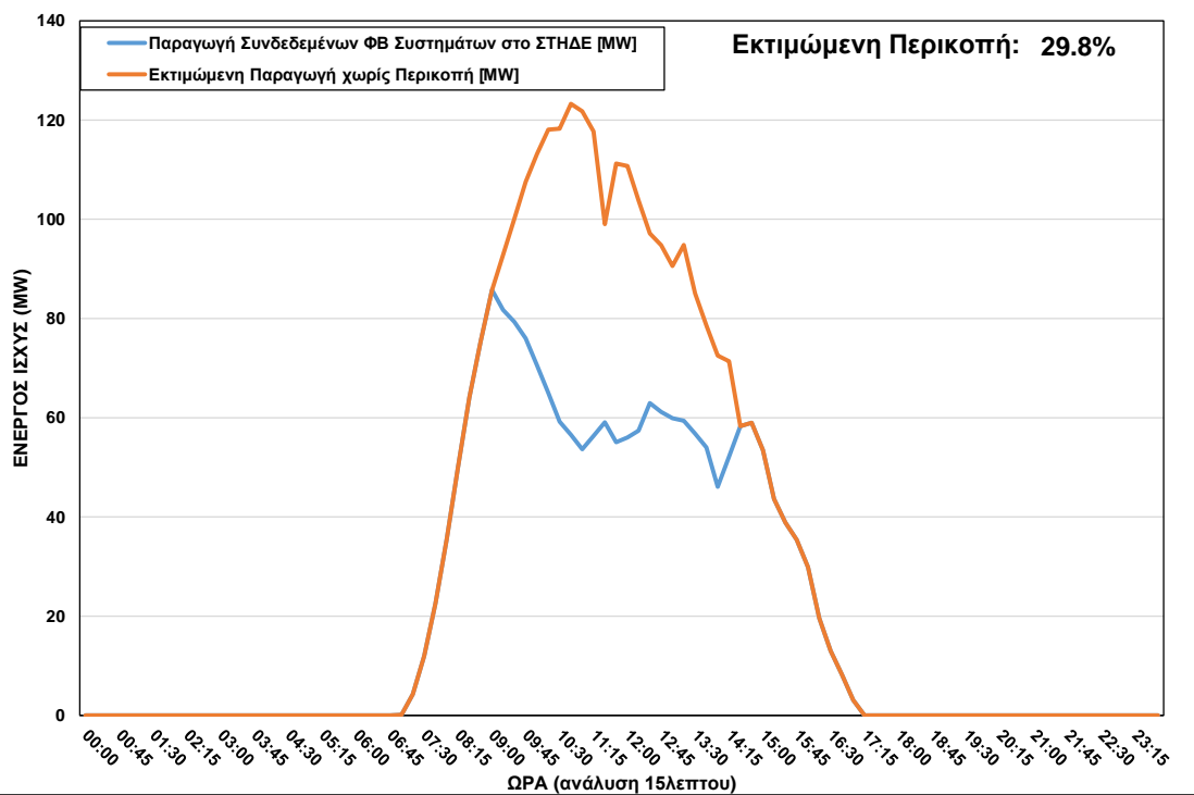
ΦΒ Παραγωγή στο ΣΤΗΔΕ κατά τη διάρκεια περικοπής στις 29/01/2023 ώρα 09:00 – 14:15
