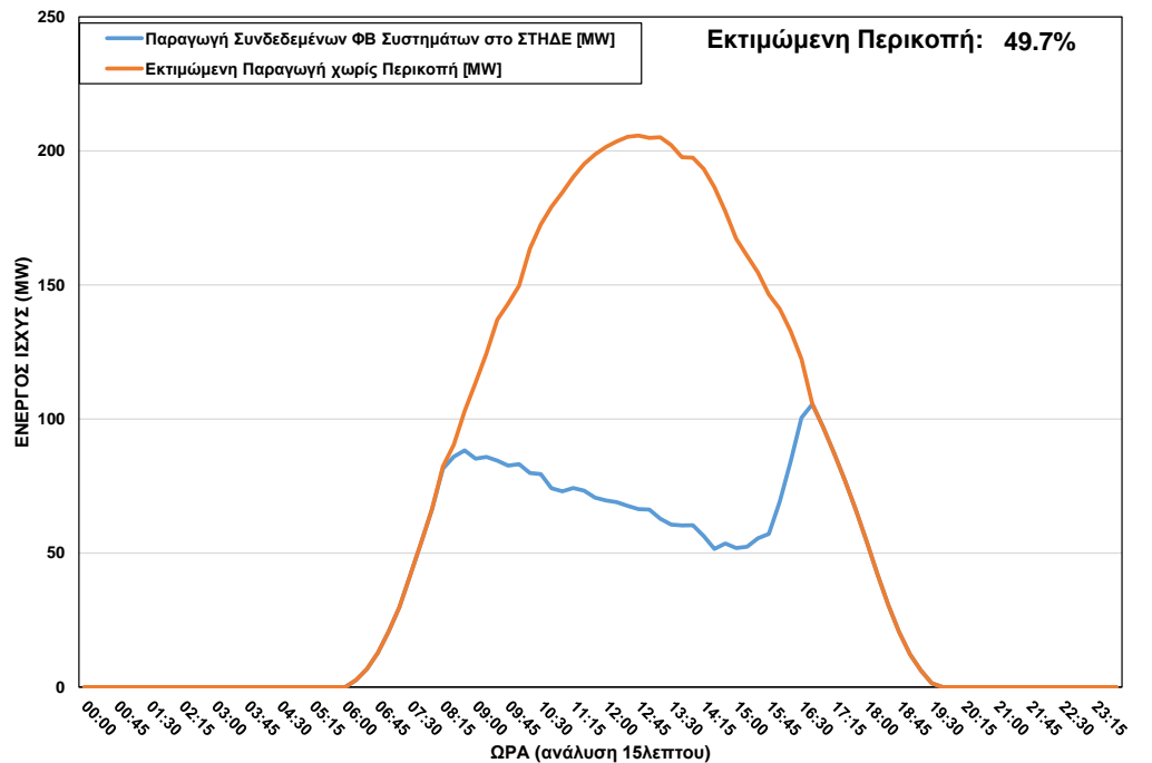
ΦΒ Παραγωγή στο ΣΤΗΔΕ κατά τη διάρκεια περικοπής στις 14/05/2023 ώρα 08:15 – 16:30
