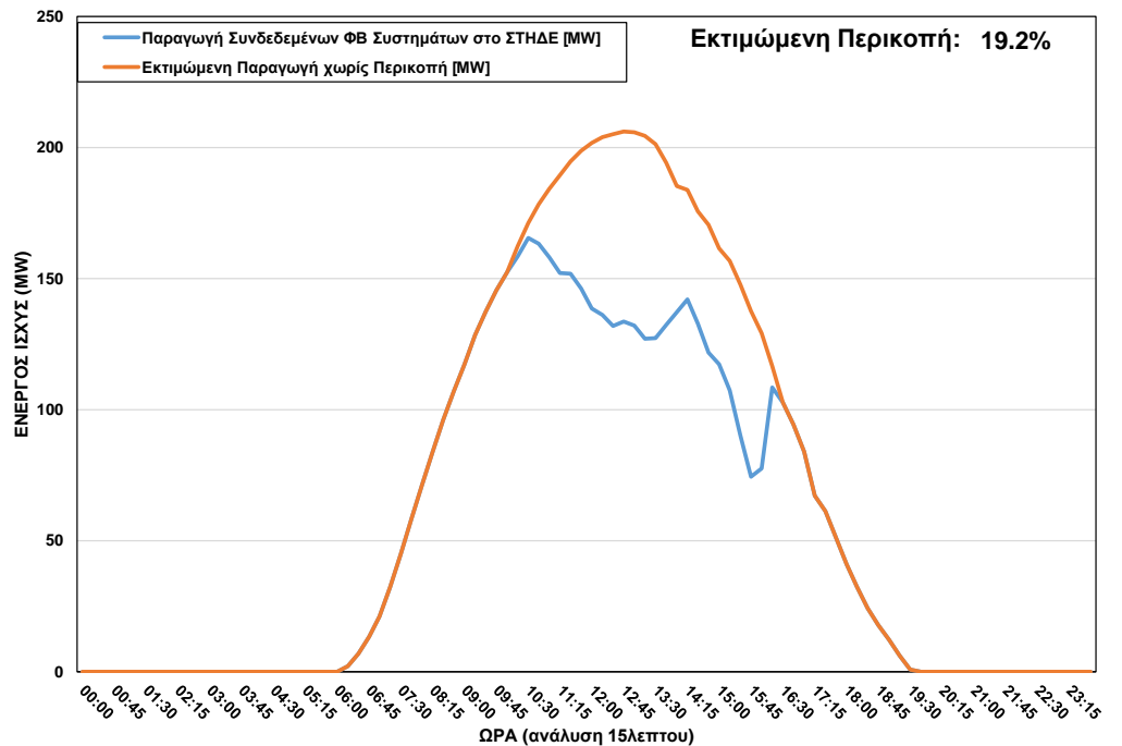
ΦΒ Παραγωγή στο ΣΤΗΔΕ κατά τη διάρκεια περικοπής στις 10/05/2023 ώρα 10:15 – 16:15
