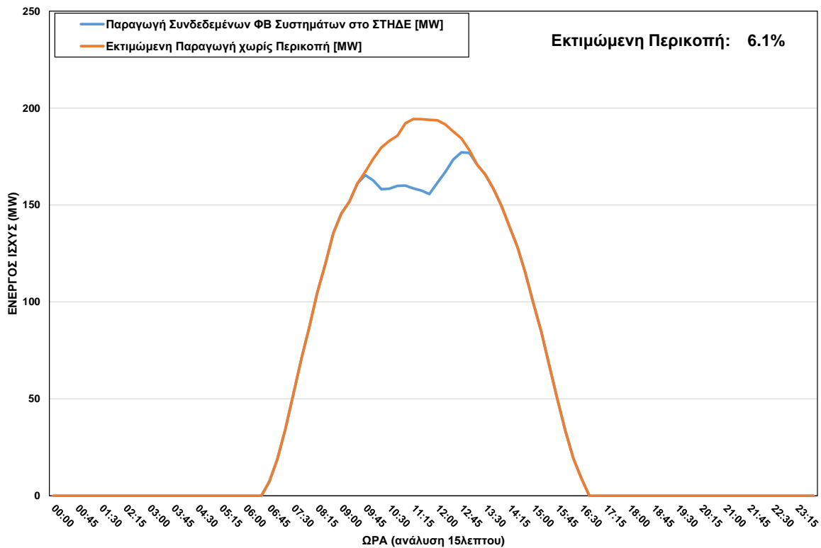
ΦΒ Παραγωγή στο ΣΤΗΔΕ κατά τη διάρκεια περικοπής στις 06/11/2023 ώρα 09:45 - 13:00
