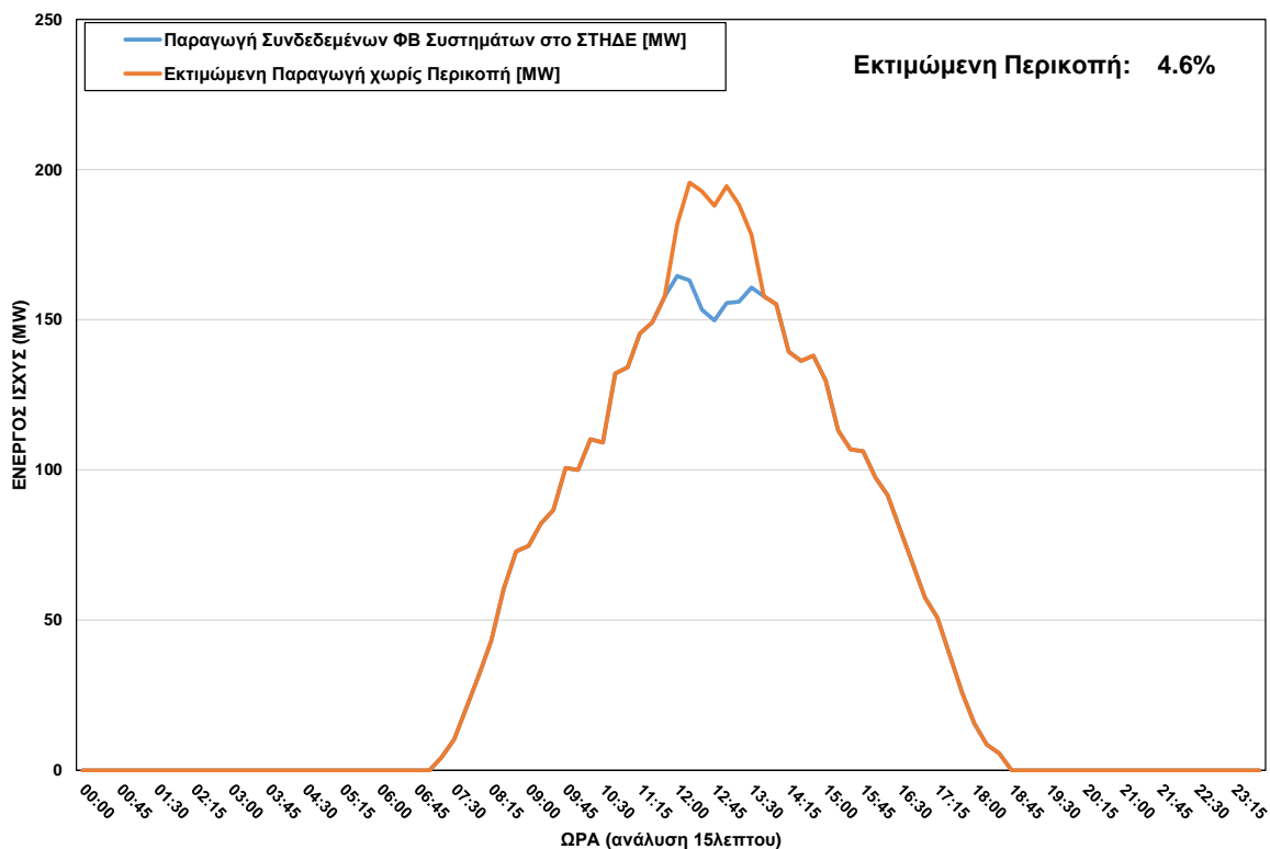
ΦΒ Παραγωγή στο ΣΤΗΔΕ κατά τη διάρκεια περικοπής στις 05/10/2023 ώρα 12:00 - 13:30
