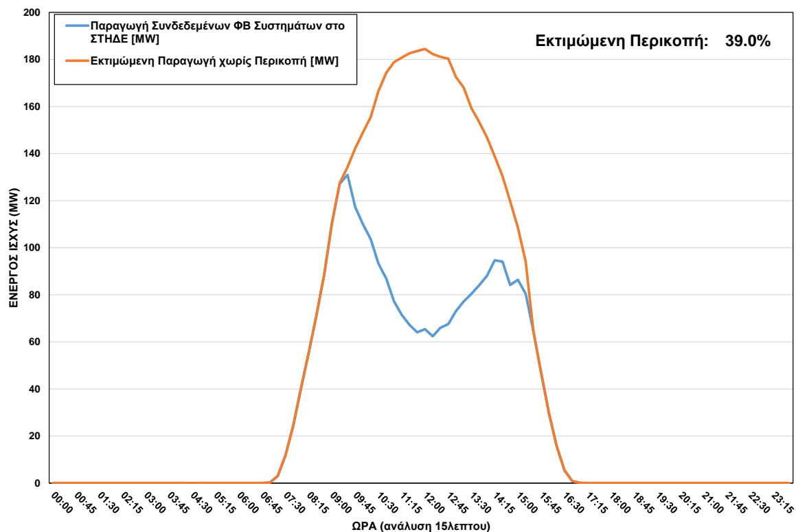
Φ/Β Παραγωγή στο ΣΤΗΔΕ κατά τη διάρκεια περικοπής στις 26/12/2023 ώρα 09:15 - 15:15
