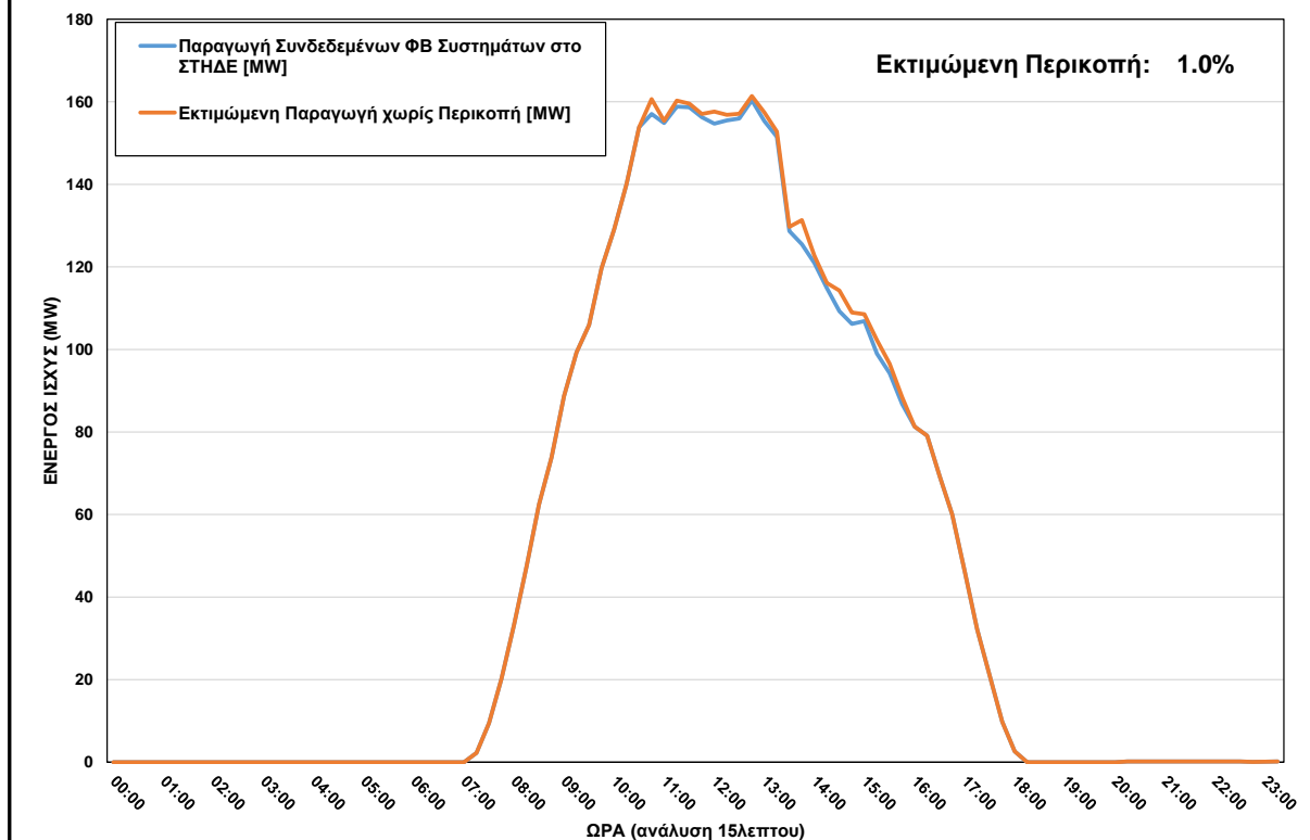
ΦΒ Παραγωγή στο ΣΤΗΔΕ κατά τη διάρκεια περικοπής στις 14/10/2023 ώρα 10:45 - 15:45
