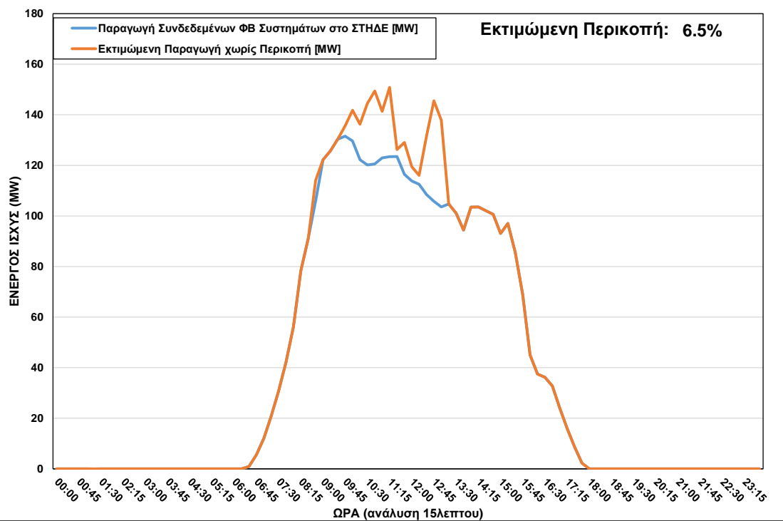
ΦΒ Παραγωγή στο ΣΤΗΔΕ κατά τη διάρκεια περικοπής στις 08/03/2023 ώρα 08:45 – 13:00
