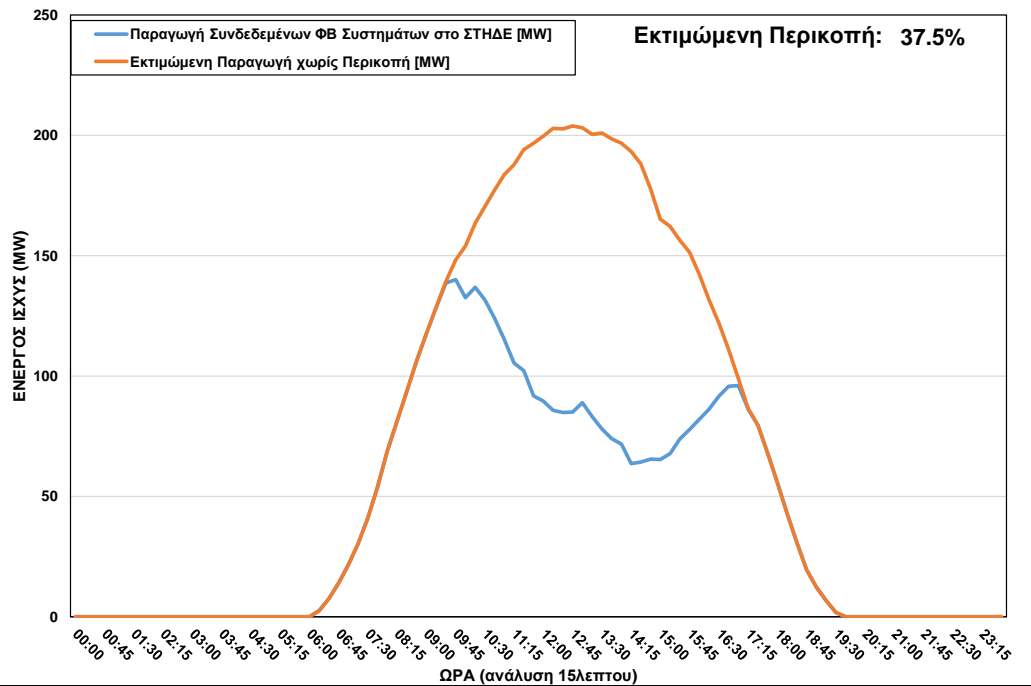
ΦΒ Παραγωγή στο ΣΤΗΔΕ κατά τη διάρκεια περικοπής στις 13/05/2023 ώρα 09:30 – 17:15
