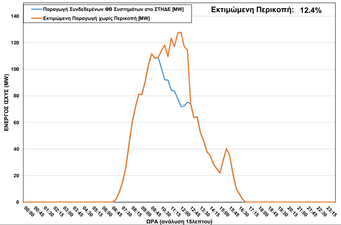
ΦΒ Παραγωγή στο ΣΤΗΔΕ κατά τη διάρκεια περικοπής στις 03/02/2023 ώρα 10:15 – 12:30
