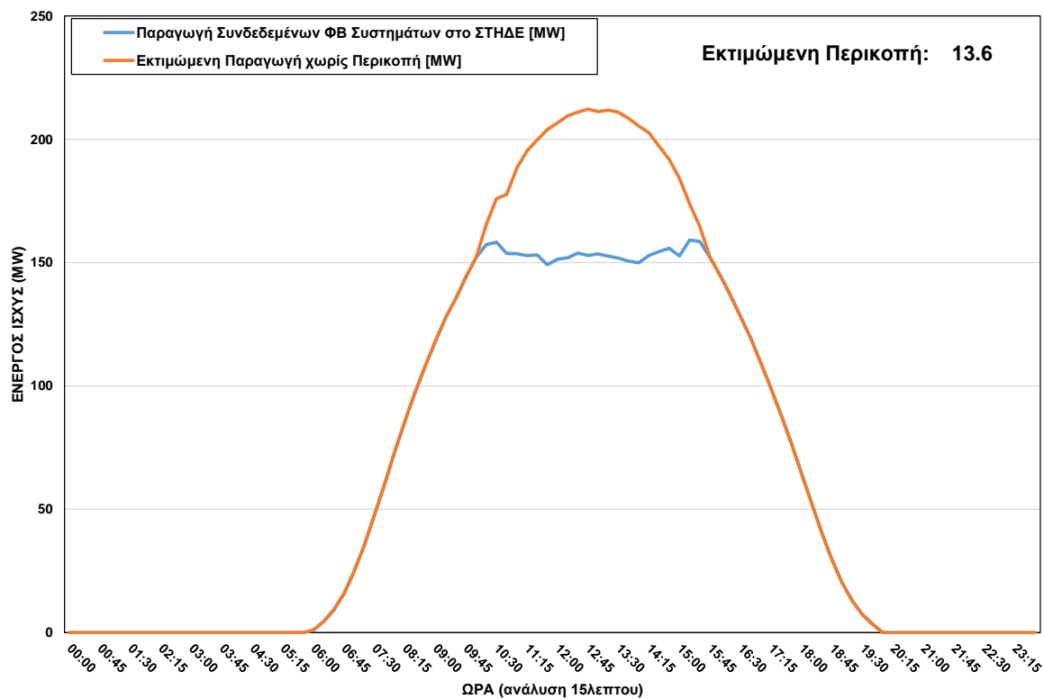
ΦΒ Παραγωγή στο ΣΤΗΔΕ κατά τη διάρκεια περικοπής στις 25/06/2023 ώρα 10:15 - 15:30
