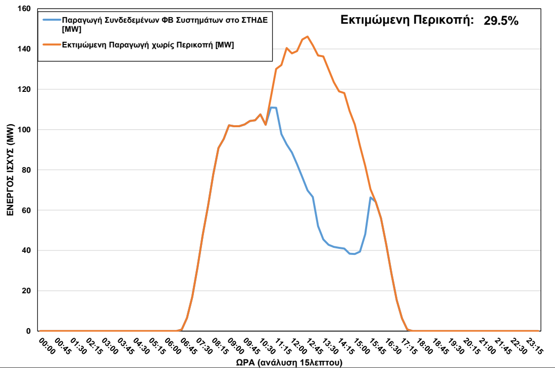
ΦΒ Παραγωγή στο ΣΤΗΔΕ κατά τη διάρκεια περικοπής στις 18/02/2023 ώρα 11:00 – 15:45
