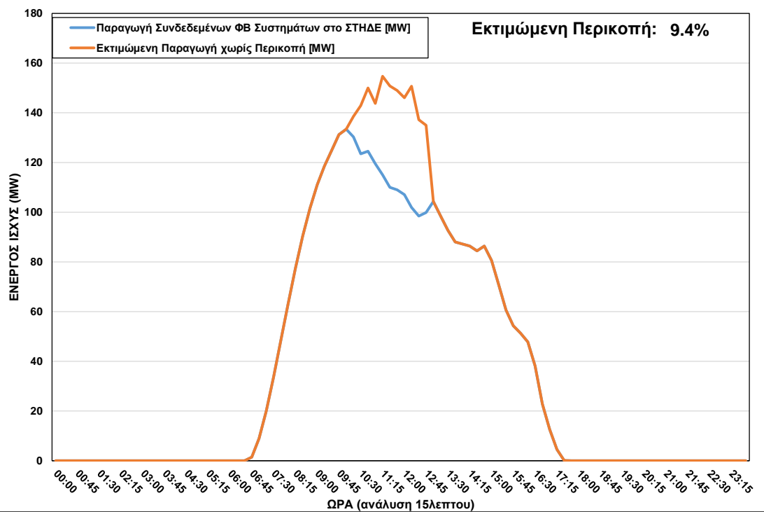
ΦΒ Παραγωγή στο ΣΤΗΔΕ κατά τη διάρκεια περικοπής στις 25/02/2023 ώρα 10:00 – 12:45
