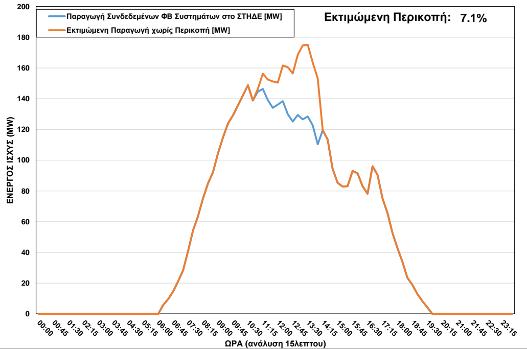
ΦΒ Παραγωγή στο ΣΤΗΔΕ κατά τη διάρκεια περικοπής στις 29/05/2023 ώρα 11:00 – 14:00
