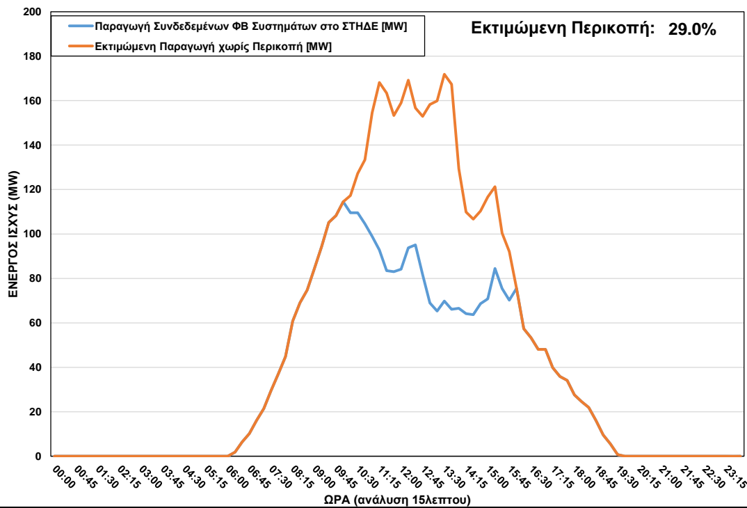
ΦΒ Παραγωγή στο ΣΤΗΔΕ κατά τη διάρκεια περικοπής στις 06/05/2023 ώρα 10:15 – 15:45
