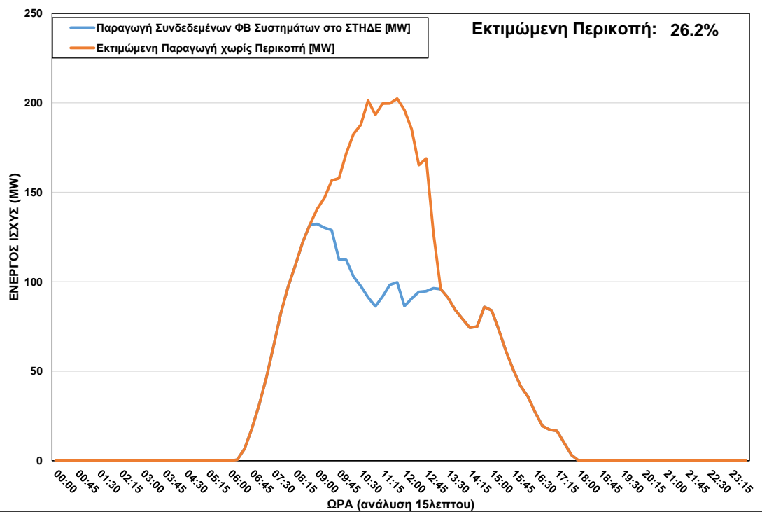
ΦΒ Παραγωγή στο ΣΤΗΔΕ κατά τη διάρκεια περικοπής στις 16/03/2023 ώρα 09:00 – 13:00
