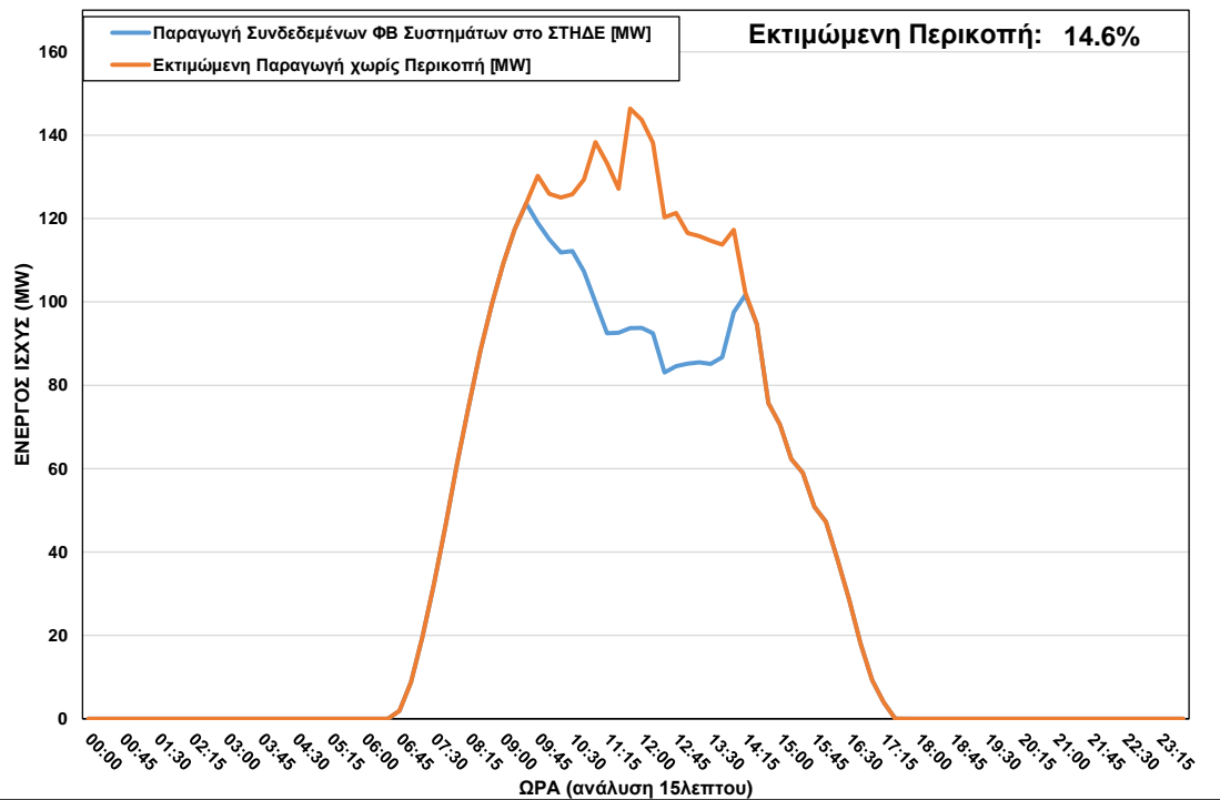
ΦΒ Παραγωγή στο ΣΤΗΔΕ κατά τη διάρκεια περικοπής στις 24/02/2023 ώρα 09:30 – 14:15
