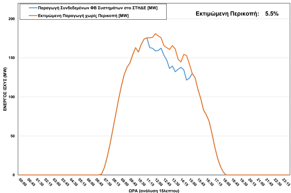
ΦΒ Παραγωγή στο ΣΤΗΔΕ κατά τη διάρκεια περικοπής στις 18/10/2023 ώρα 11:15 - 15:00
