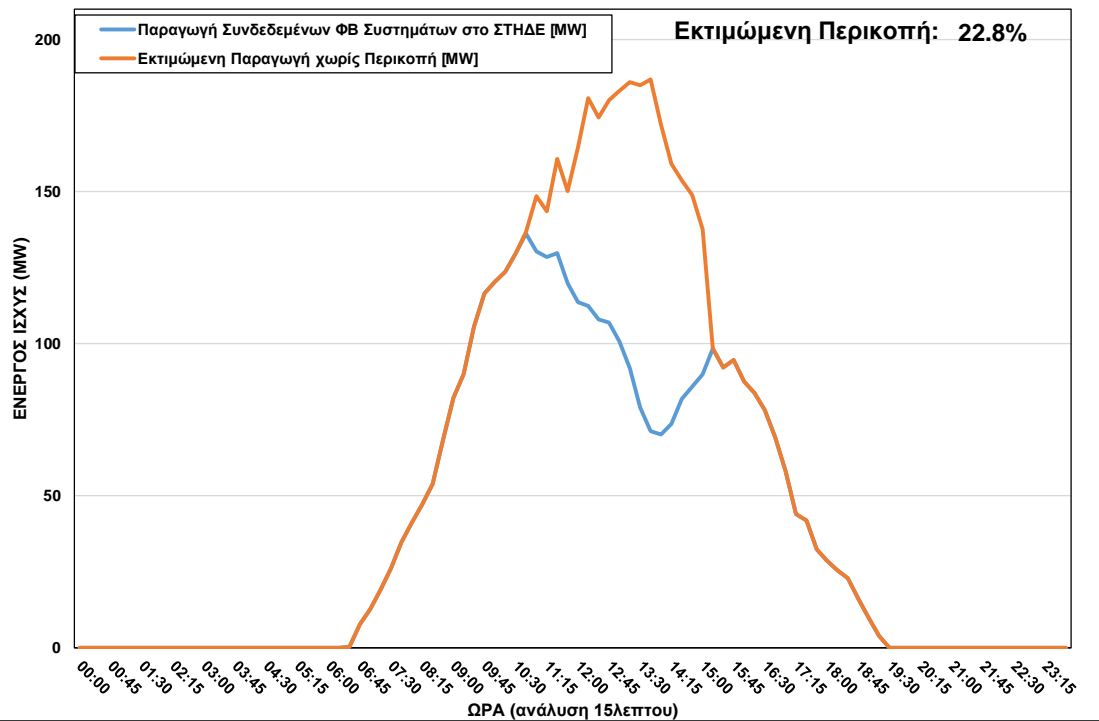
ΦΒ Παραγωγή στο ΣΤΗΔΕ κατά τη διάρκεια περικοπής στις 22/04/2023 ώρα 10:45 – 15:00
